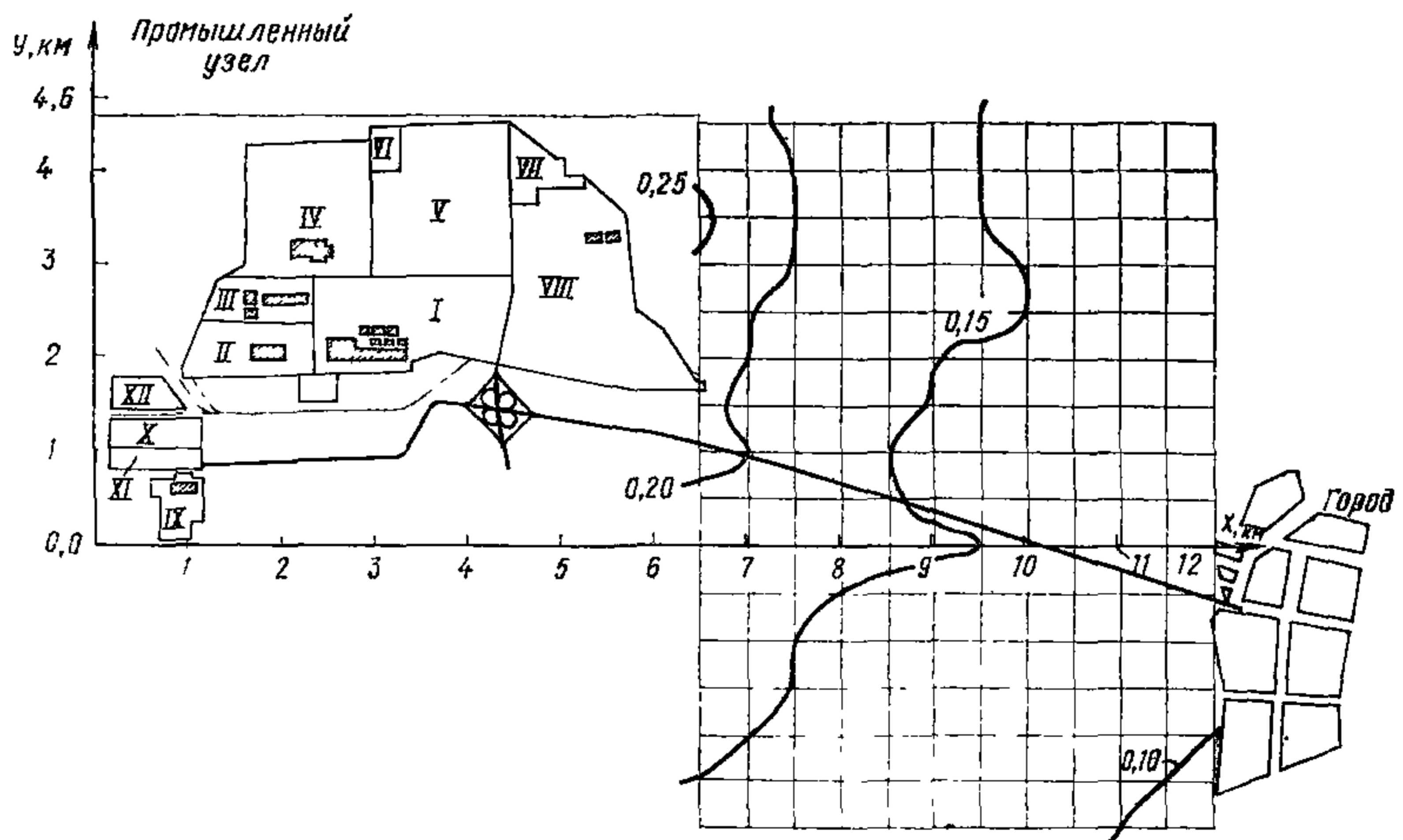
Рис. 4. Распространение сернистого ангидрида между промышленным узлом и городом, \text{мг/м}^3 \text{ПДК}=0.5 \text{ мг/м}^3 ; C_{\text{max}}=0.26 \text{ мг/м}^3
