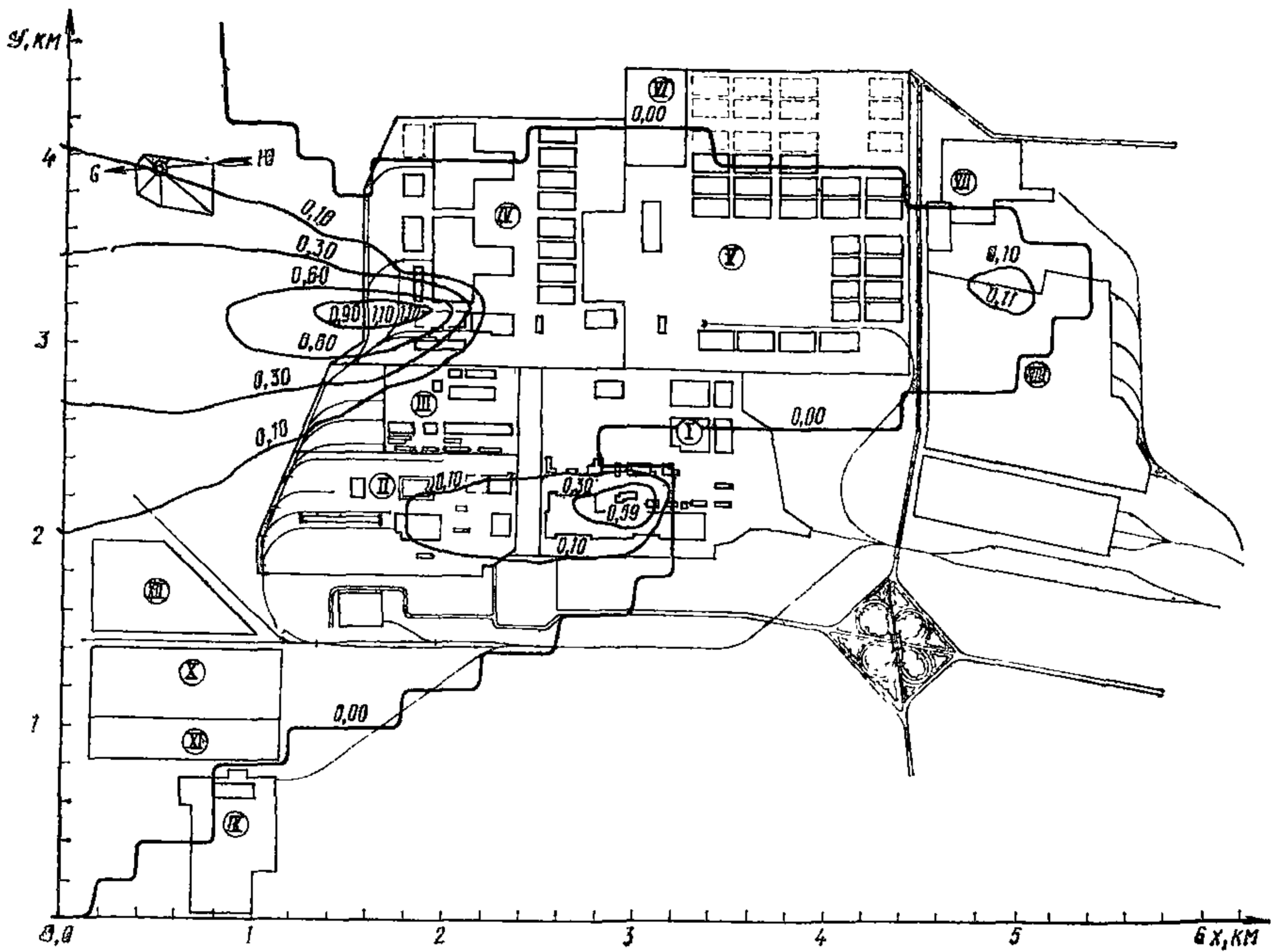
Рис. 3. Распространение сернистого ангидрида на территории промышленного узла, \text{мг/м}^3 \text{ПДК}=3.0 \text{ мг/м}^3 ; C_{\text{max}}=1.10 \text{ мг/м}^3
