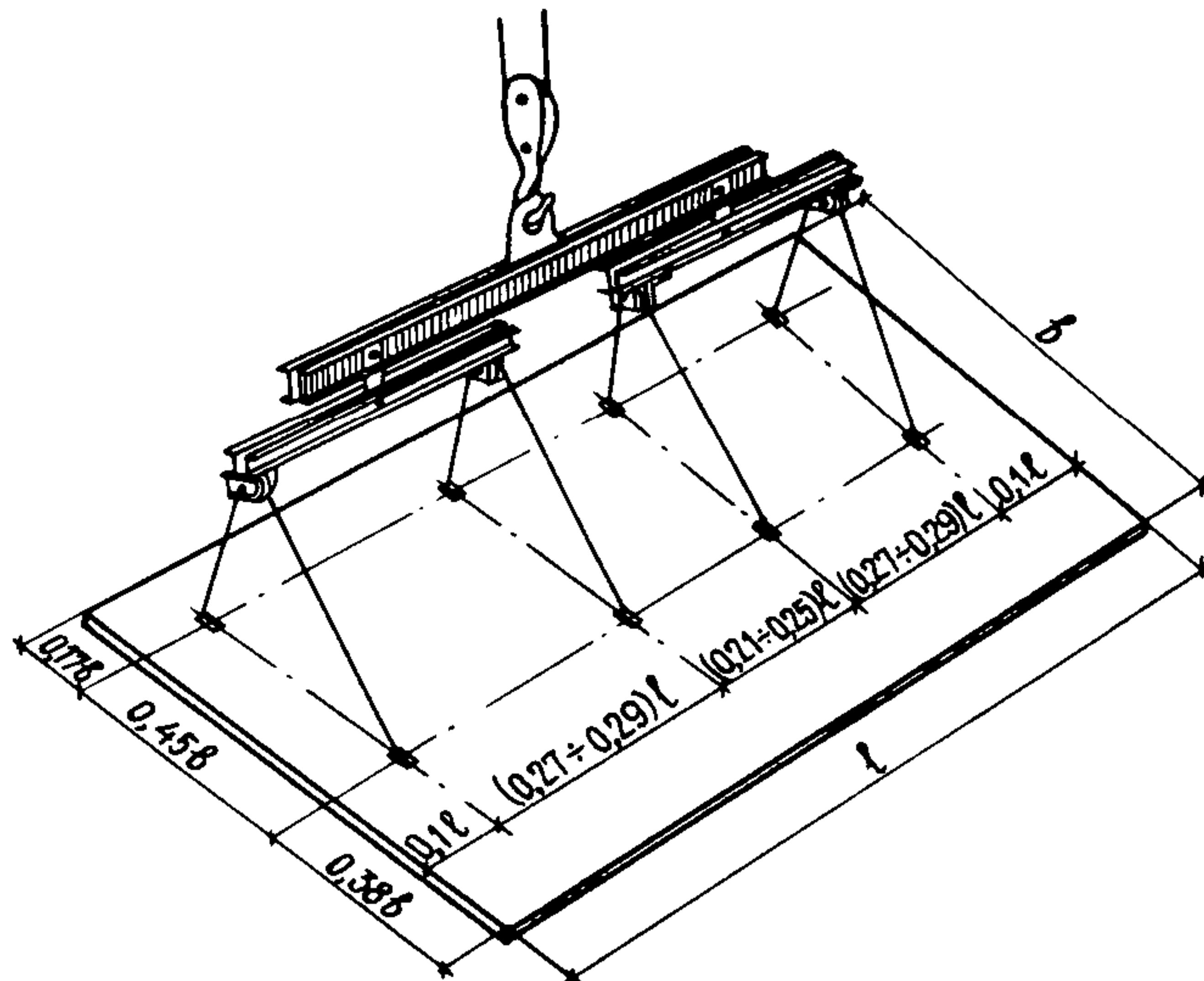
Рис.2. Монтажная схема панели основания пола
