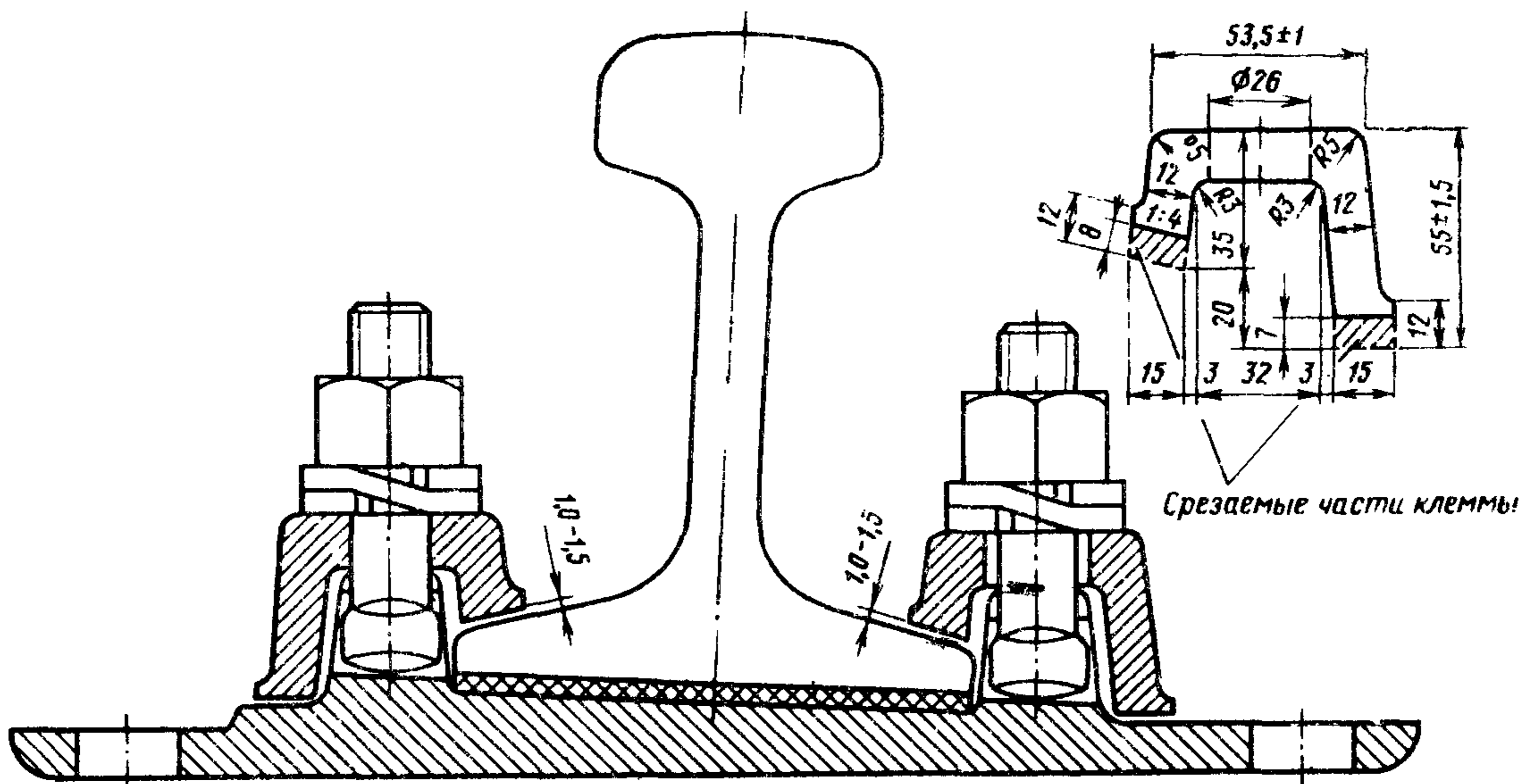
Рис. 19. Раздельное клеммно-шурупное крепление рельсов на мостах (с подрезанными клеммами)
