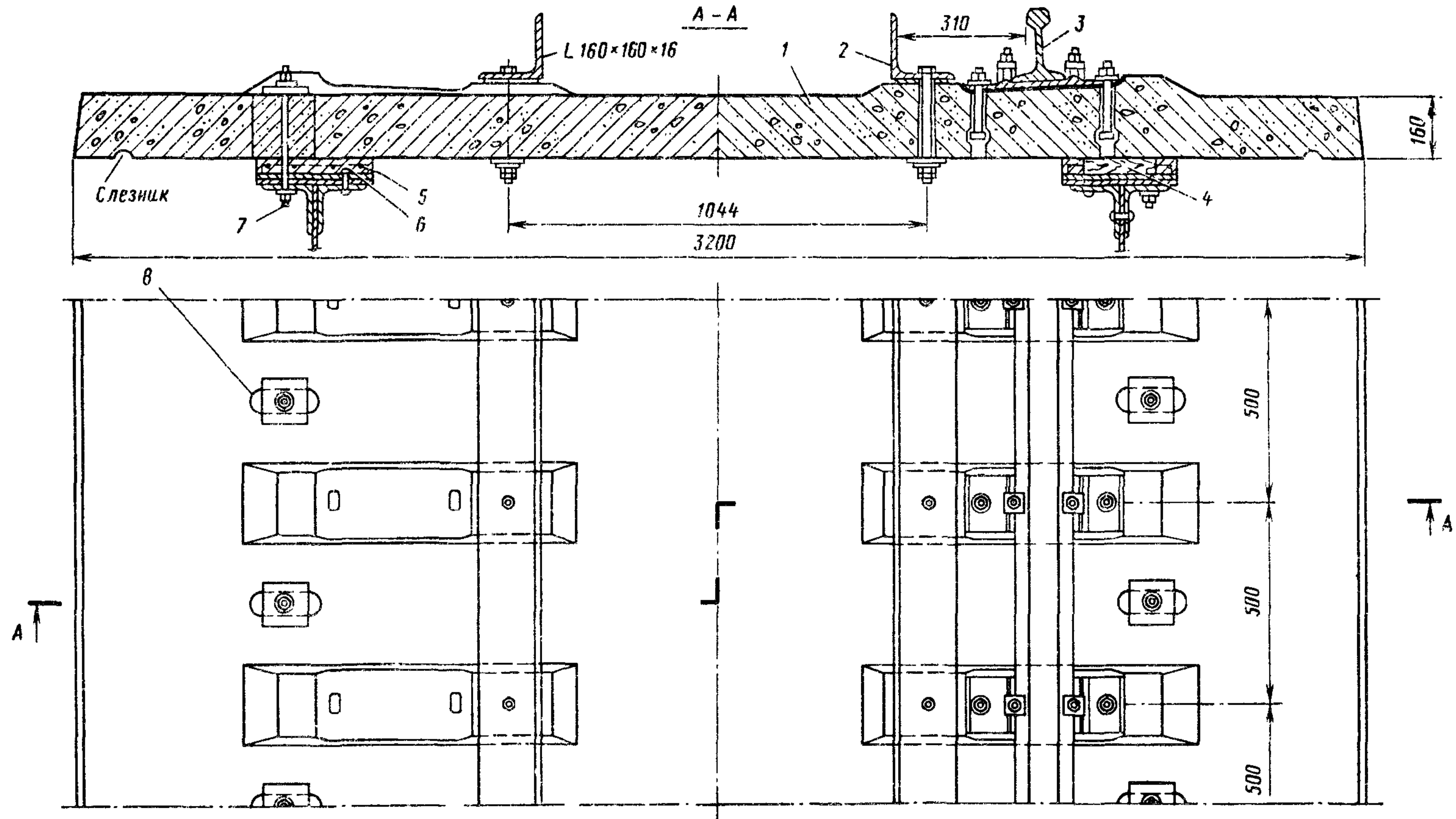
Рис. 16. Мостовое полотно на безбалластных железобетонных плитах:
