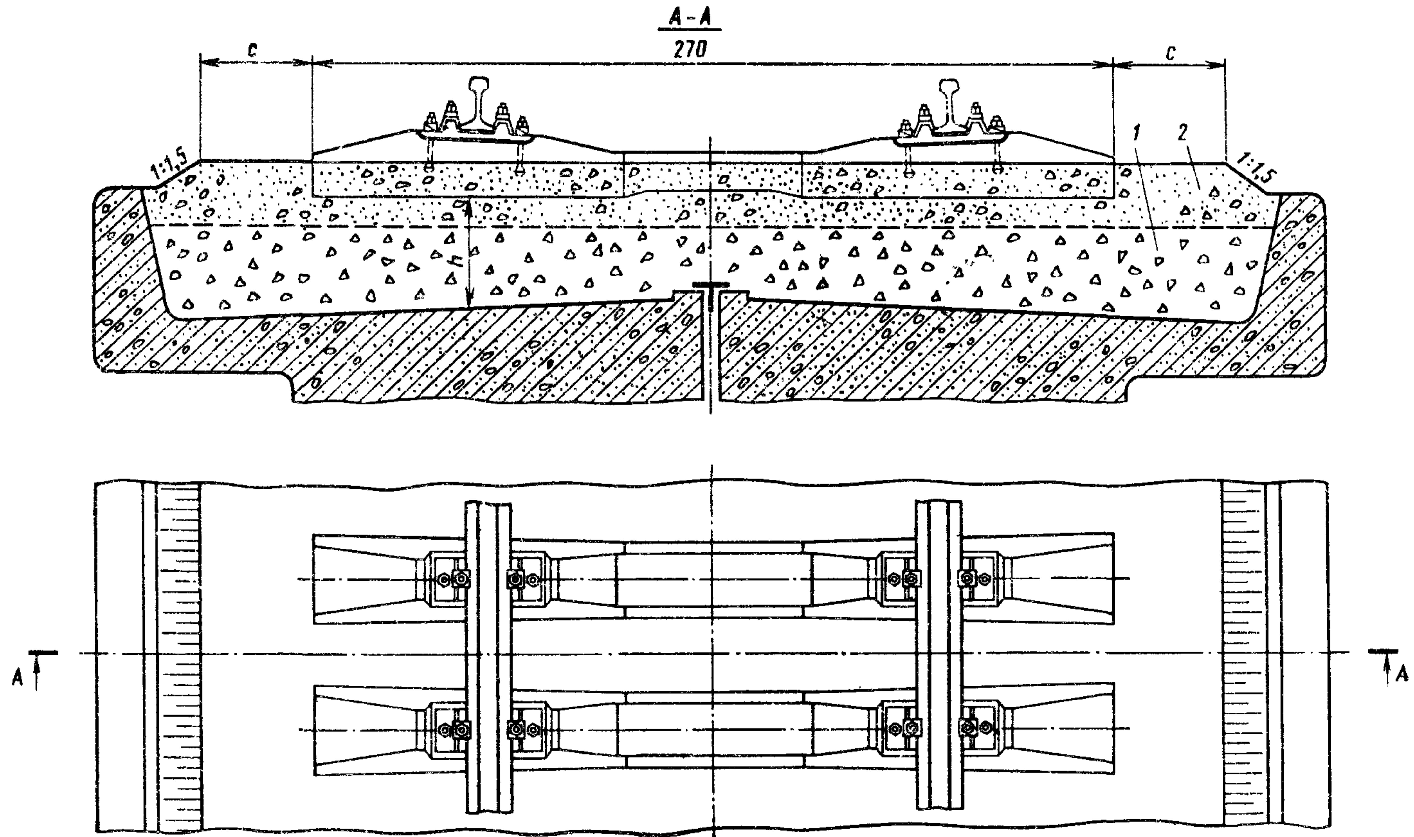
Рис. 4. Поперечный профиль балластной призмы при асбестовом балласте: 1 — дренарующий слой щебня (фракции 5—25 мм); 2 — асбестовый балласт
