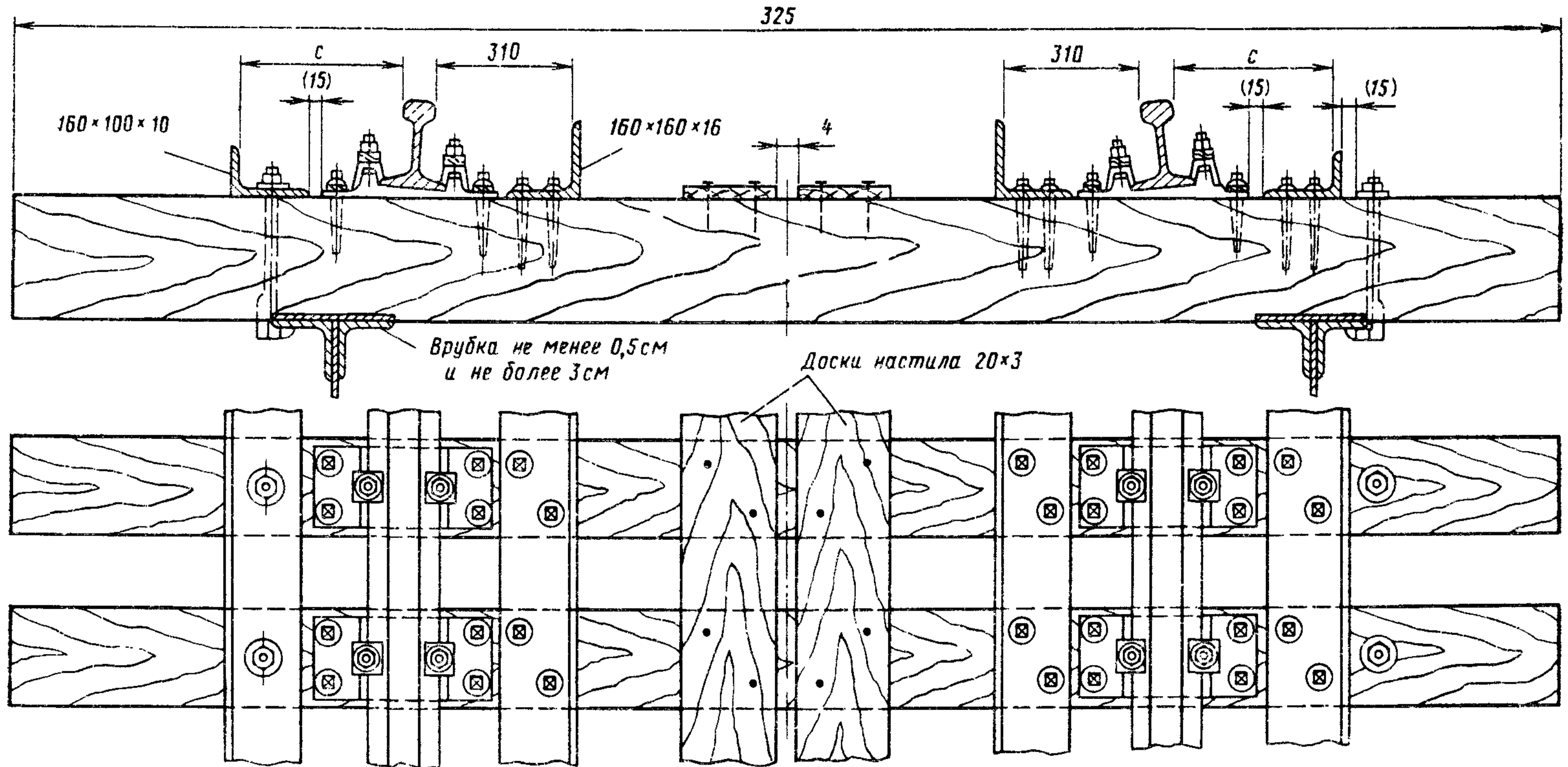
Рис. 7. Мостовое полотно на мостовых брусках с отдельным клеммно-шурупным креплением рельсов: слева — охранный уголок прикреплен лапчатым болтом; справа — охранный уголок прикреплен шурунами. Примечание см. к рис. 6
