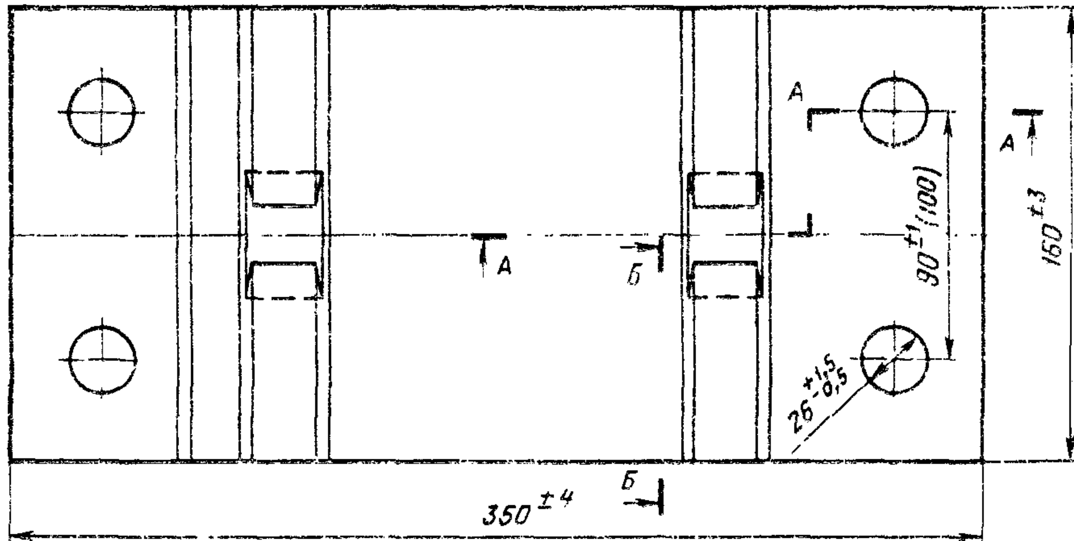
Рис. 1. Рельсовая подкладка КД65 (ЦП 45-72)
