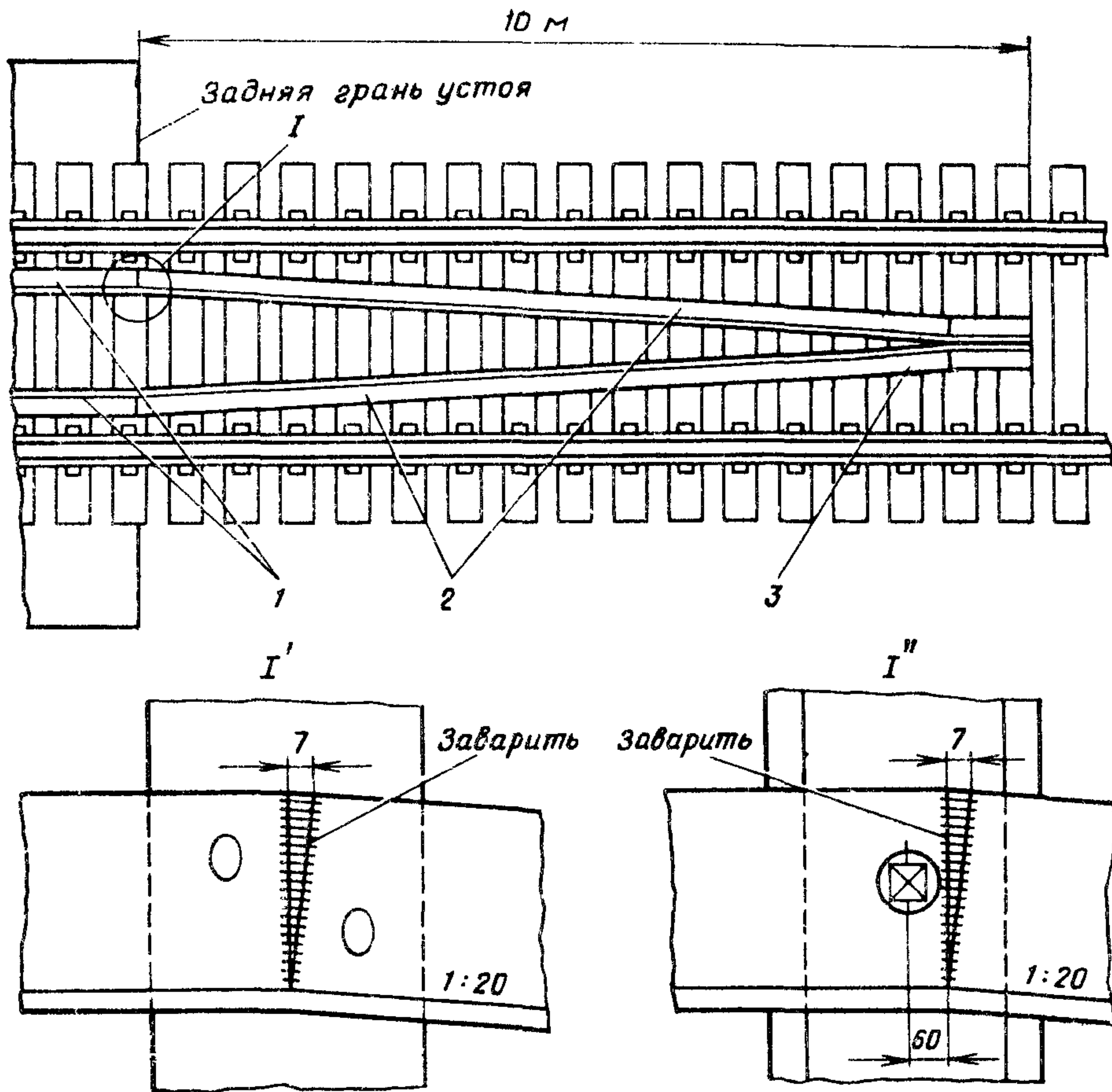
Рис. 21. Схема укладки «челнока» контруголков (контррельсов):
