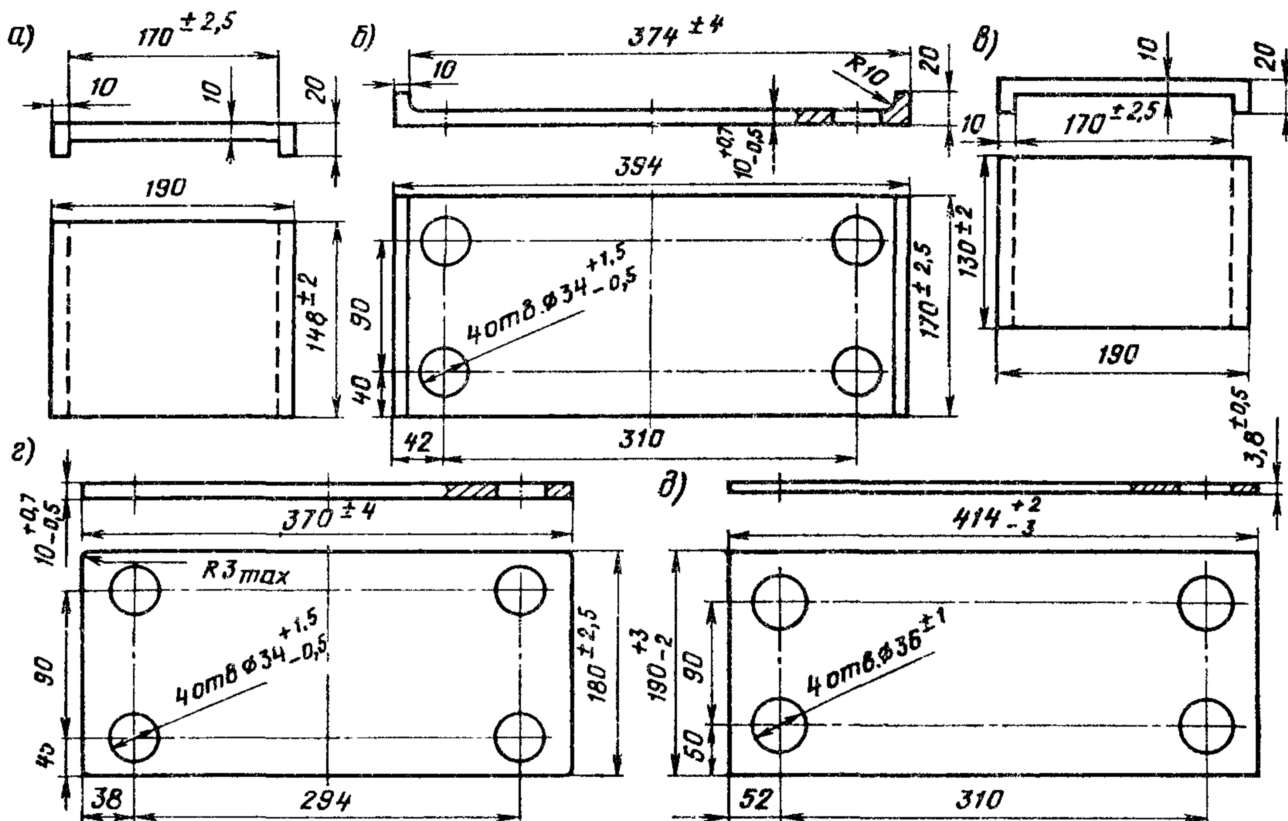
Рис. 2. Прокладки на металлических поперечинах:
