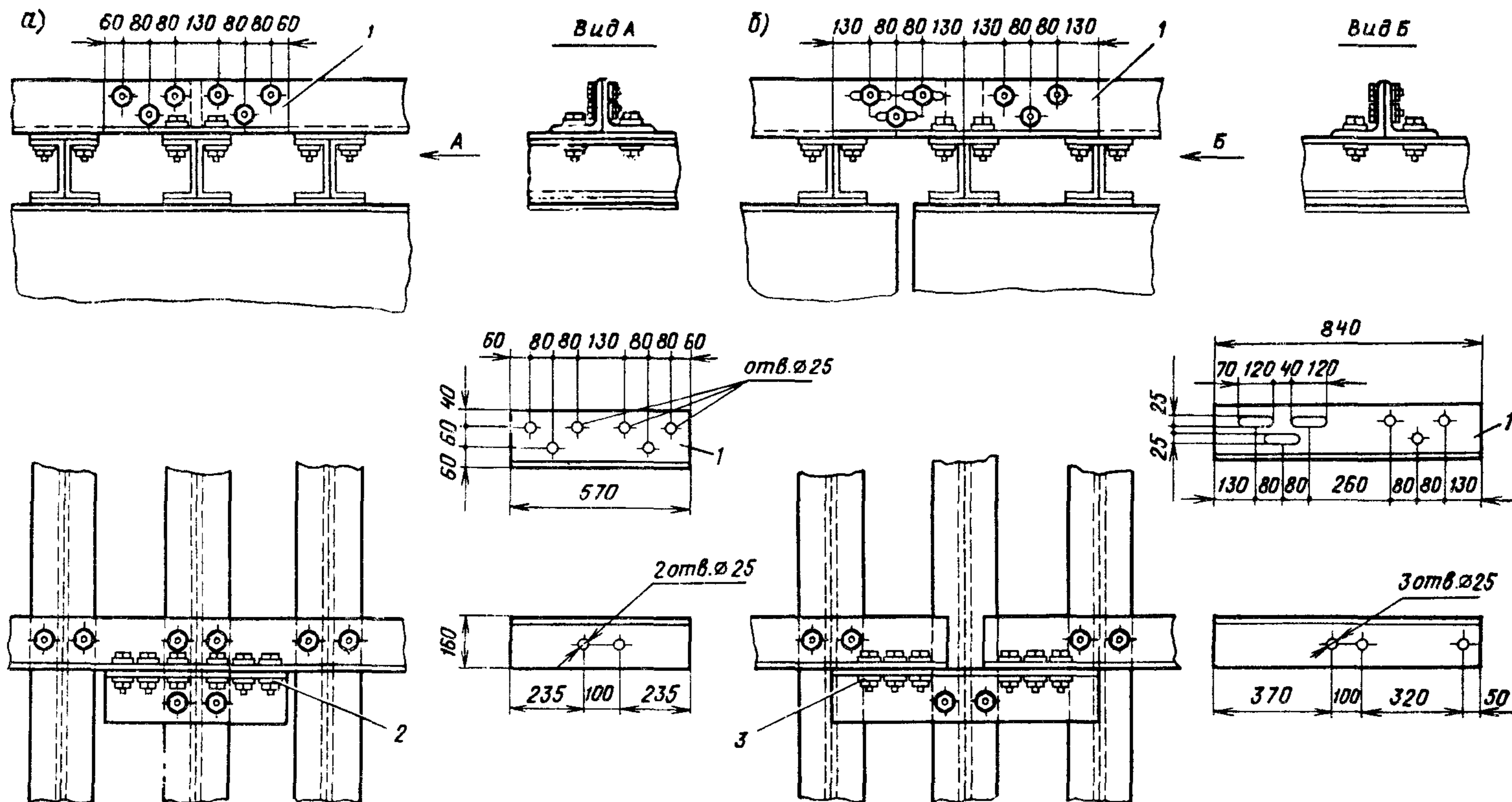
Рис. 26. Стык контруголков на металлических поперечинах:
