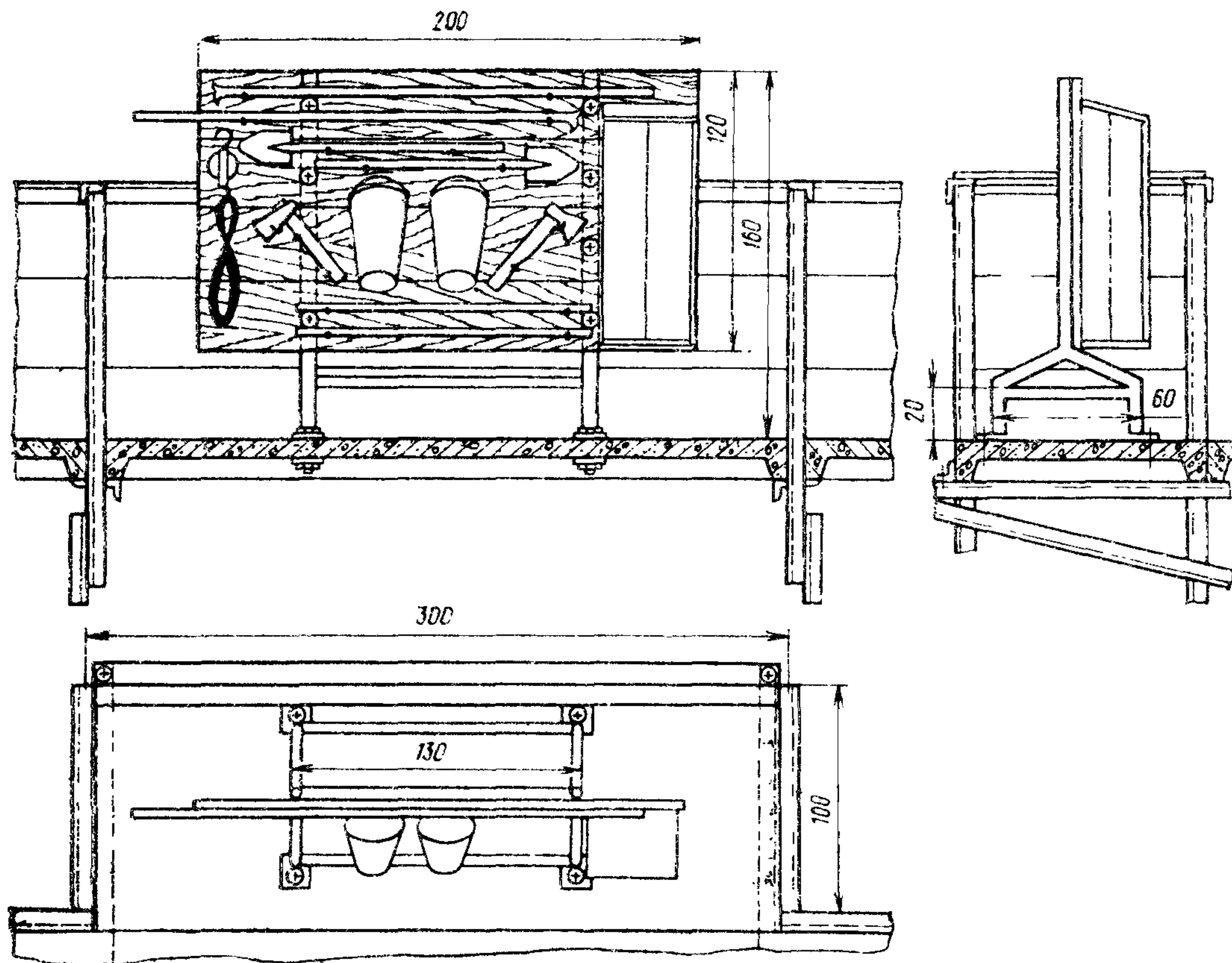
Рис. 4. Противопожарный щит
