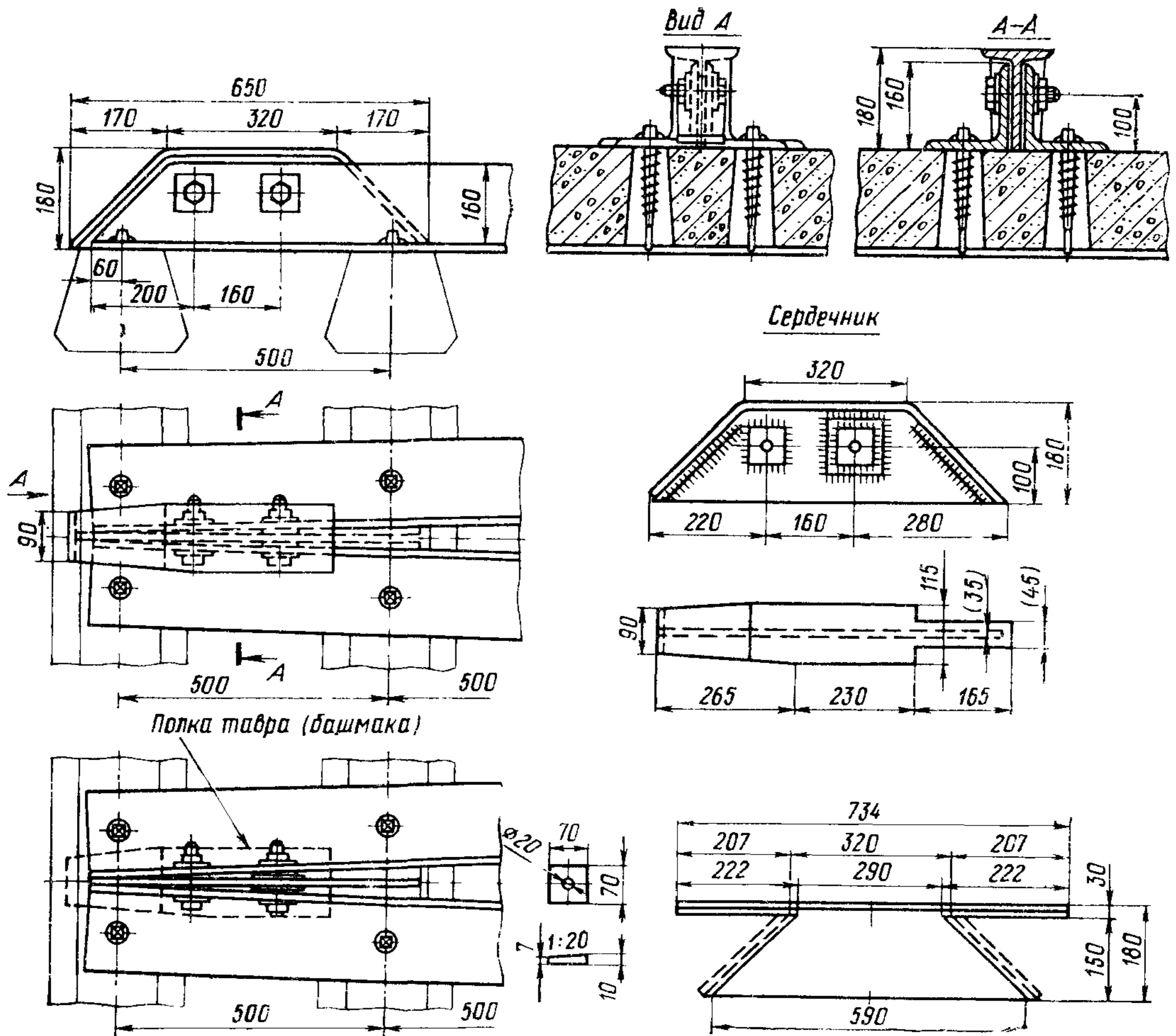
Рис. 29. Допустимый тип башмака контруголков при железобетонных шпалах.
