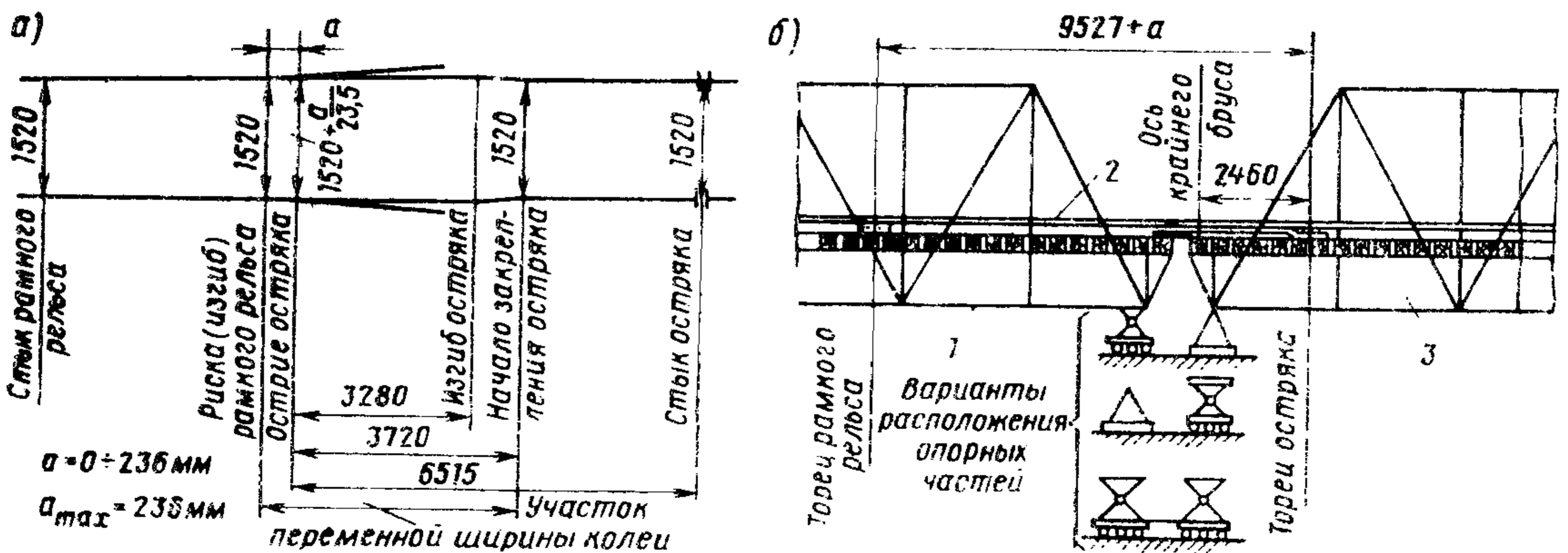
Рис. 3. Уровнительный прибор типа Р50 (проект № 012.00.000):
