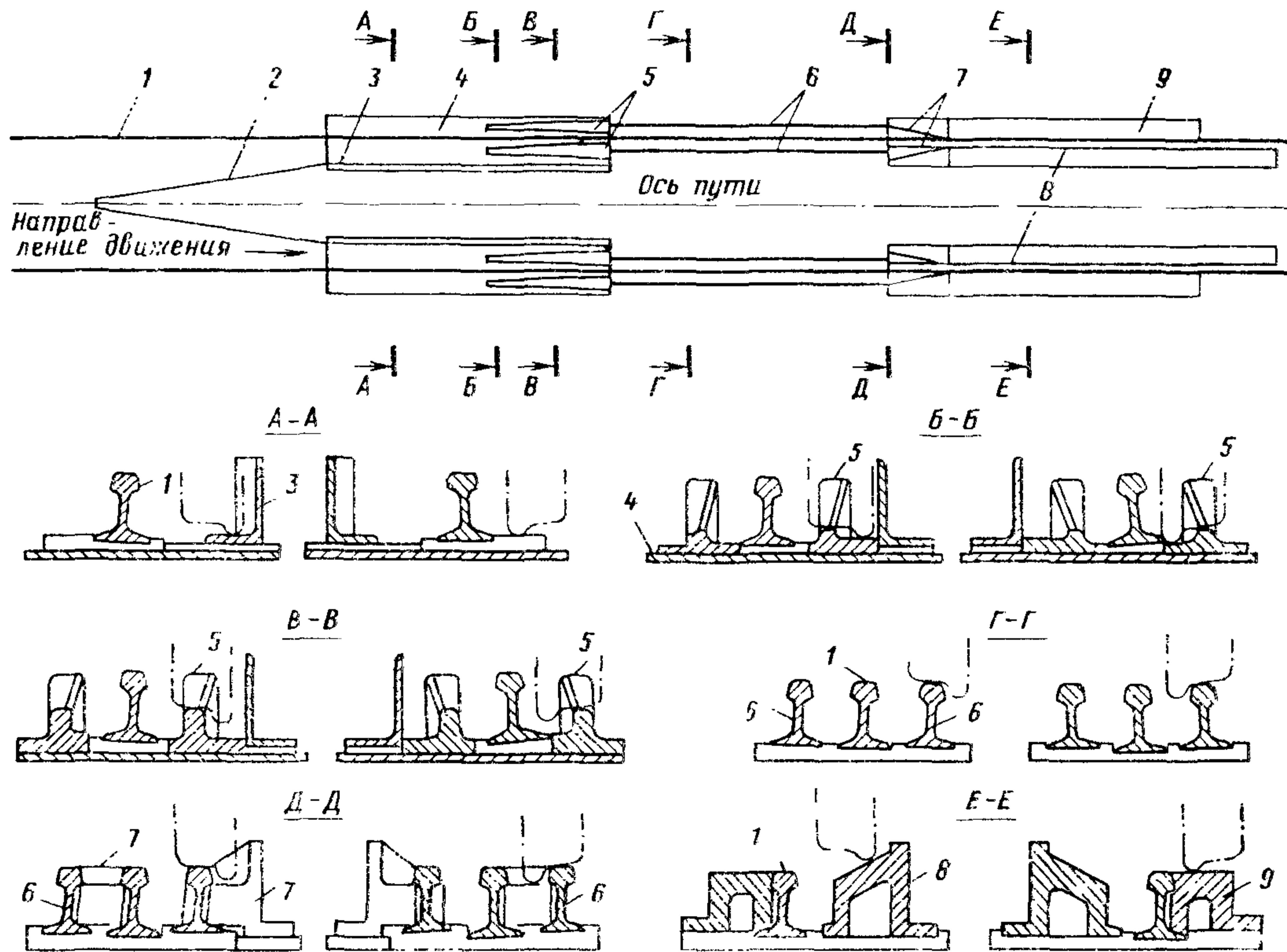
Вкатыватель подвижного состава
