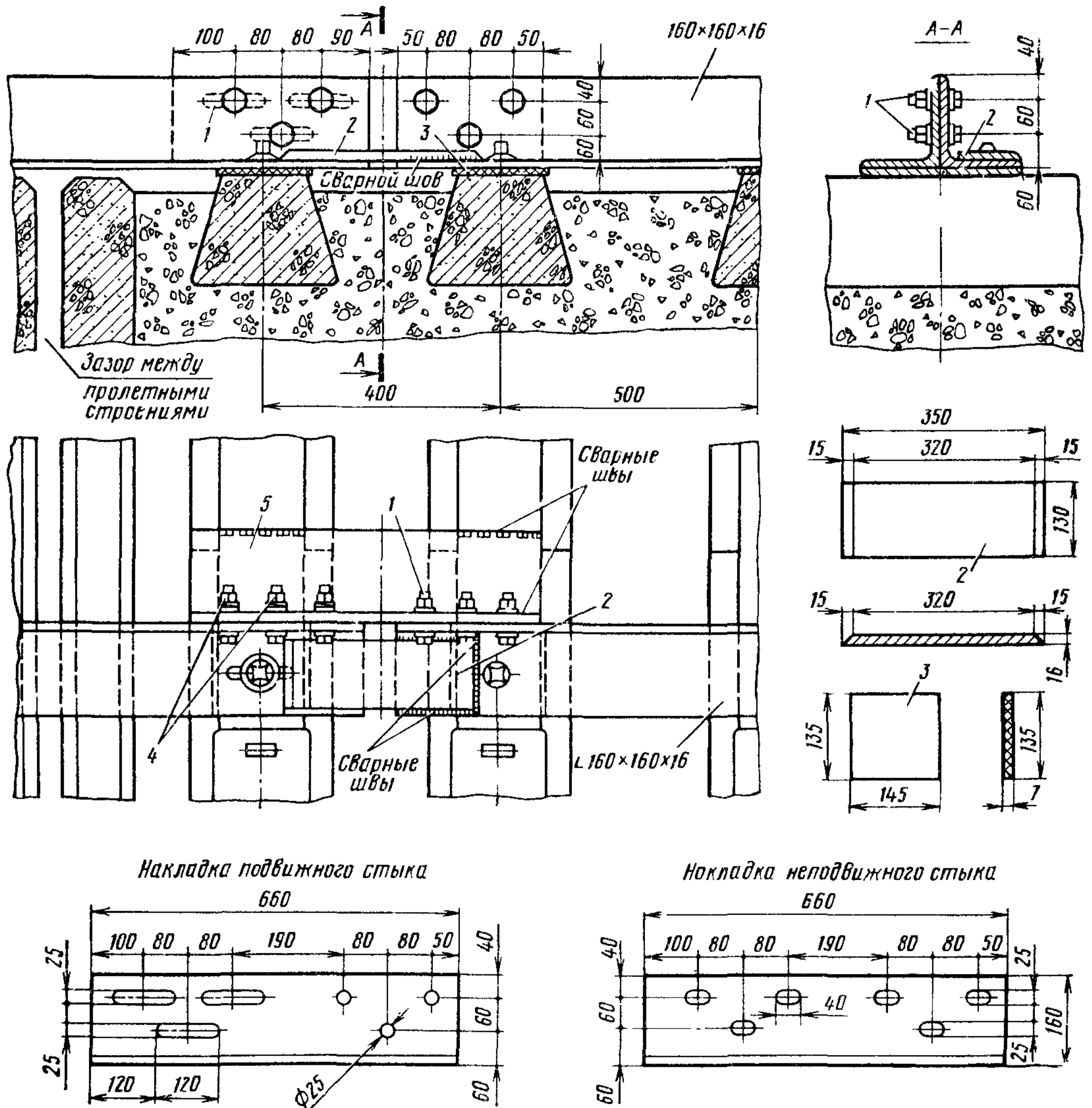
Рис. 25. Стыки контруголков на железобетонных шпалах:
