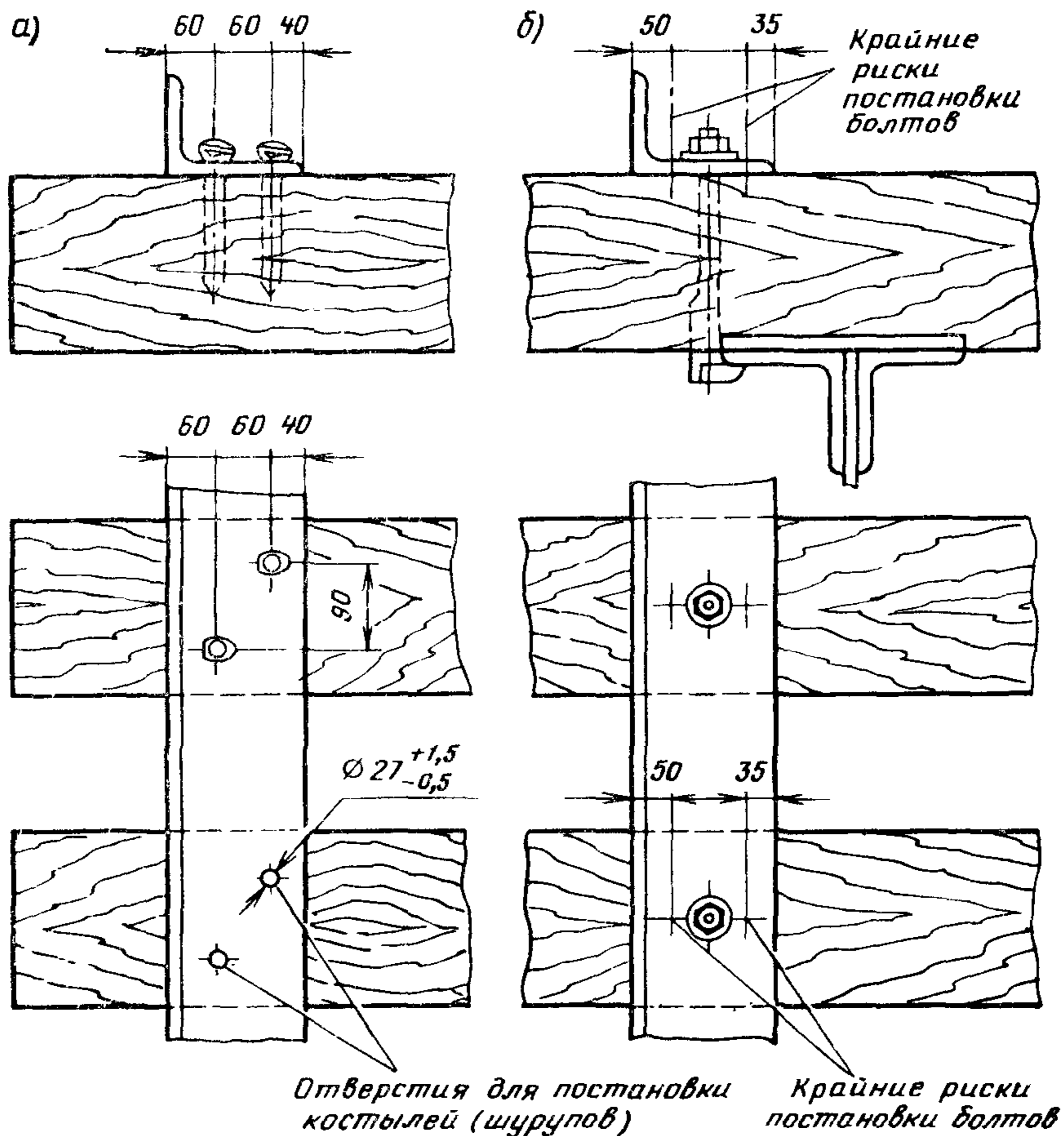
Рис. 33. Крепление противоугольных (охранных) уголков:
