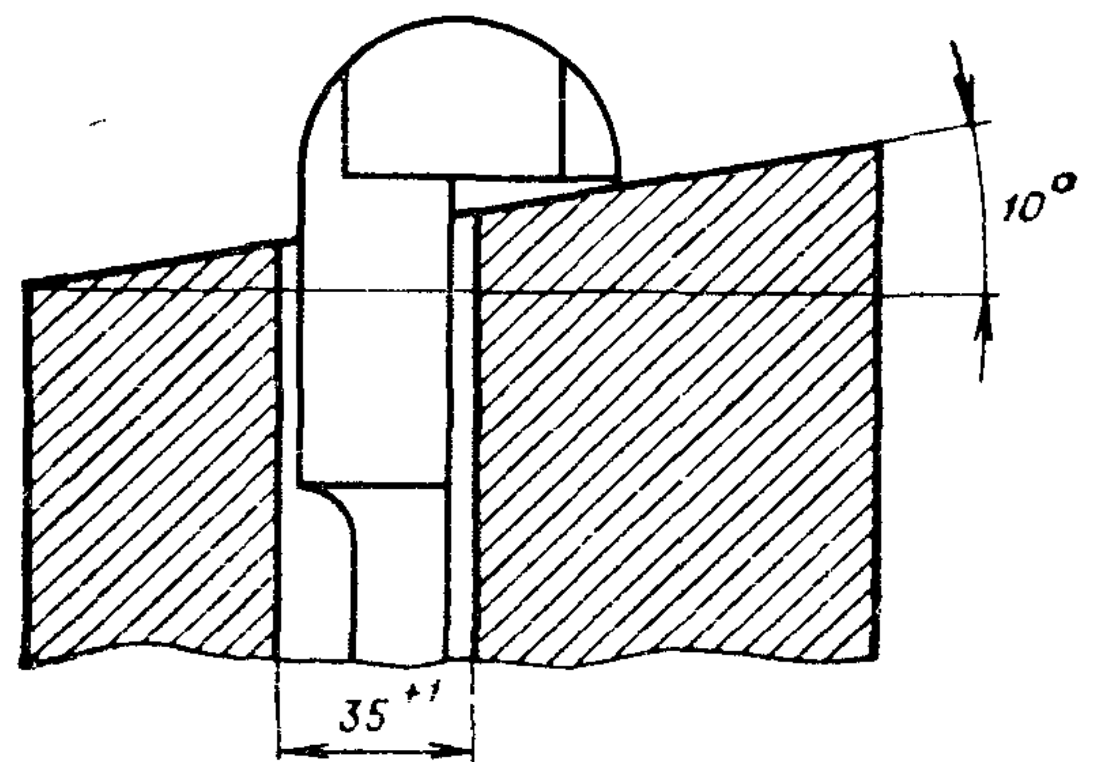
Рис. 2. Матрица для испытания лапчатых болтов
