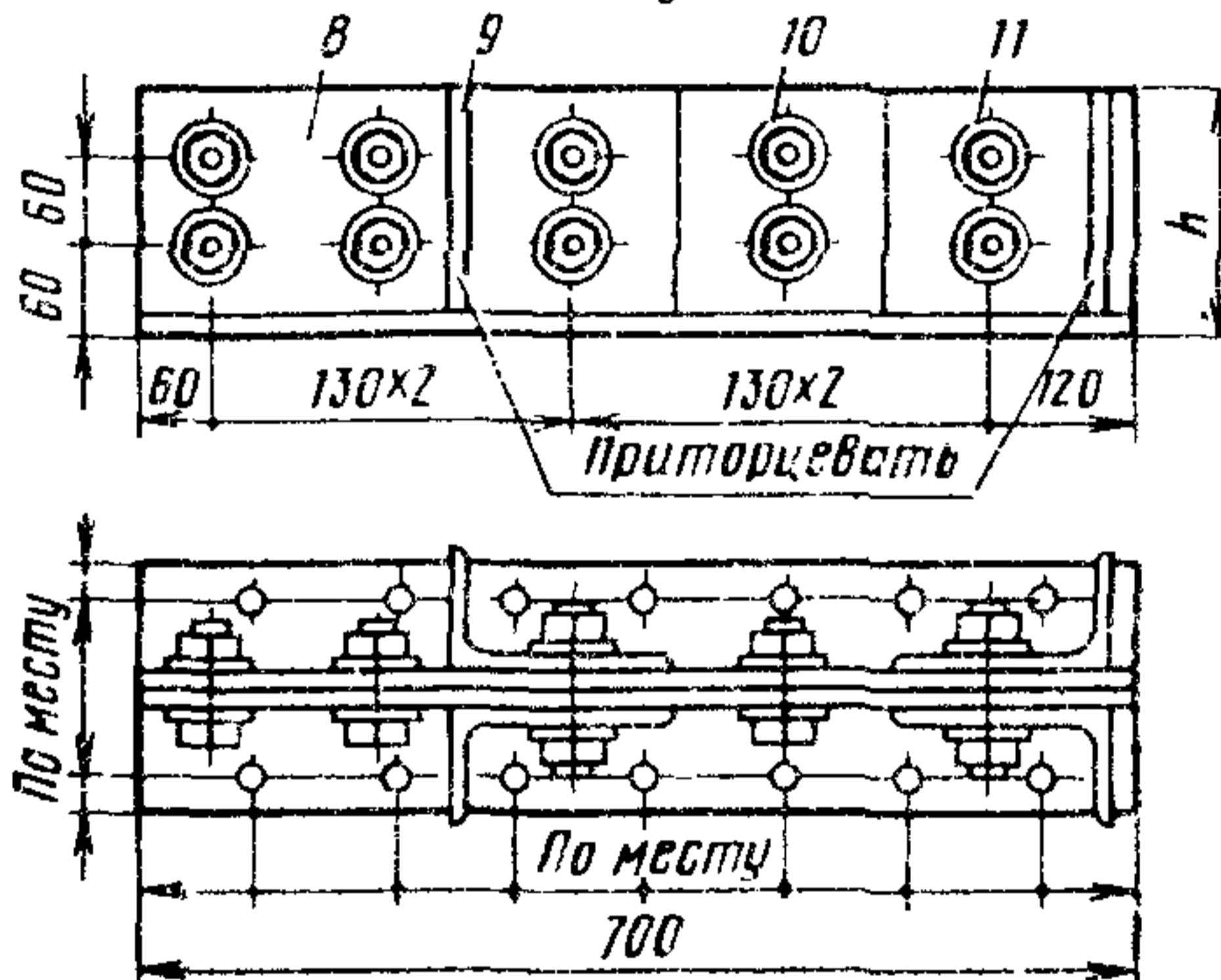
Рис. 39. Столики на поперечной балке:
