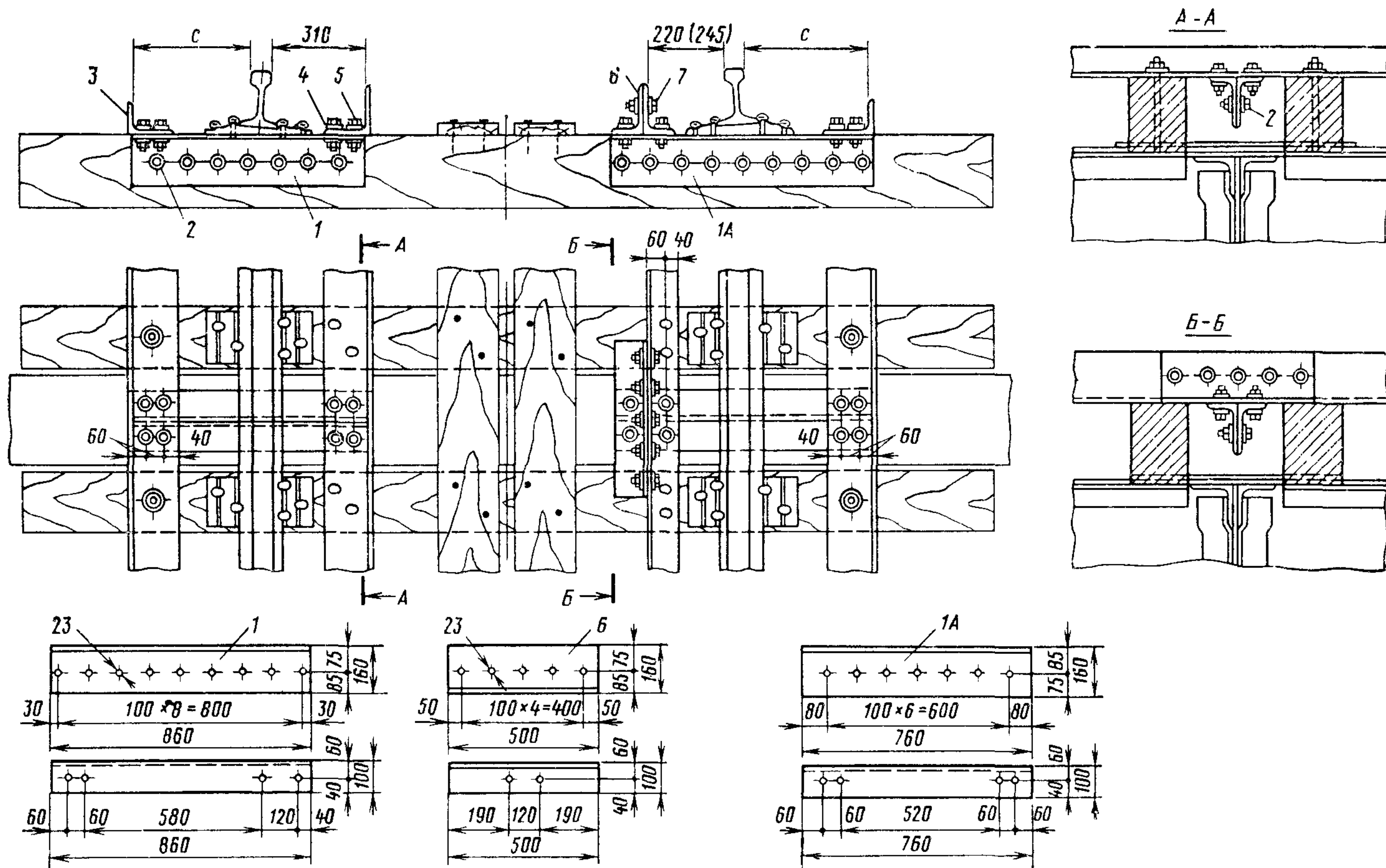
Рис. 38. Подвесной мостик над поперечной балкой:
