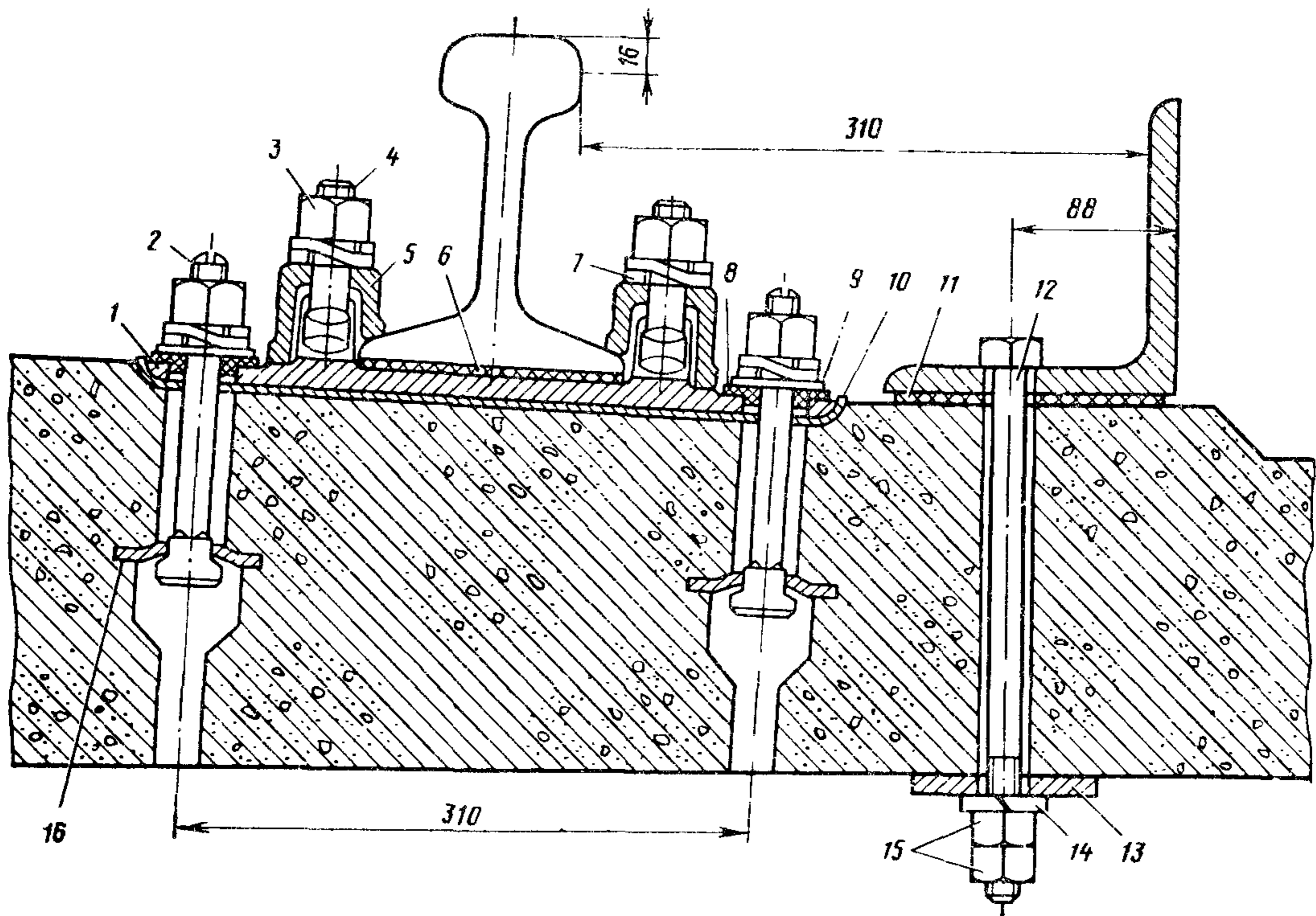
Рис. 17. Крепление рельсов и контррельсов к плите:
