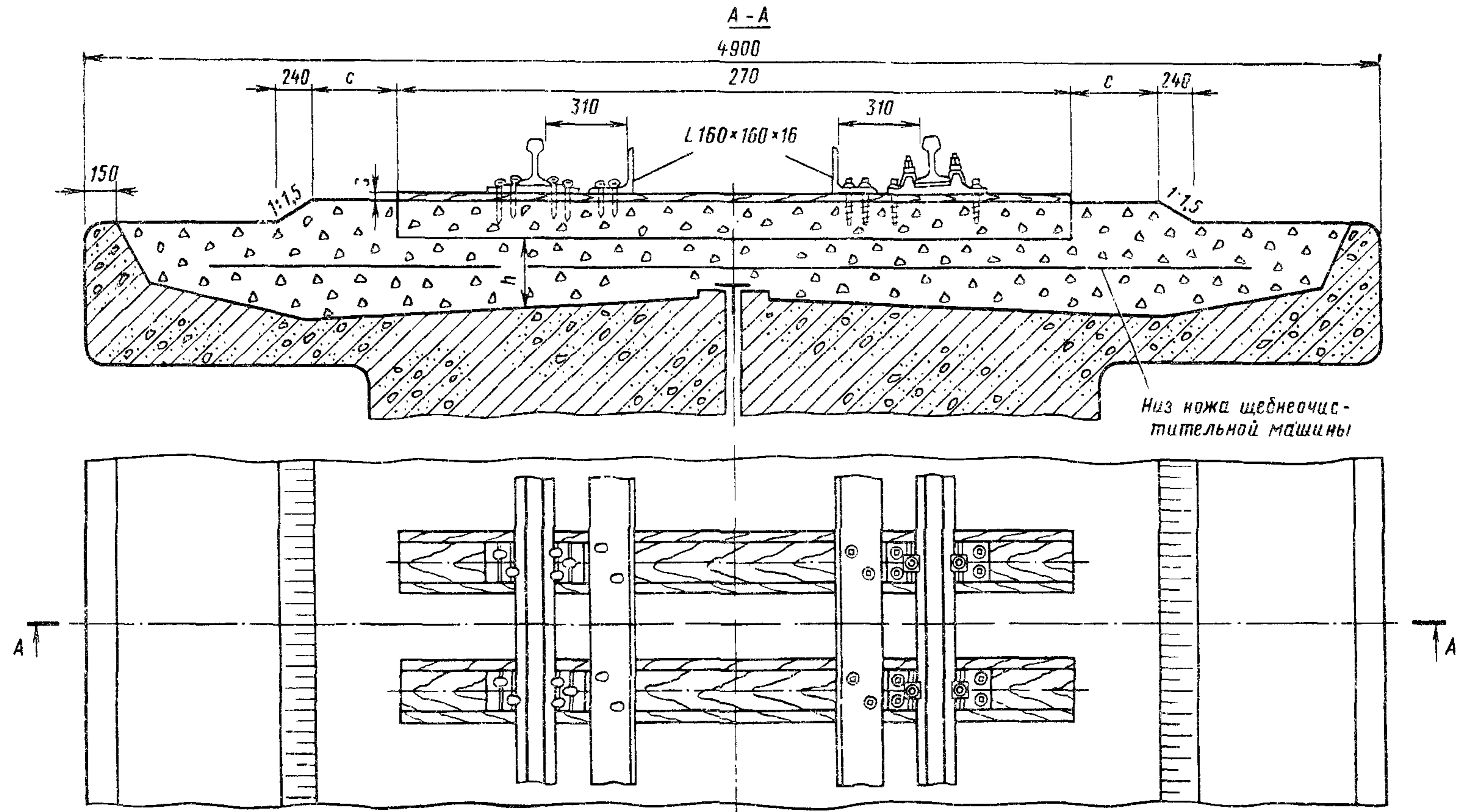
Рис. 2. Мостовое полотно с ездой на щебеночном балласте и деревянных шпалах при балластном корыте, предусматривающем пропуск щебнеочистительных машин: слева — при костыльном креплении рельсов; справа — при клеммно-шурупном креплении рельсов
