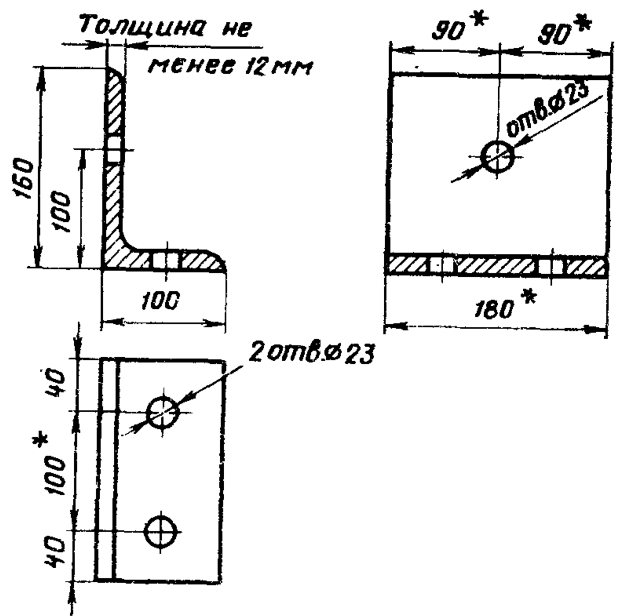
Рис. 40. Противоугольный угольковый коротыш.
