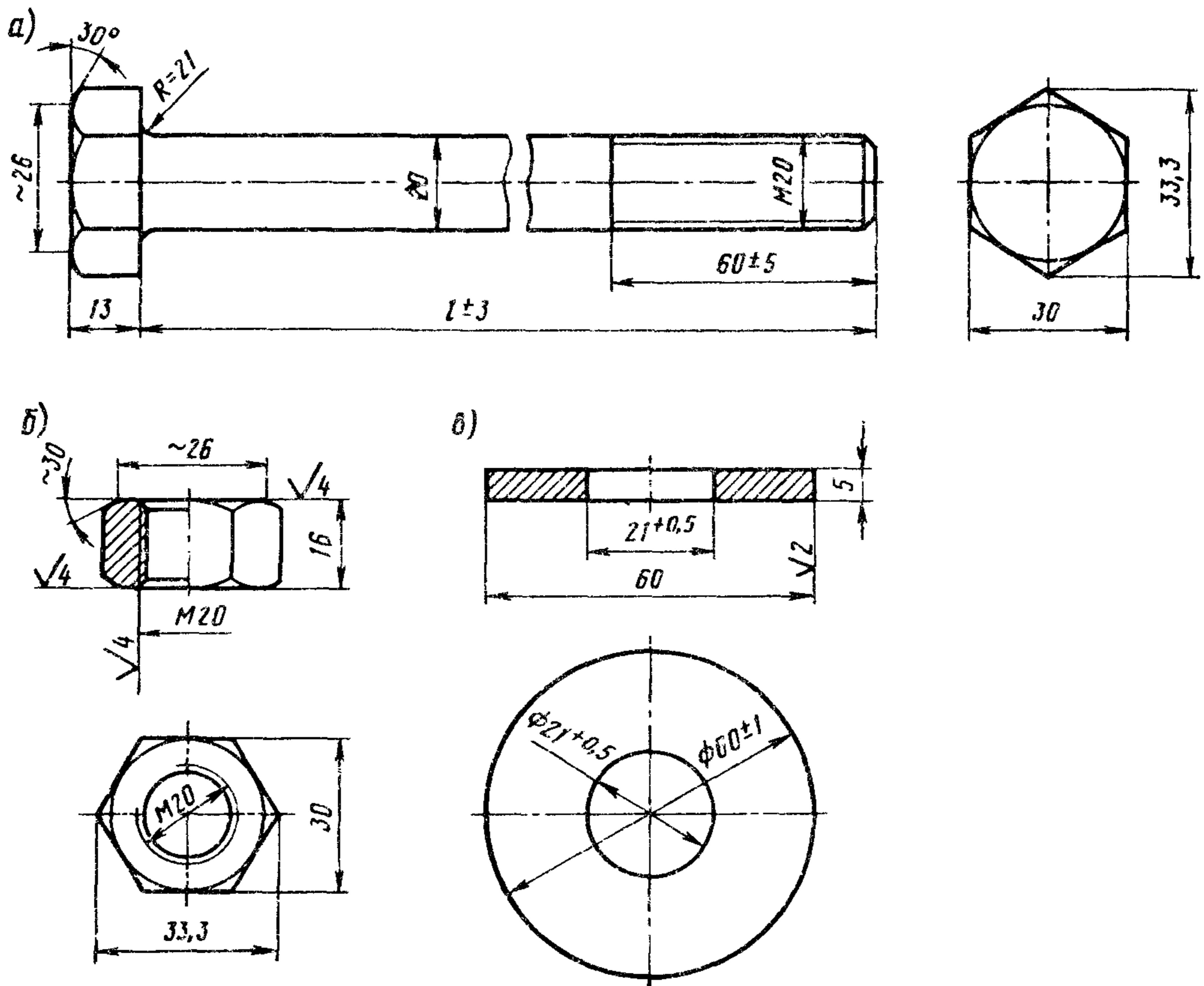
Рис. 6. Болт прикрепления противоугольных (охранных) брусьев к мостовым и мостовым брусьям к противоугольным уголкам: а — болт; б — гайка; в — шайба
