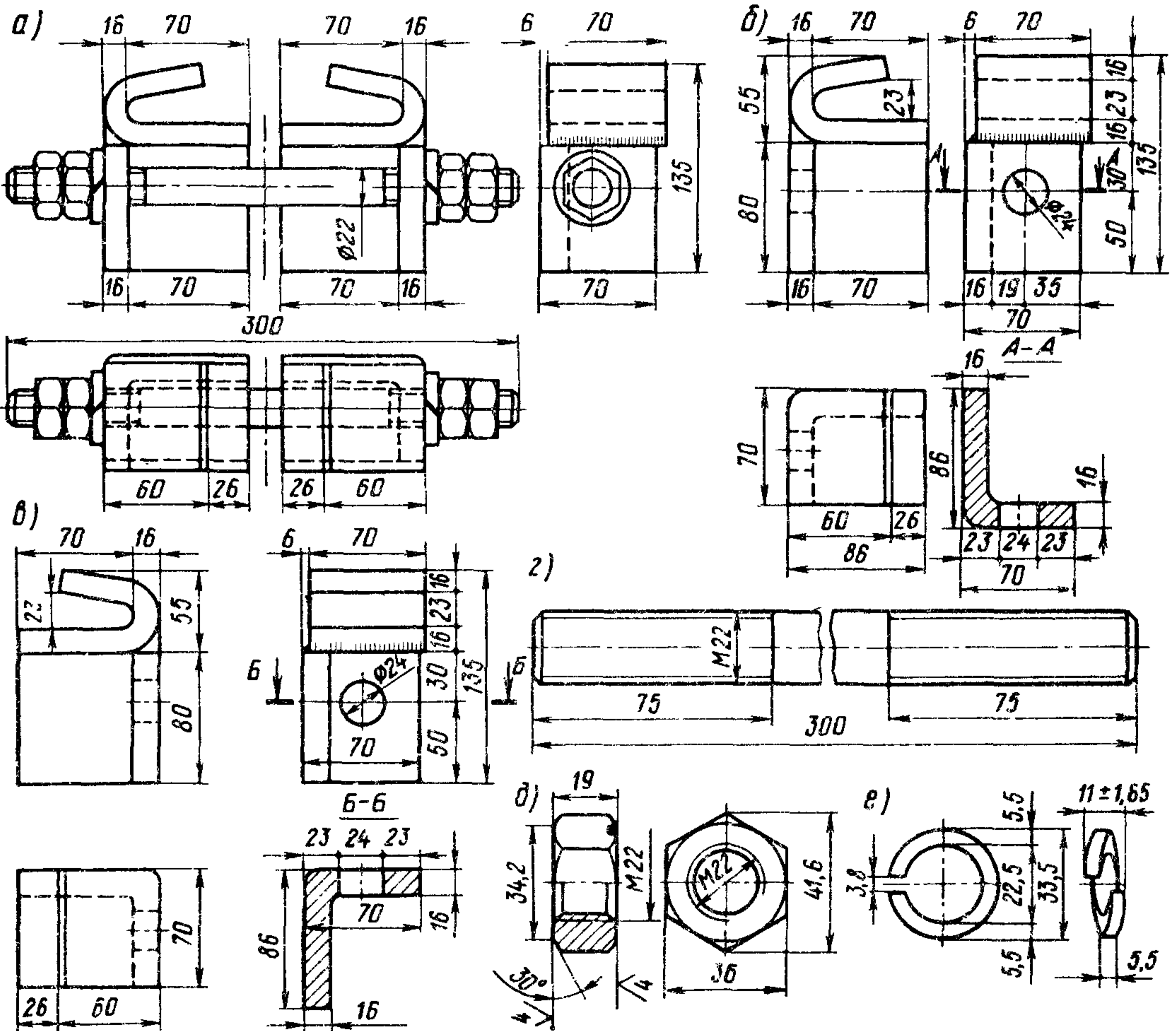
Рис. 10. Противоуго́н винтовой:
