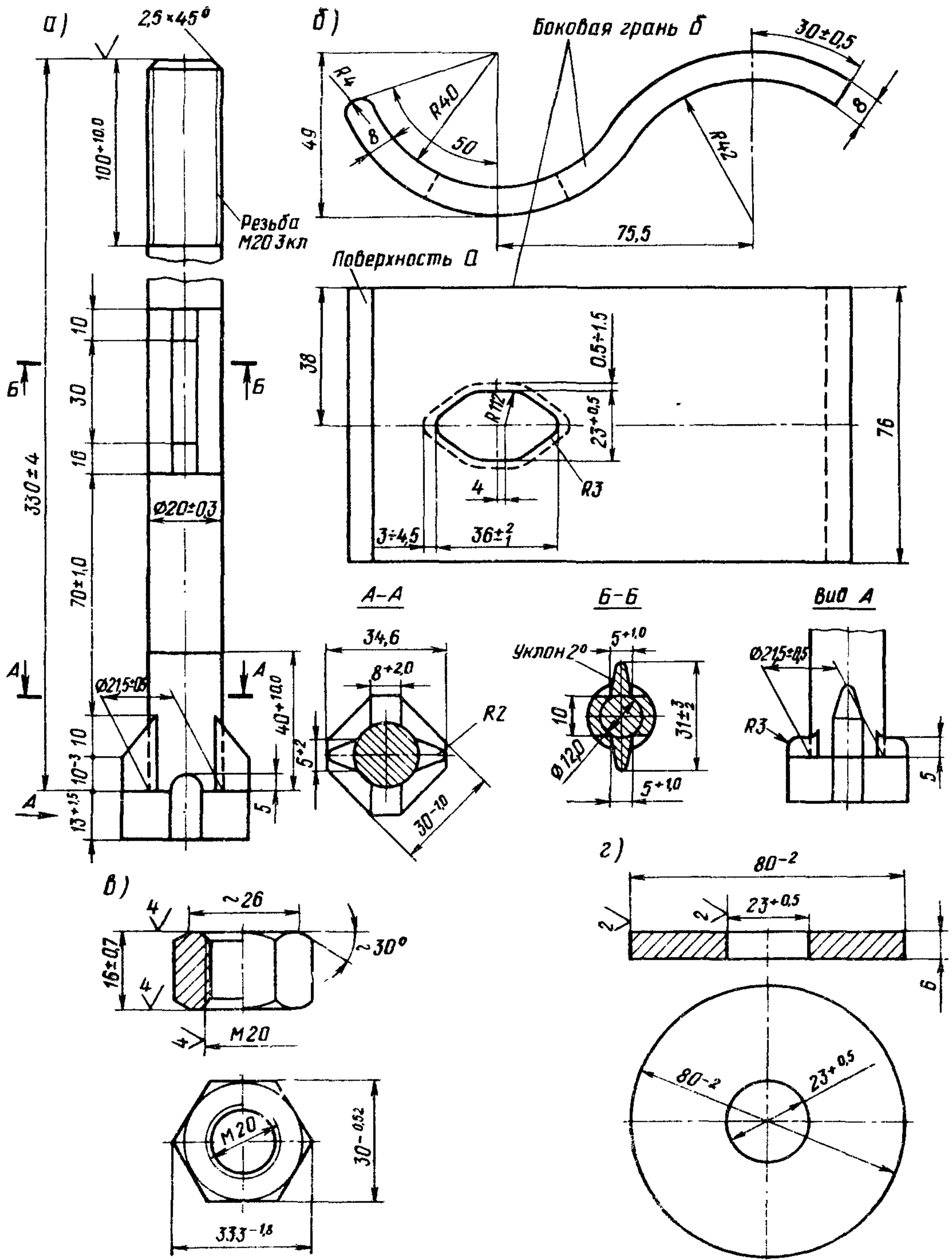
Рис. 4. Лапчатый болт с пружинной лапой:
