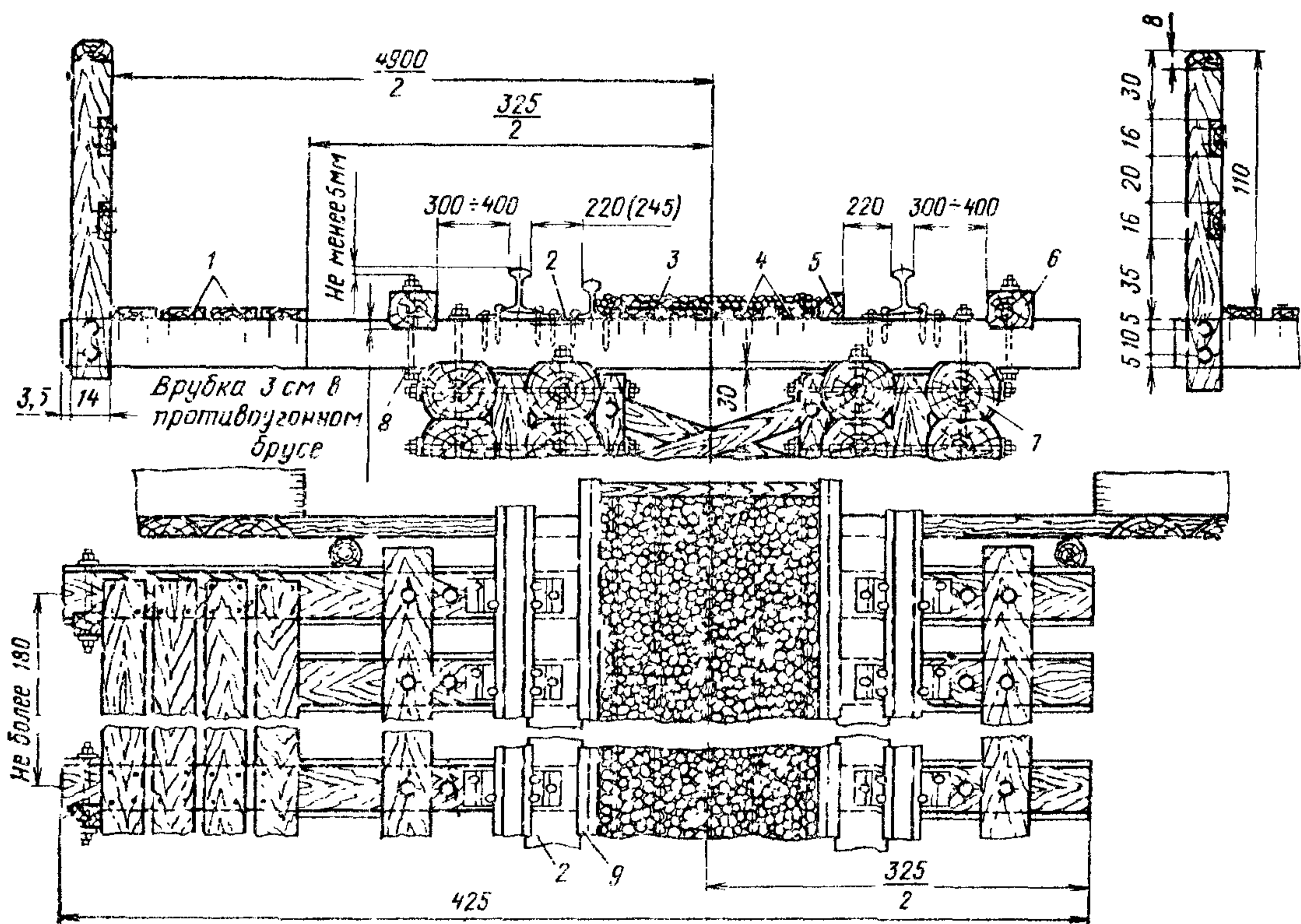
Рис. 18. Мостовое полотно на деревянных пролетных строениях:
