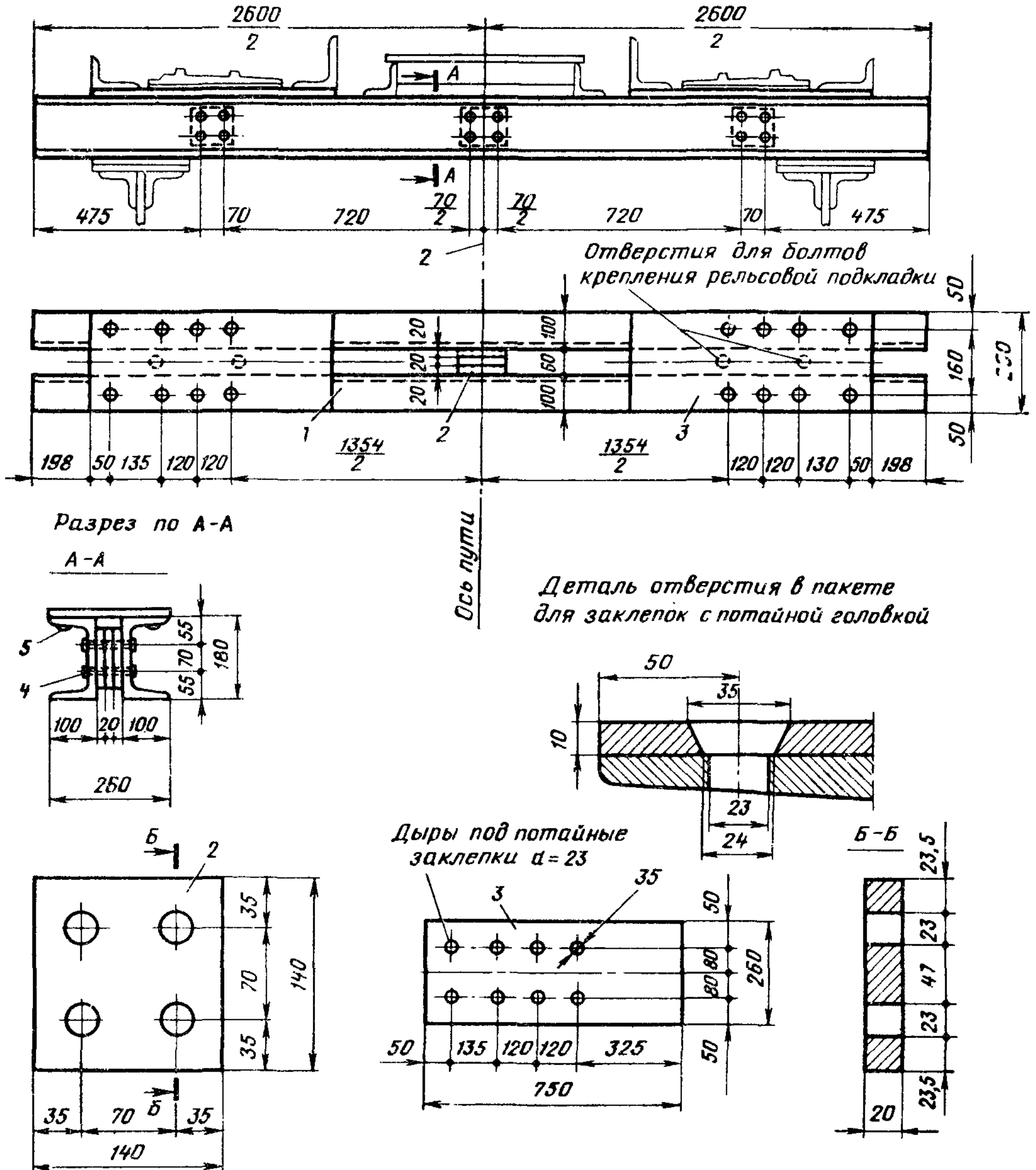
Рис. 1. Металлическая поперечина из прокатных швеллеров:
