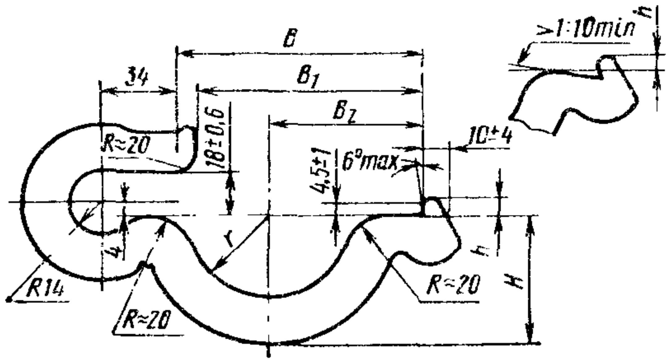
Рис. 9. Противоуго́н пружинный
