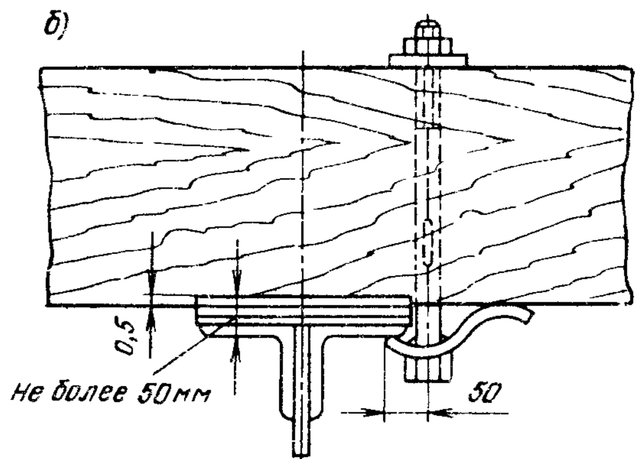
Рис. 3. Схема постановки лапчатого болта с пружинной лапой:
