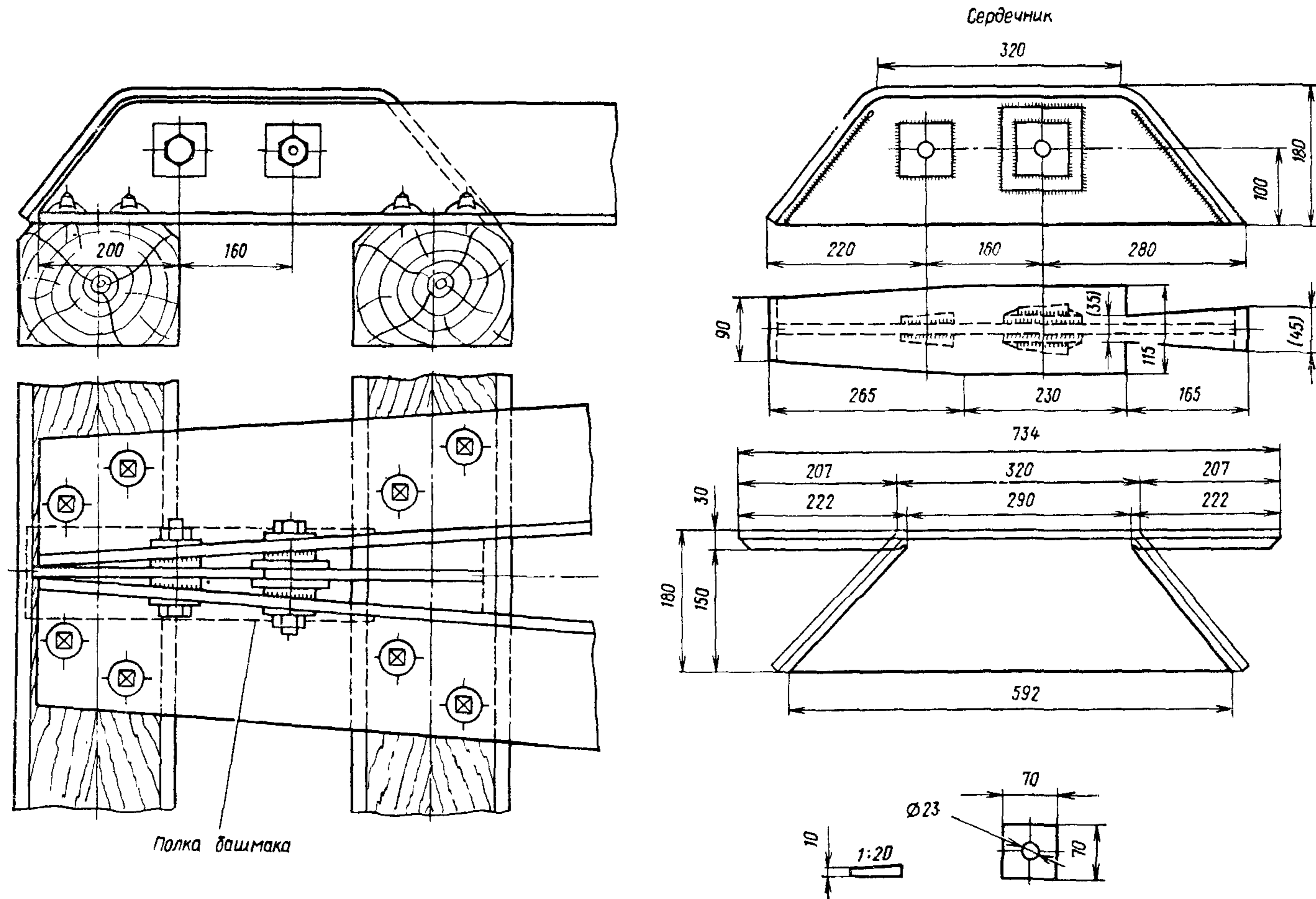
Рис. 28. Допустимый тип башмака коитруголков при деревянных шпалах
