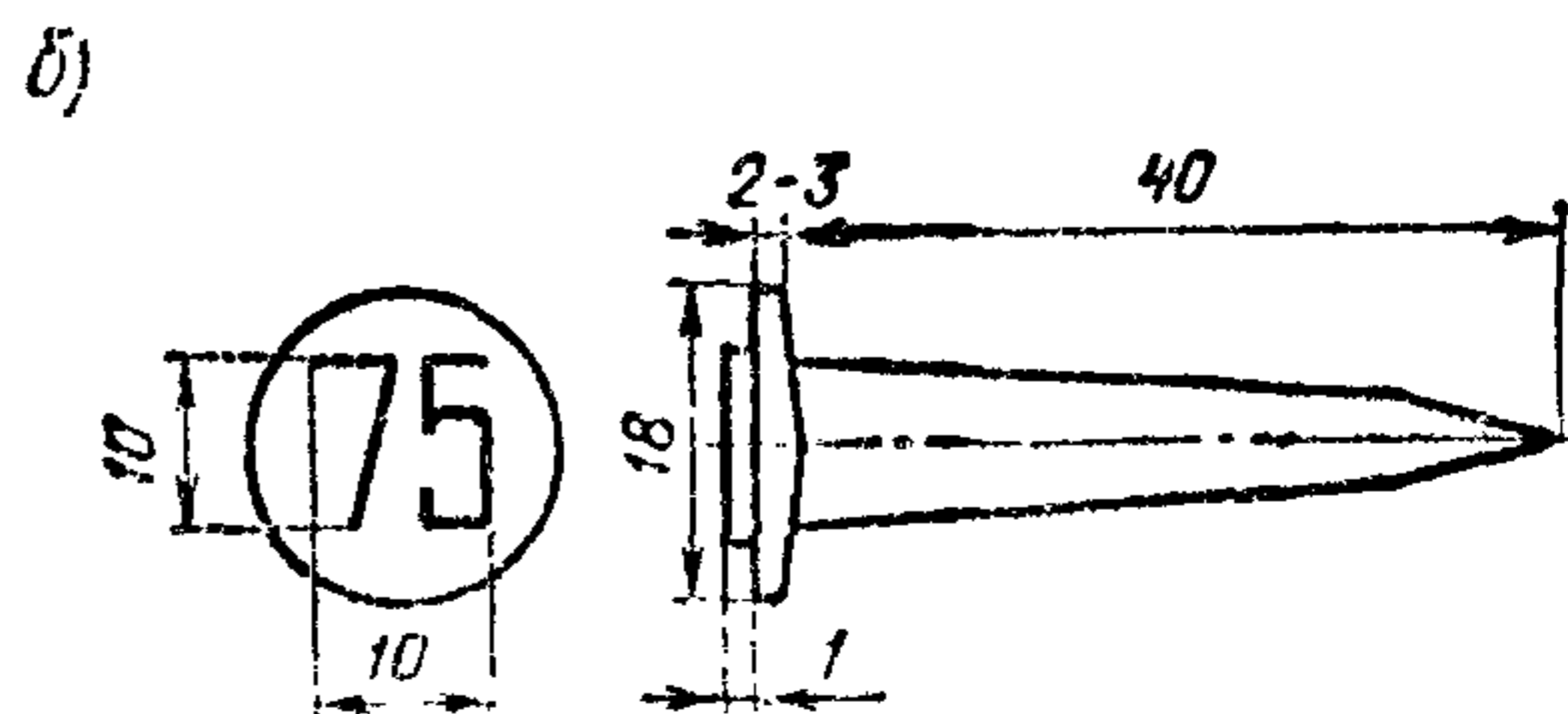
Клейма для мостовых брусьев: а — двухстержневые; б — одностержневые
