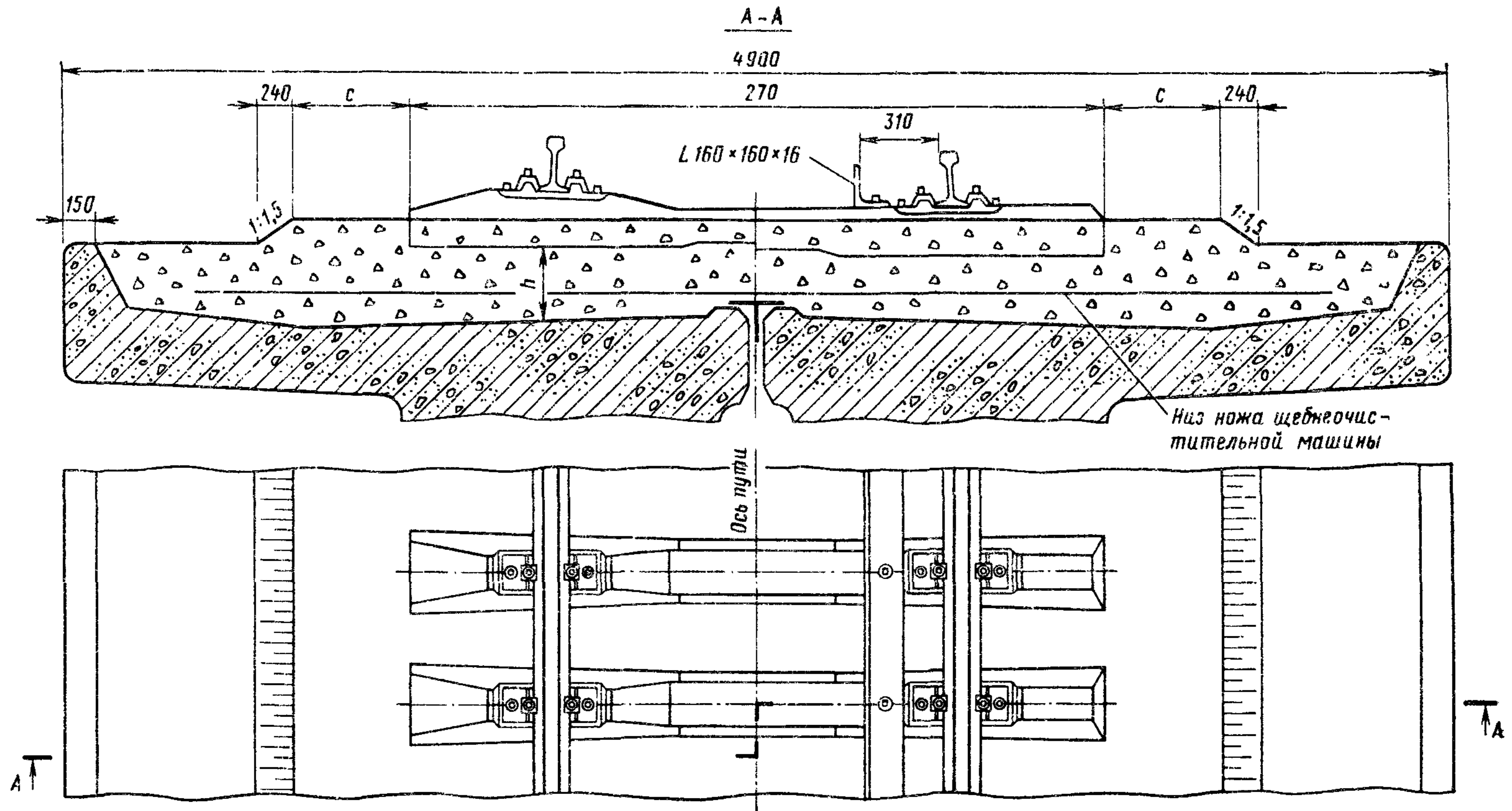
Рис. 1. Мостовое полотно с ездой на щебёночном балласте и железобетонных шпалах при балластном корыте, предусматривающем пропуск щебнеочистительных машин: слева — без охранных приспособлений (с обычными железобетонными шпалами); справа — с охранными приспособлениями (шпалы железобетонные для укладки на мостах)
