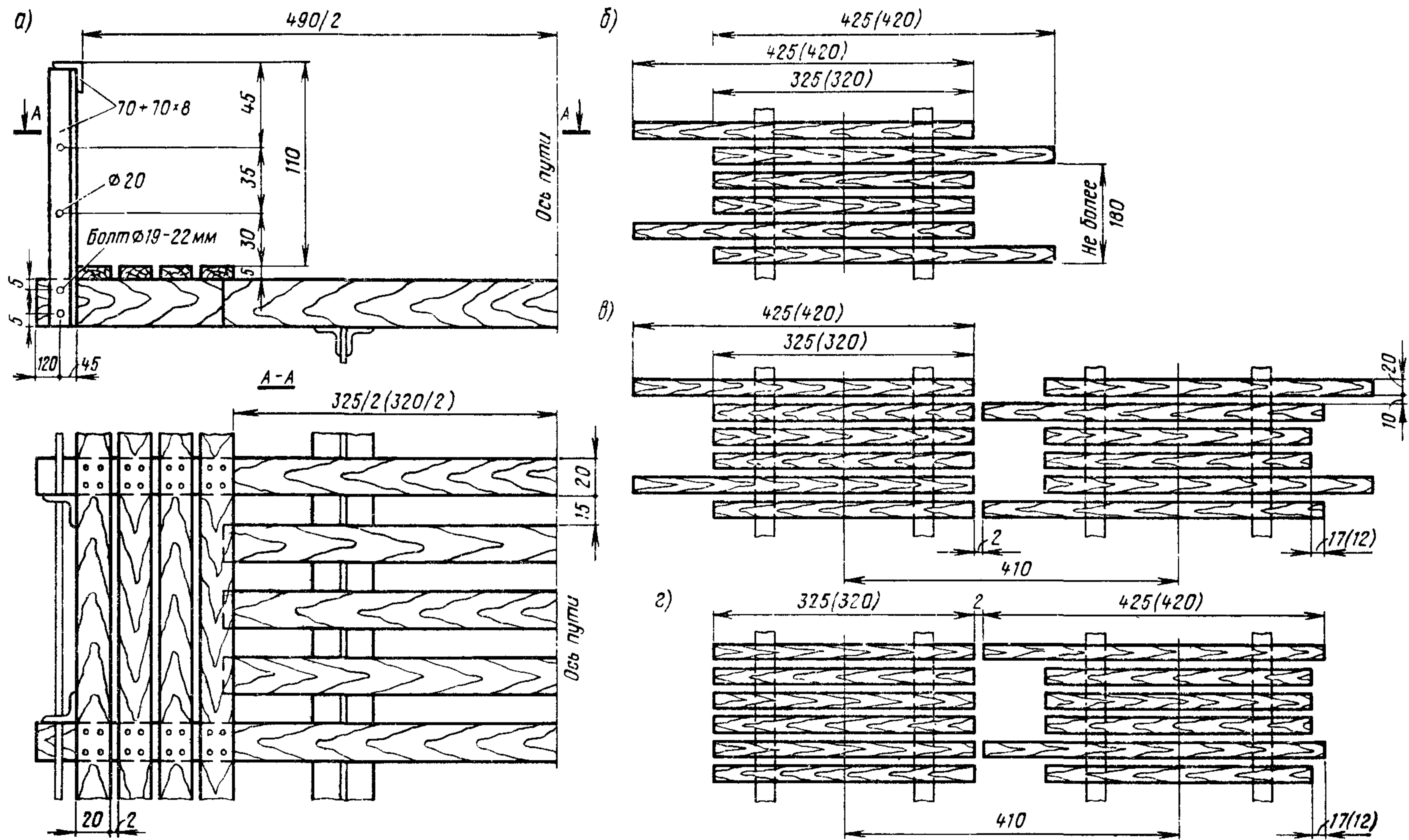
Рис. 41. Устройство тротуаров на длинных мостовых брусках (а) и эюры укладки мостовых брусков на однопутных мостах (б), на двухпутных мостах с боковыми тротуарами (в), при отсутствии боковых тротуаров (г).
