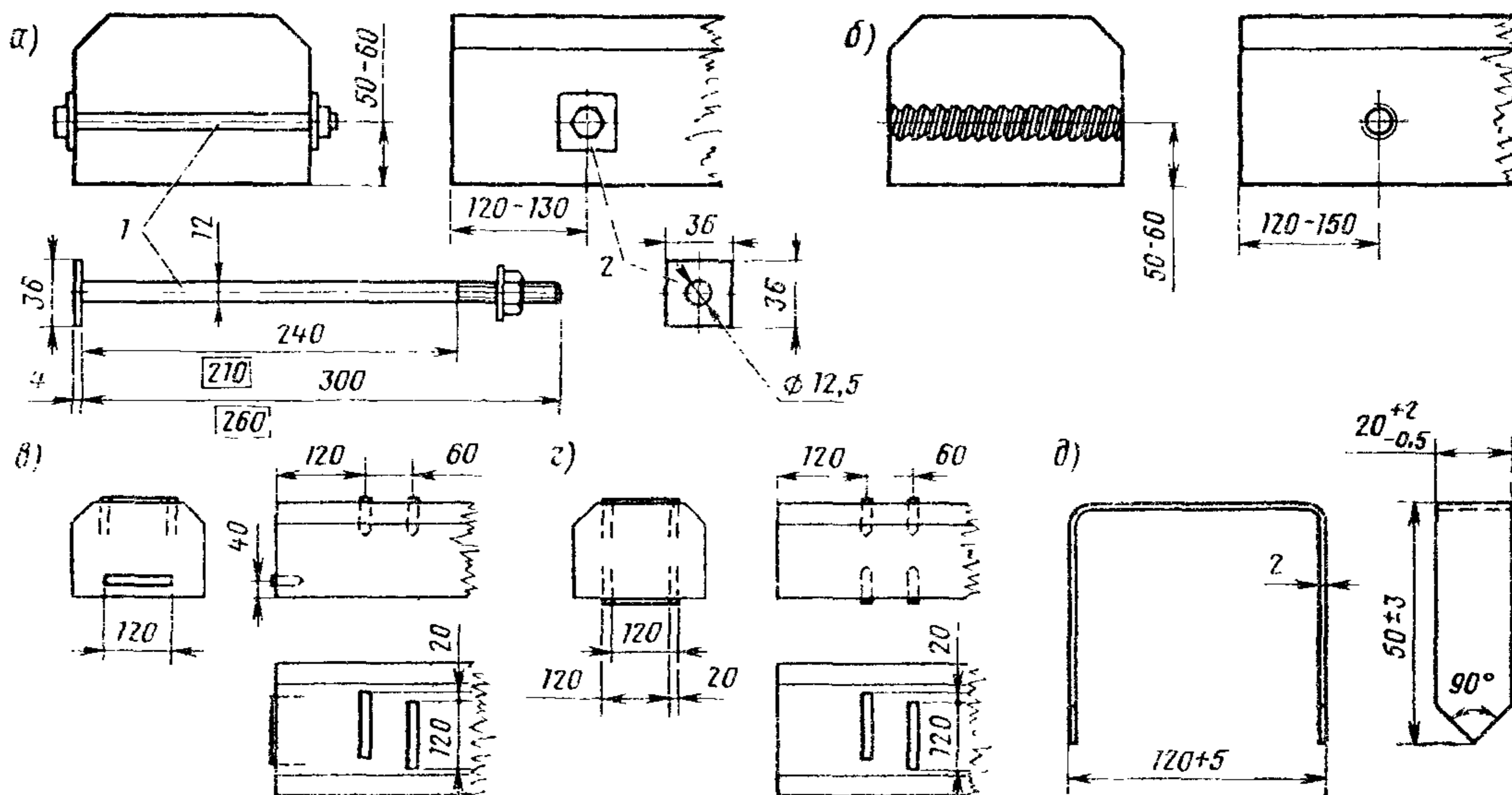
Укрепление мостовых брусьев от растрескивания
