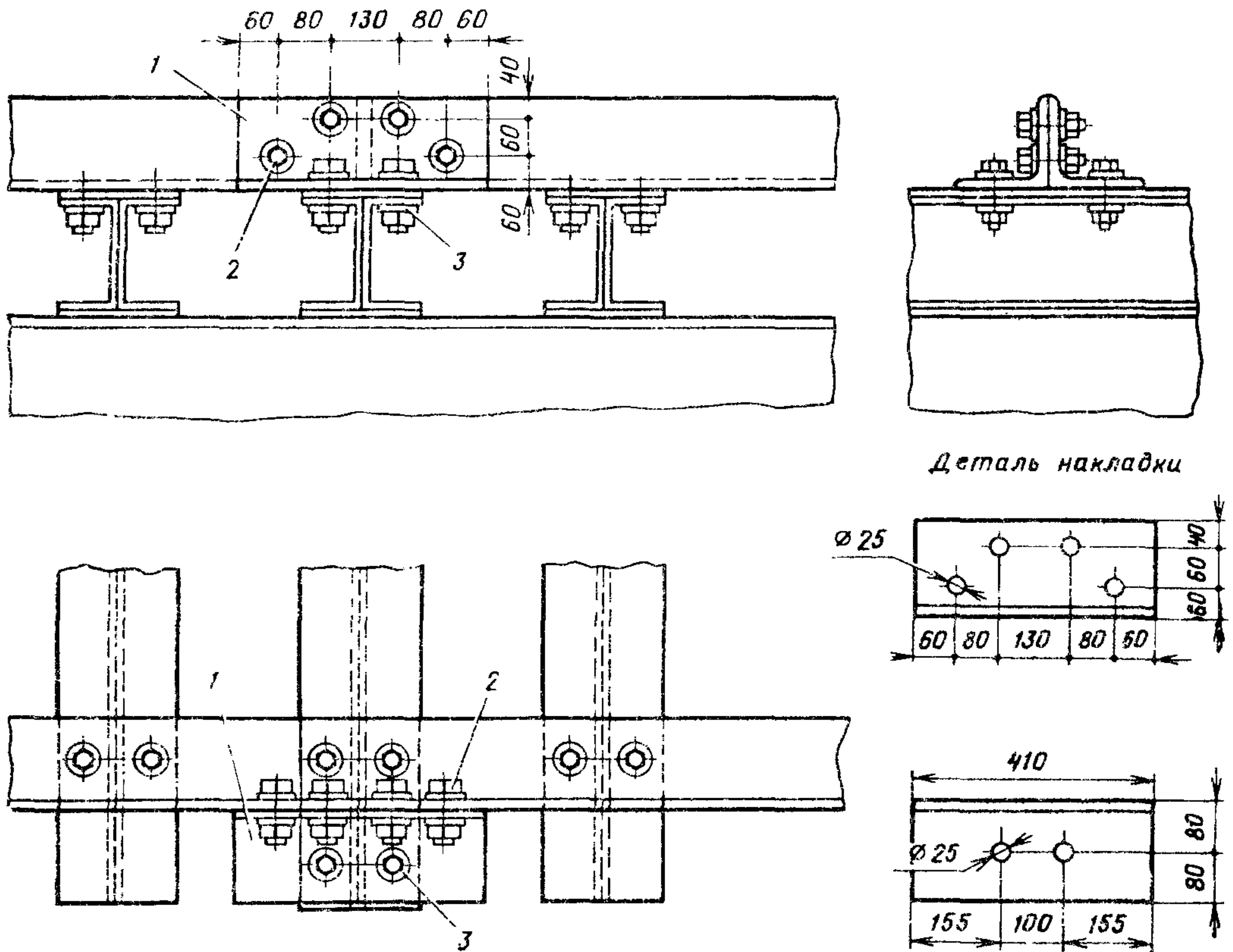
Рис. 35 Стыки противоугольных (охранных) уголков на металлических поперечинах: 1 — стыковая угольковая накладка; 2 — стыковой болт; 3 — высокопрочный болт
