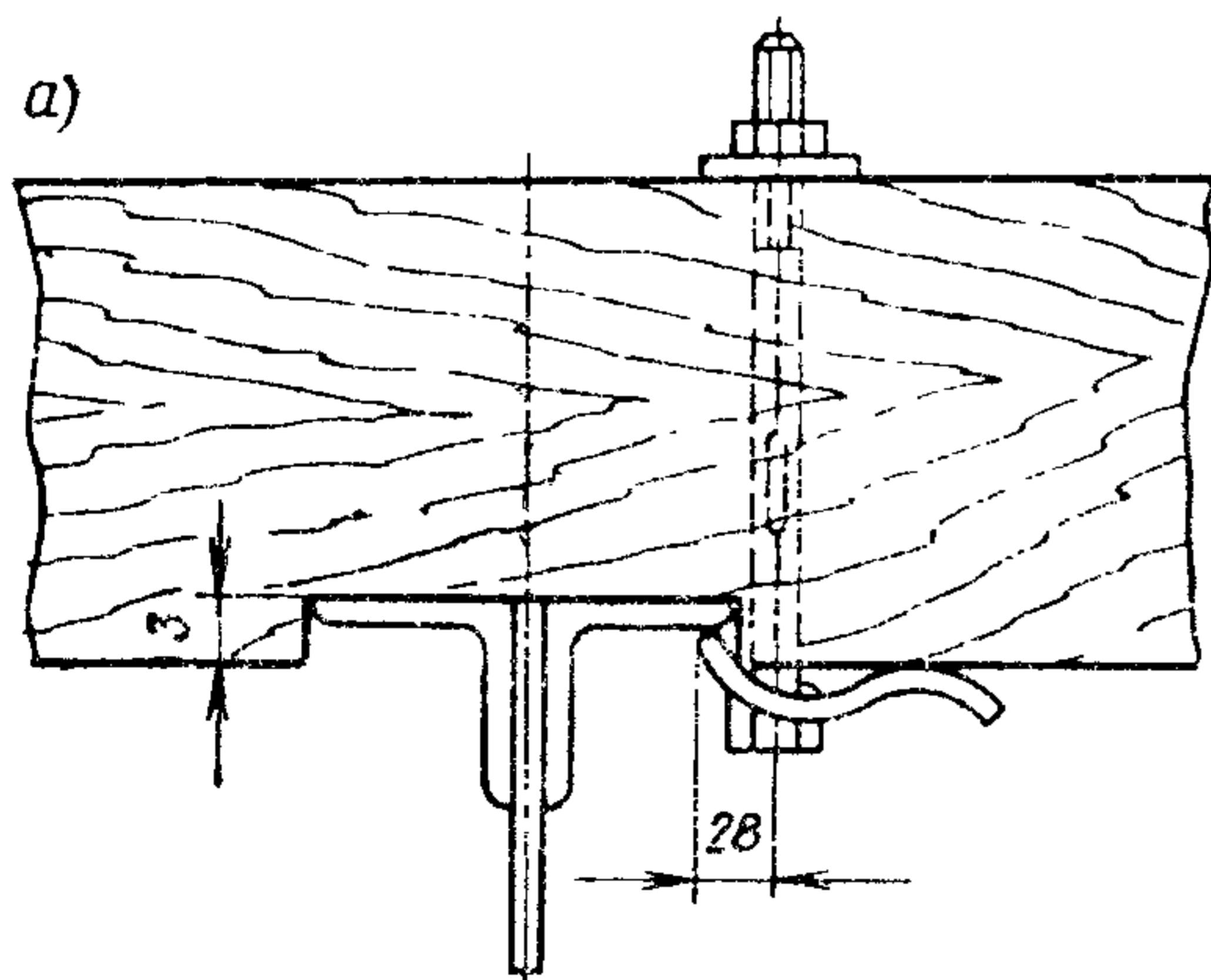
Рис. 3. Схема постановки лапчатого болта с пружинной лапой:
