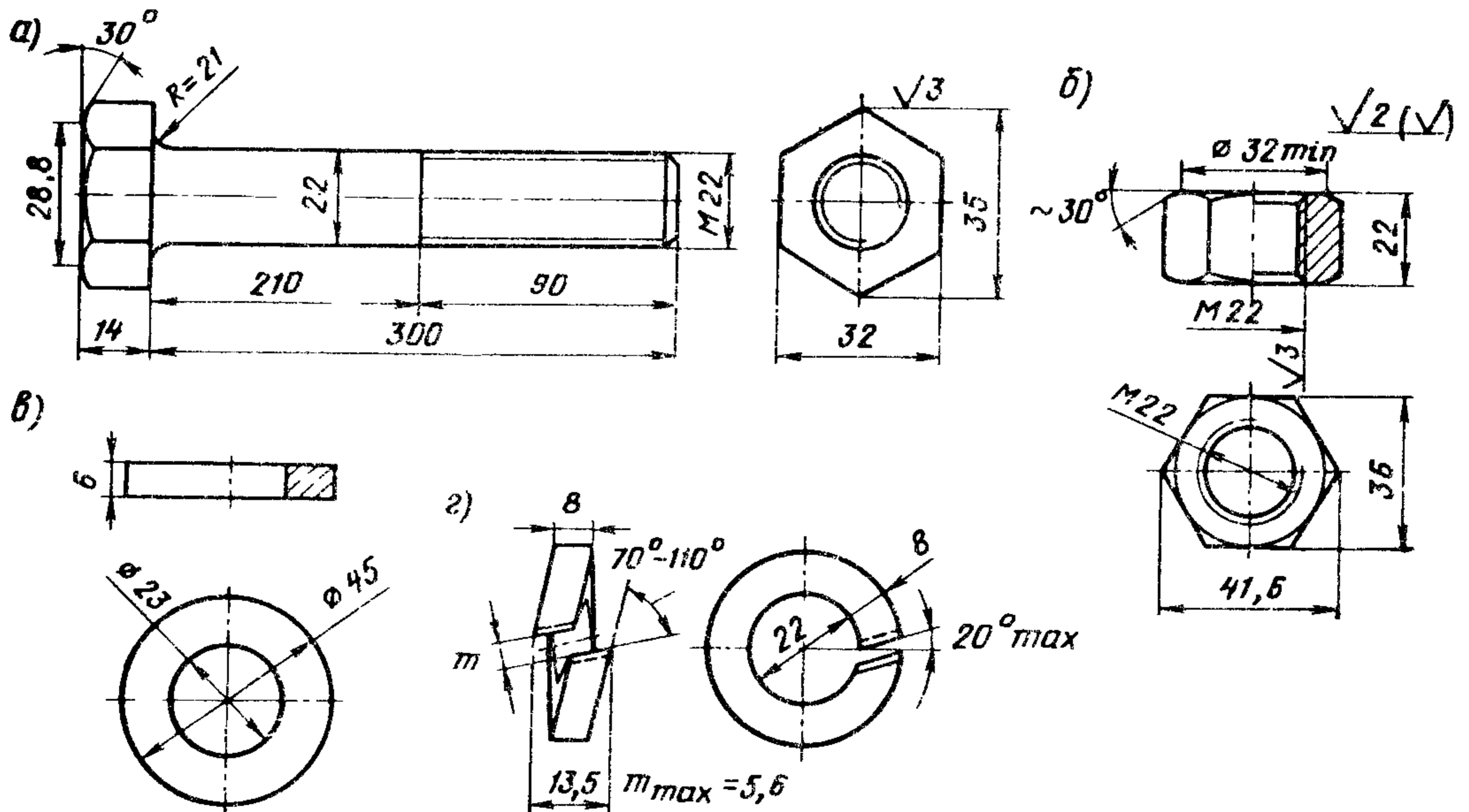
Рис. 5. Болт для прикрепления мостового полотна к пролетным строениям (продольным балкам) через противоугольные (охранные) уголки:
