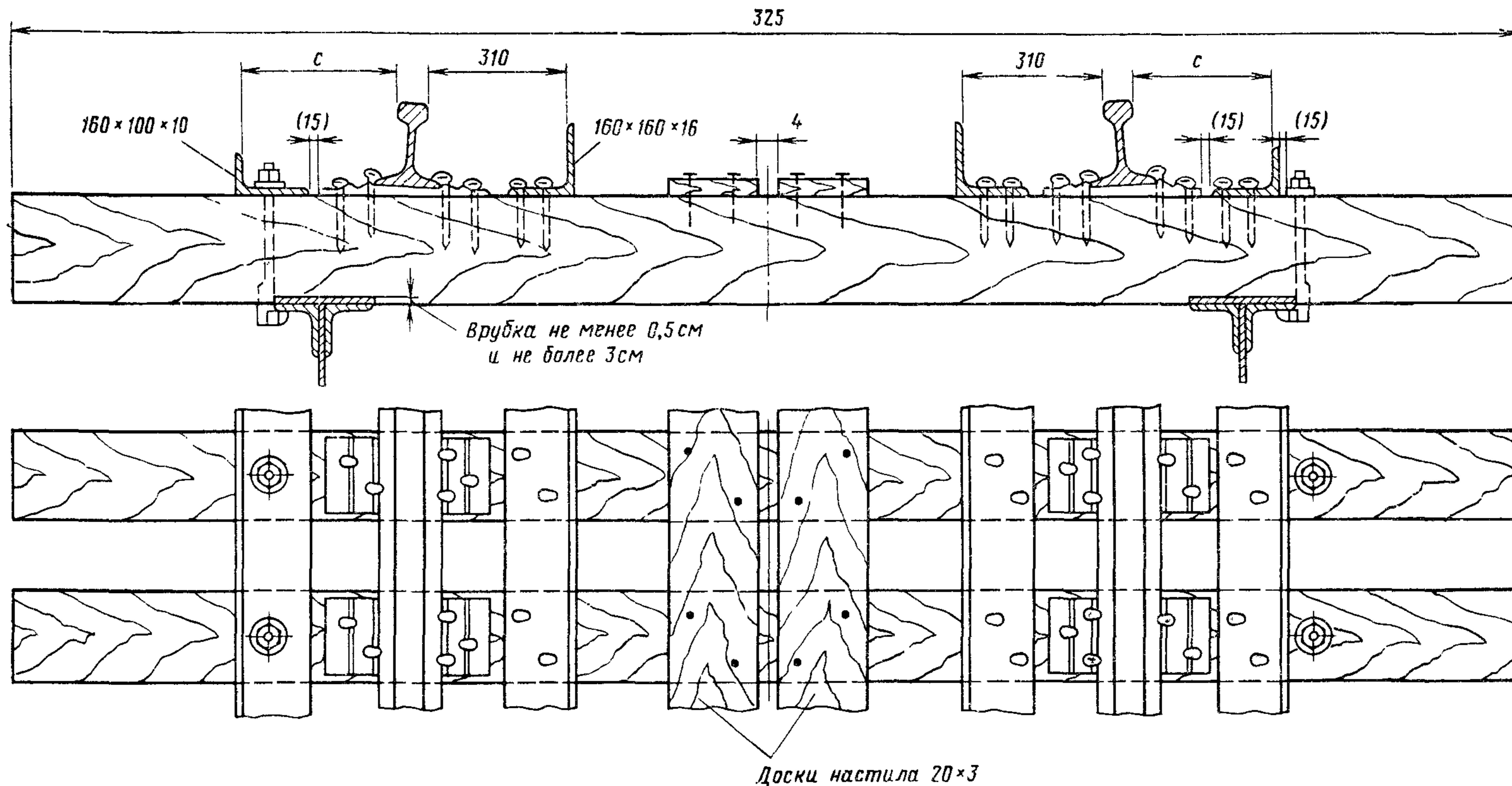
Рис. 6. Мостовое полотно на мостовых брусьях с костыльным креплением рельсов:
