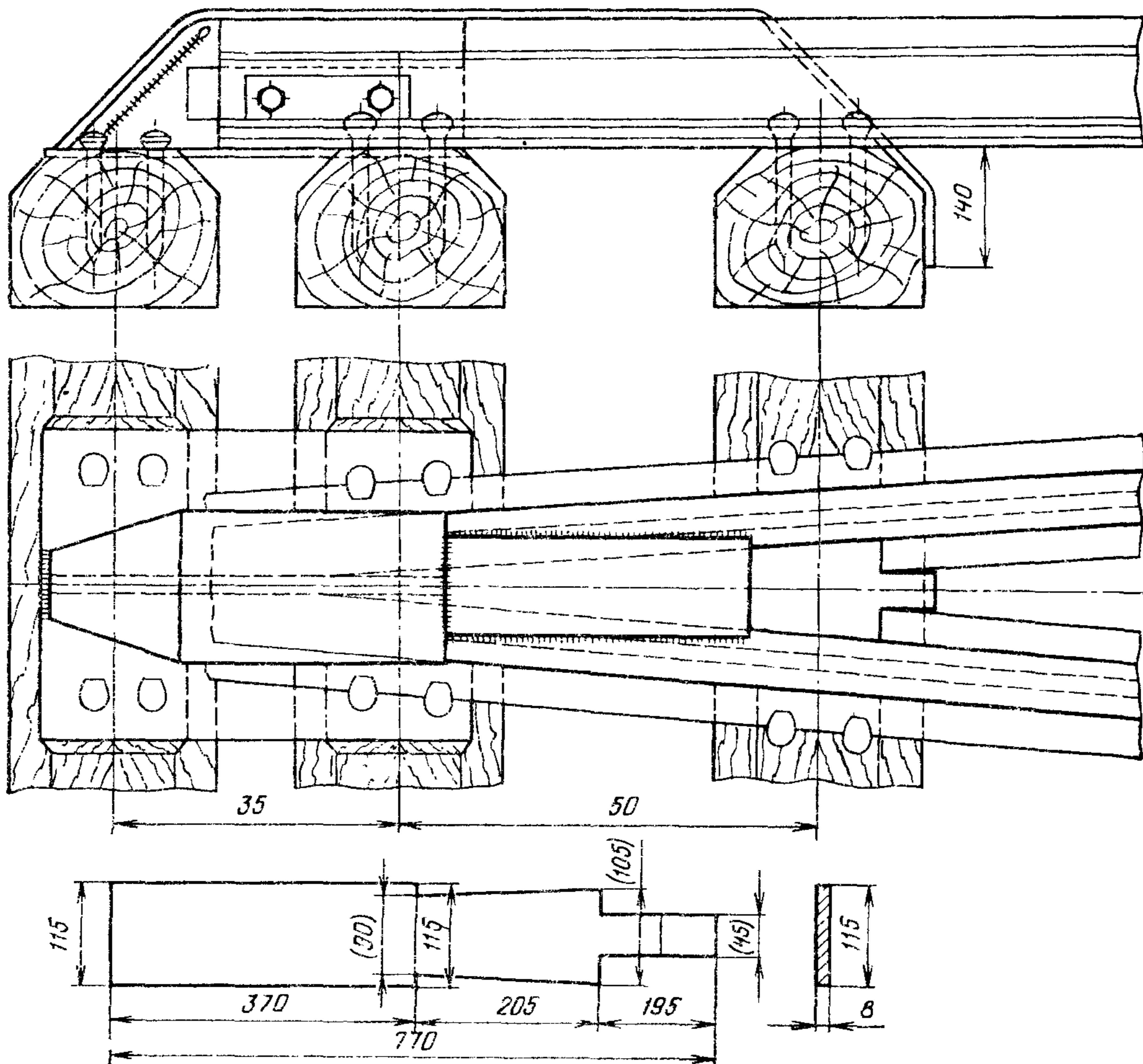
Рис. 31 Укрытие хвостовой части башмака челюока контррельсов без замены сердечника.
