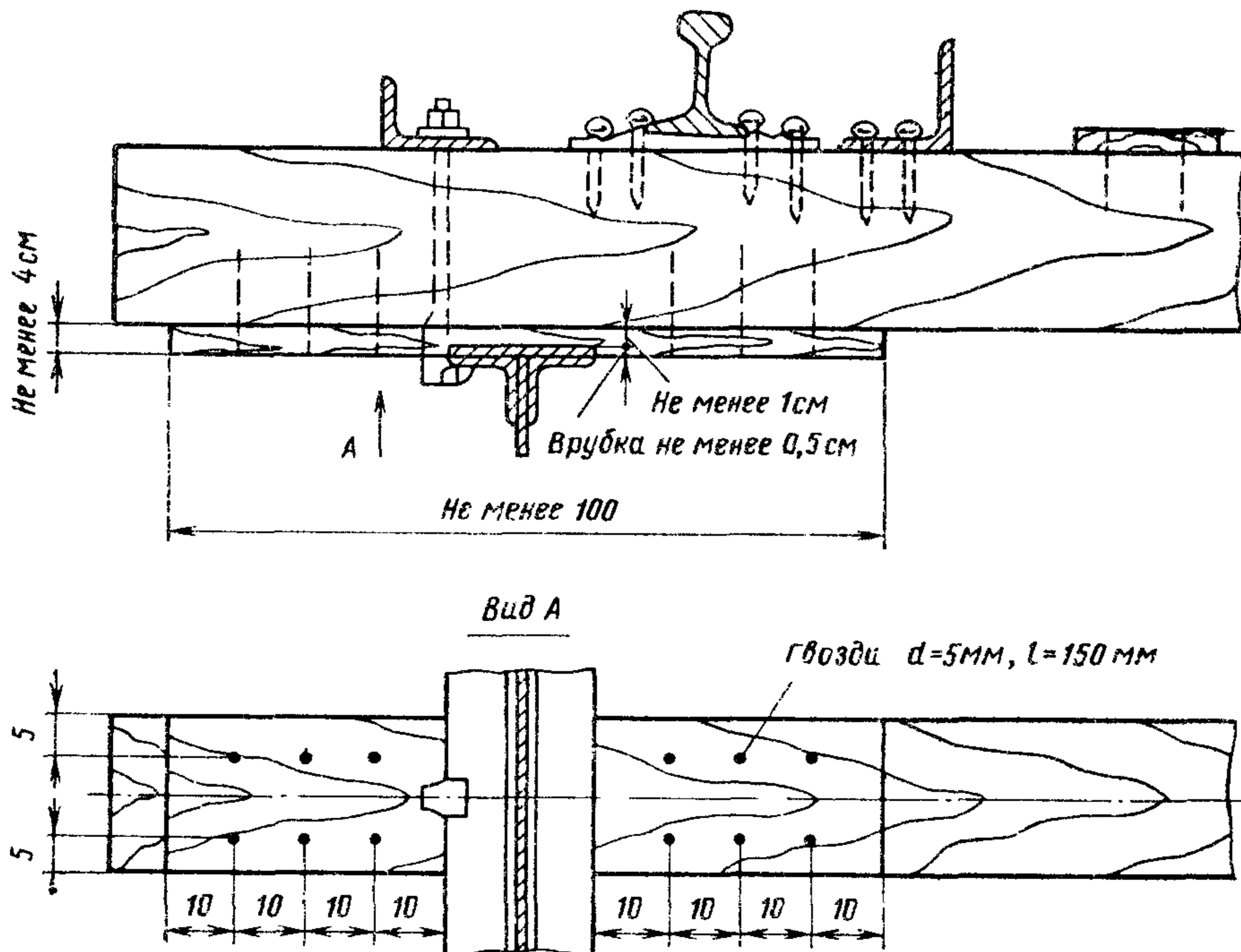
Рис. 11. Увеличение высоты мостового бруса подкладкой доски
