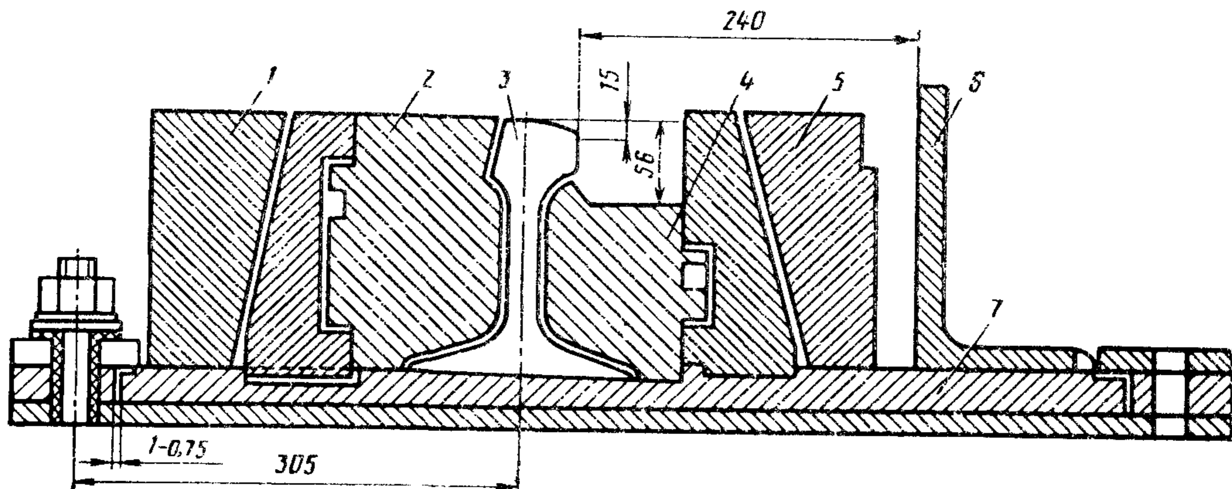
Поперечный разрез рельсового замка в месте стыка:
