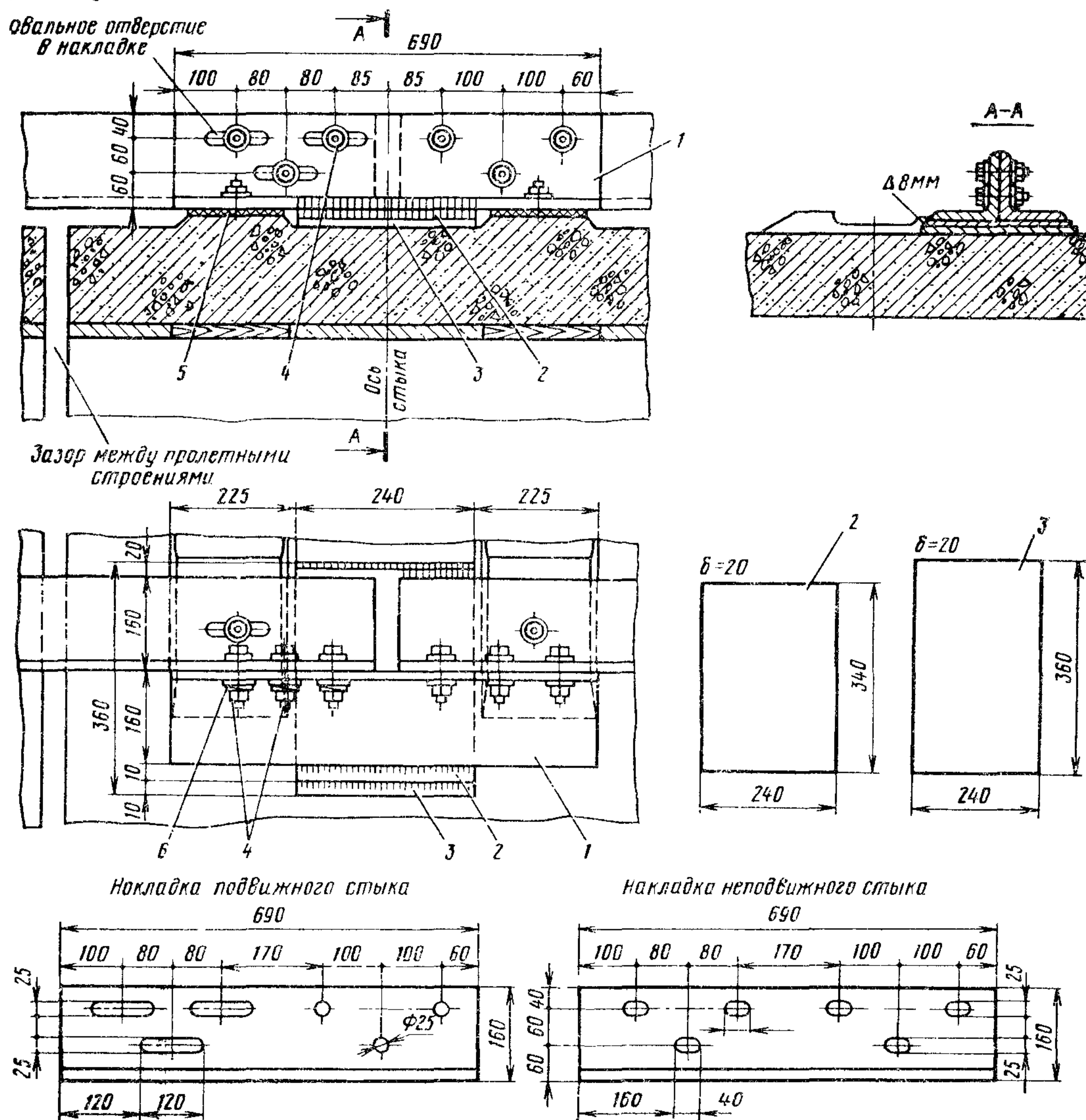
Рис. 24. Стык контруголков на безбалластных плитах:
