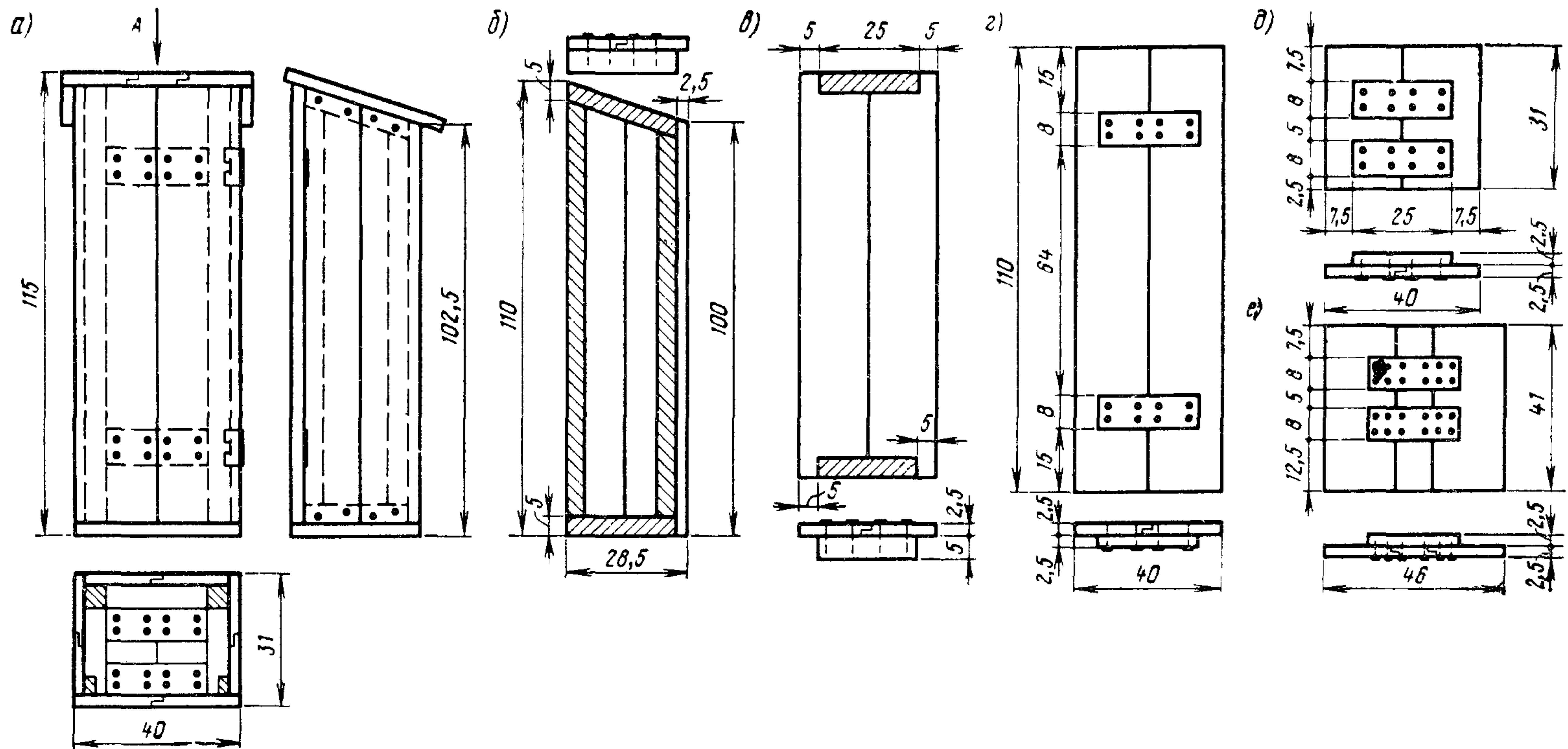
Рис. 3. Ящик для двух обогревателей: а — общий вид; б — боковая стенка; в — задняя стенка; г — дверь; д — дно; е — крышка
