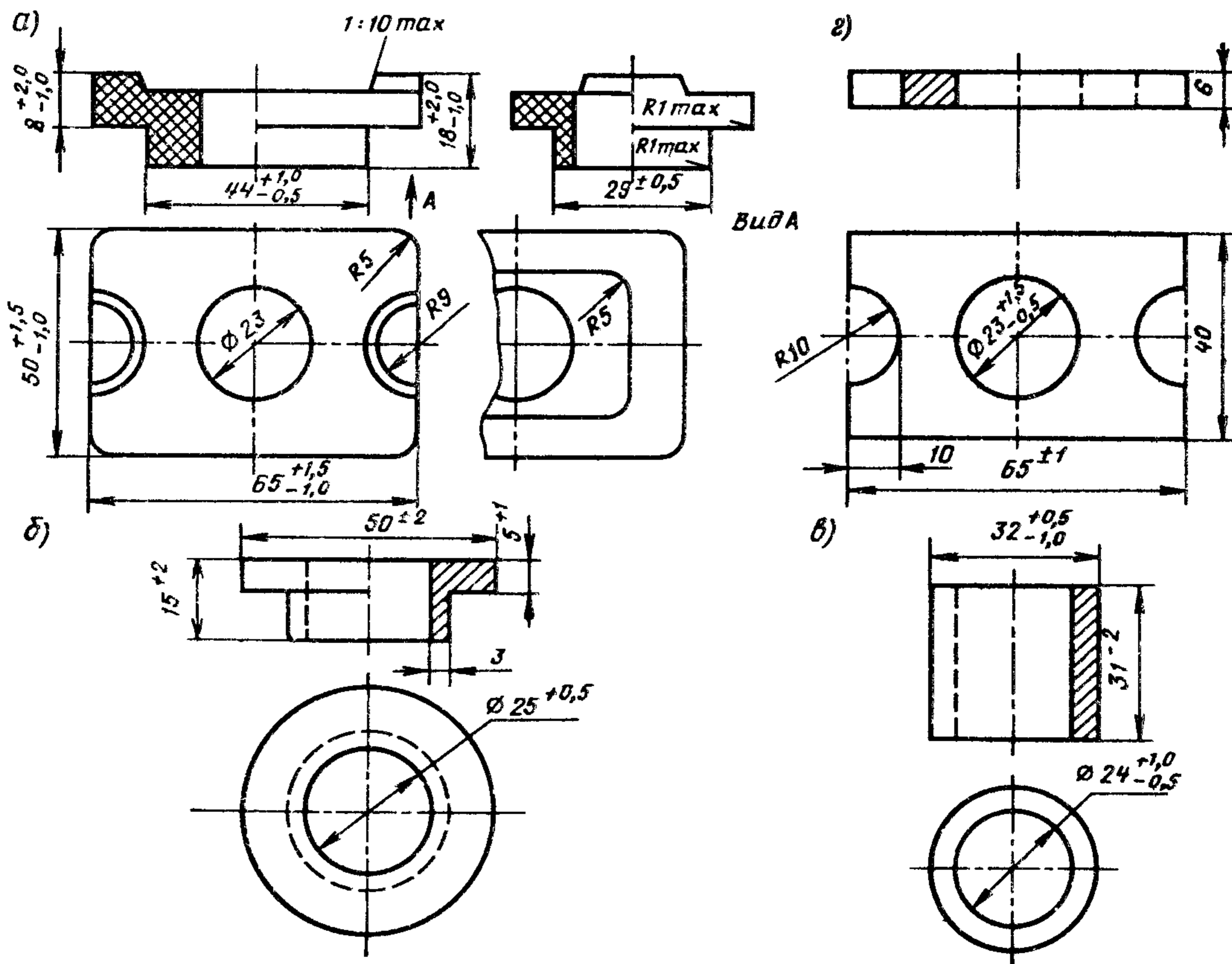
Рис. 5. Изолирующие втулки и трубки:
