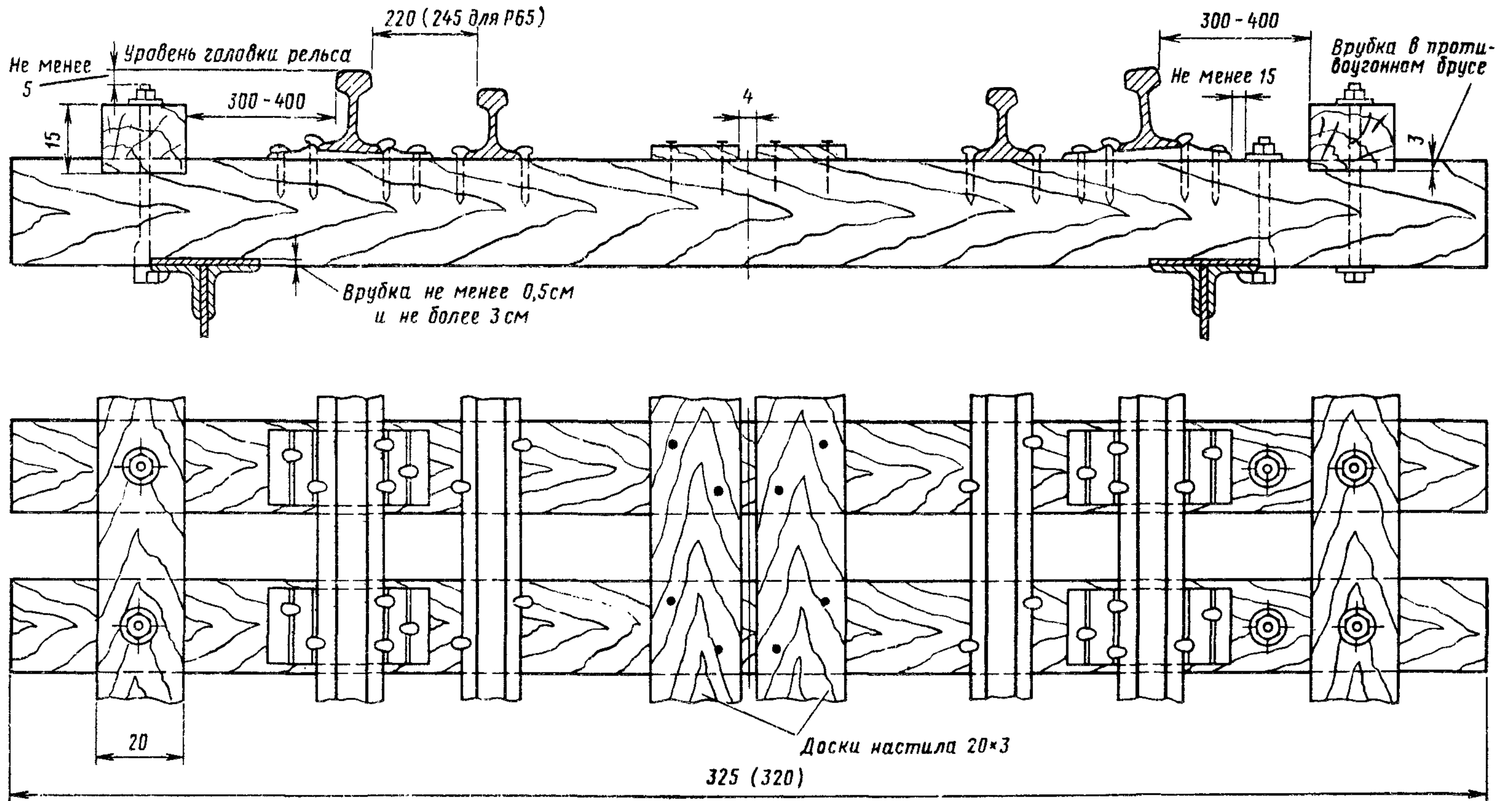
Рис 8. Мостовое полотно на мостовых брусьях с контррельсами и противоугонными (охранными) брусьями: слева - мостовые и противоугонные брусья прикреплены общим лапчатым болтом; справа -- мостовые и противоугонные брусья имеют раздельное крепление. П р и м е ч а н и е. Контррельсы должны быть не более чем на один тип легче путевых рельсов. Настил внутри колеи показан при наличии на пролетном строении боковых тротуаров, при их отсутствии внутри колеи должно быть три доски. В скобках дана длина мостовых брусьев по старому ГОСТу
