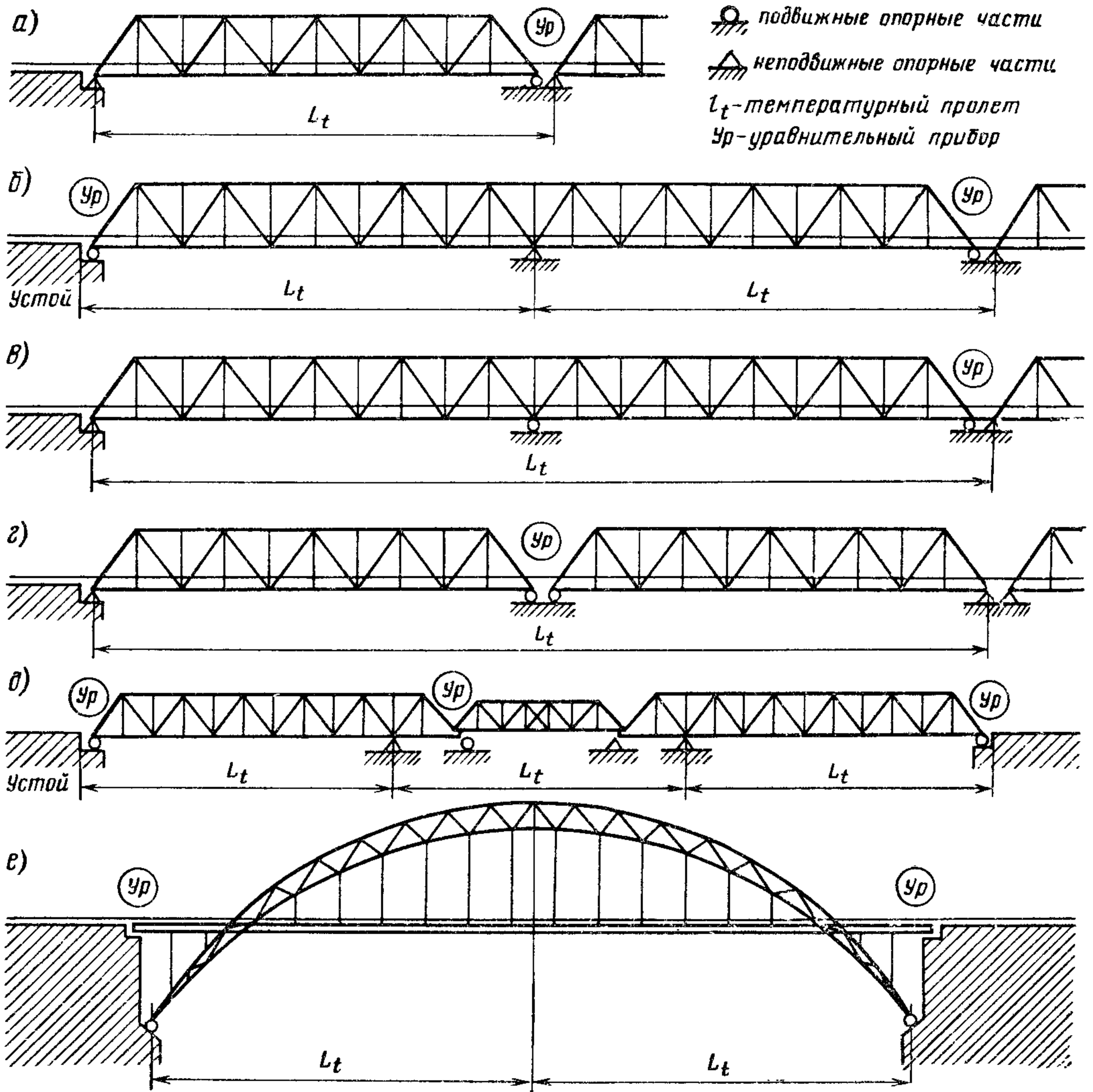
Рис. 20. Температурные пролеты мостов:
