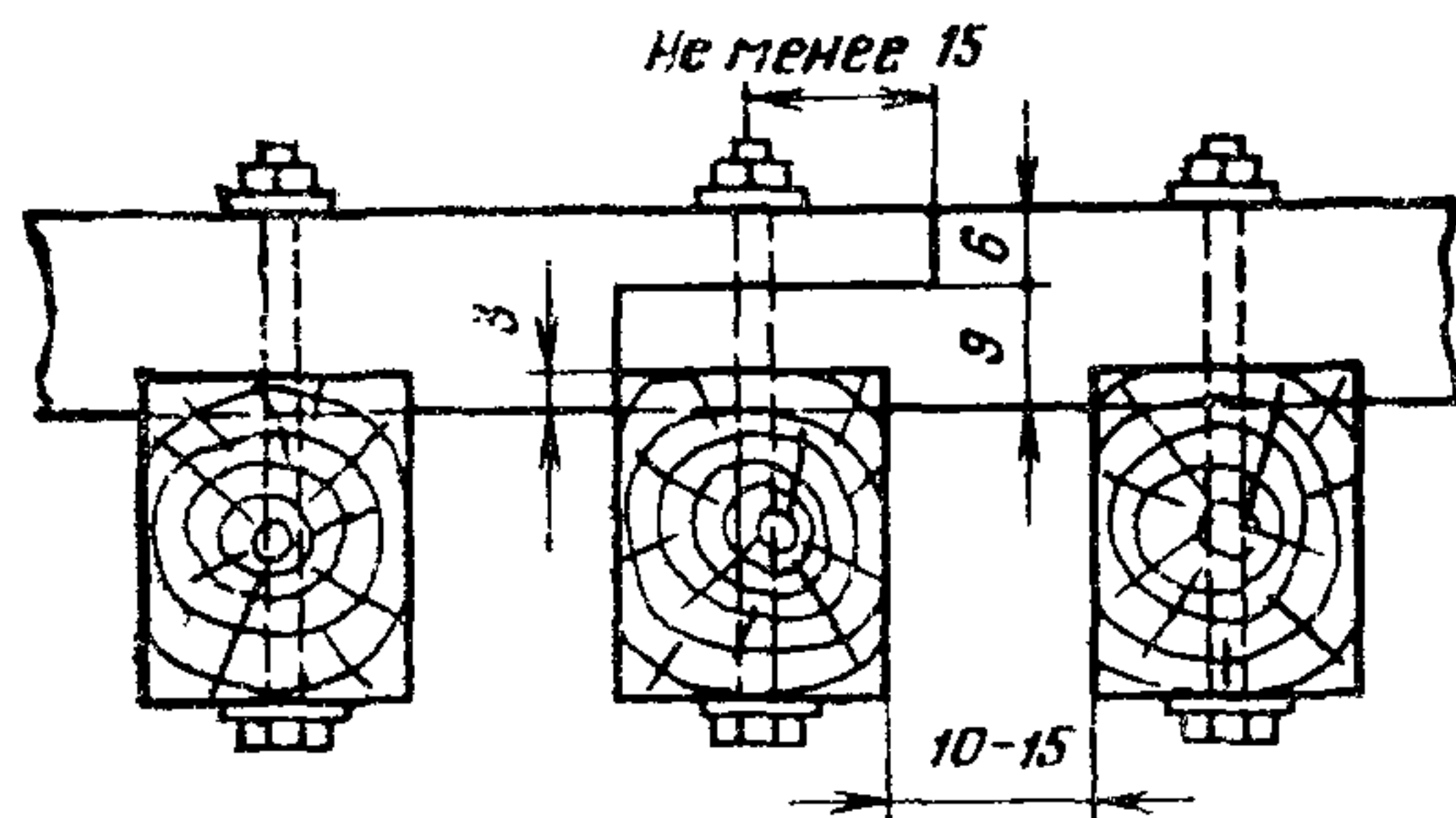
Рис. 37. Стык охранных брусьев
