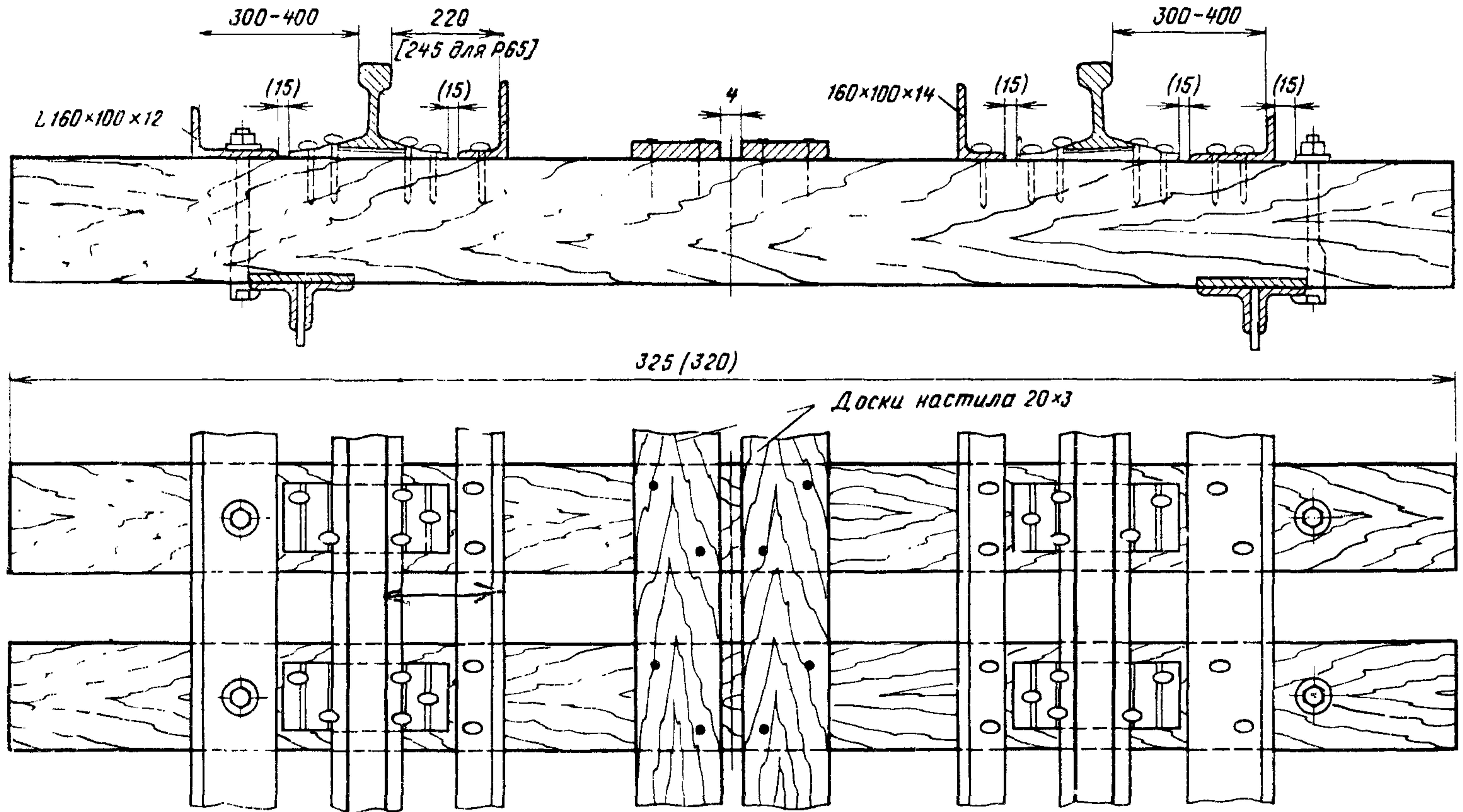
Рис. 9. Мостовое полотно на мостовых брусках с неравнобокими контруголками: слева — противоугонный уголок прикреплен лапчатым болтом; справа — то же костылями.
