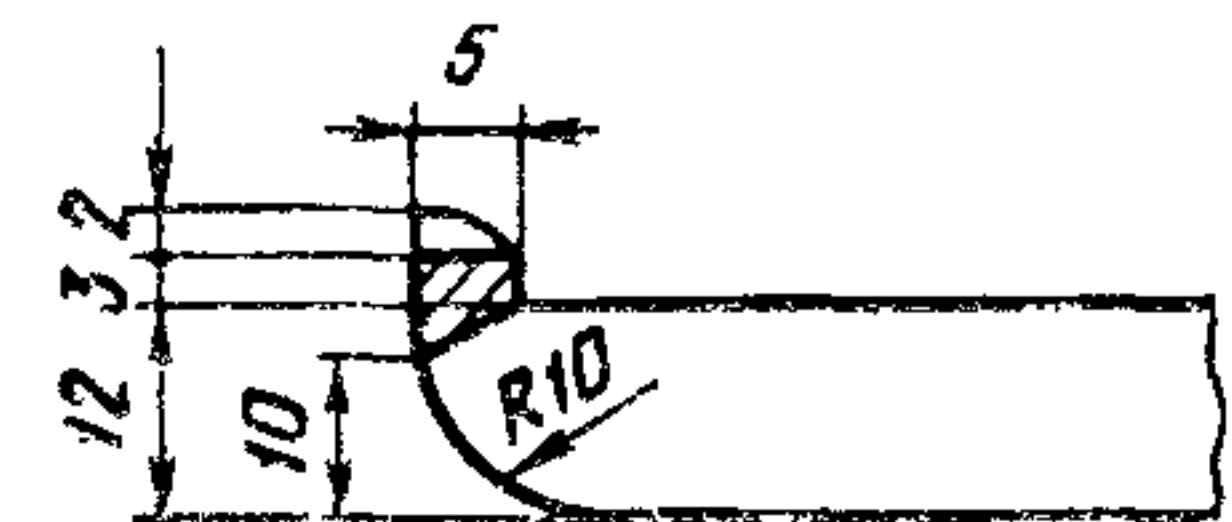
Предельные допускаемые очертания продольных кромок подкладки
