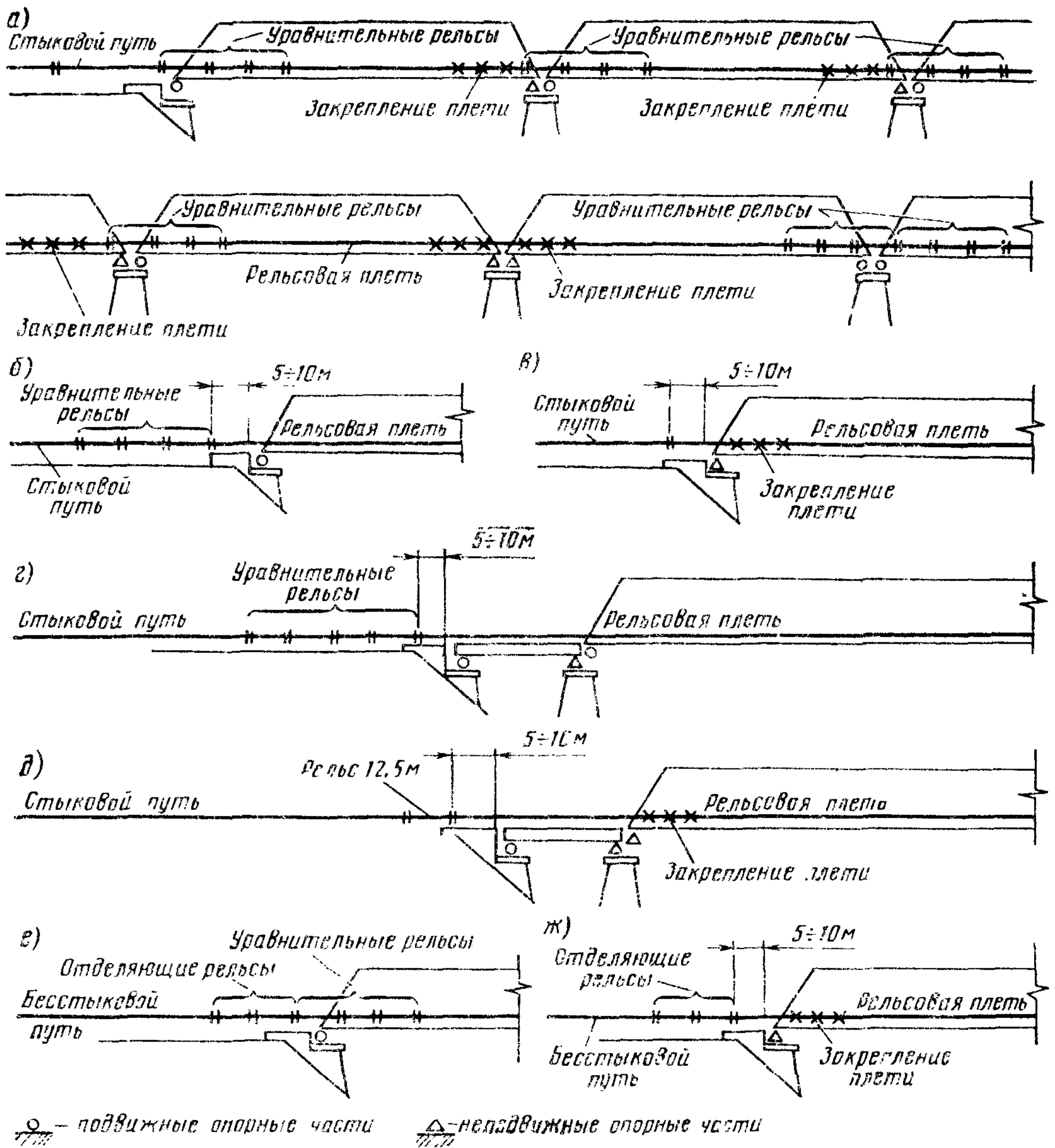
Рис 1. Схемы укладки уровнительных рельсов на мостах
