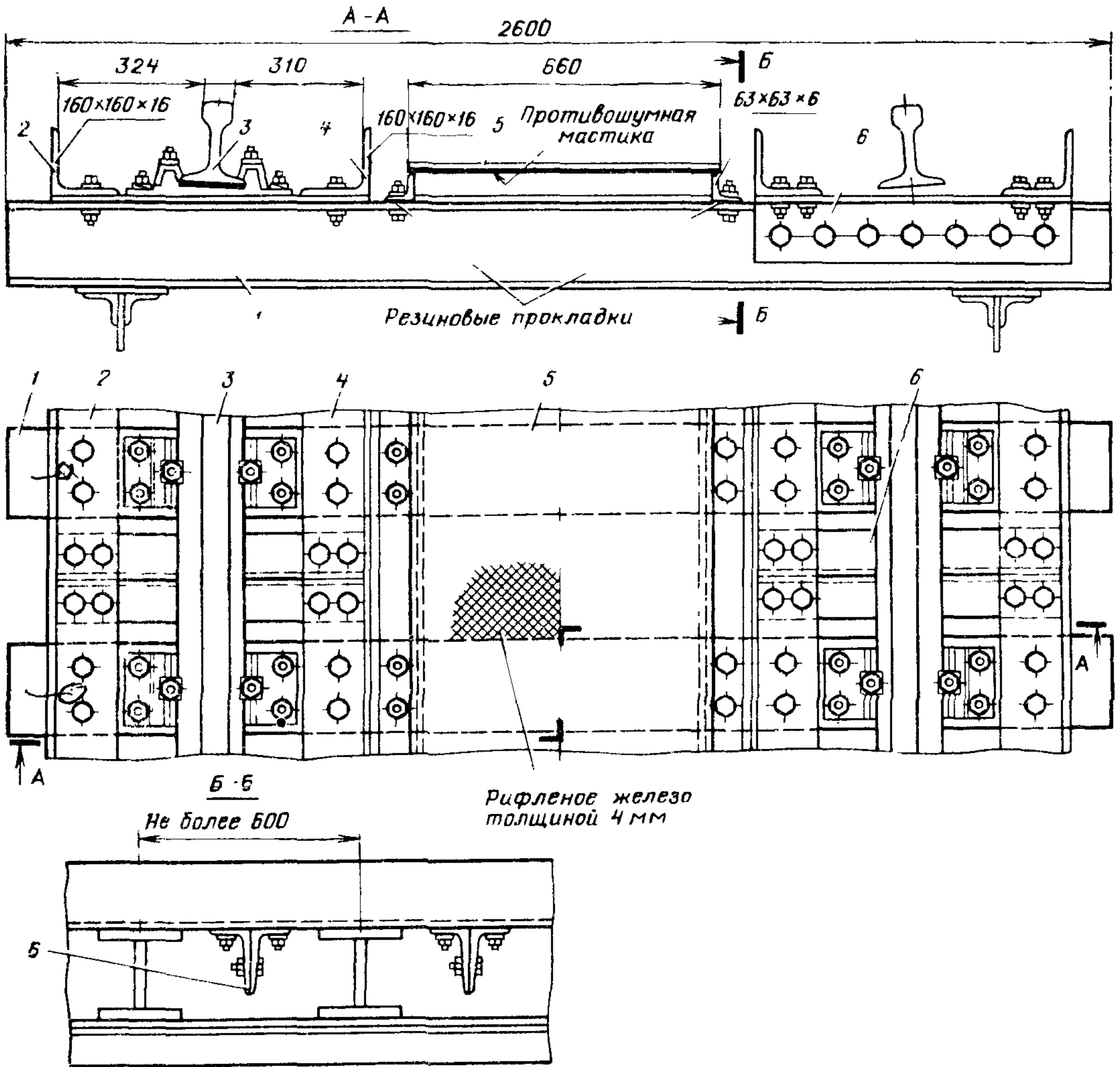
Рис. 14. Мостовое полотно на металлических поперечинах:
