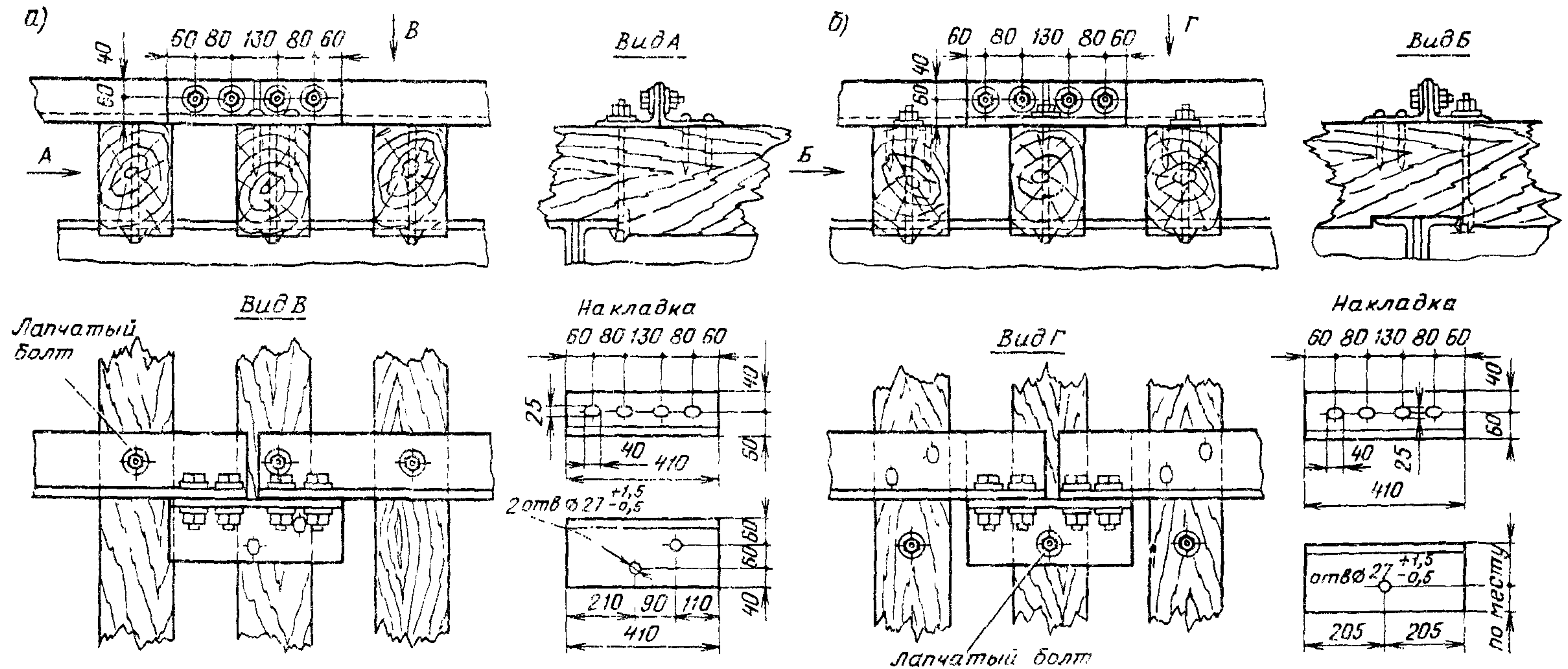
Рис. 34. Стыки противоугонных (охранных) уголков на мостовых брусках:
