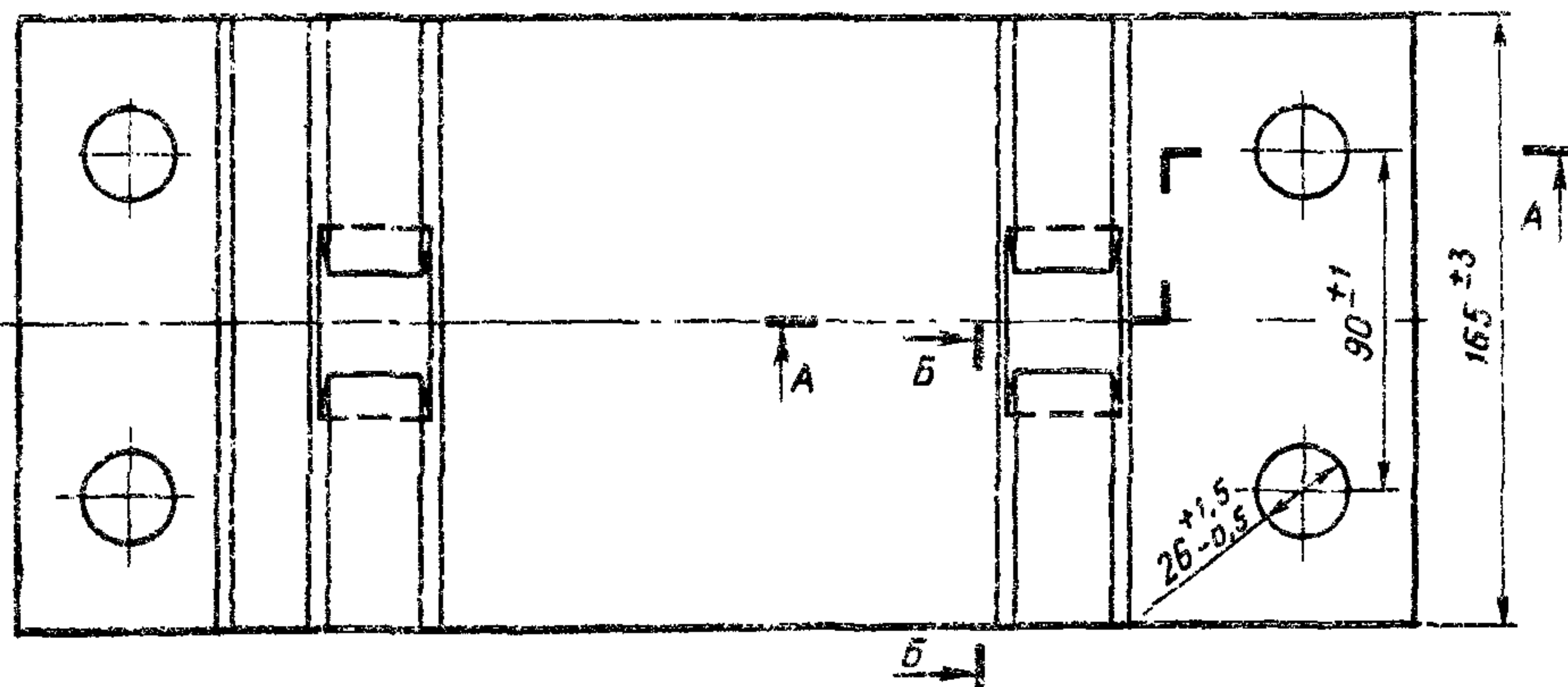
Рис. 2. Рельсовая подкладка КД50 (ЦП 14-72)
