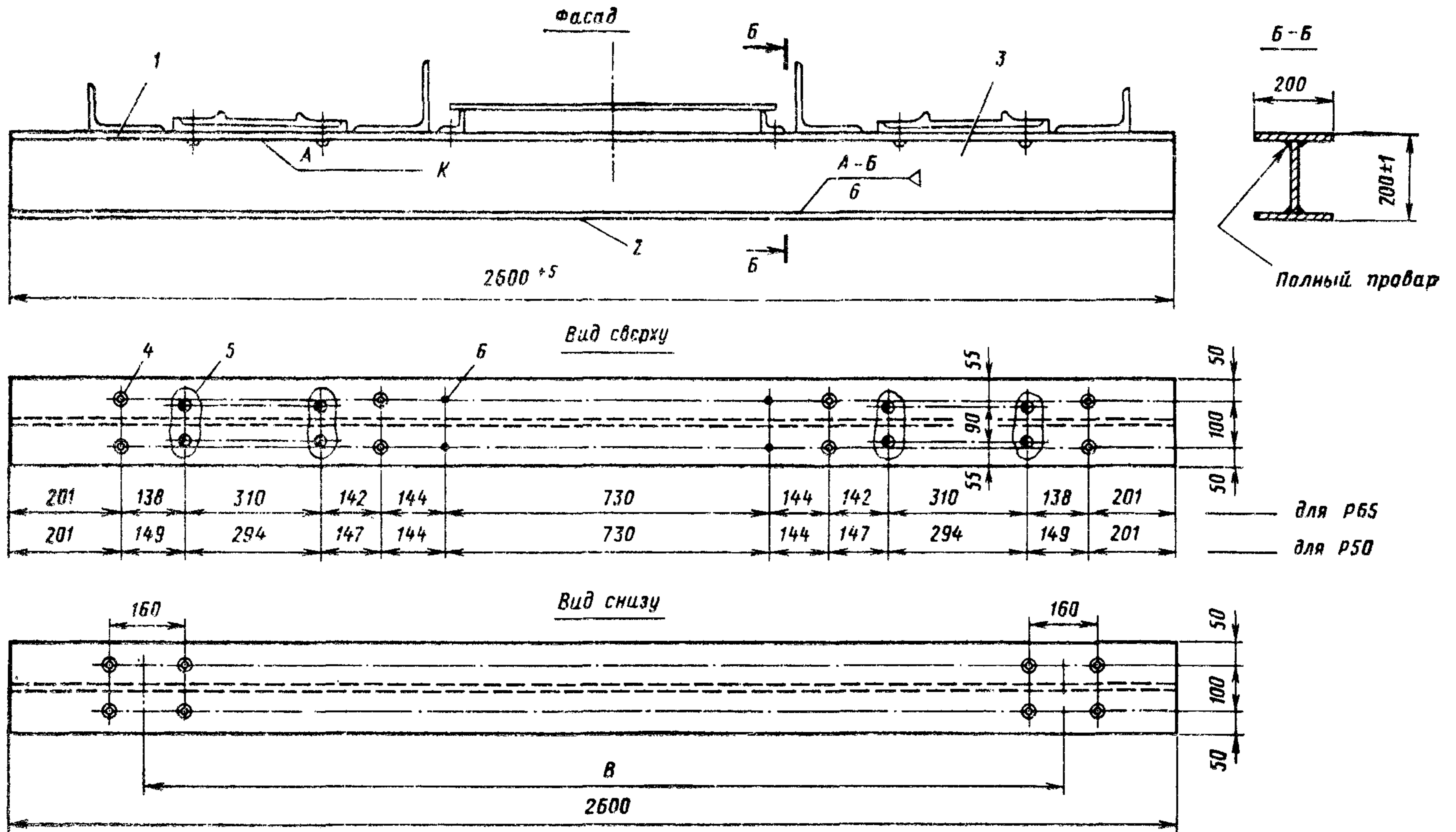
Рис. 2. Металлическая сварная поперечина:
