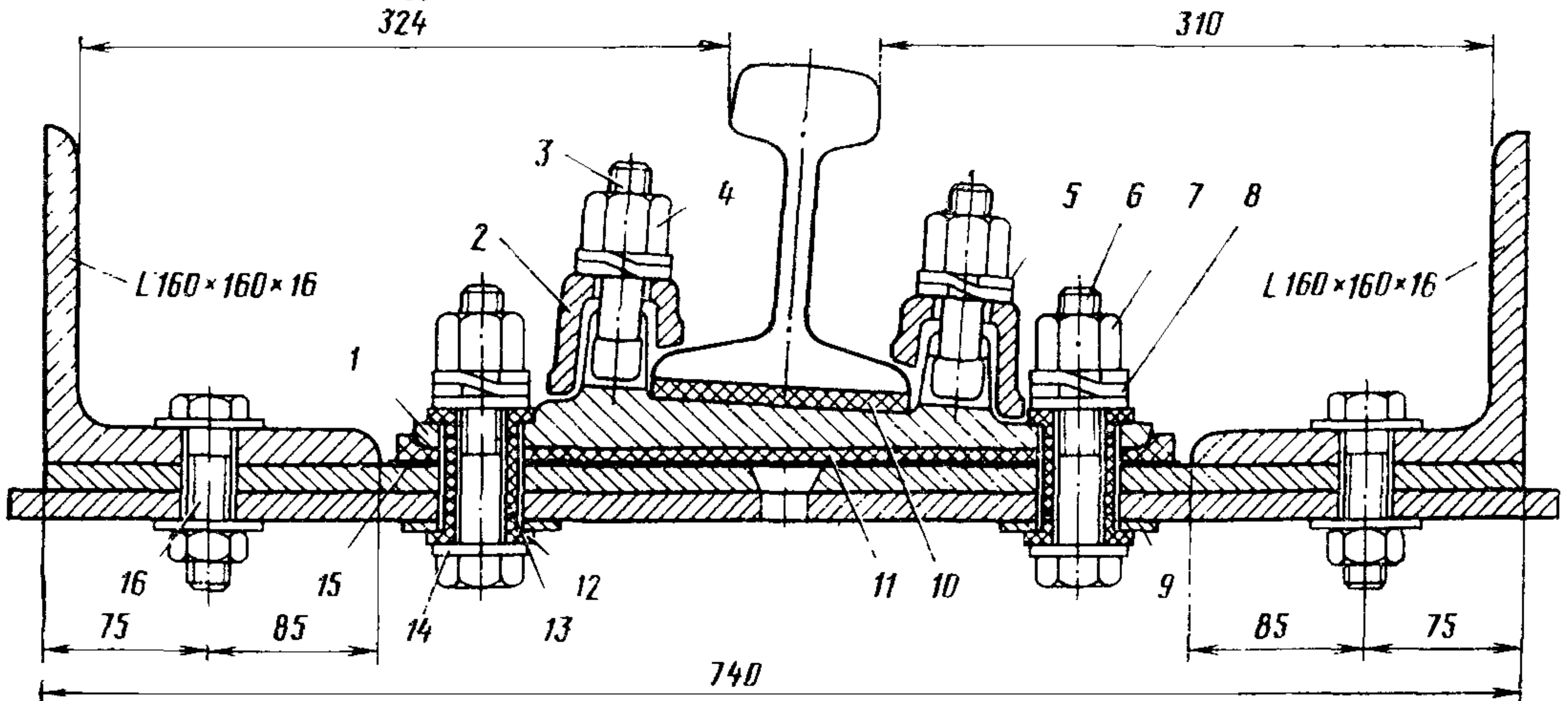
Рис. 14. Мостовое полотно на металлических поперечинах:
