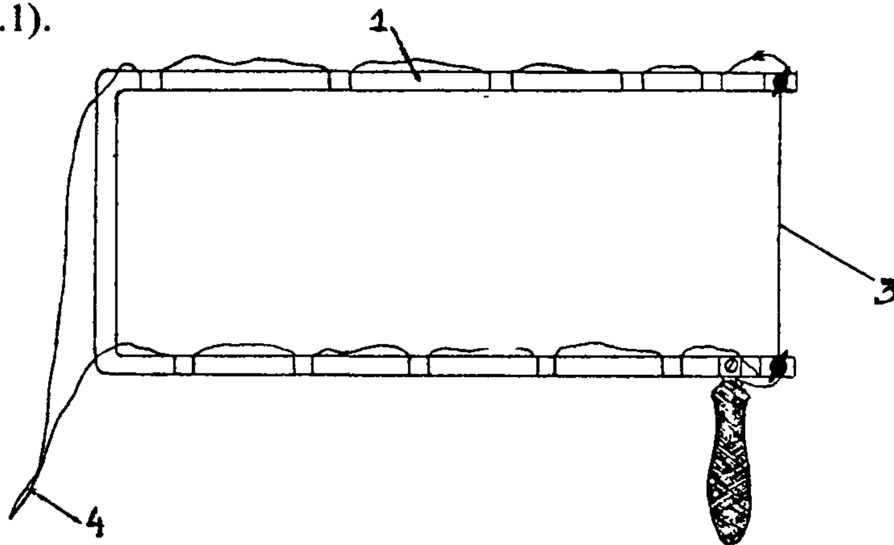
Рис. 3.1. Электропрожигающий лобзик 1- дуга, 2 - рукоятка, 3 - нихромовая проволока, 4 - электрошнур
