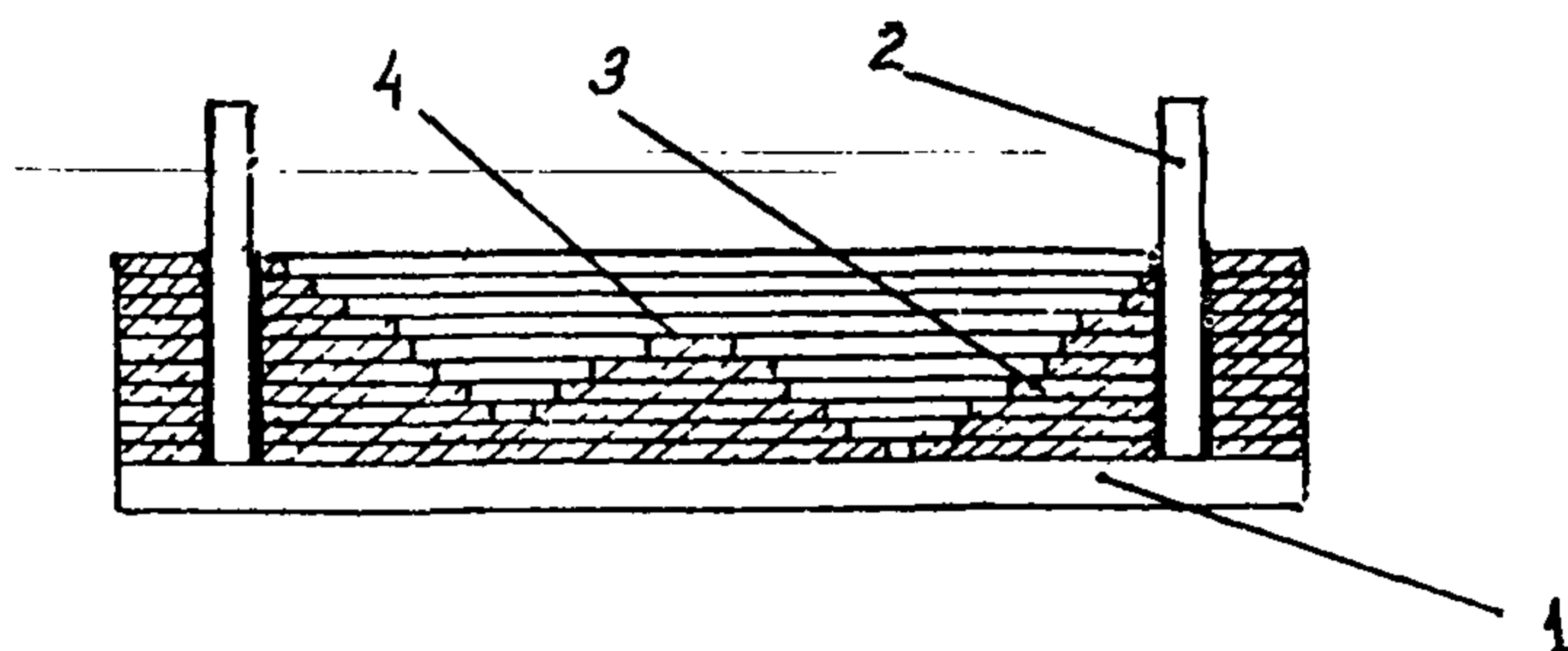
Рис. 3.5 Негативная ступенчатая рельефная модель 1 - основа; 2 - штифты; 3,4 - картонные слои
