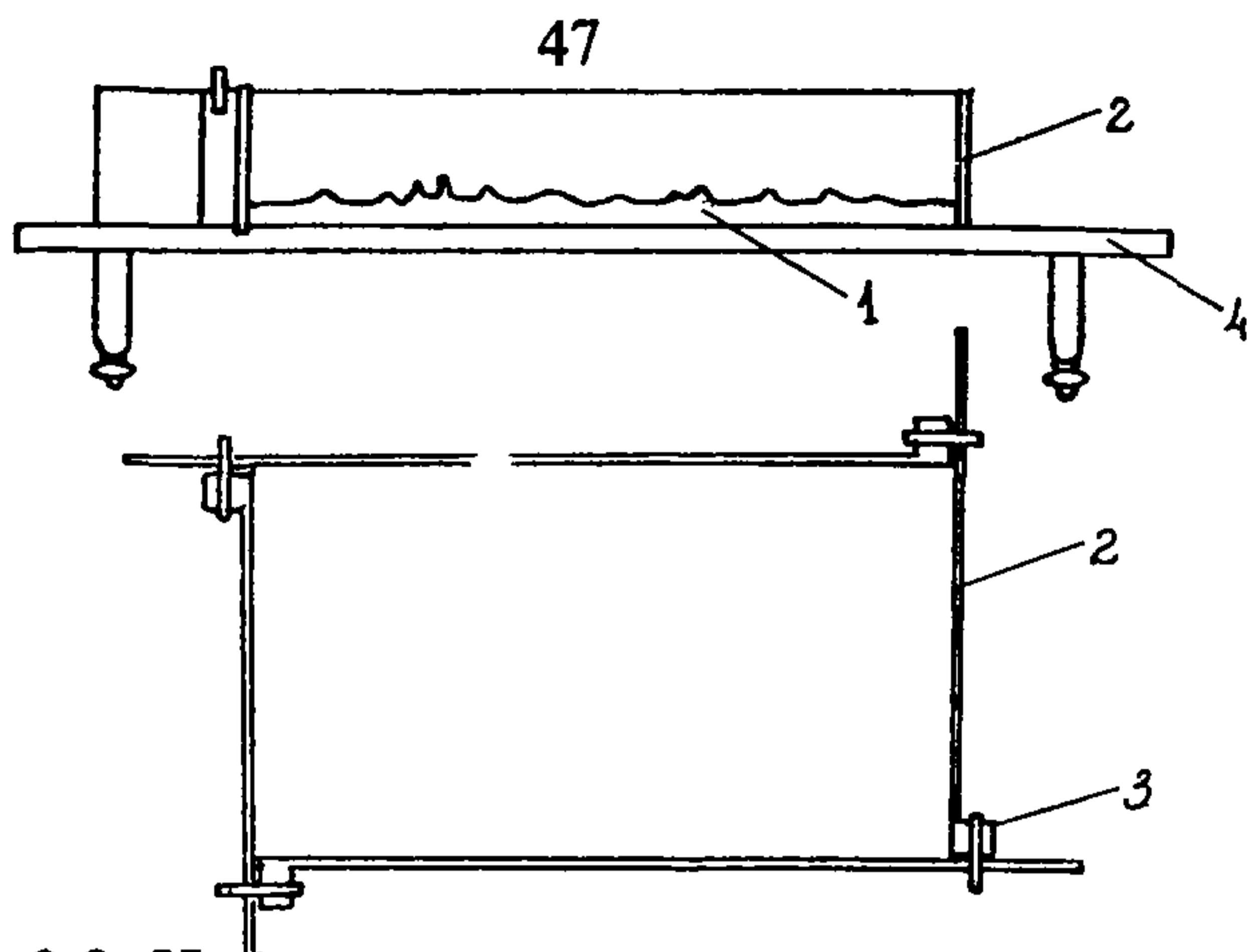
Рис.3.9. Исходная модель, заключенная в опалубку на формовочном столе
