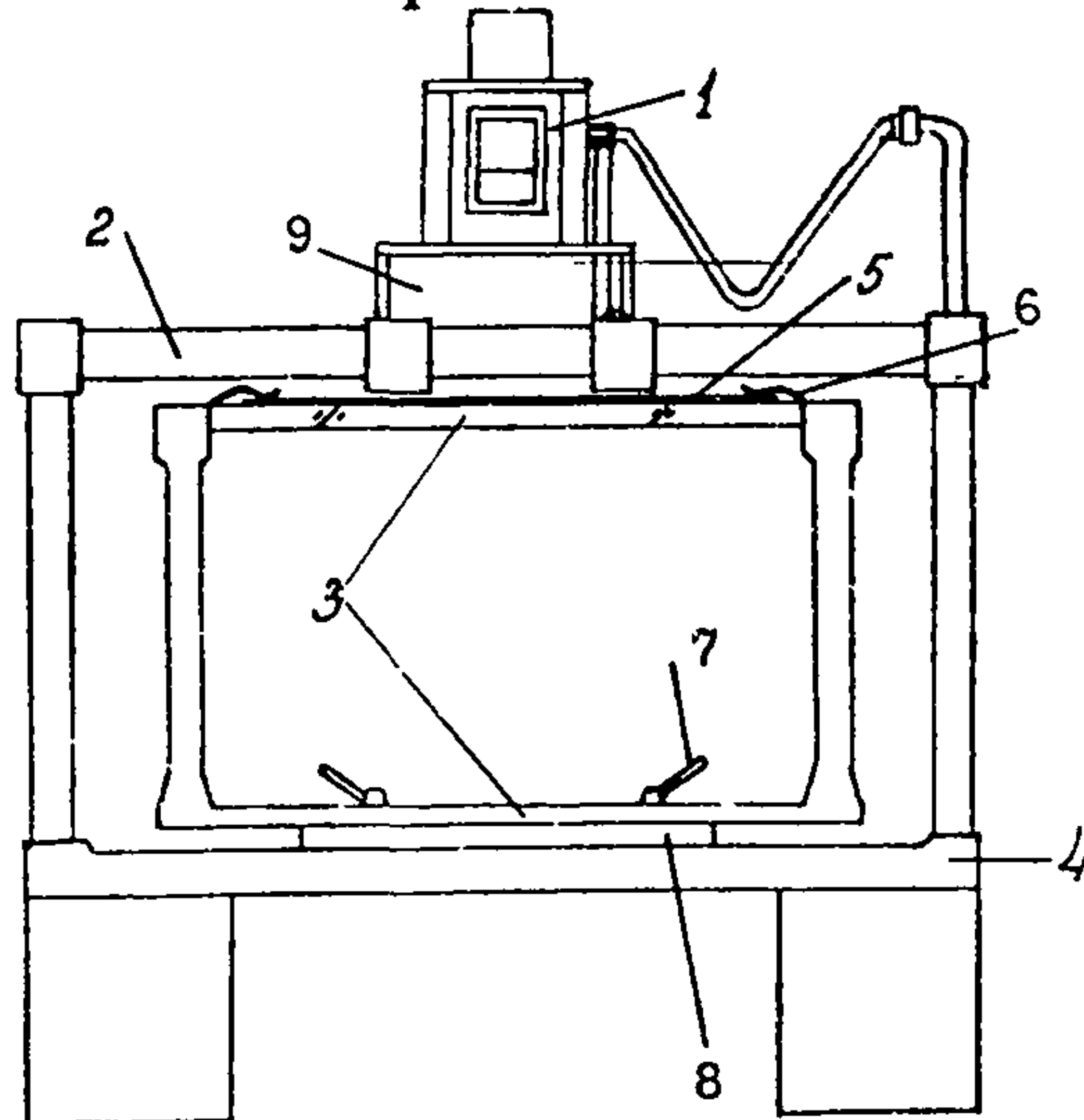
Рис. 3.8. Теневой проектор
