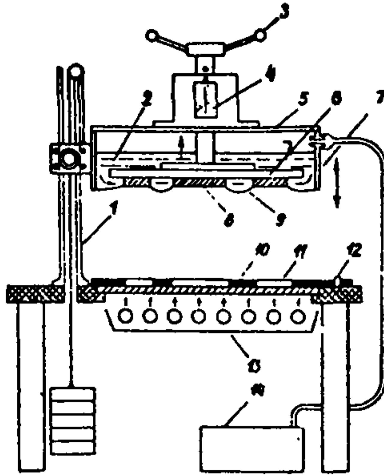
Рис.3.6. Принципиальная схема копирующей установки
