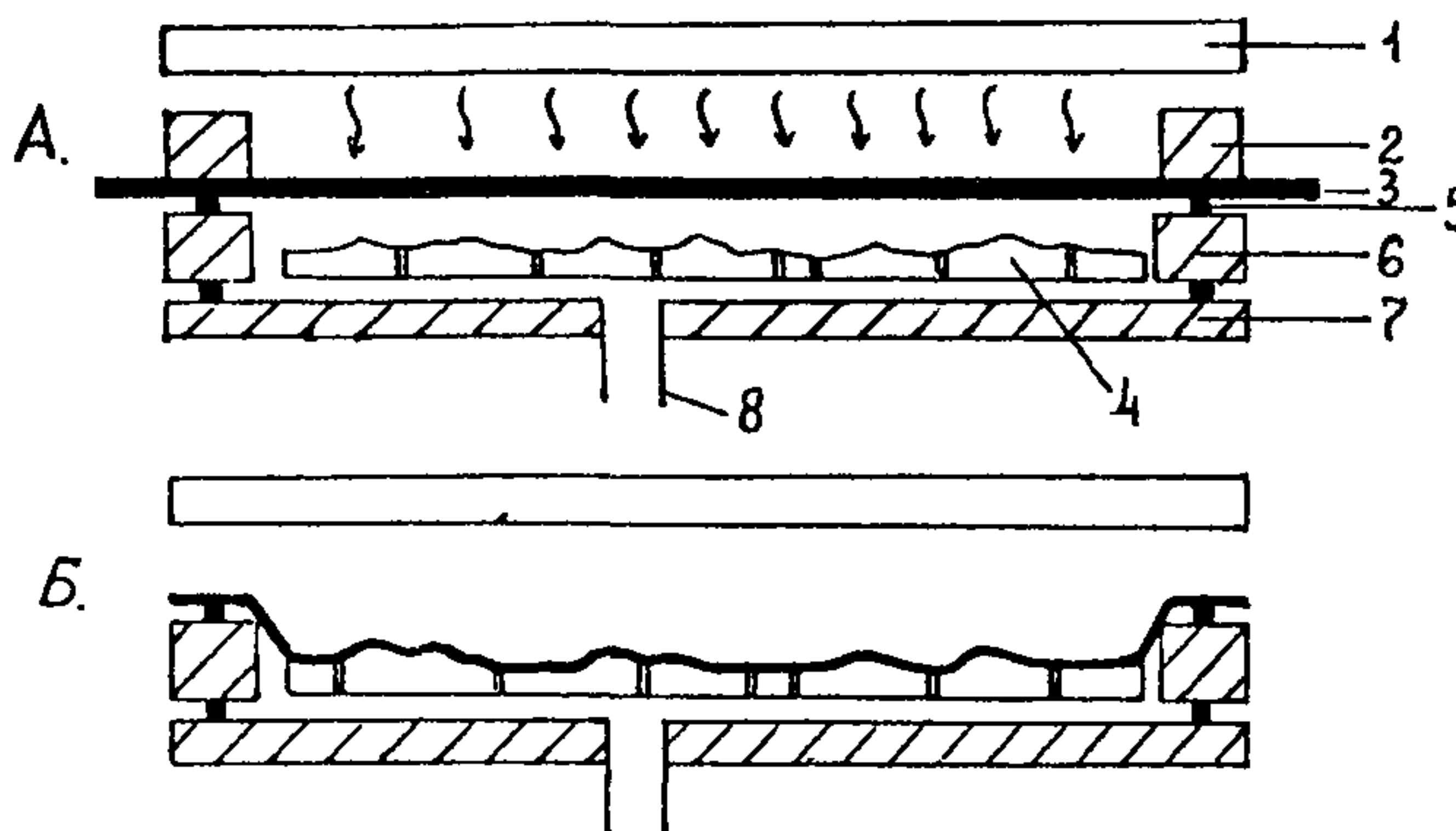
Рис. 4.1. Принципиальная схема устройства вакуум-формовочной машины
