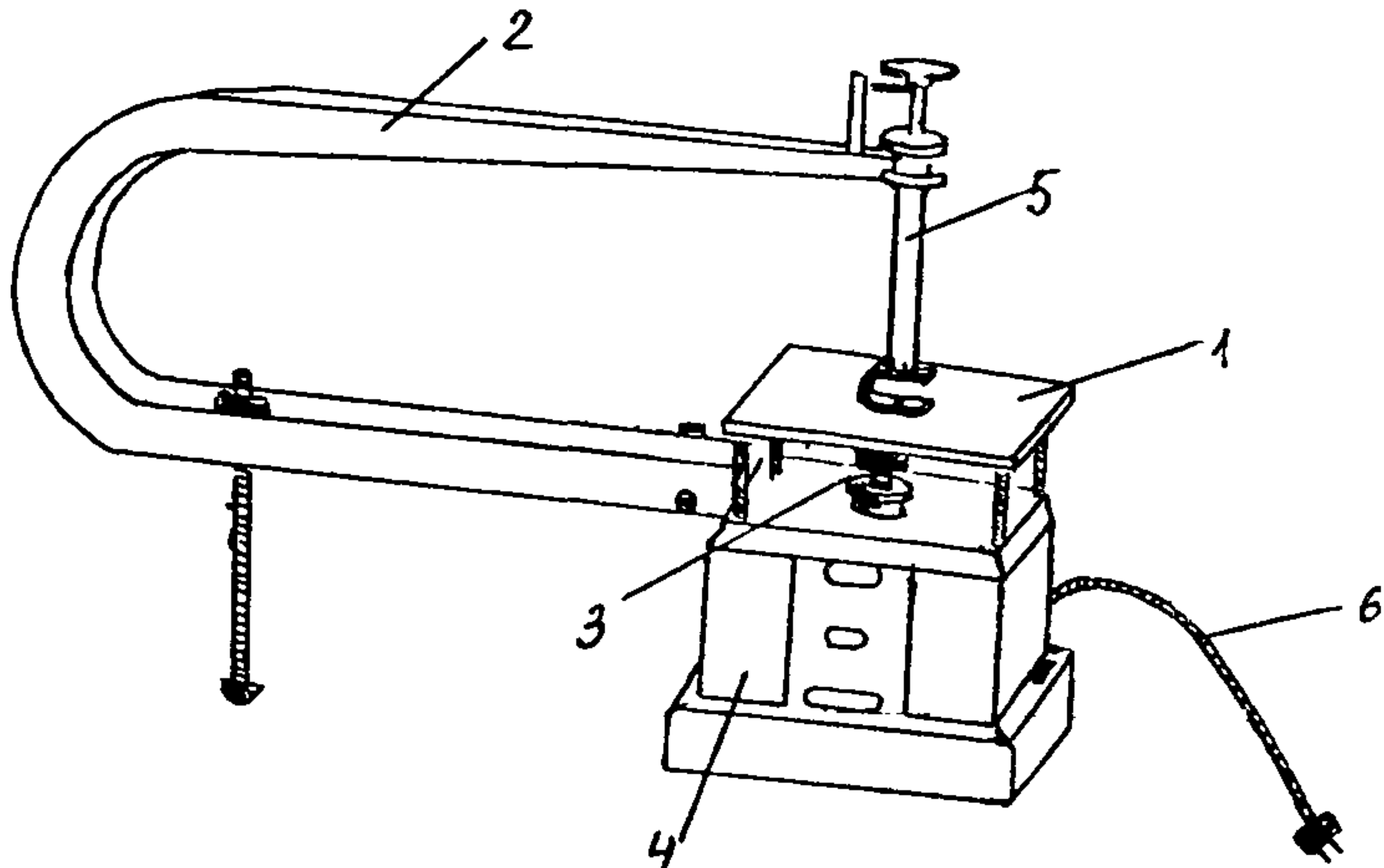
Рис. 3.3. Прошивочный станок 1 - крышка столика; 2 - дуга; 3 - стержень электропривода; 4 - корпус; 5 - фиксатор картона; 6 - электрошнур; 7- игла.
