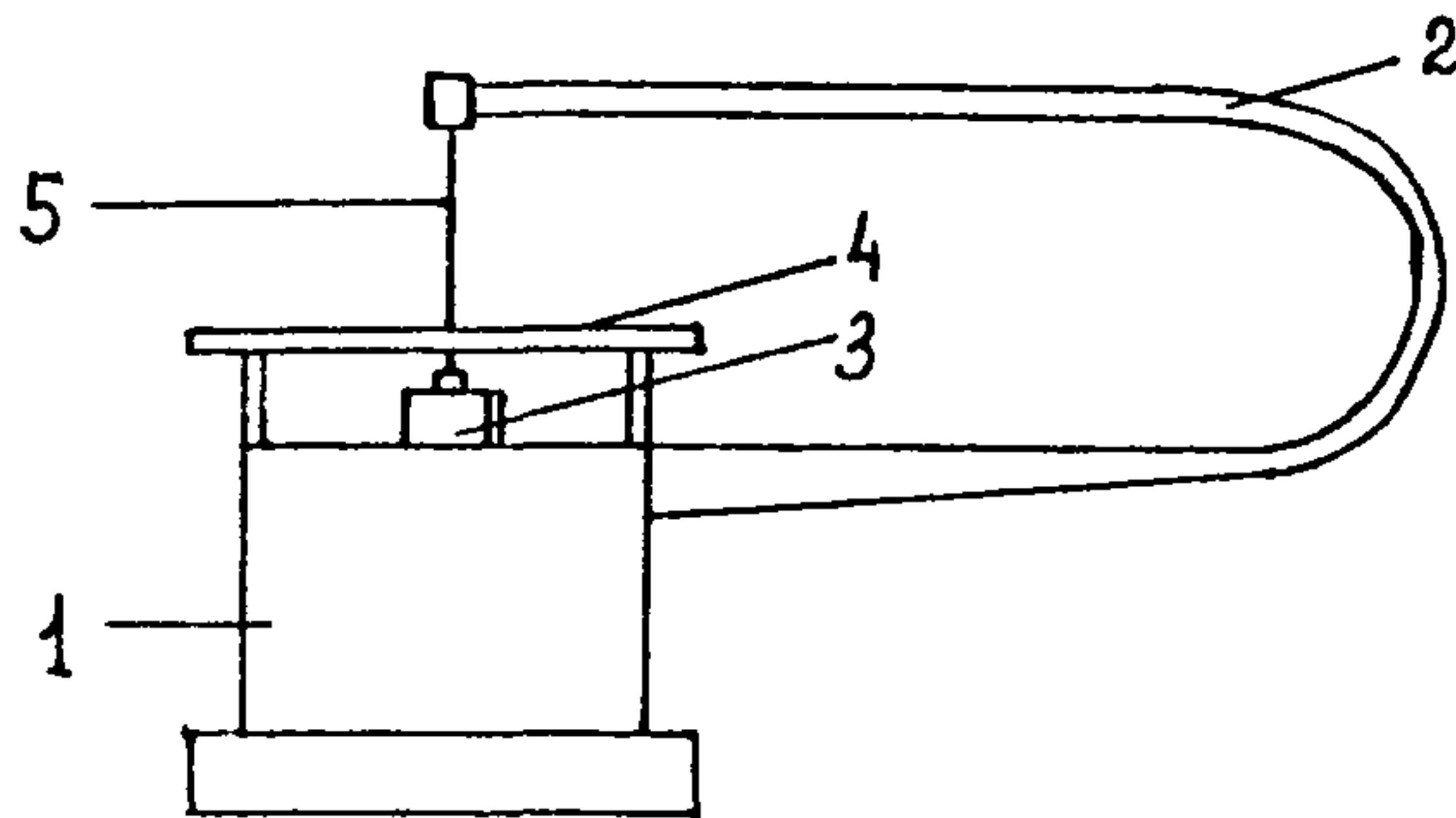
Рис. 3.2 Электромеханический лобзик 1 - корпус; 2 - дуга; 3 - стержень; 4 - крышка; 5 - пила
