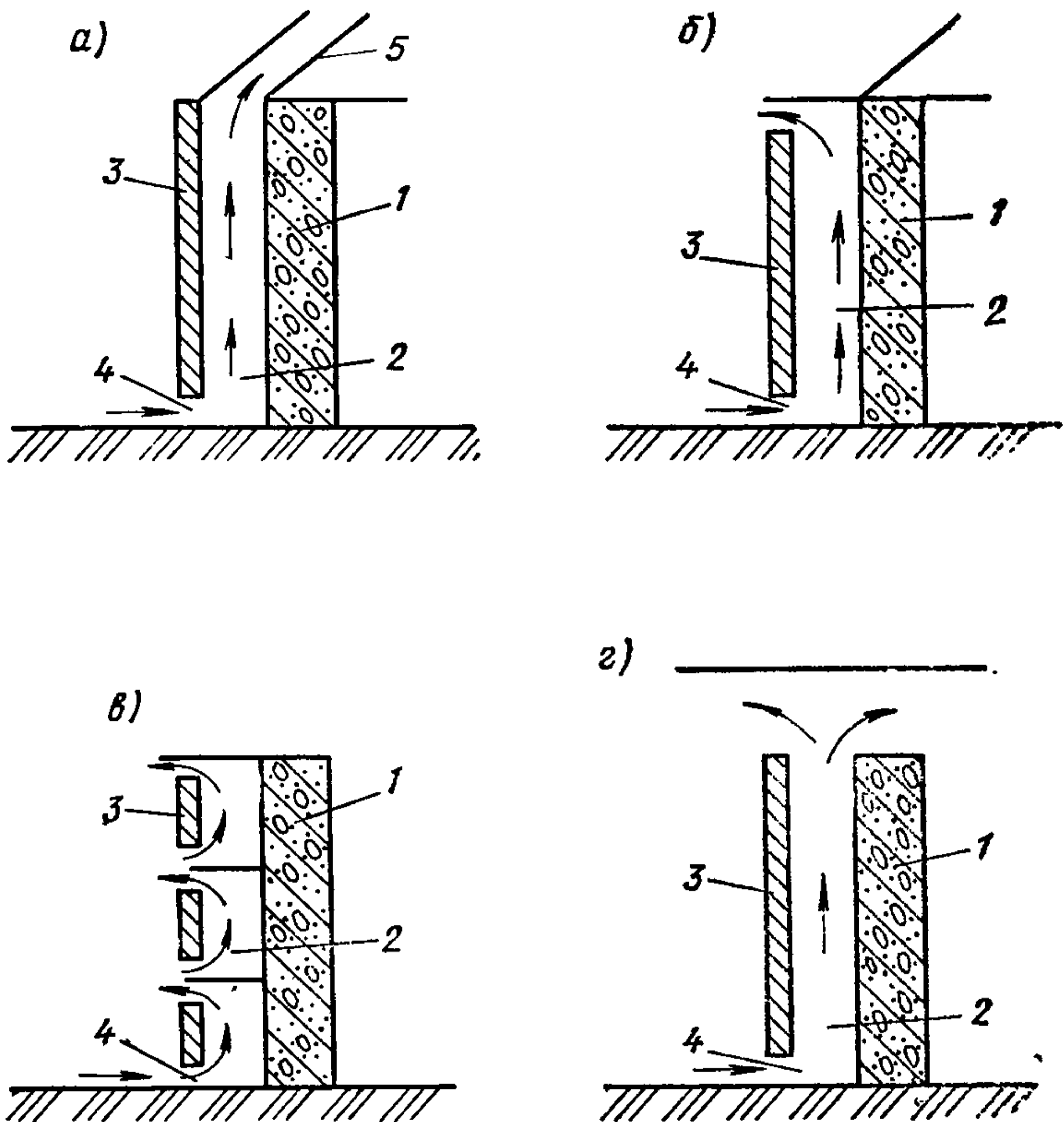
Рис. 8. Аэродинамические схемы вентилируемых стен
