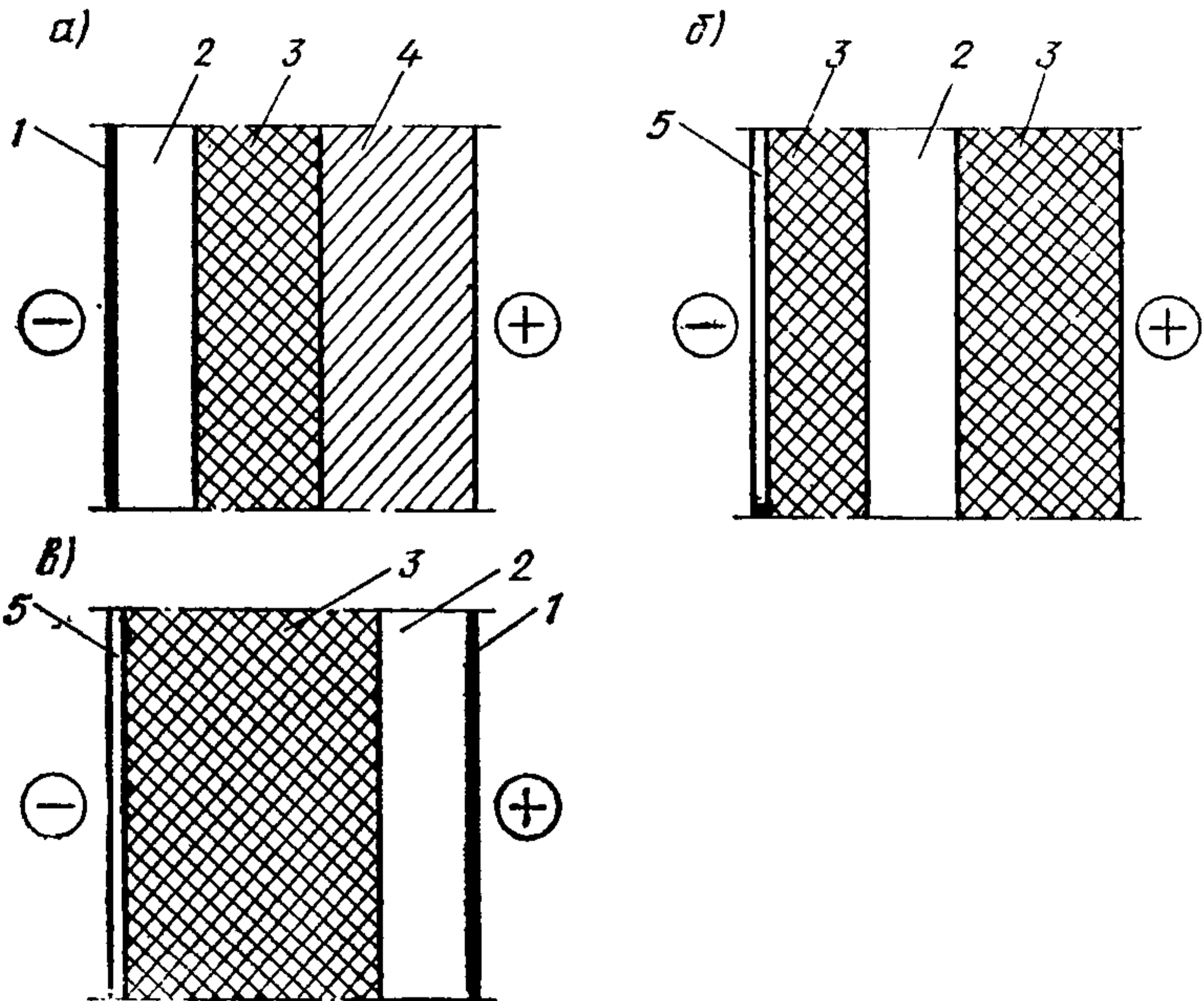
Рис. 1. Схемы стен с различным расположением воздушной прослойки
