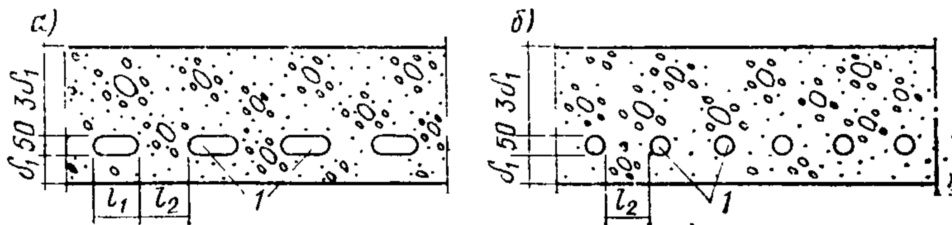
Рис. 10. Схемы расположения каналов в однослойных вентилируемых стенах
