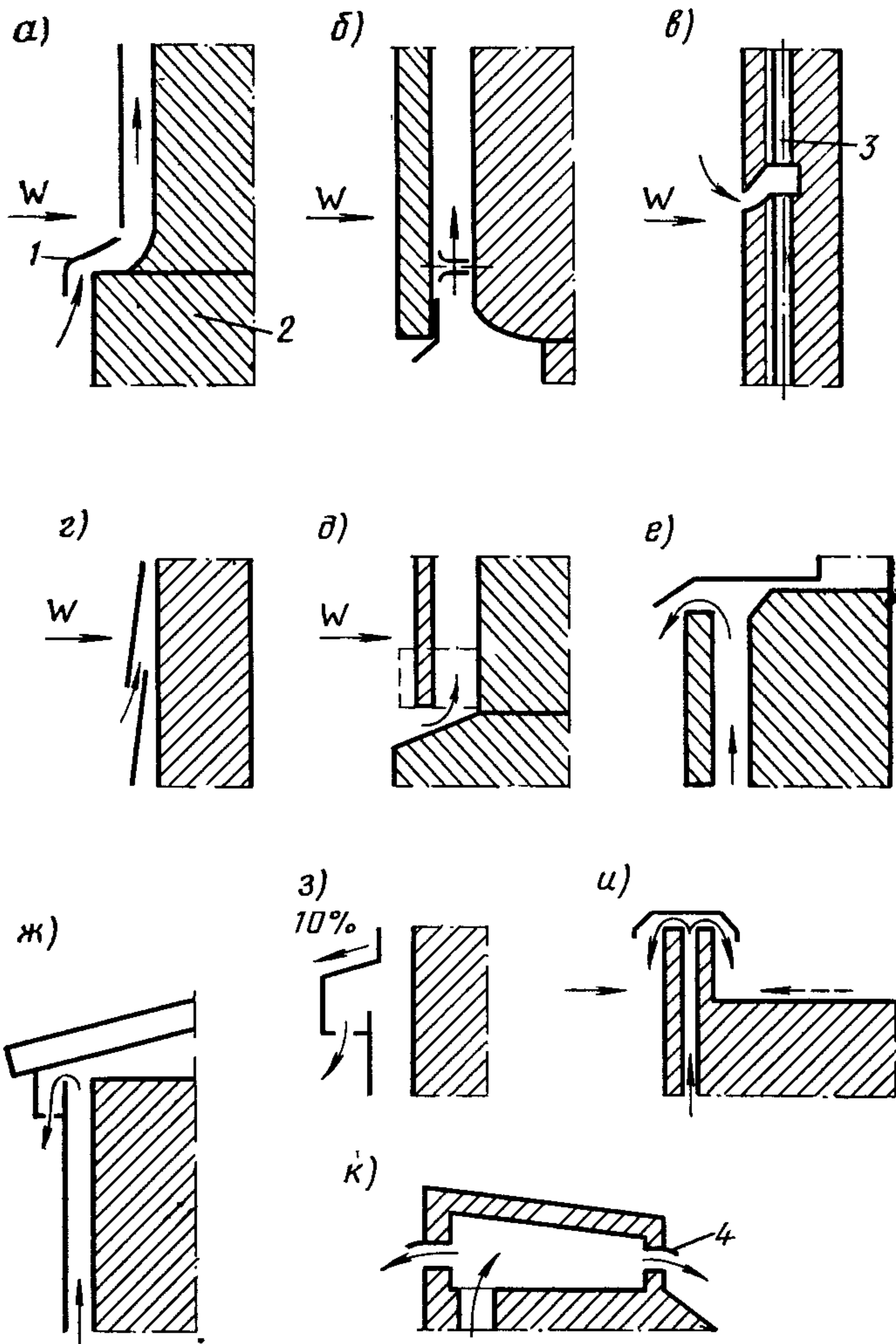
Рис. 3. Вентиляционные отверстия входа и выхода воздуха a—d — отверстия входа воздуха; a, d — у цоколя; b — над оконным проемом; в —к каналу в массиве стены; г —при чешуйчатом экране; е—к —отверстия выхода воздуха; е —под оконным проемом; ж—к —для вариантов кровель; 1 —слив; 2 —цоколь; 3 —канал в массиве стены;
