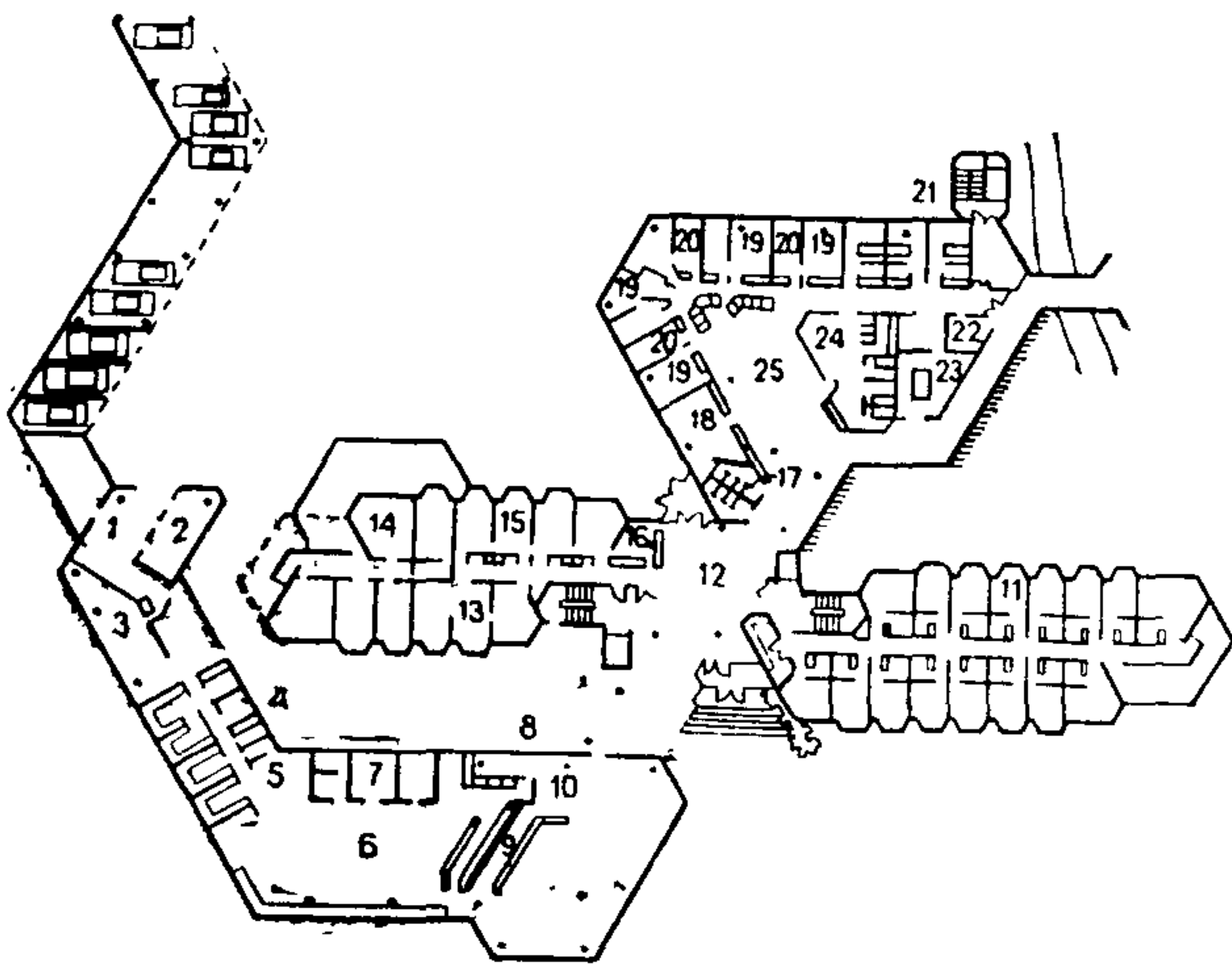
Рис. 1.11. Санаторий на 200 мест ревматологического профиля в Зеккингене, ФРГ. План первого этажа
