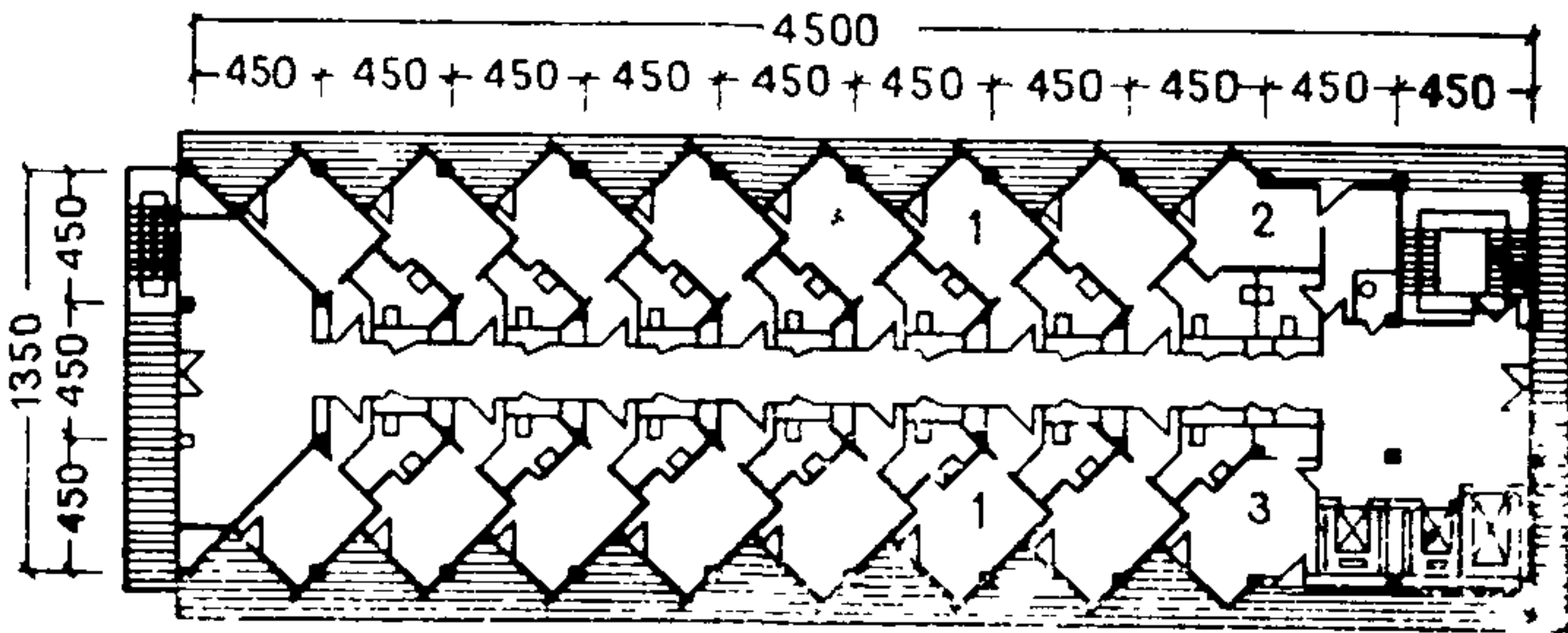
Рис. 3.13. Санаторий «Сухуми» на 340 мест. Авторы: С. Цинцабадзе, Я. Кахиани, Ш. Блуашвили. План типового этажа
