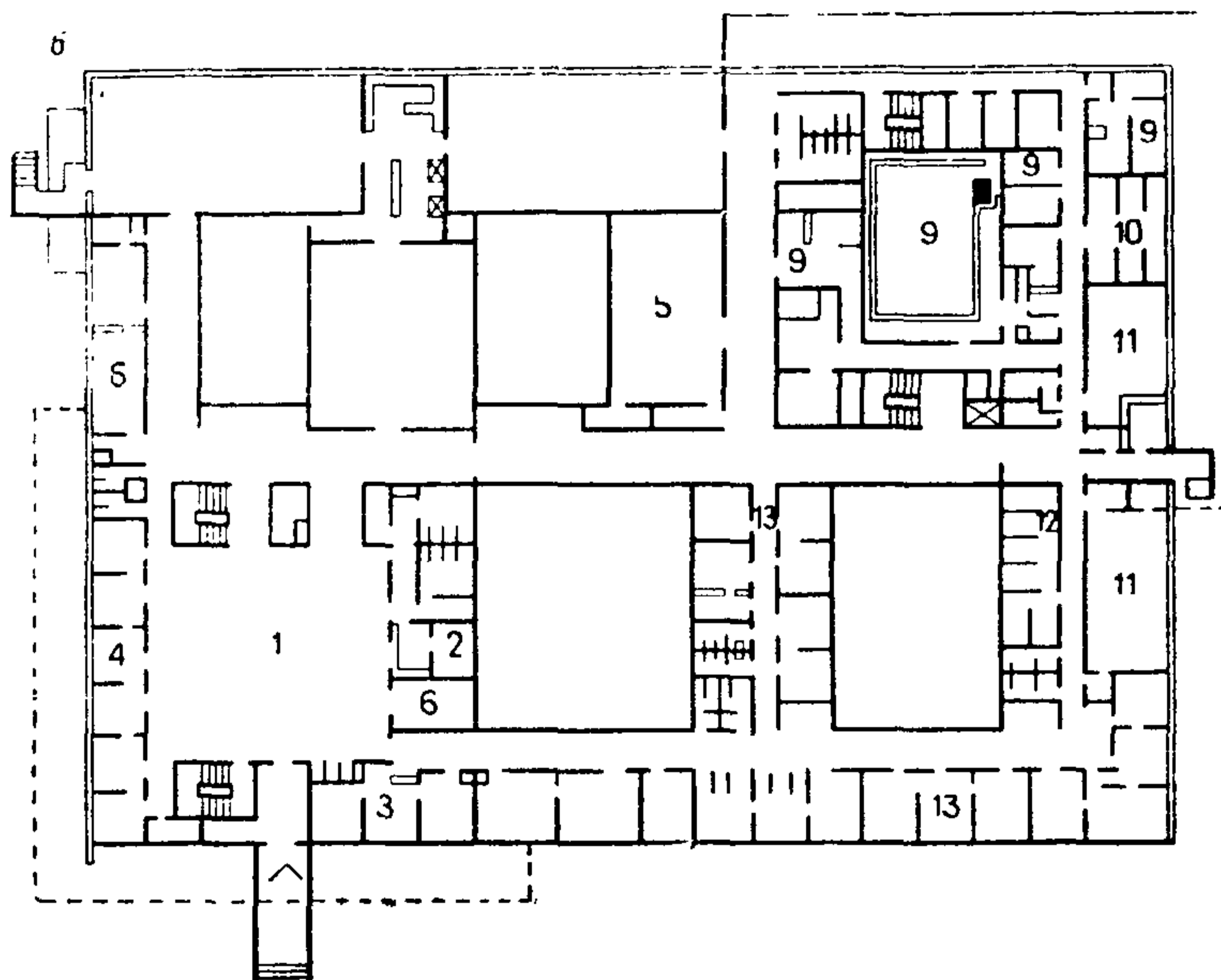
Рис. 1.10. Санаторий «Беттерау», ФРГ
