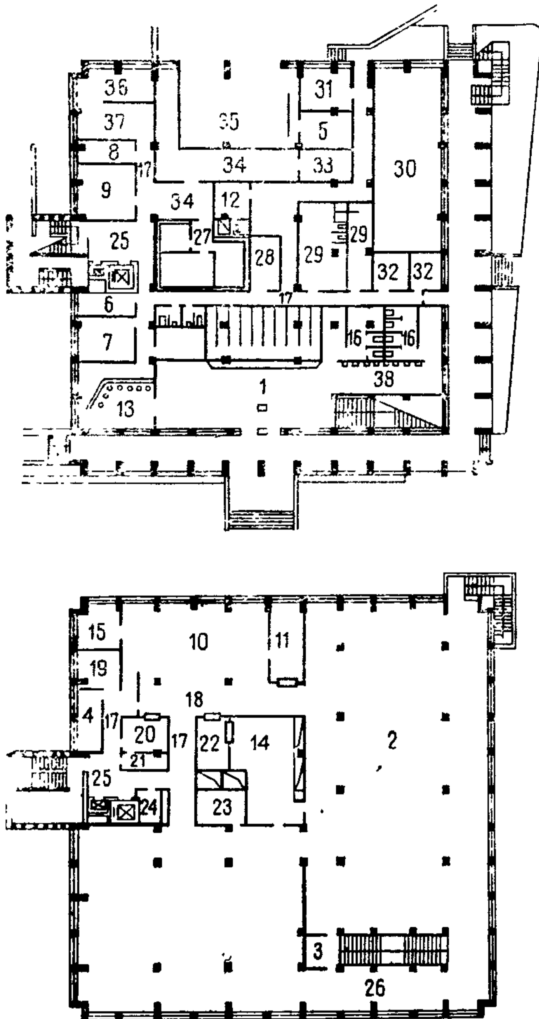
Рис. 6.3. Пример объемно - планировочного решения столовой на 500 мест
