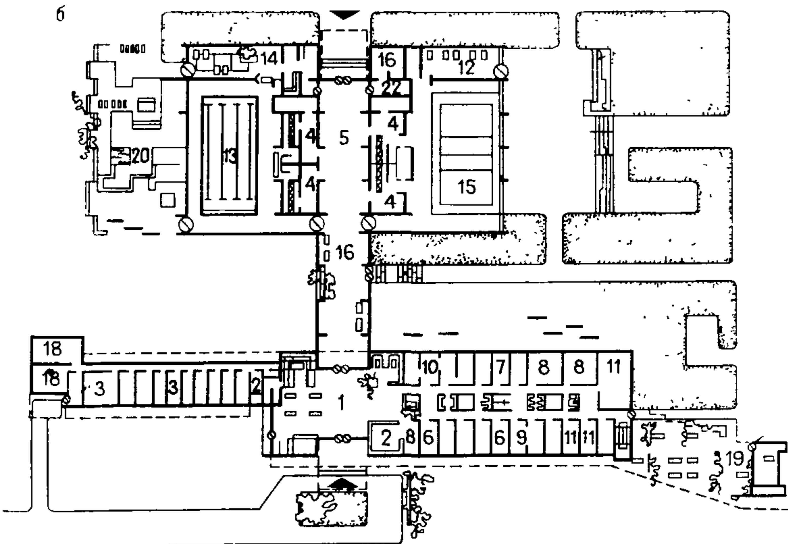
Рис. 1.15. Санаторий на 300 мест в Мошней. Польша
