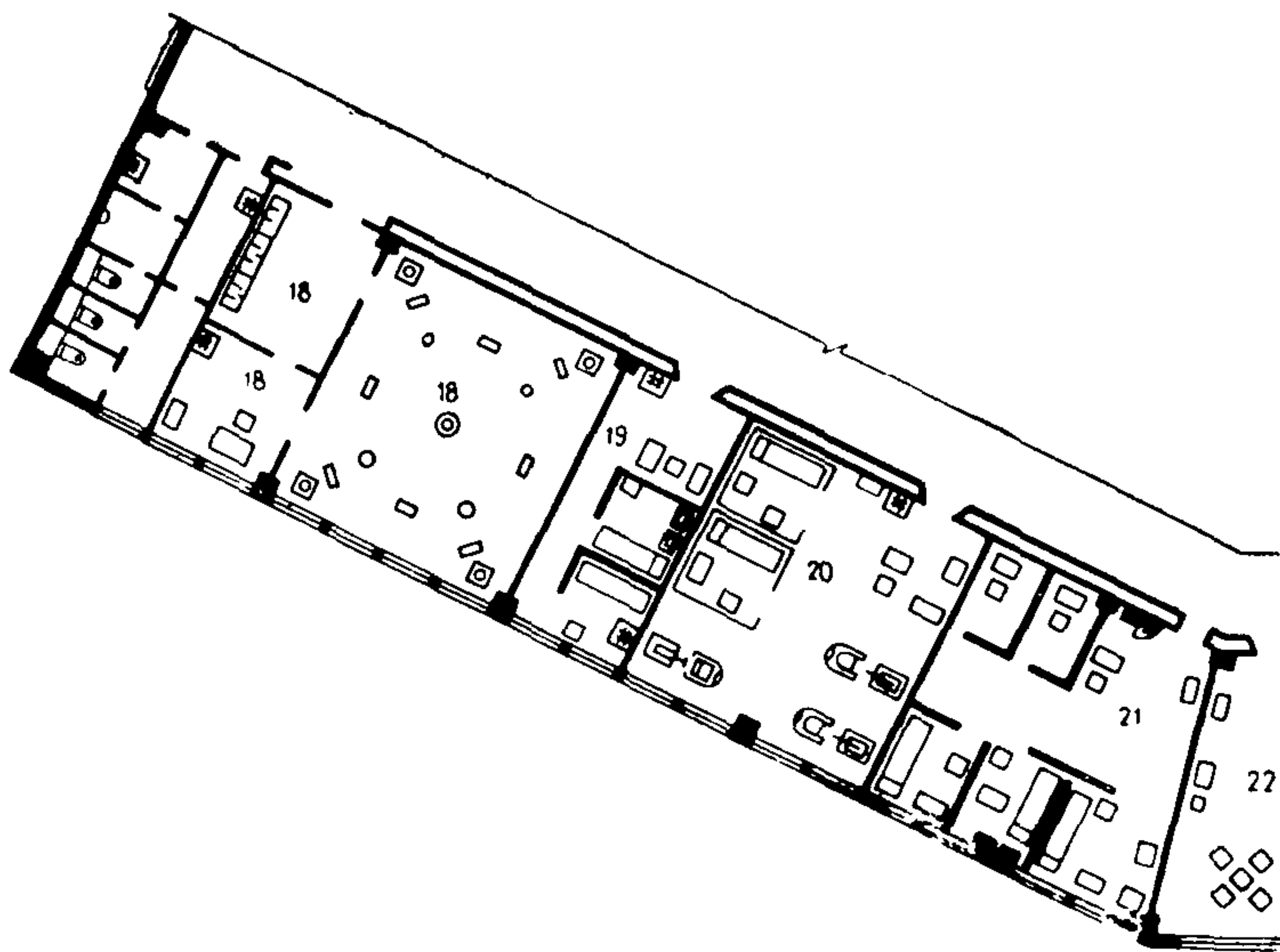
Рис. 4.4. Санаторий «Ленинские скалы» на 1000 мест в Пятигорске.
