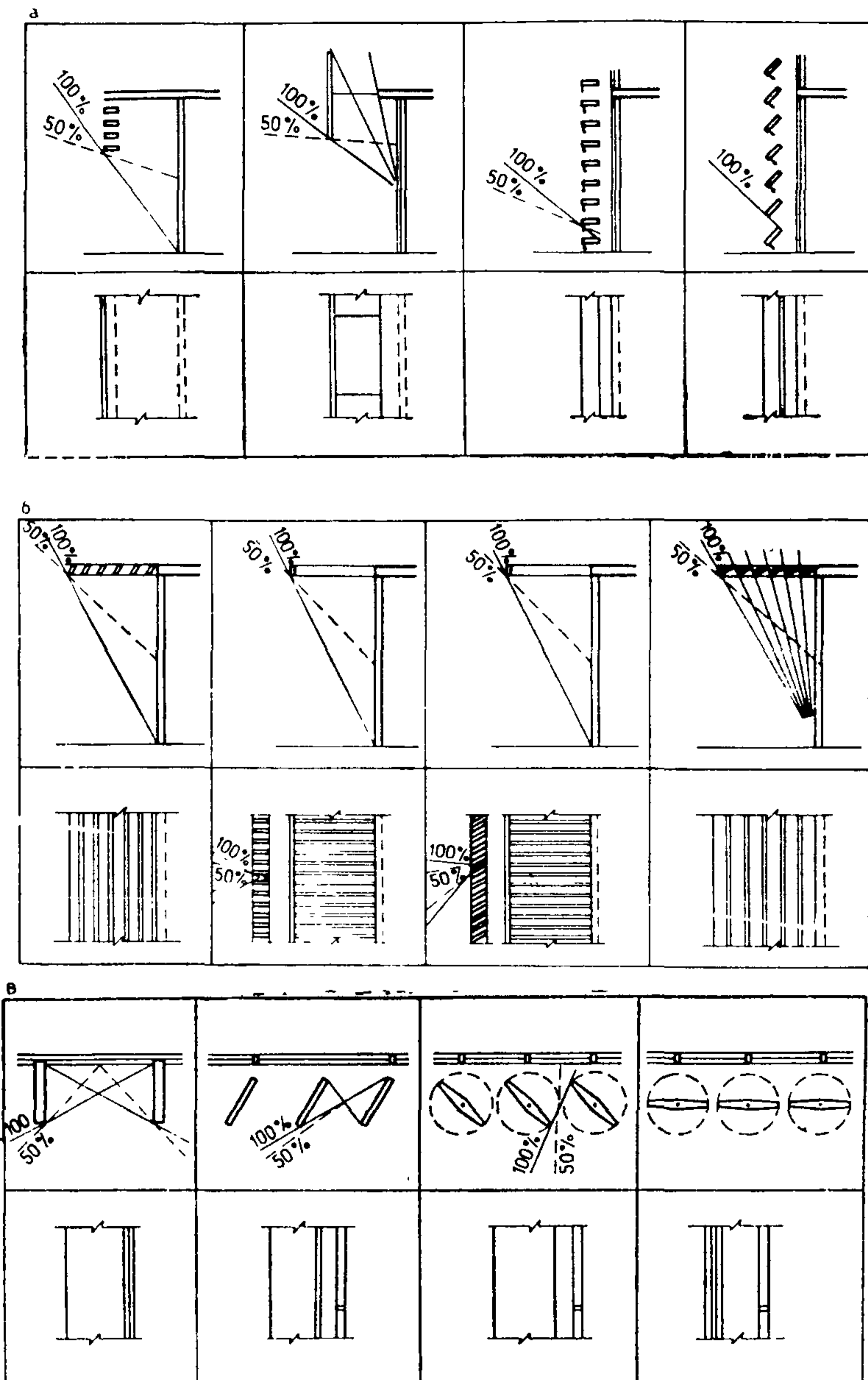
Рис. 3.11. Солнцезащитные устройства а, б—горизонтальные; в—вертикальные
