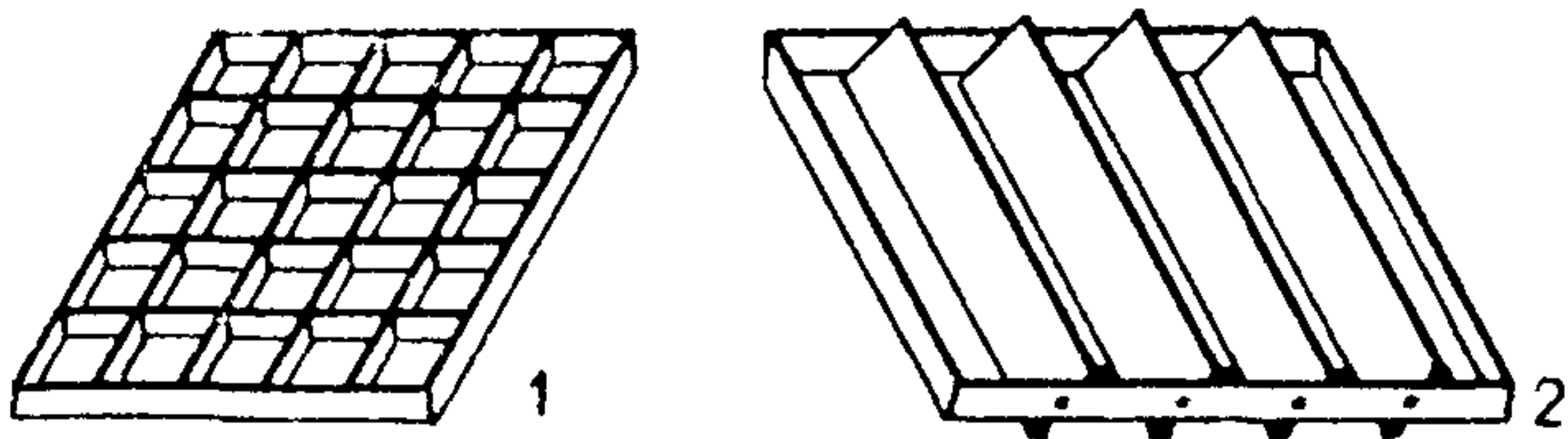
Рис. 5.1. Конструкции перекрытий
