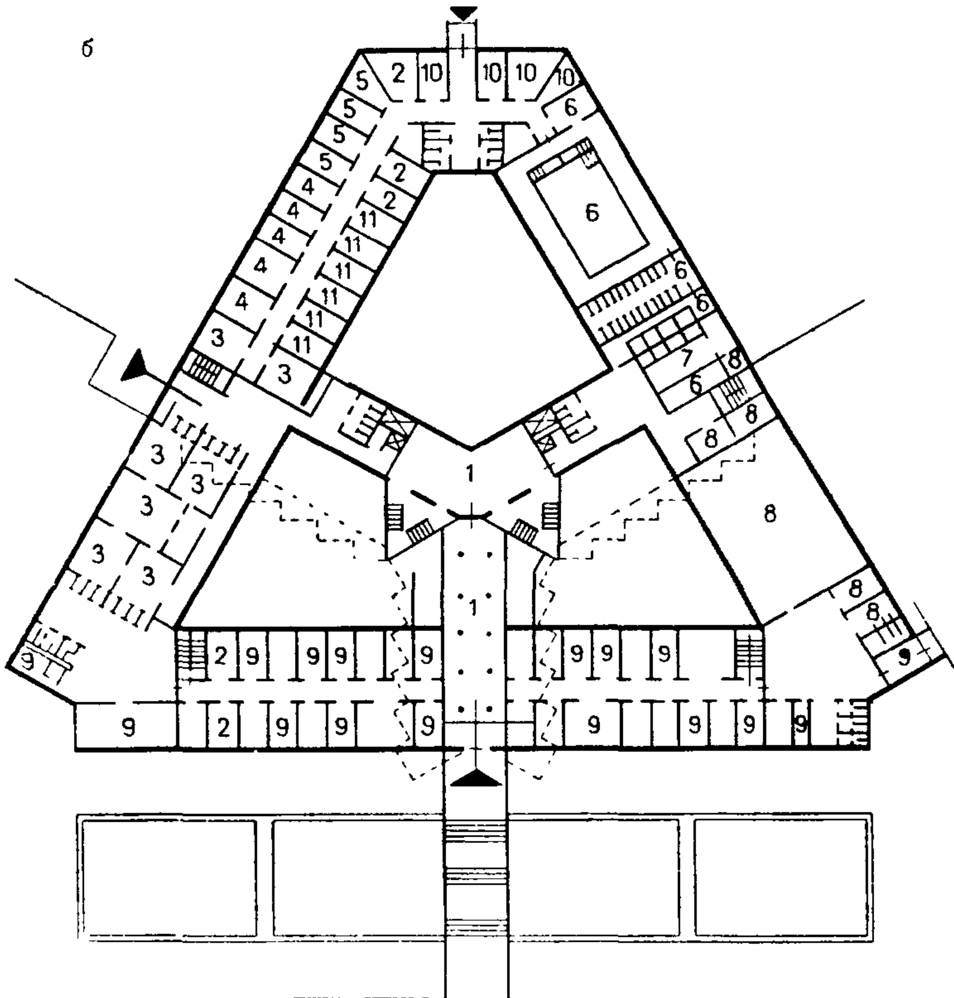
Рис. 1.9. Санаторий «Родербиркен» на 252 места в Ляйхлинае, Австрия
