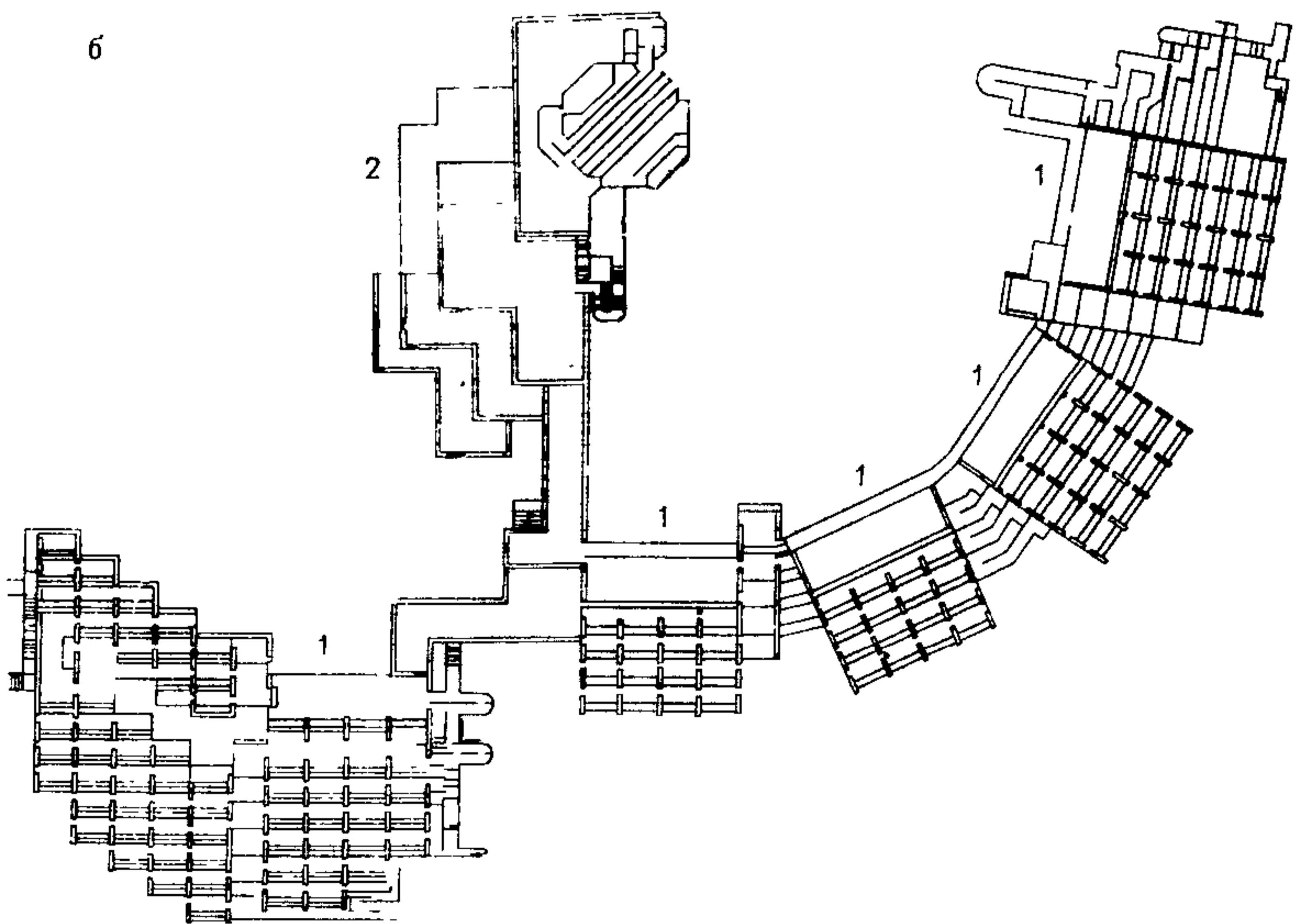
Рис. 3.5. Санаторий на 500 мест. Авторы: А. Пшеничный, Е. Руд- минский, В. Тимохин (КиевНИИПград) а—общий вид; б—схема плана; 1—спальный блок; 2—общественный блок
