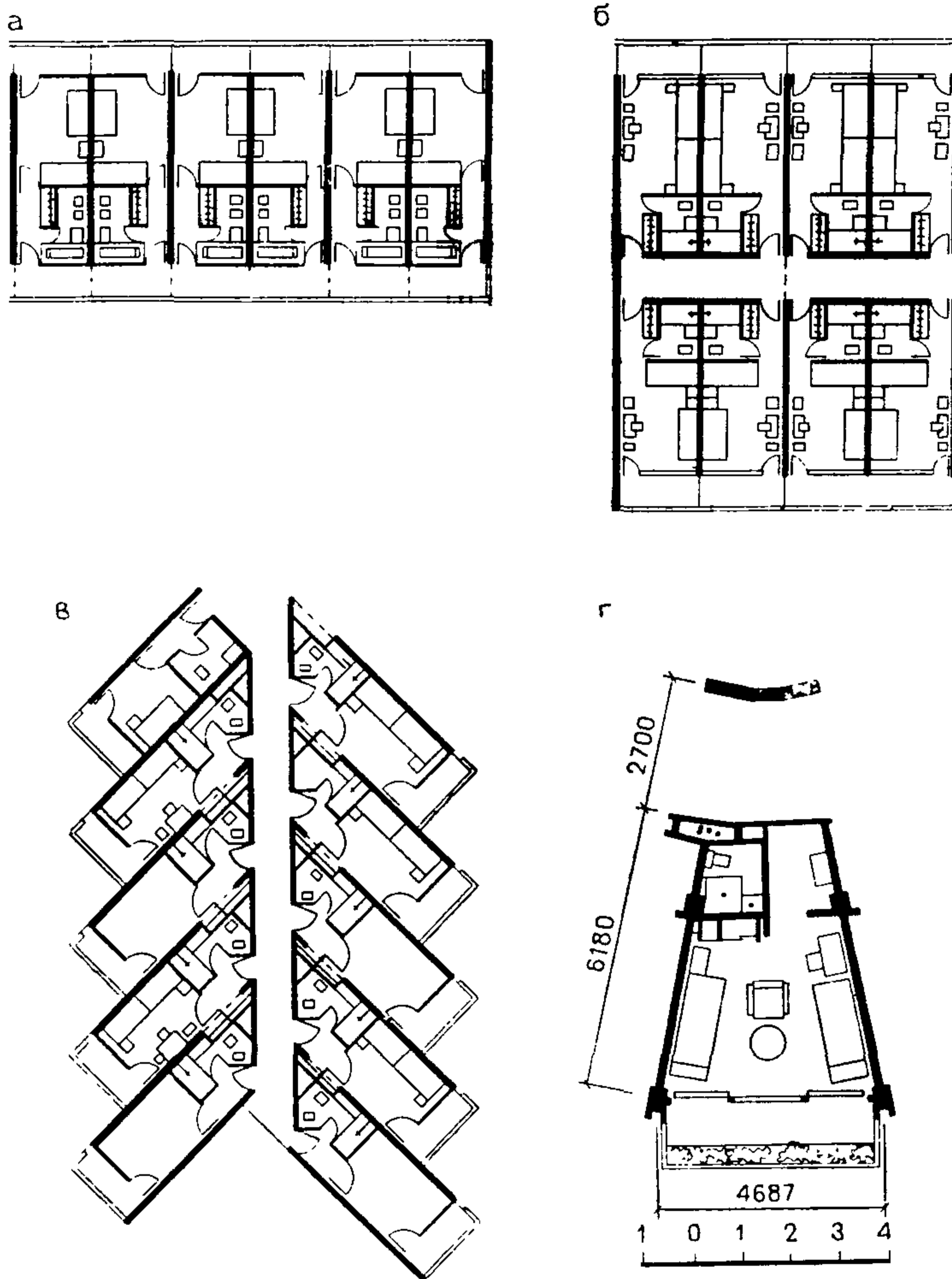
Рис. 3.17. Типы жилых ячеек
