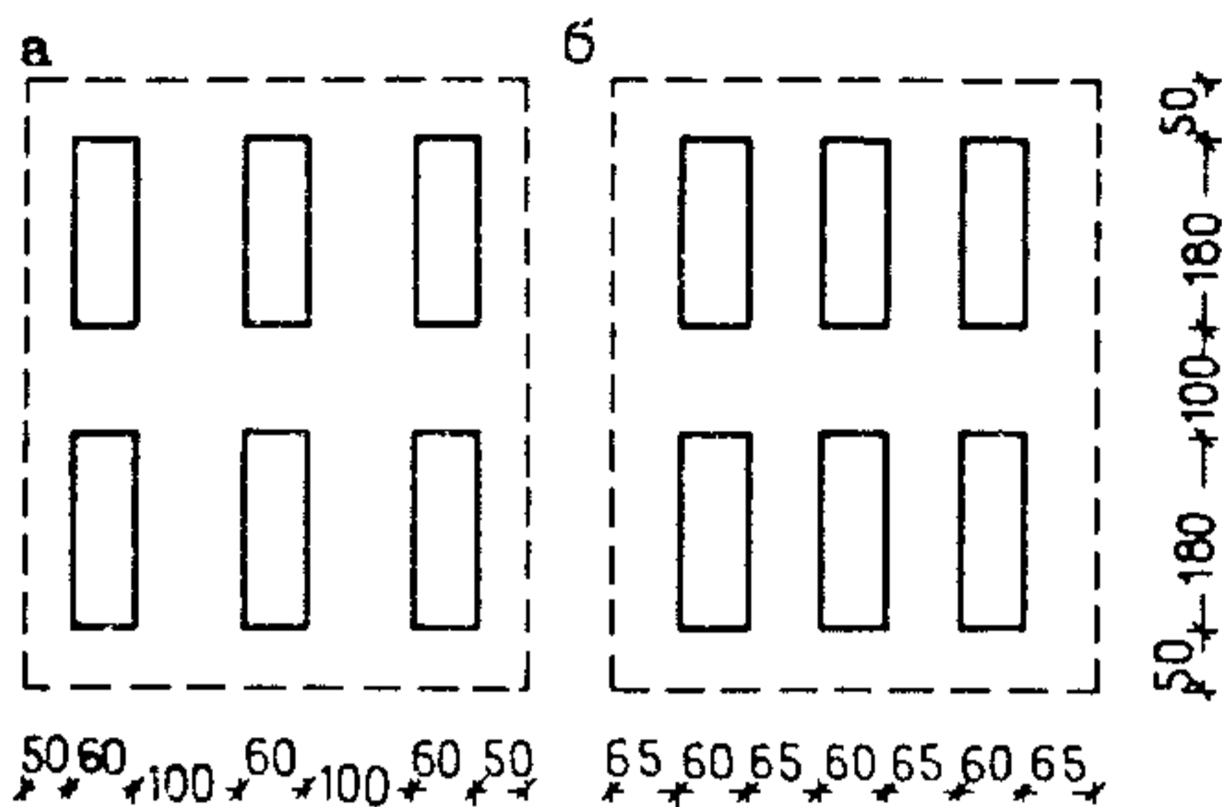
Рис. 5.3. Схема расстановки лежаков
