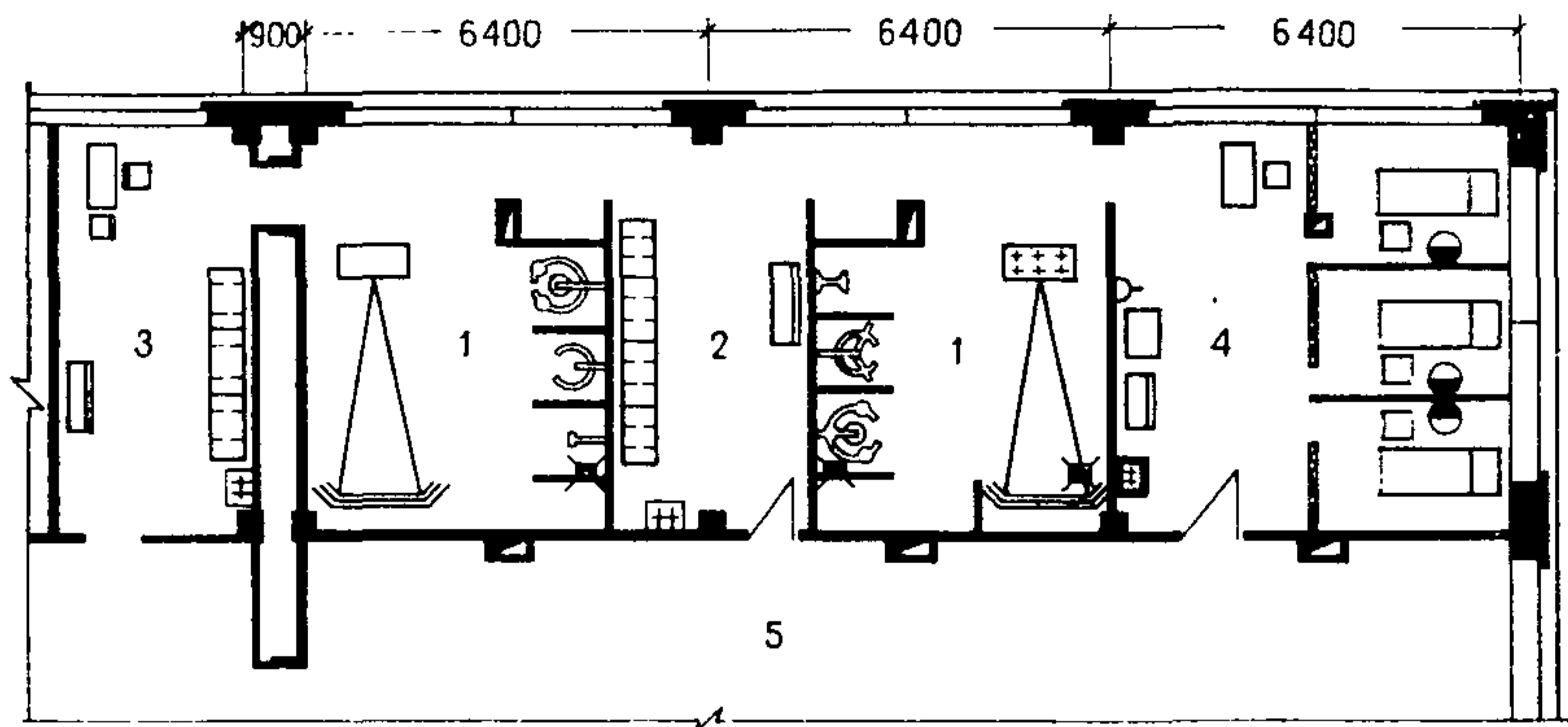
Рис. 4.9. Фрагмент душевого зала санатория «Ленинские скалы»
