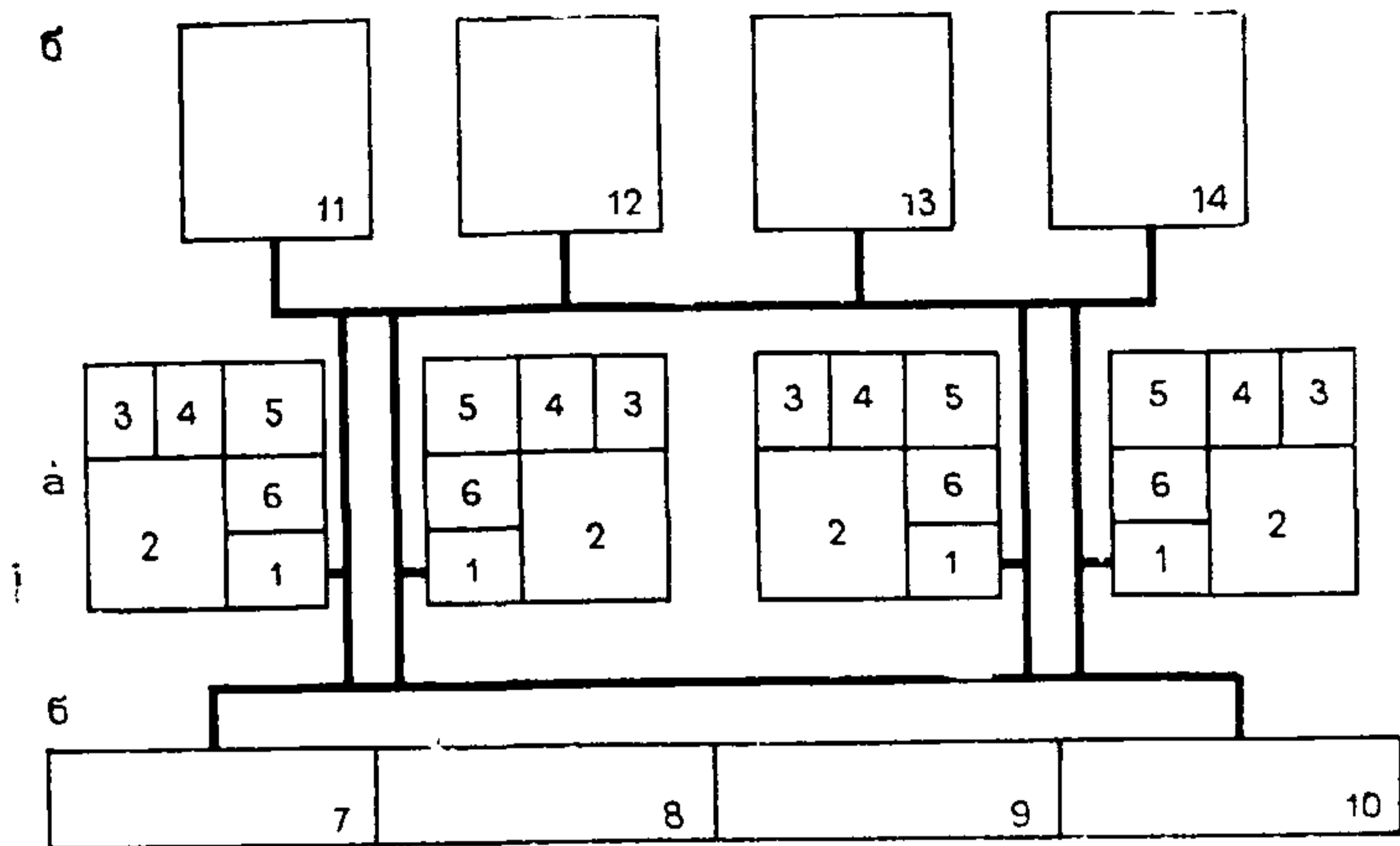
Рис. 1.1. Функциональная схема планировочной организации санаторного комплекса
