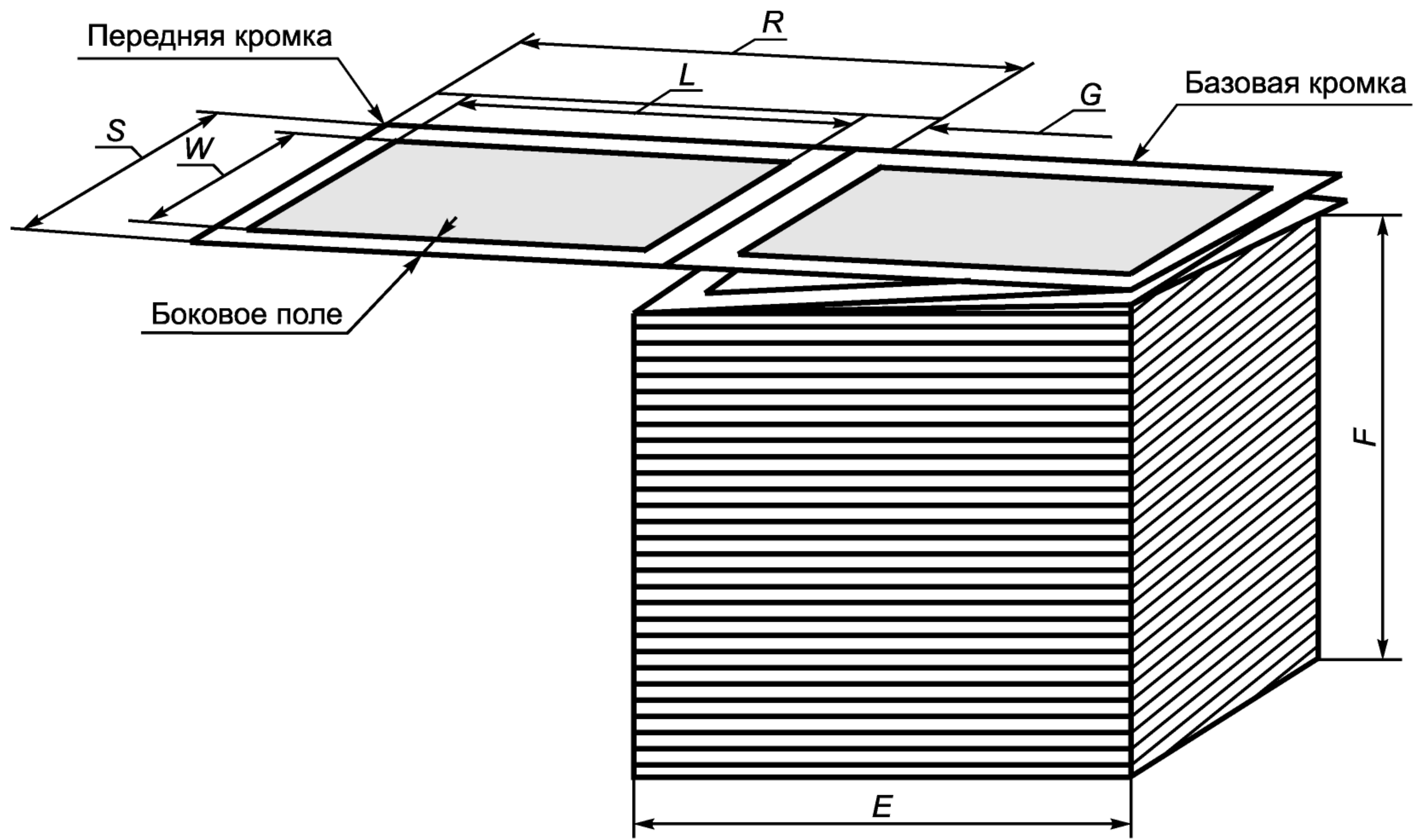
Рисунок А.2 — Размеры пачки фальцованных этикеток
