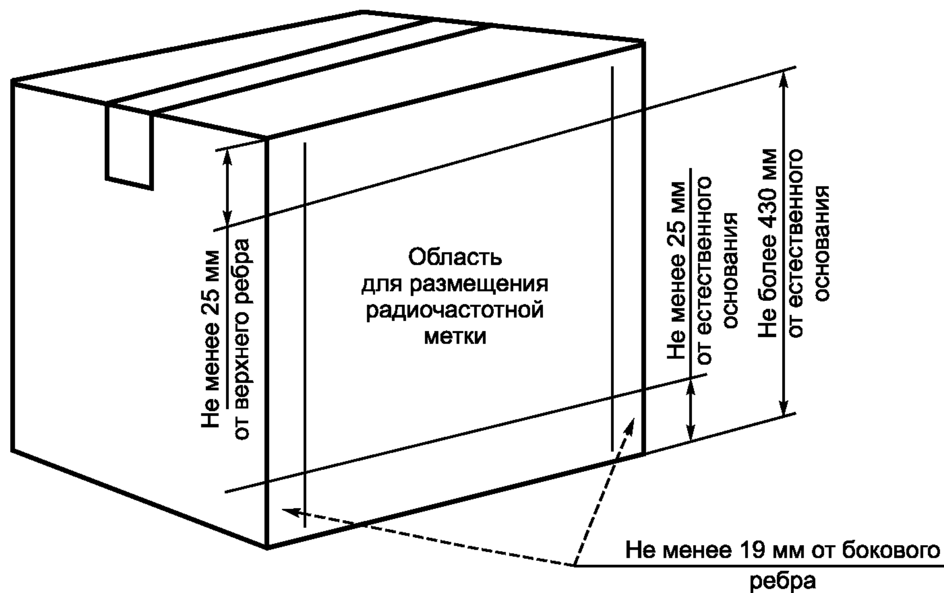
Рисунок 5 — Рекомендуемое размещение радиочастотной метки на транспортируемой единице
