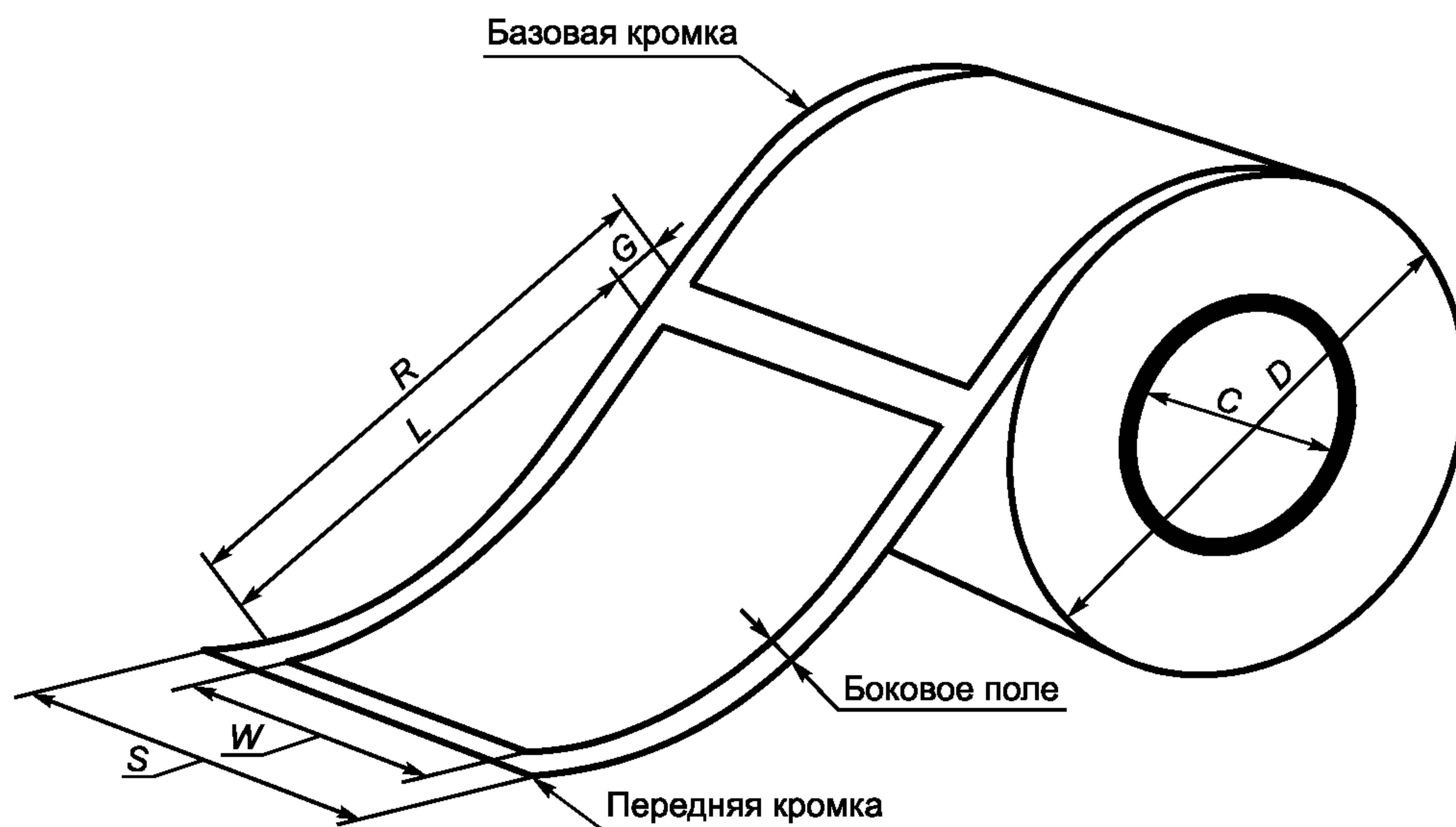
Рисунок А.1 — Размеры этикеток в рулоне
