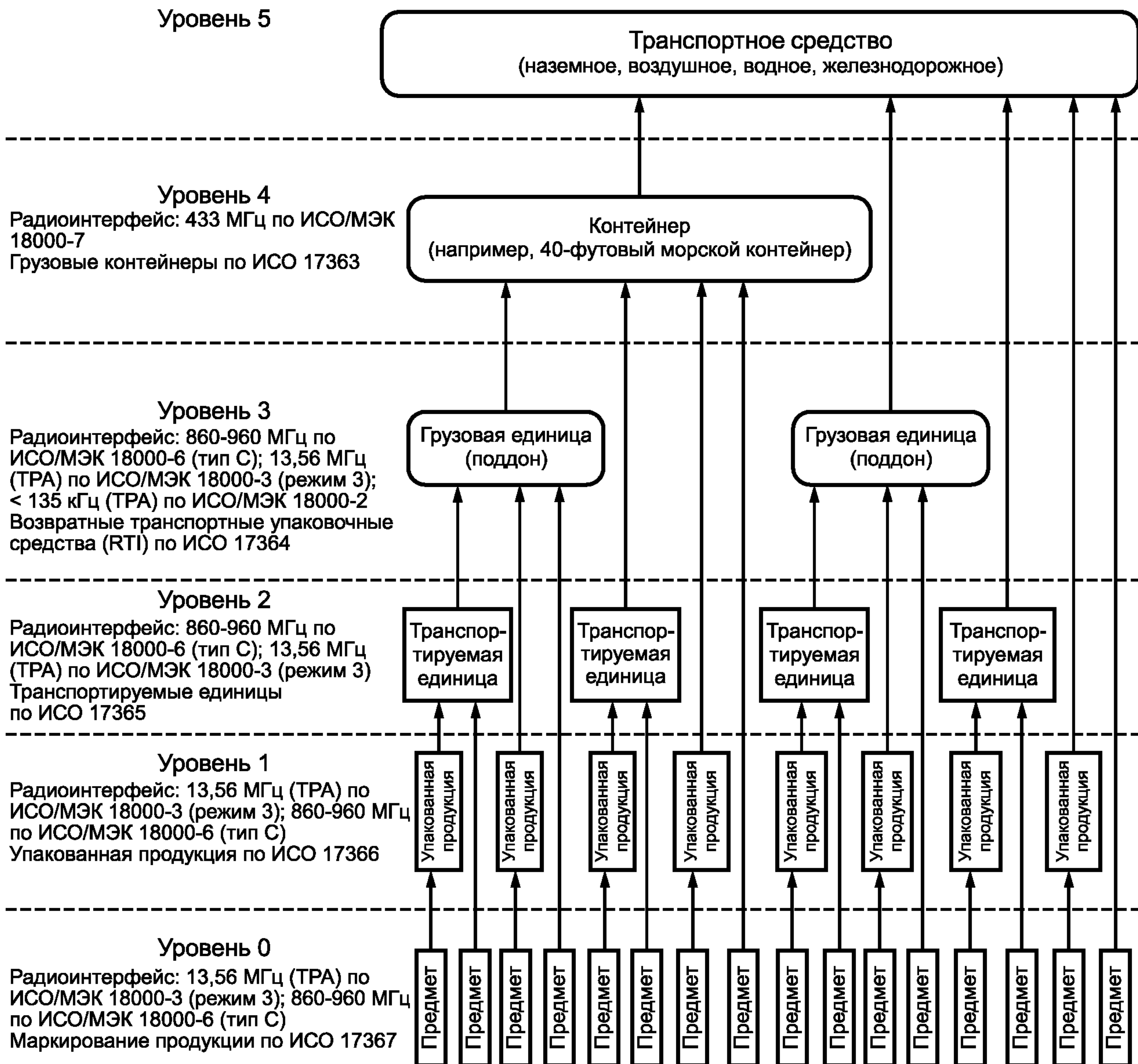
Рисунок 1 — Уровни цепи поставки при использовании радиочастотной идентификации
