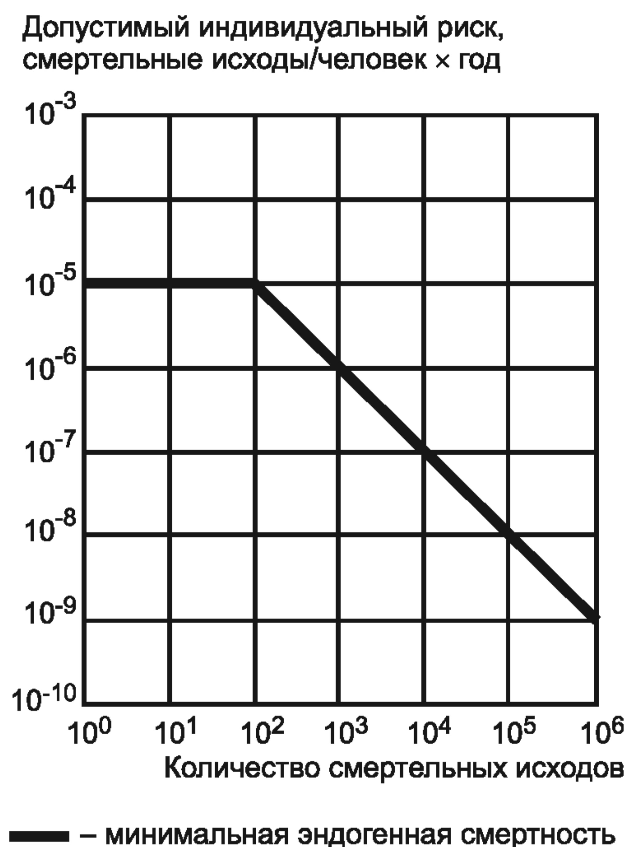
Рисунок Г.3 — Кривая минимальной эндогенной смертности
