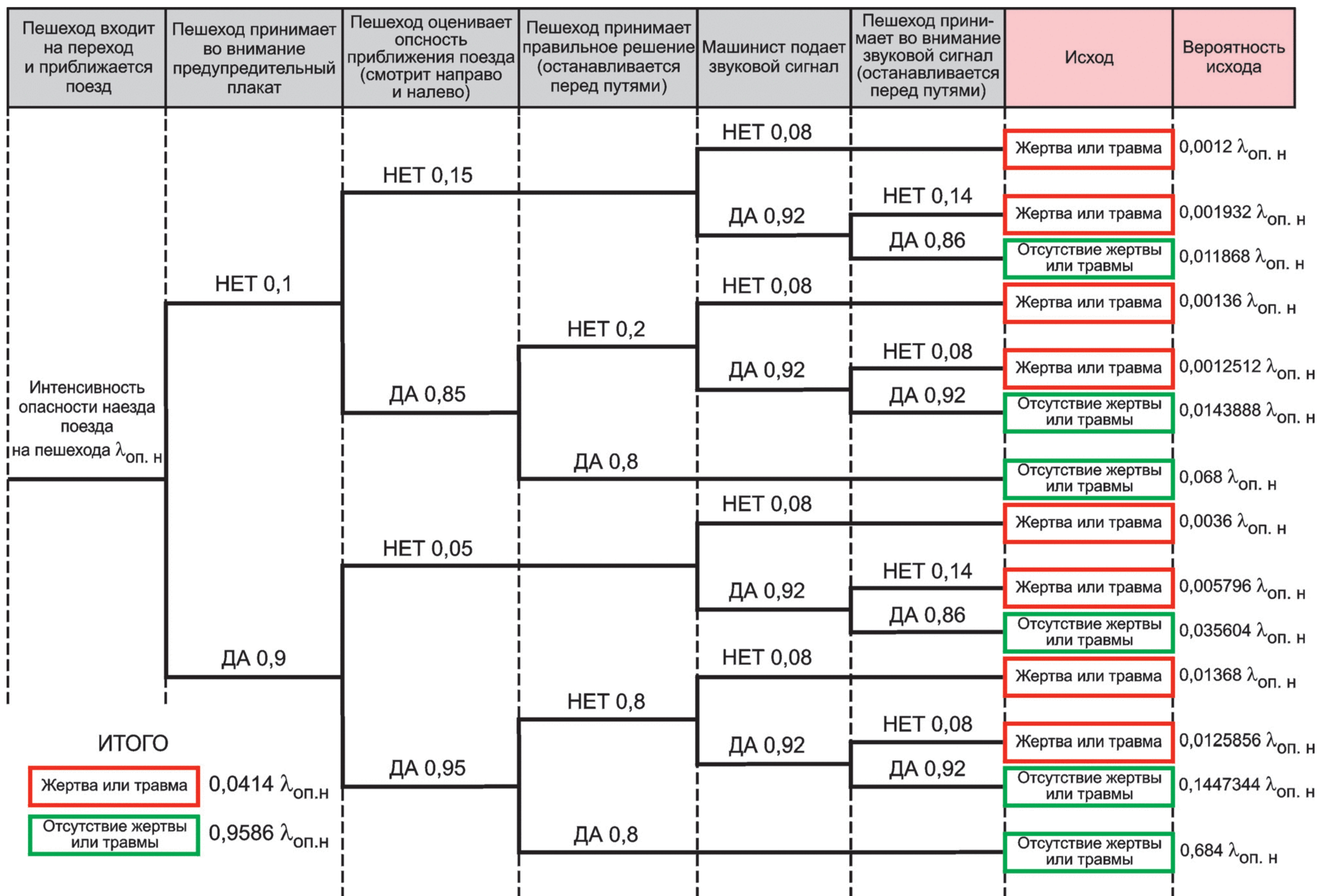
Рисунок А.3 — Пример дерева событий для оценки риска травматизма пешеходов на пешеходном переходе третьей категории
