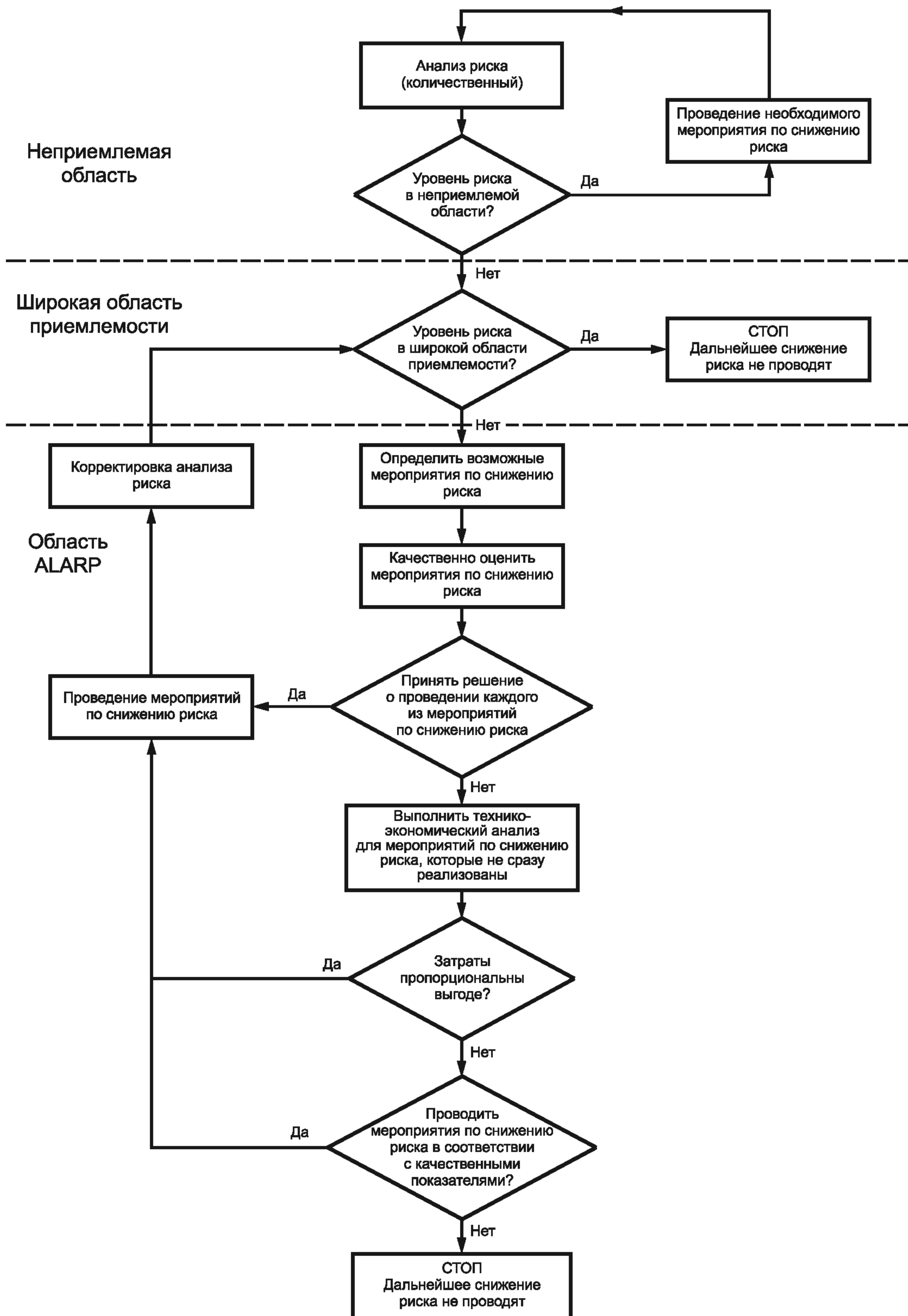
Рисунок Г.2 — Демонстрация использования принципа ALARP
