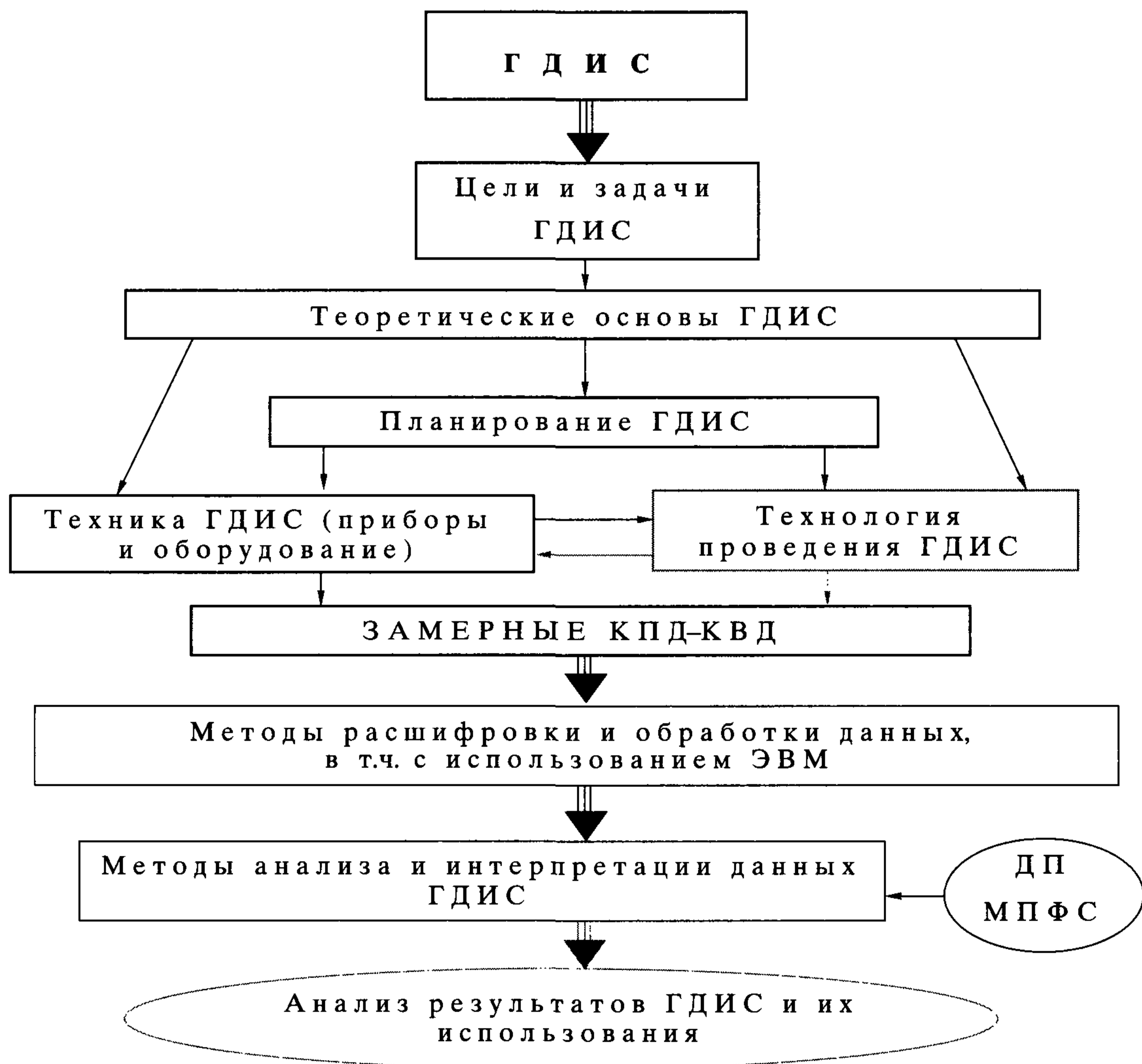
Рисунок А3. Структура системы ГДИС.
