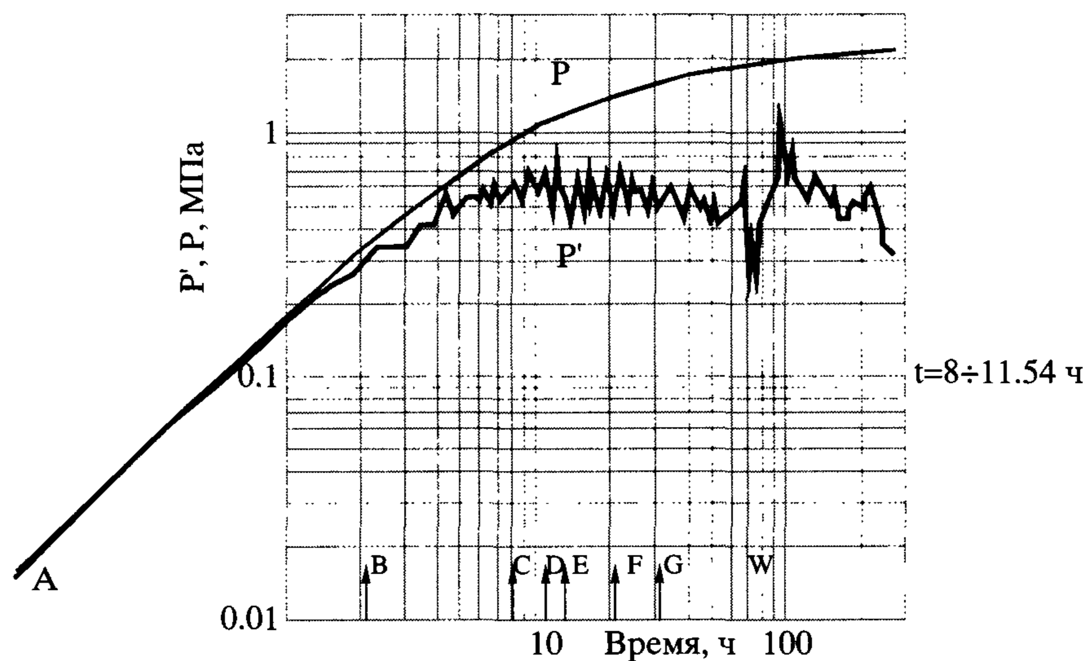
Рисунок А9. Диагностический бигарифмический график ГДИС горизонтальной скв. 11412 КВД-1. Буквы – диагностические участки.
