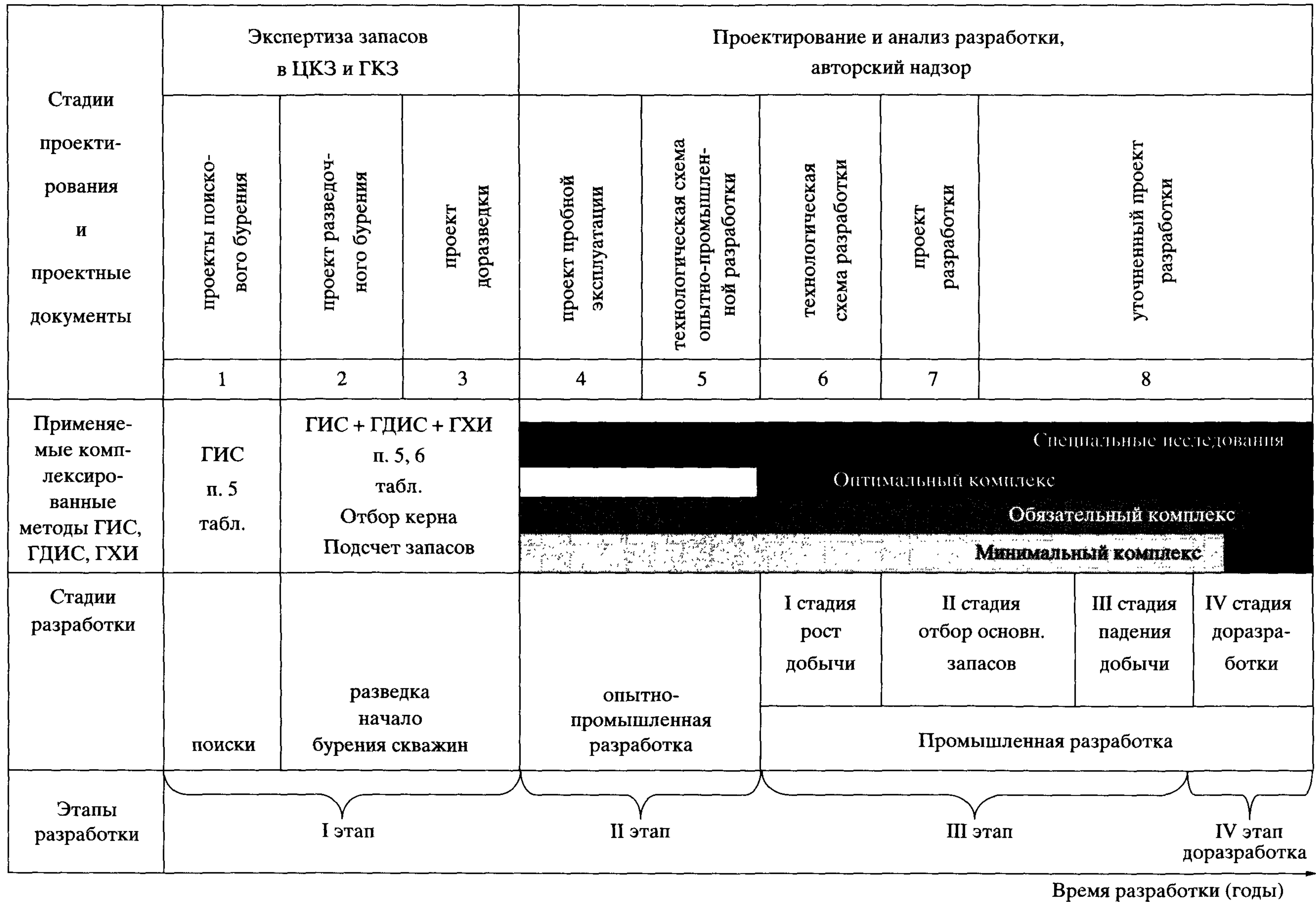
Рисунок 4. Схематическое соотношение различных этапов разработки, стадий проектирования и применения комплексированных методов исследования скважин и пластов.
