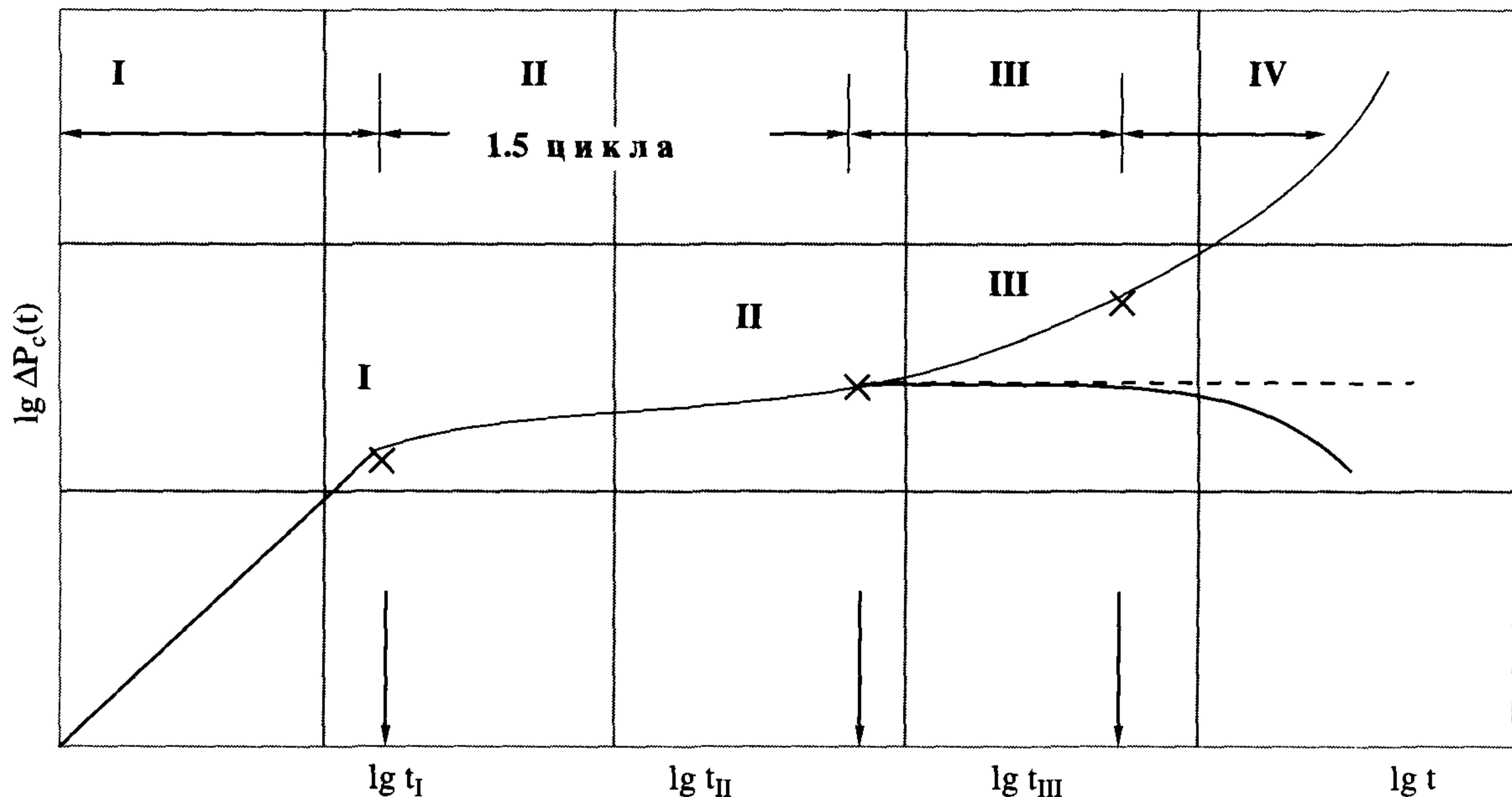
Рисунок А6. Билогарифмический диагностический график КВД-КВД идентификации режимов течения, типов фильтрационных потоков.
