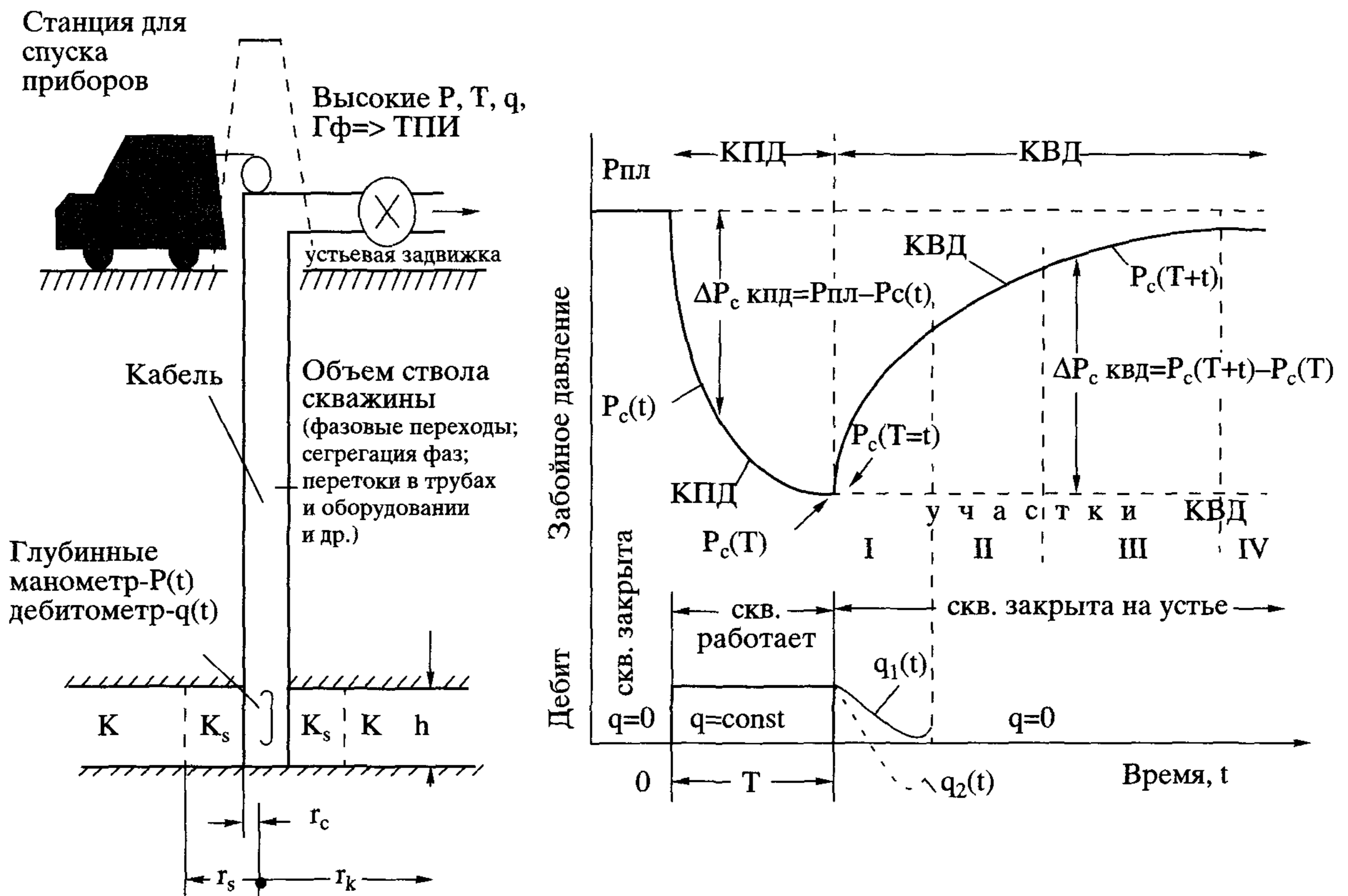
Рисунок А2. Схема снятия КПД-КВД.
