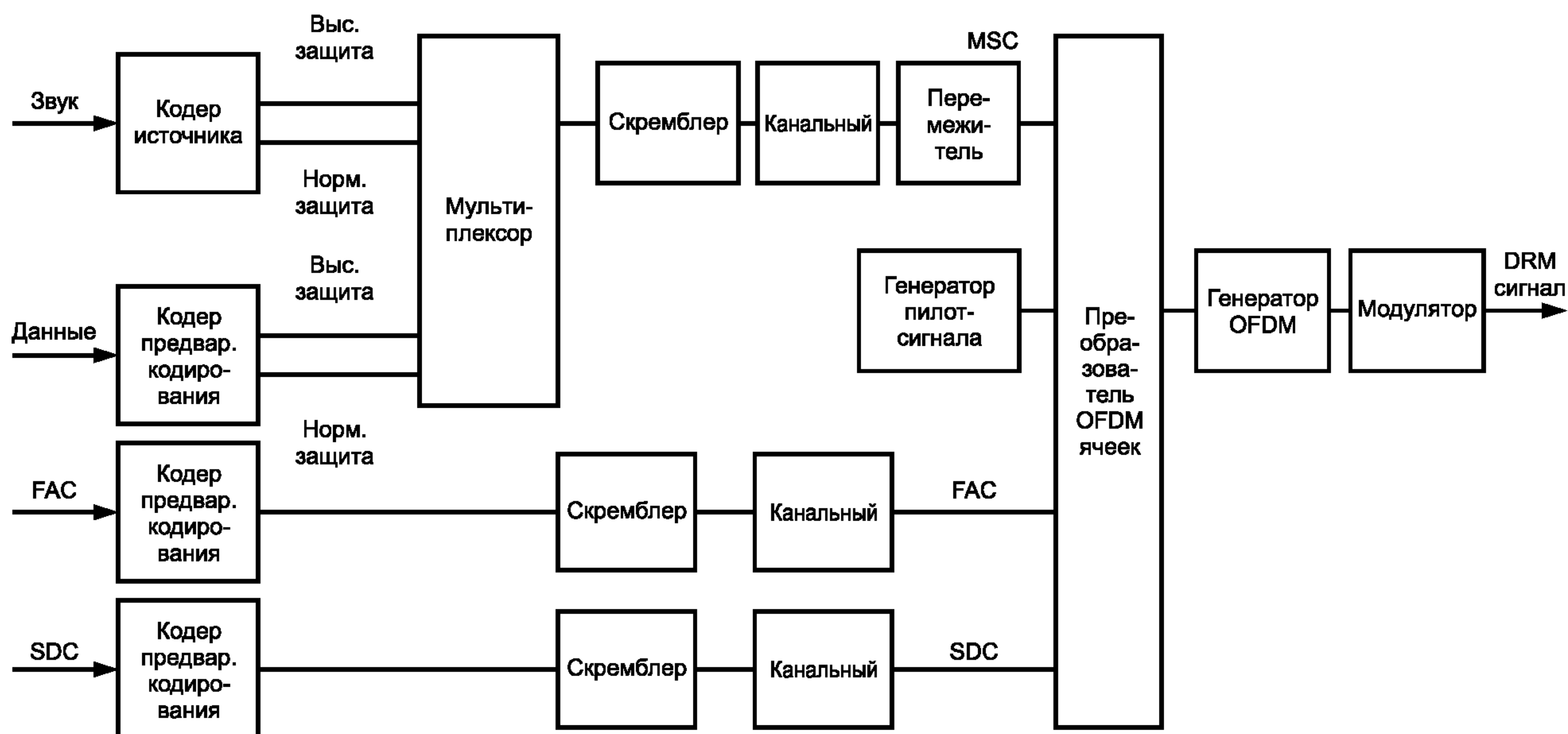
Рисунок 1 — Структурная схема передающей части системы DRM
