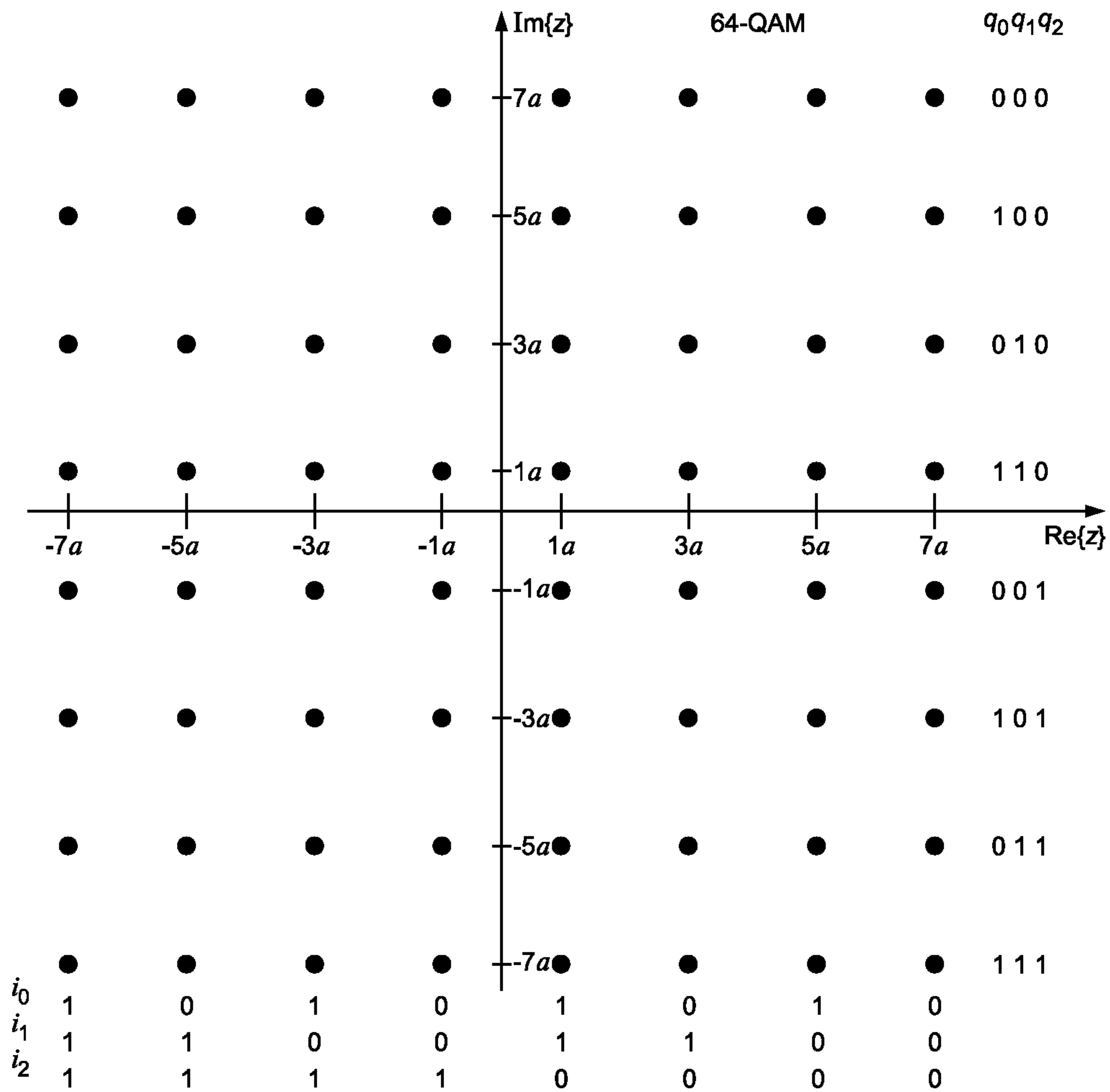
Рисунок 4 — SM 64-QAM отображение с соответствующей битовой комбинацией
