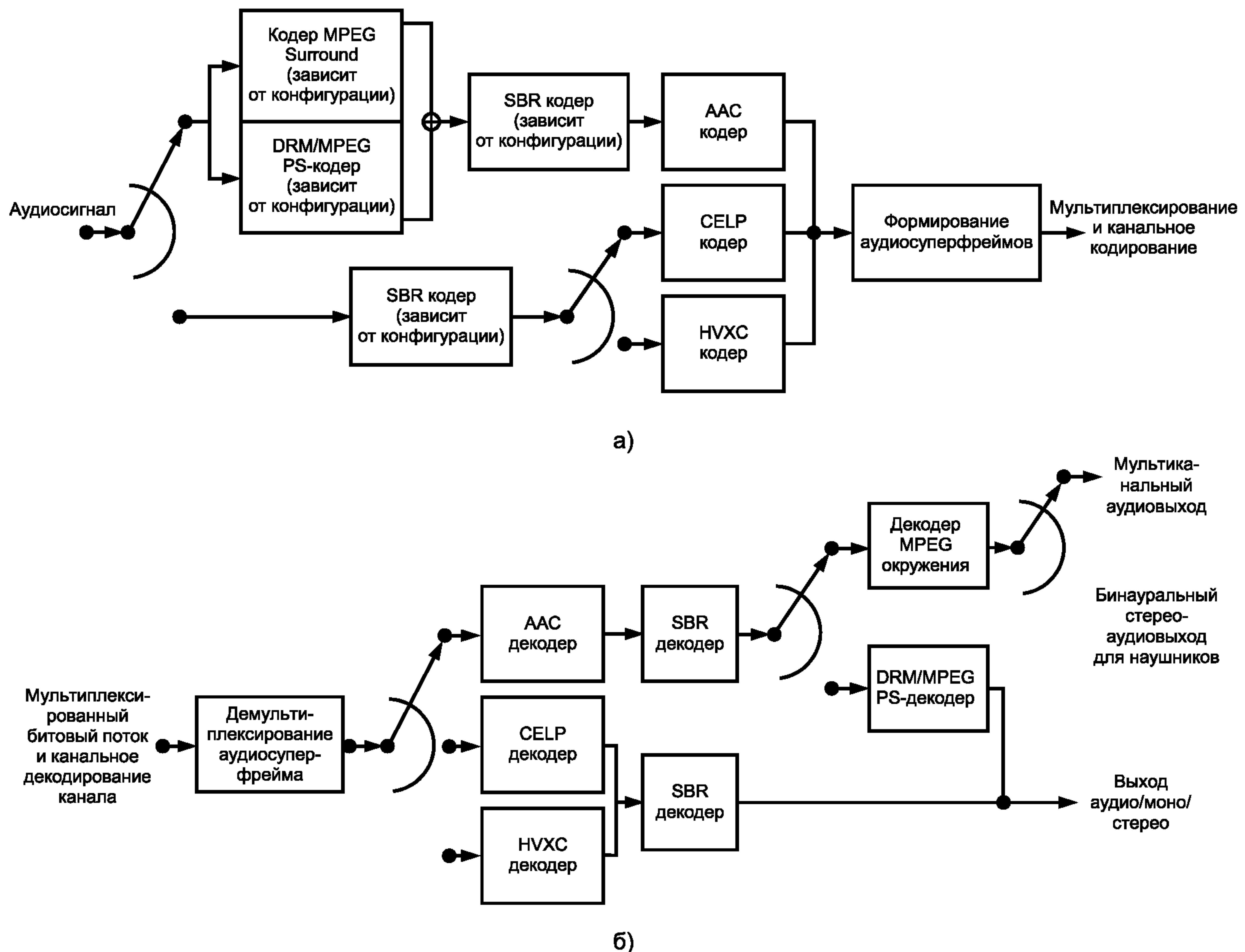
Рисунок 2 — Кодирование (а) и декодирование (б) источников аудиосигналов
