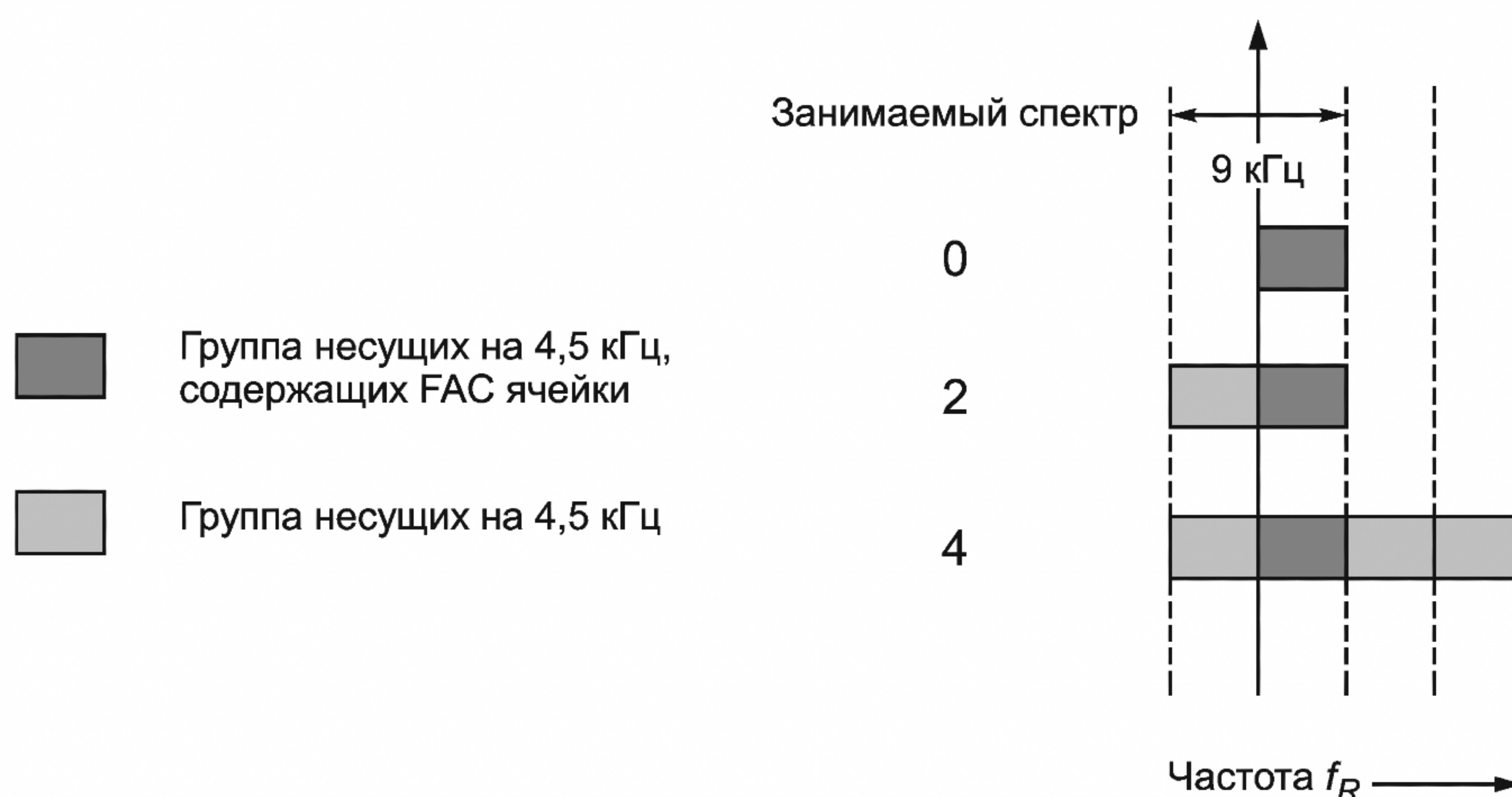
Рисунок 7 — Занимаемый спектр для 9 кГц каналов
