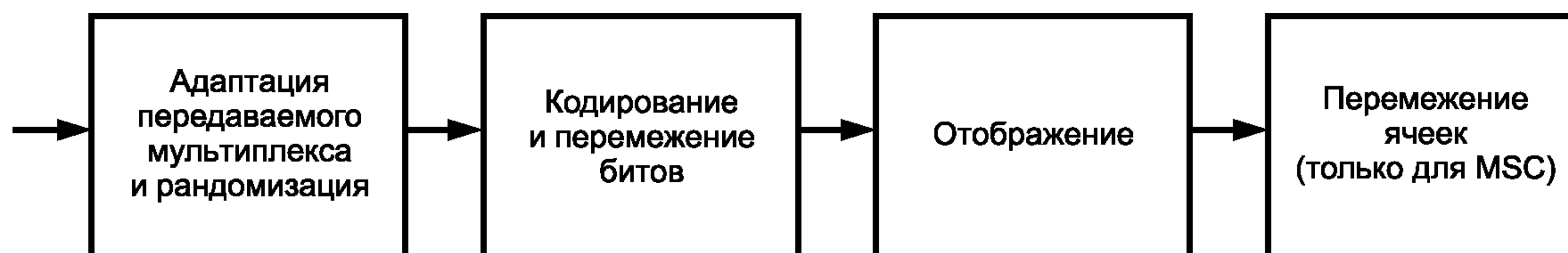
Рисунок 3 — Функциональная блок-схема кодирования и перемежения
