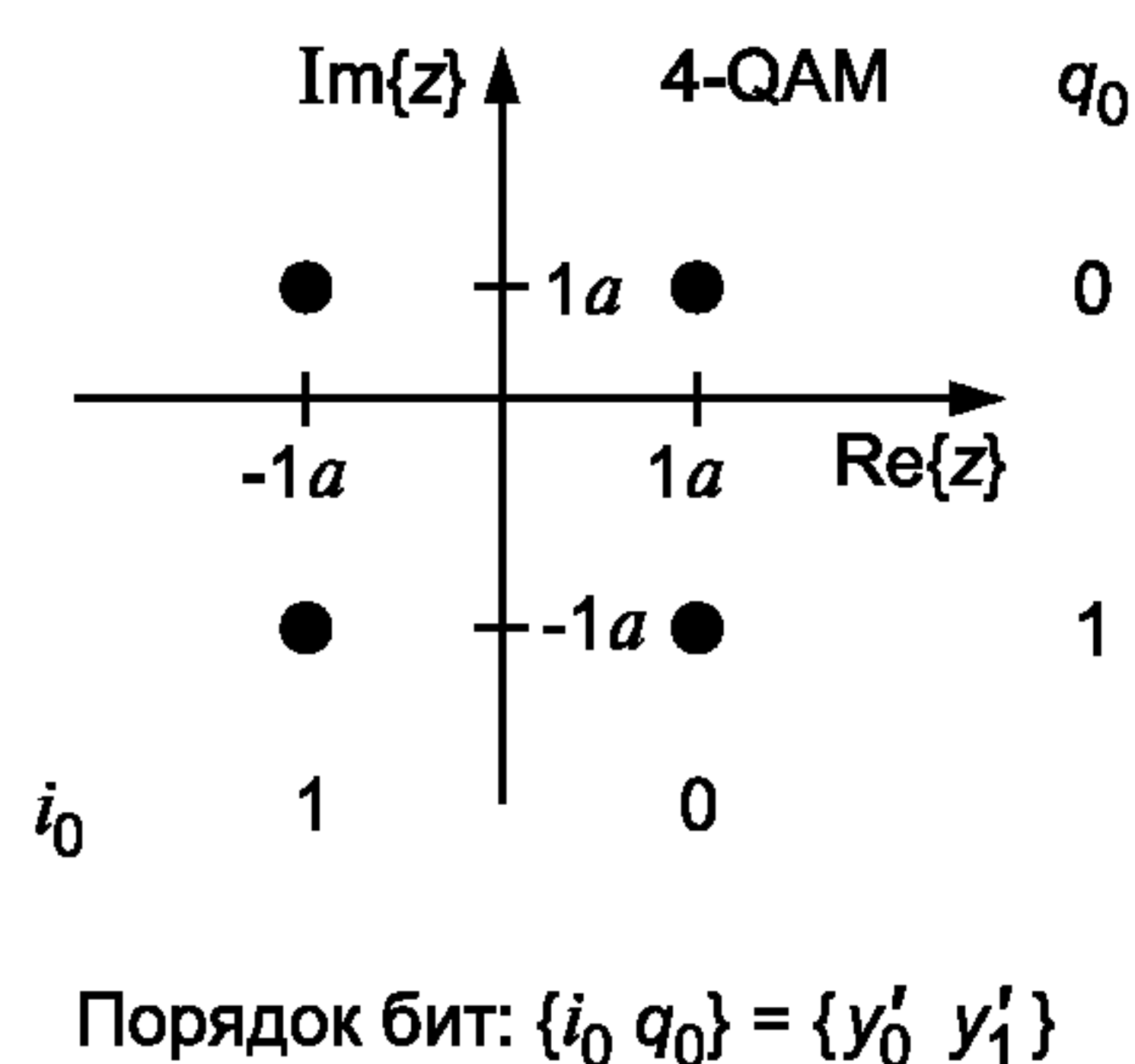
Рисунок 6 — SM 4-QAM отображение с соответствующей битовой комбинацией
