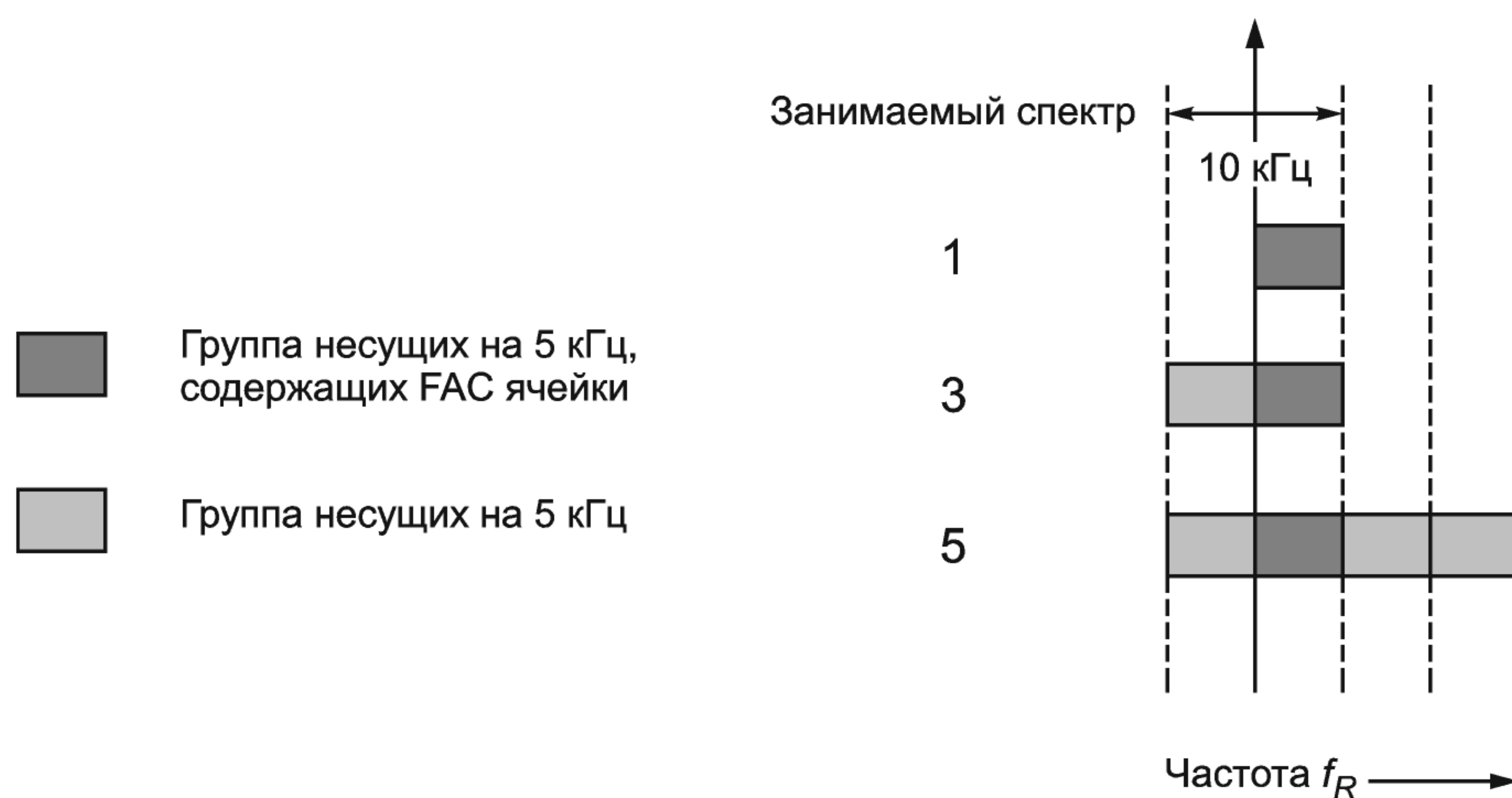
Рисунок 8 — Занимаемый спектр для 10 кГц каналов
