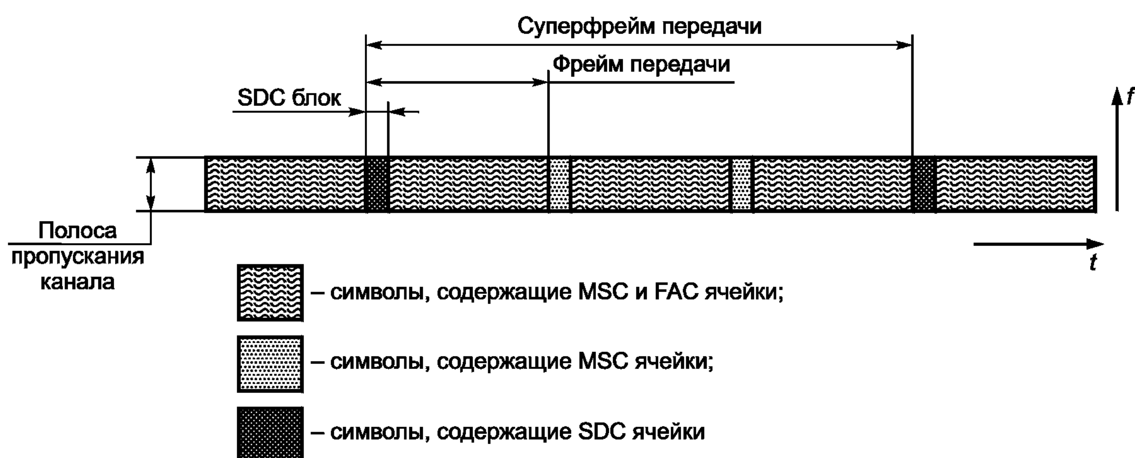
Рисунок 9 — Частотно-временное расположение FAC и SDC сигналов
