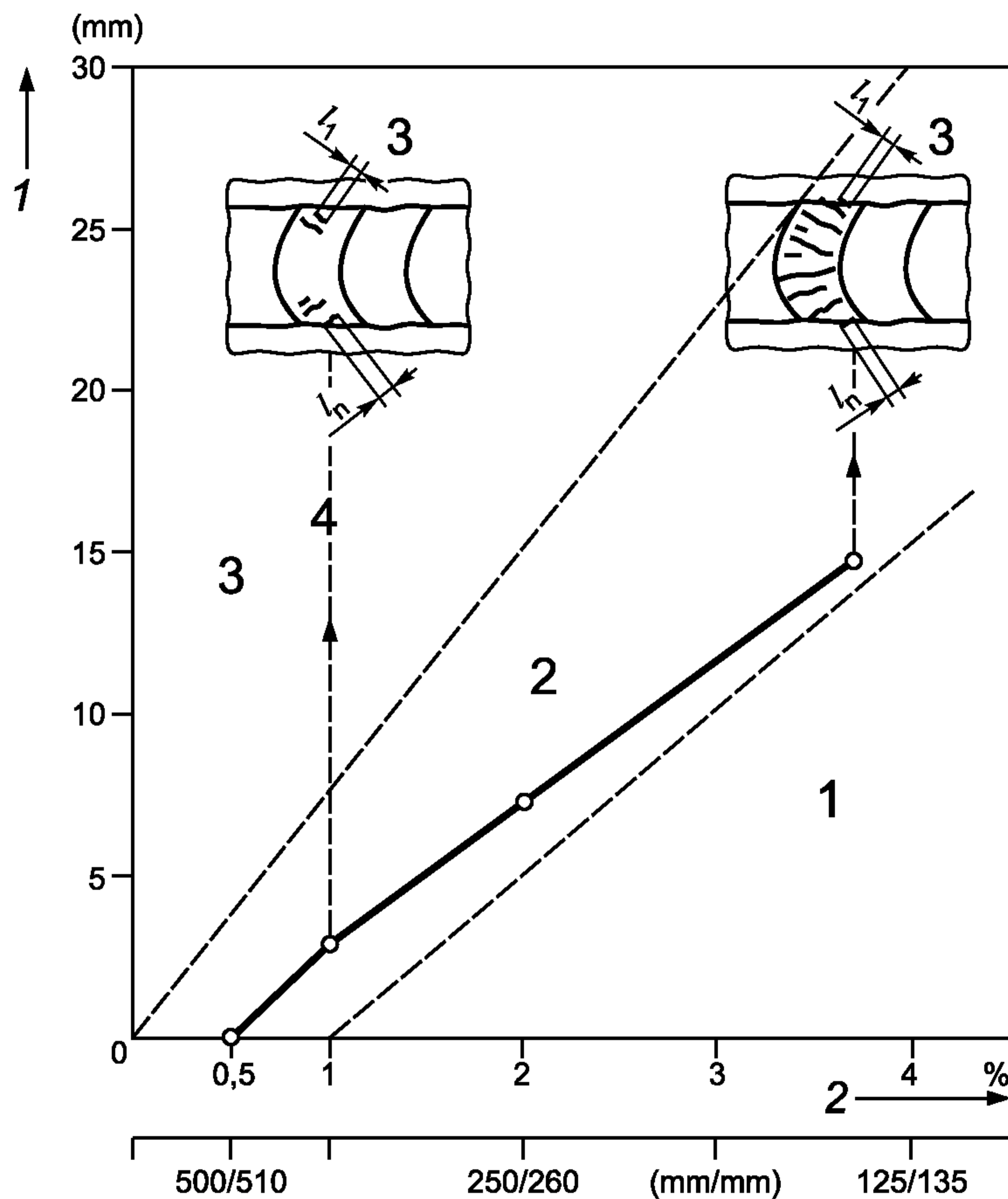
1 — суммарная длина трещин; 2 — радиус оправки/плунжера; 3 — образец для испытания нагрузкой, действующей вдоль сварного шва; 4 — длина, измеренная стереомикроскопом с 25-кратным увеличением: L_{tot} = l_1 + l_2 + \dots + l_n , 5 — скорость сварки; область 1 — высокая сопротивляемость образованию горячих трещин; область 2 — увеличенный риск образования горячих трещин; область 3 — высокий риск образования горячих трещин
