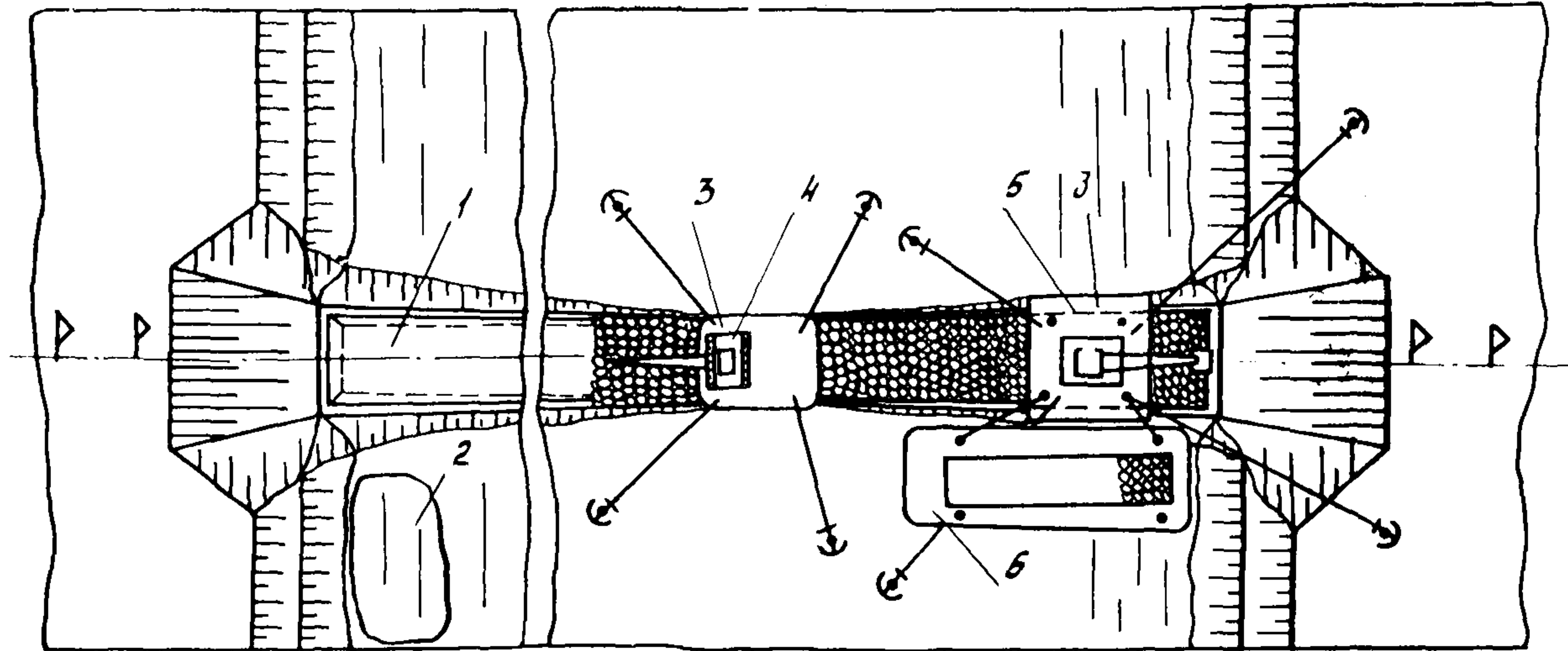
Рис.6. Схема одновременного послойного разрыхления и удаления скального грунта из подводной траншеи перехода трубопровода с применением двух экскаваторов ЭО-4121А (ЭО-5122) на отдельных понтонах (один из экскаваторов с гидромолотом СП-62 разрыхляет породу, второй — ковшом извлекает и грузит ее в шаланду): 1—траншея; 2—отвал; 3—механизированные понтоны; 4—экскаватор с гидромолотом СП-62; 5—экскаватор с ковшом; 6—шаланда
