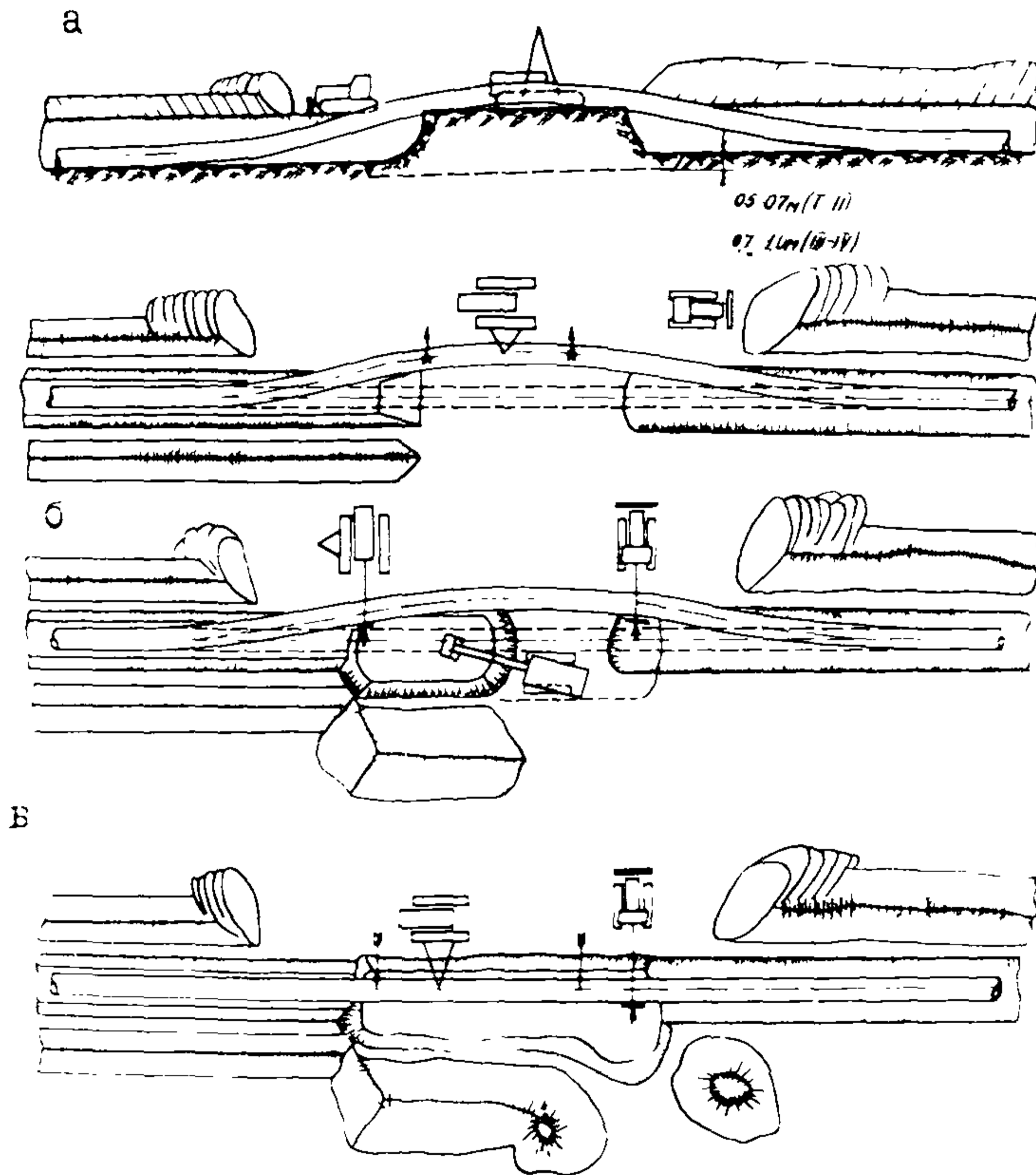
Рис.8. Укладка коротких изолированных плетей трубопровода: а-смещение плети от проектной оси; б-разработка перемычки одноковшовым экскаватором; в-укладка плети на дно траншеи
