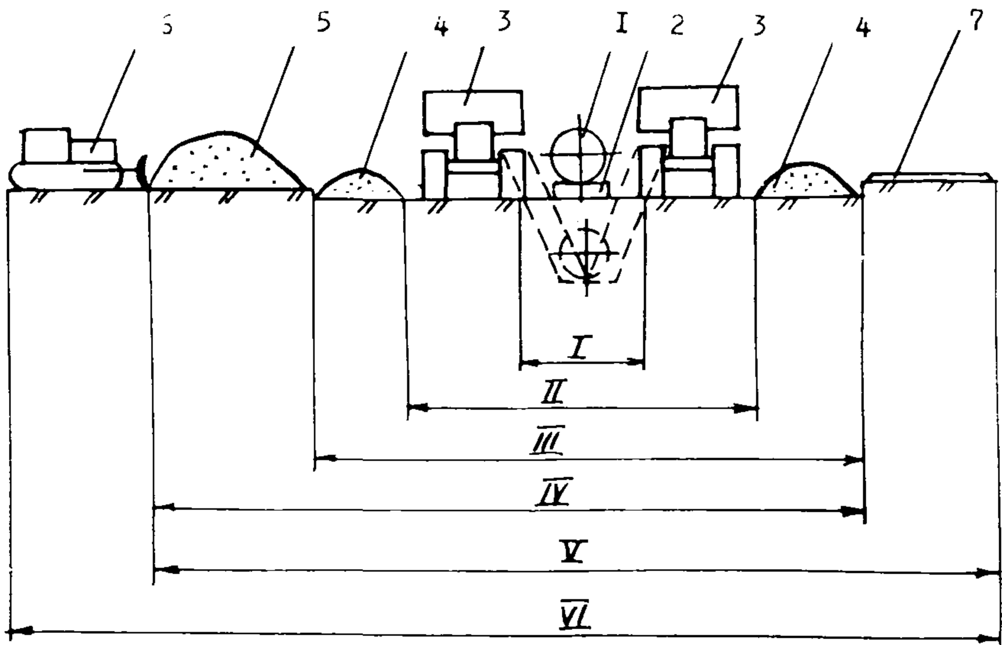
Рис.4. Полосы отвода (I-VI) для двухроторного двухотвального экскаватора-трубозаглубителя:
