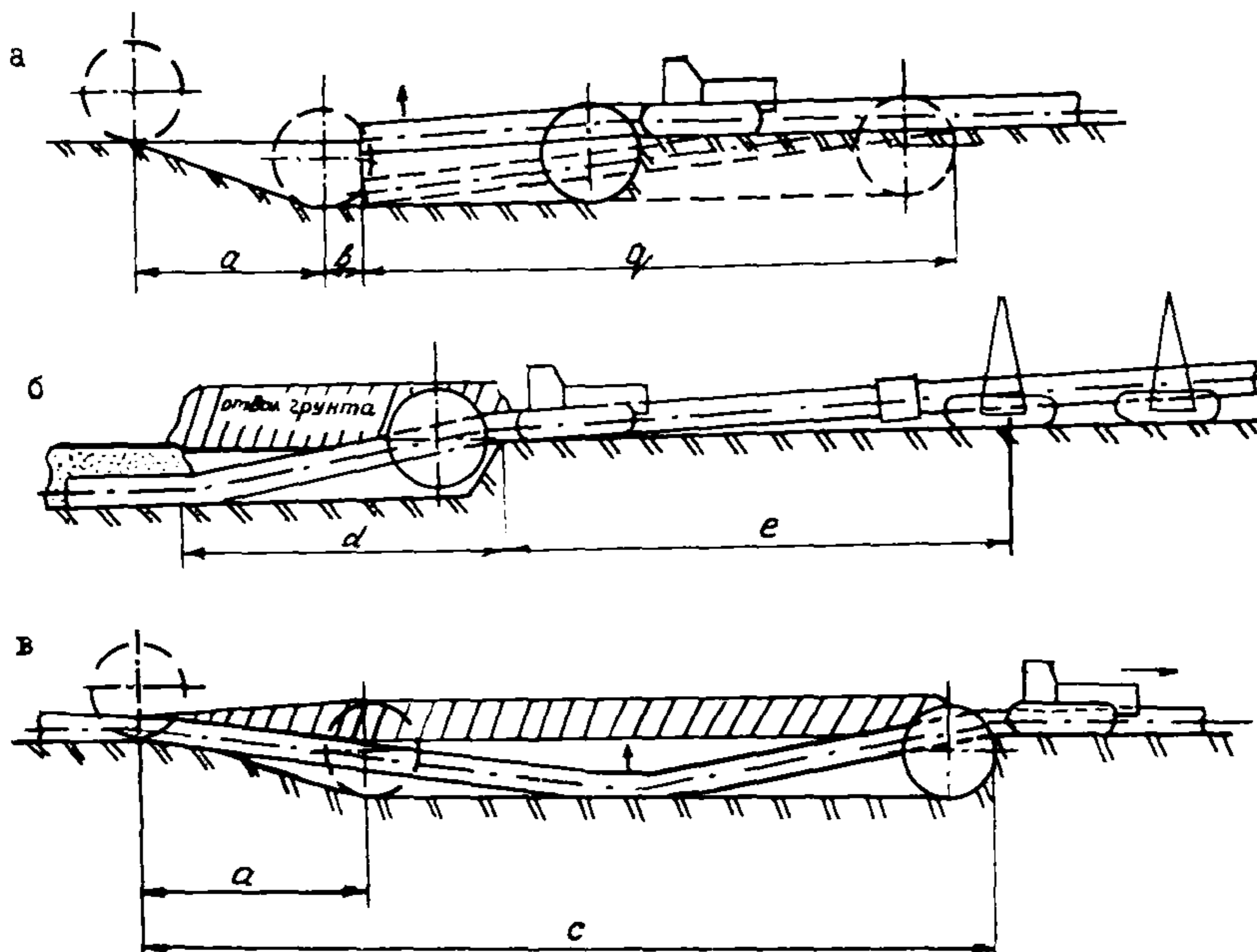
Рис.5. Заглубление экскаватора-трубозаглубителя:
