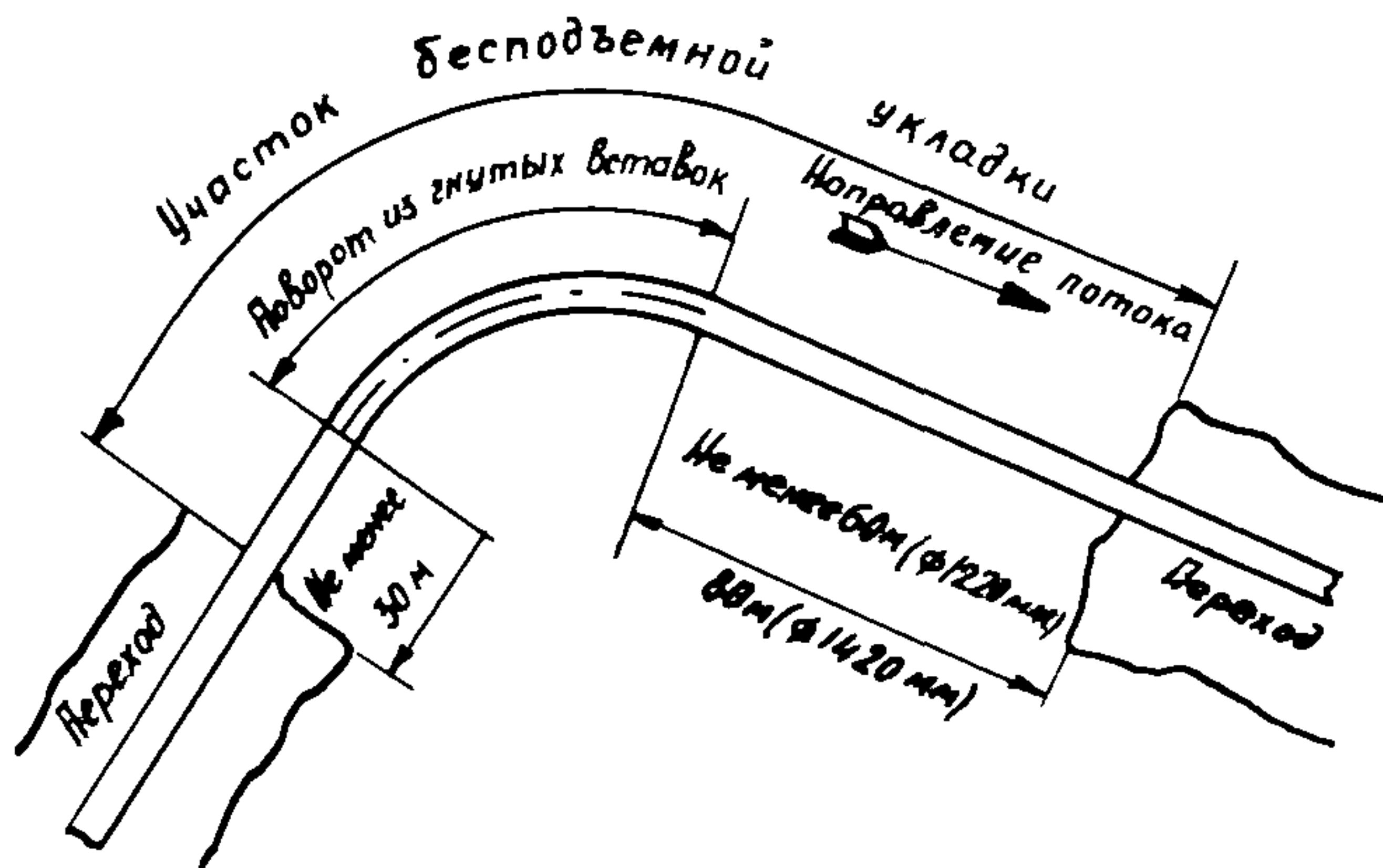
Рис.3. Переходы на участке трассы трубопровода, сооружаемого из гнутых вставок
