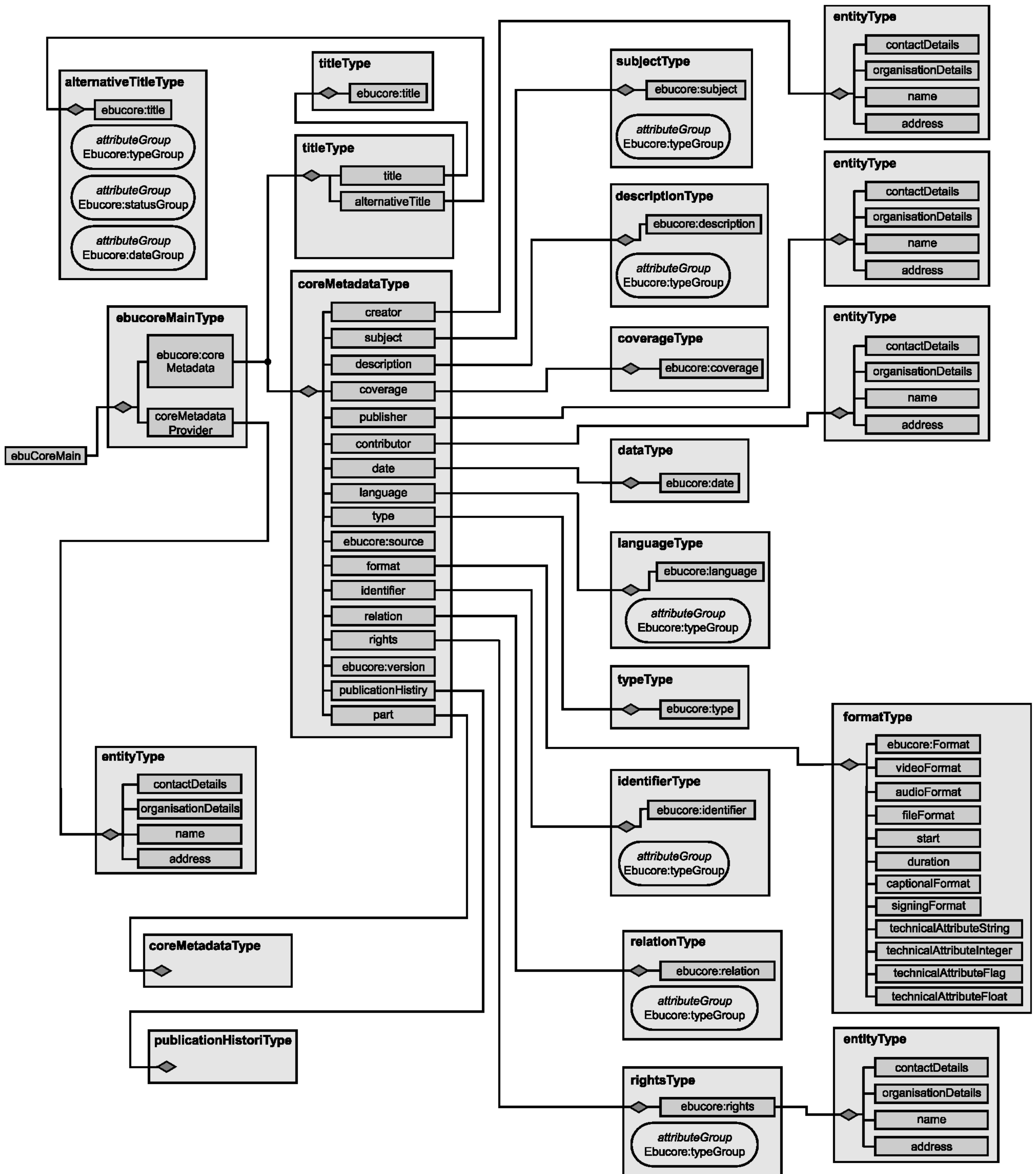
Рисунок 6.3 — Графическое представление XSD-файла, определяющего схему организации XML-документов
