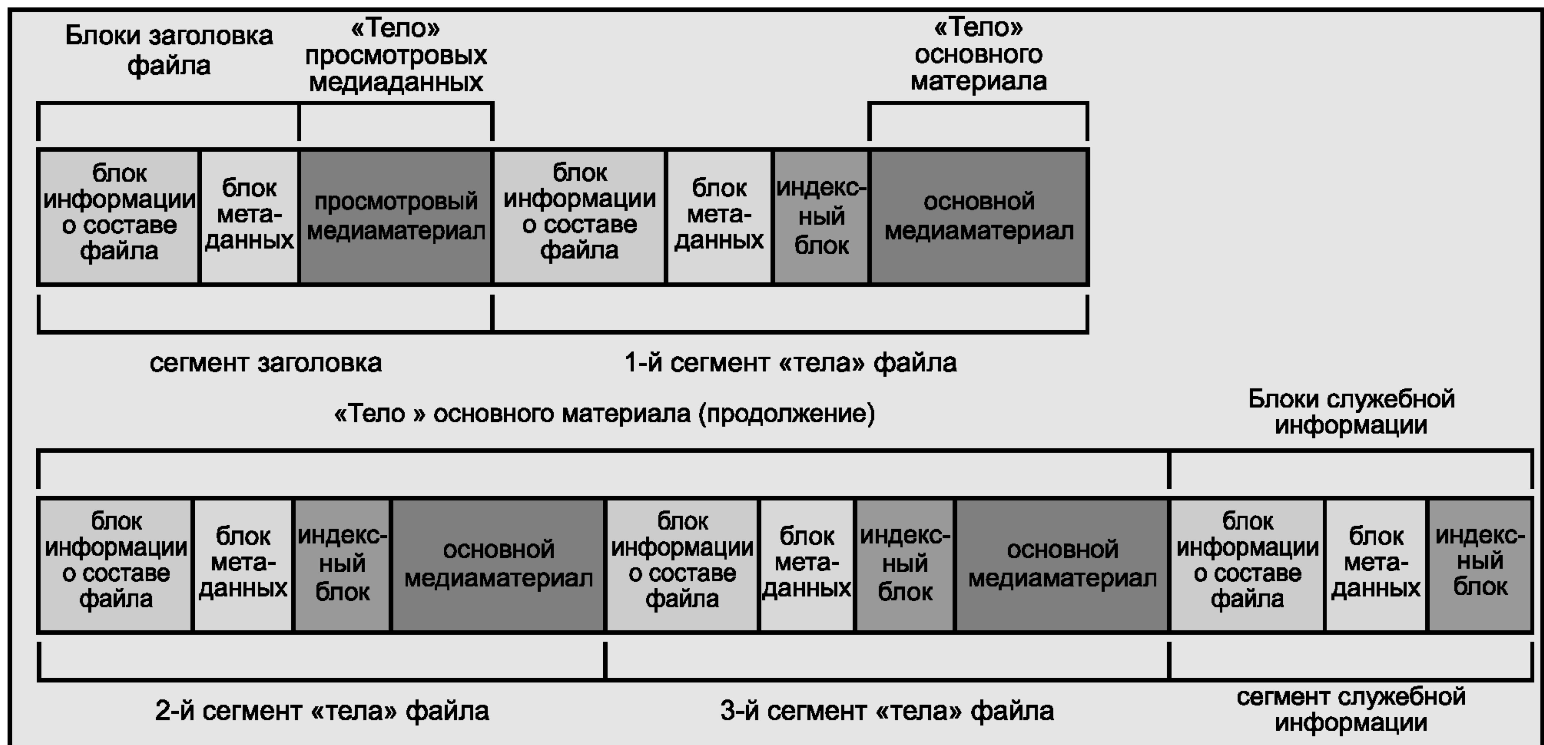
Рисунок П.3 — Схема MXF-файла, содержащего в сегменте заголовка контейнер просмотра, за которым следуют три сегмента тела файла
