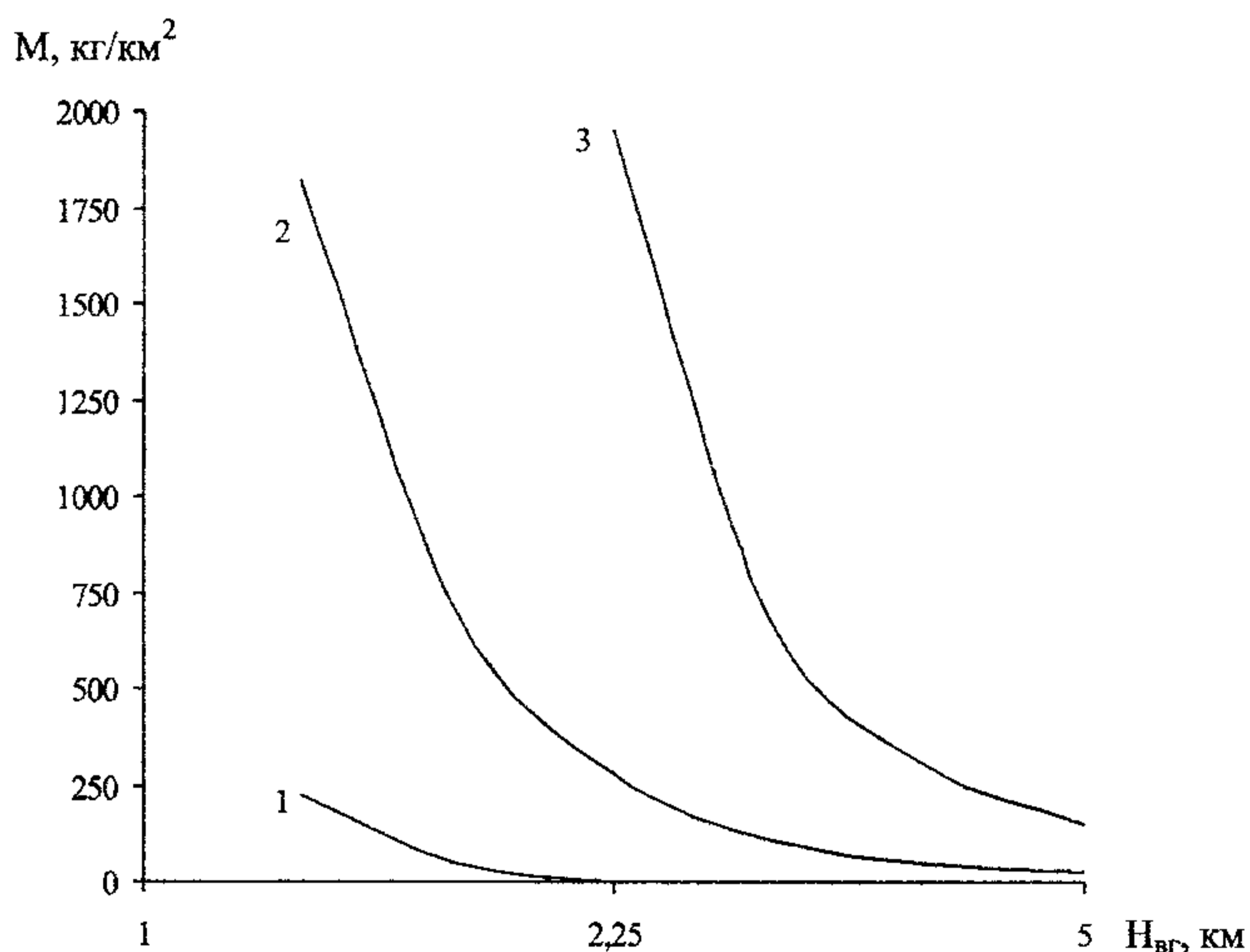
Рис. 8.2 – Зависимость оптимального количества реагента M от H_{\text{вг}} и \Gamma_0 . 1 – \Gamma_0 = 30 \text{ мкм} , 2 – \Gamma_0 = 60 \text{ мкм} , 3 – \Gamma_0 = 100 \text{ мкм}
