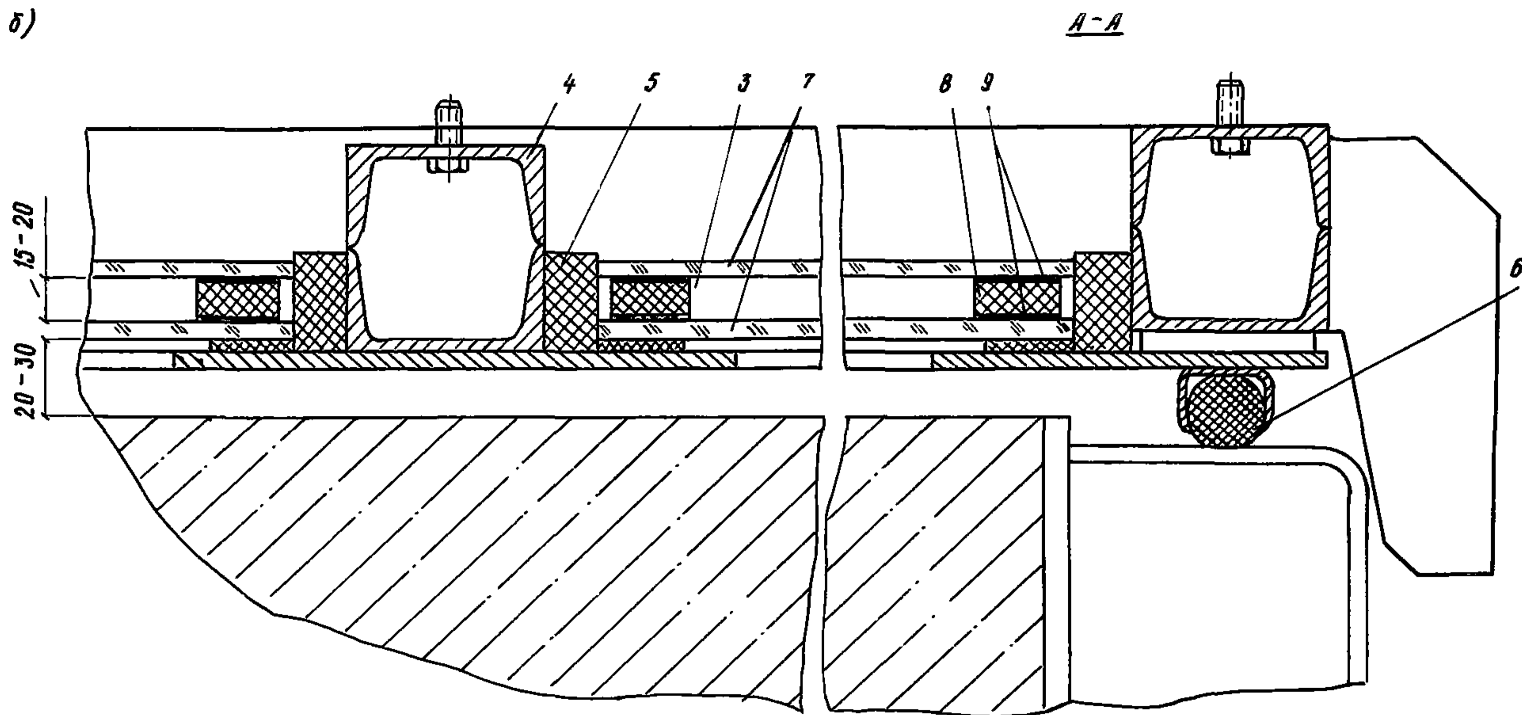
Рис. 9. Гелиокрышка со светопрозрачным вкладышем из стекла
