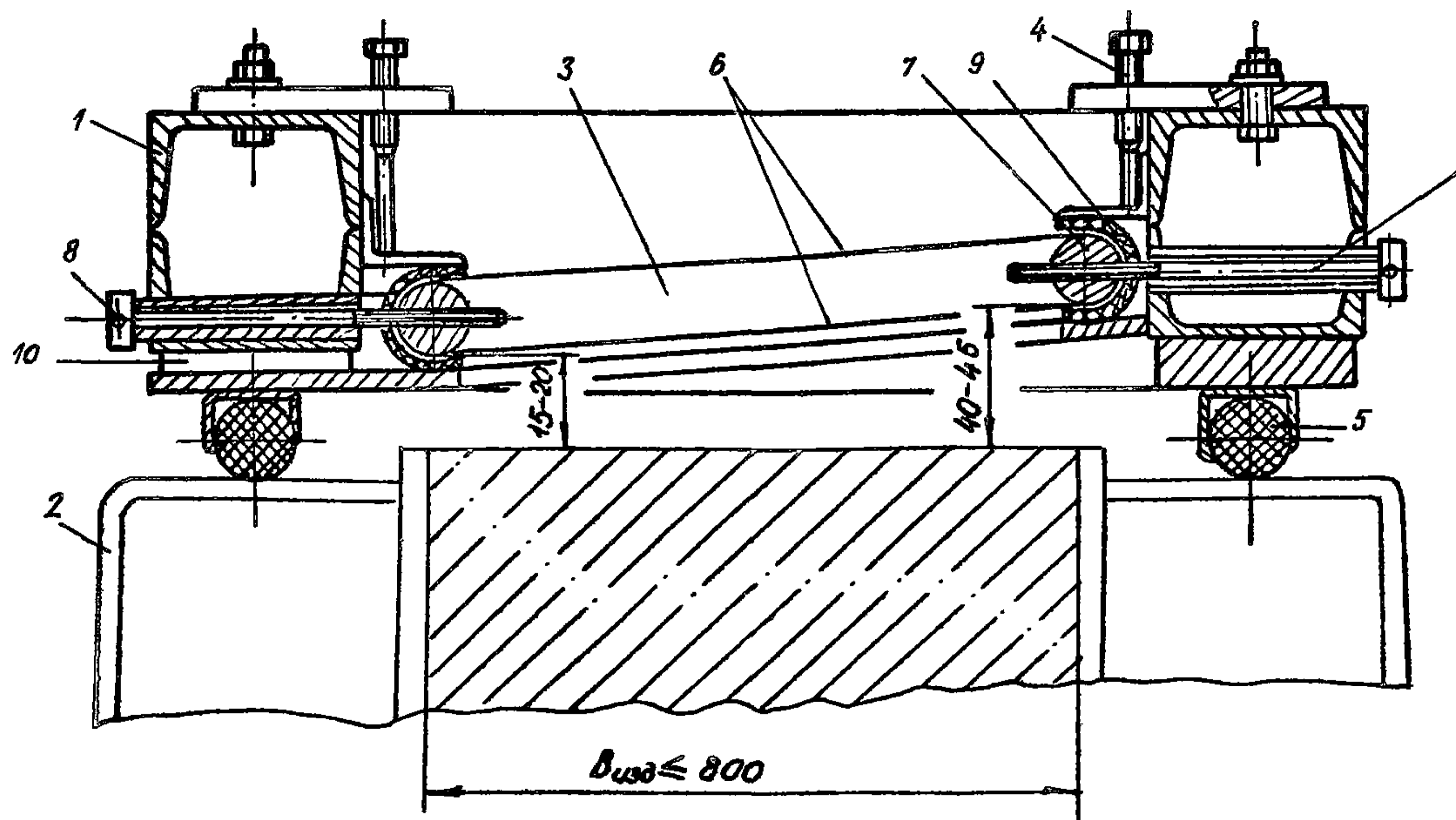
Рис. 5. Гелиокрышка со светопрозрачным вкладышем (из полимерной пленки), снабженным телескопической распорной рамкой с внешним механизмом раздвижки (по а.с. № 1295630)
