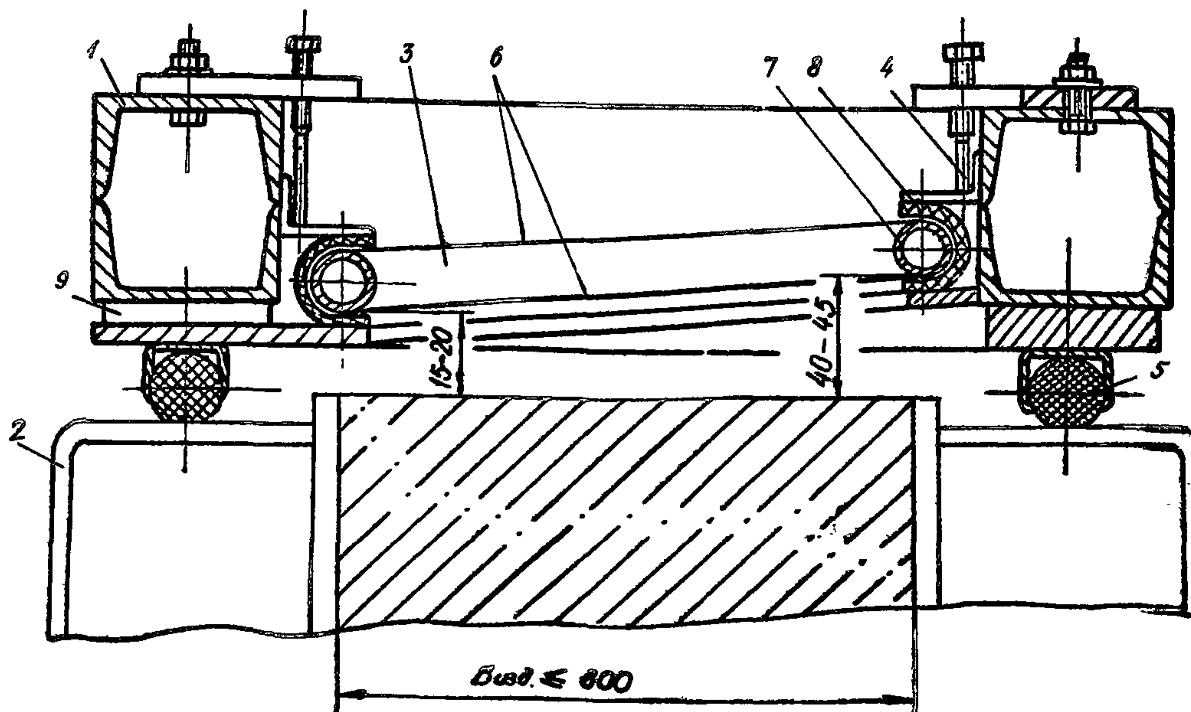
Рис. 6. Гелиокрышка со светопрозрачным вкладышем из полимерной пленки с термоусадочным натяжением (по а.с. № 1295629)
