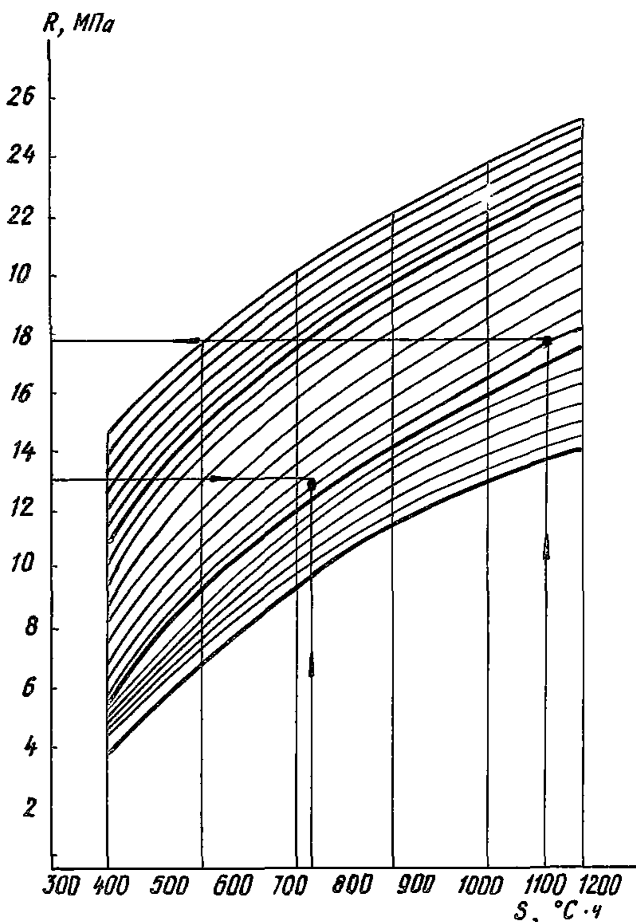
Рис. 14. Определение распалубочной прочности бетона по градуировочным зависимостям
