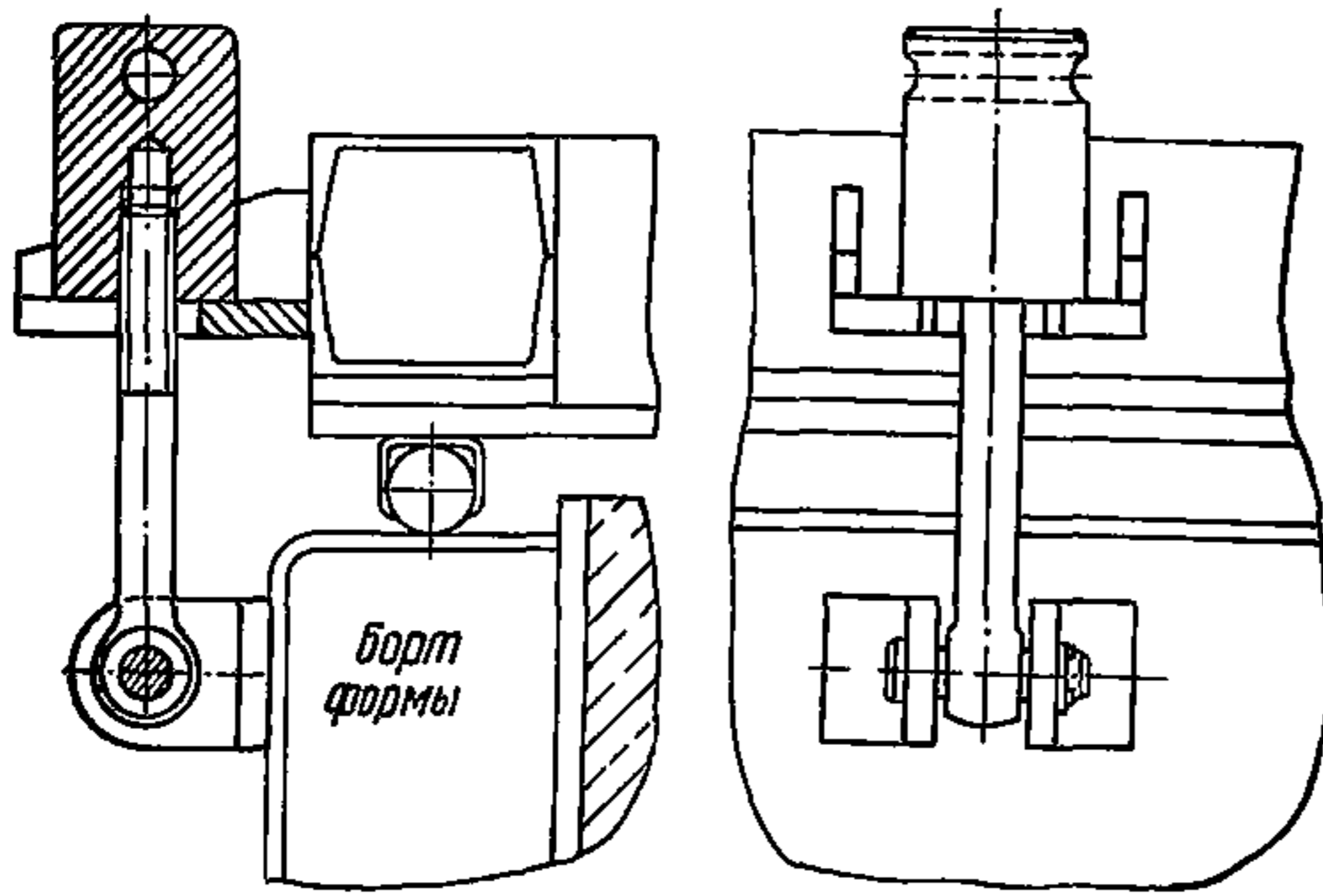
Рис. 11. Замки для соединения геликрышки с формой а - патефонного типа; б - эксцентрикового типа; в - винтового типа
