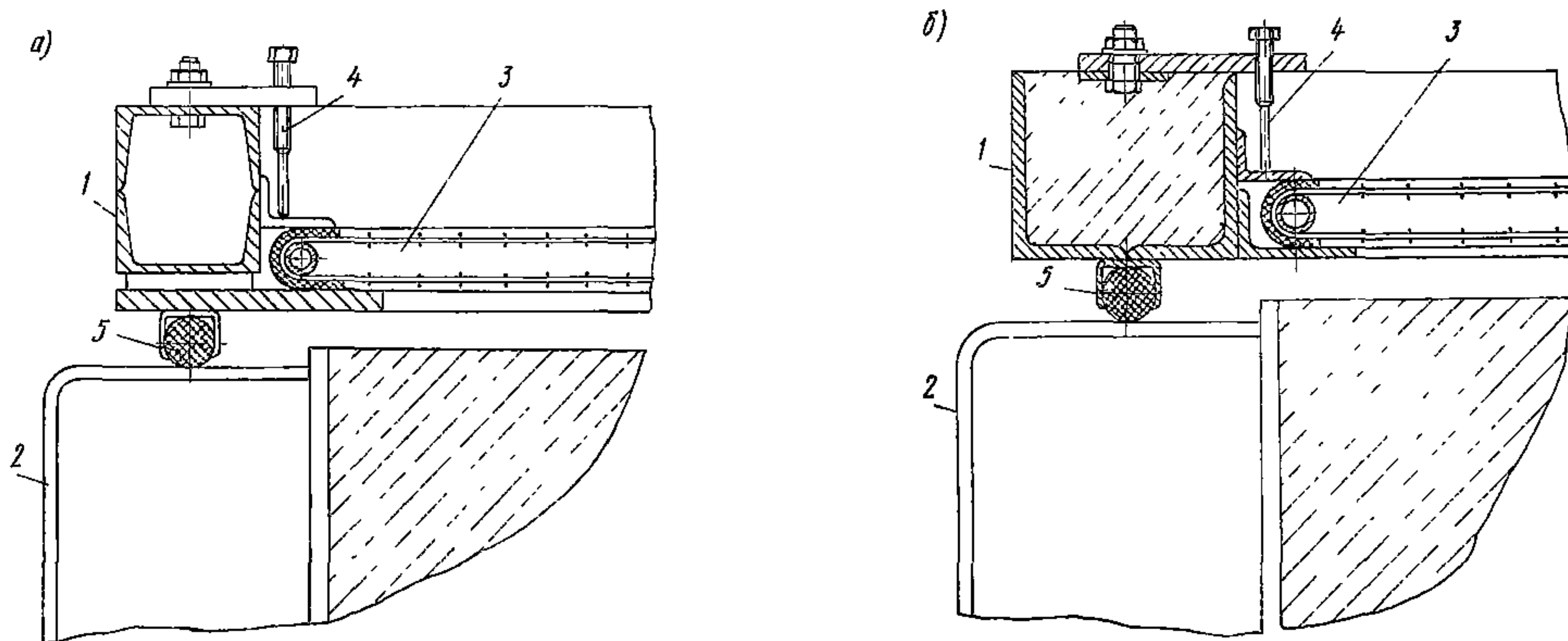
Рис. 10. Конструкция корпуса гелиокрышки
