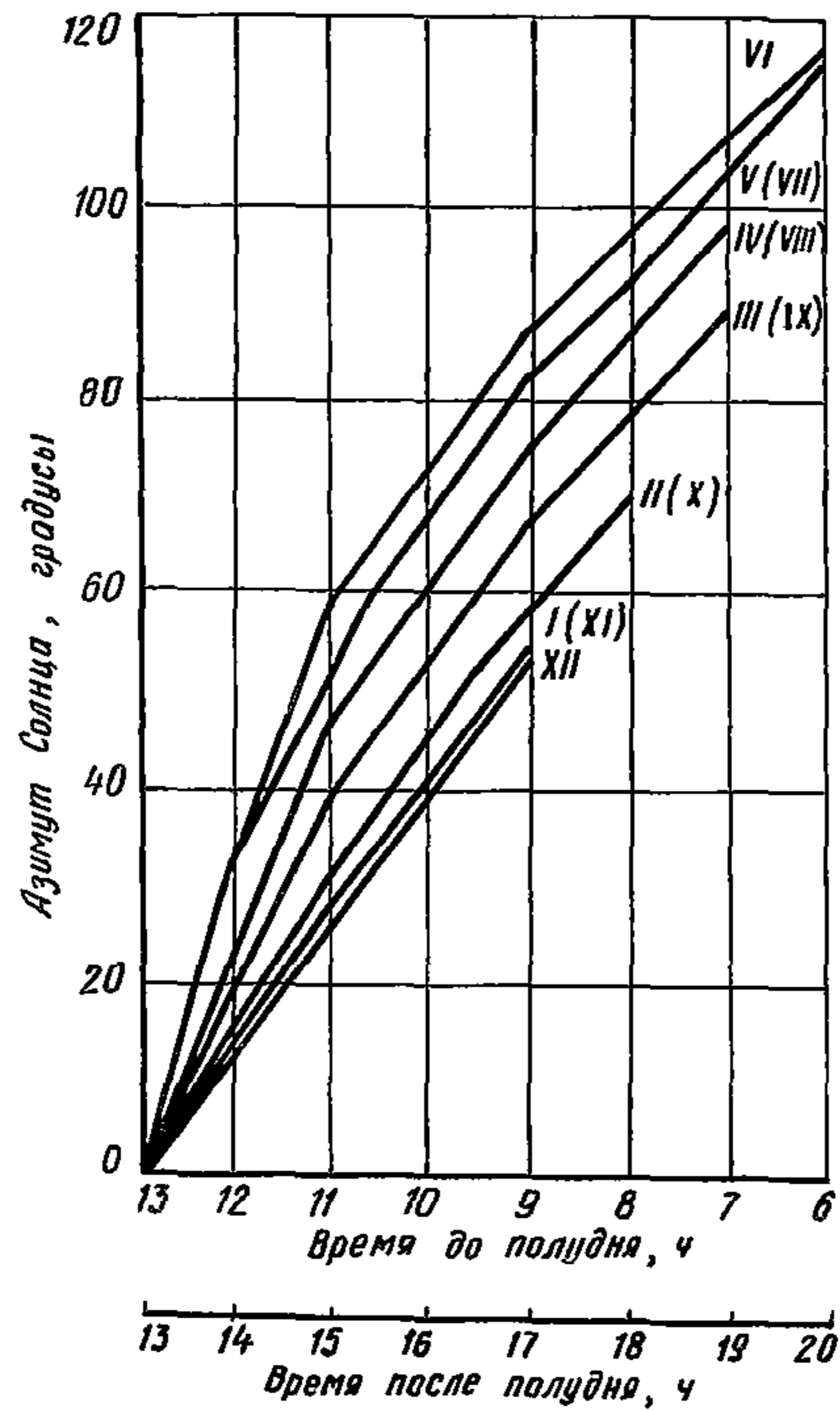
Рис. 16, д. Азимут Солнца в зависимости от времени суток и года
