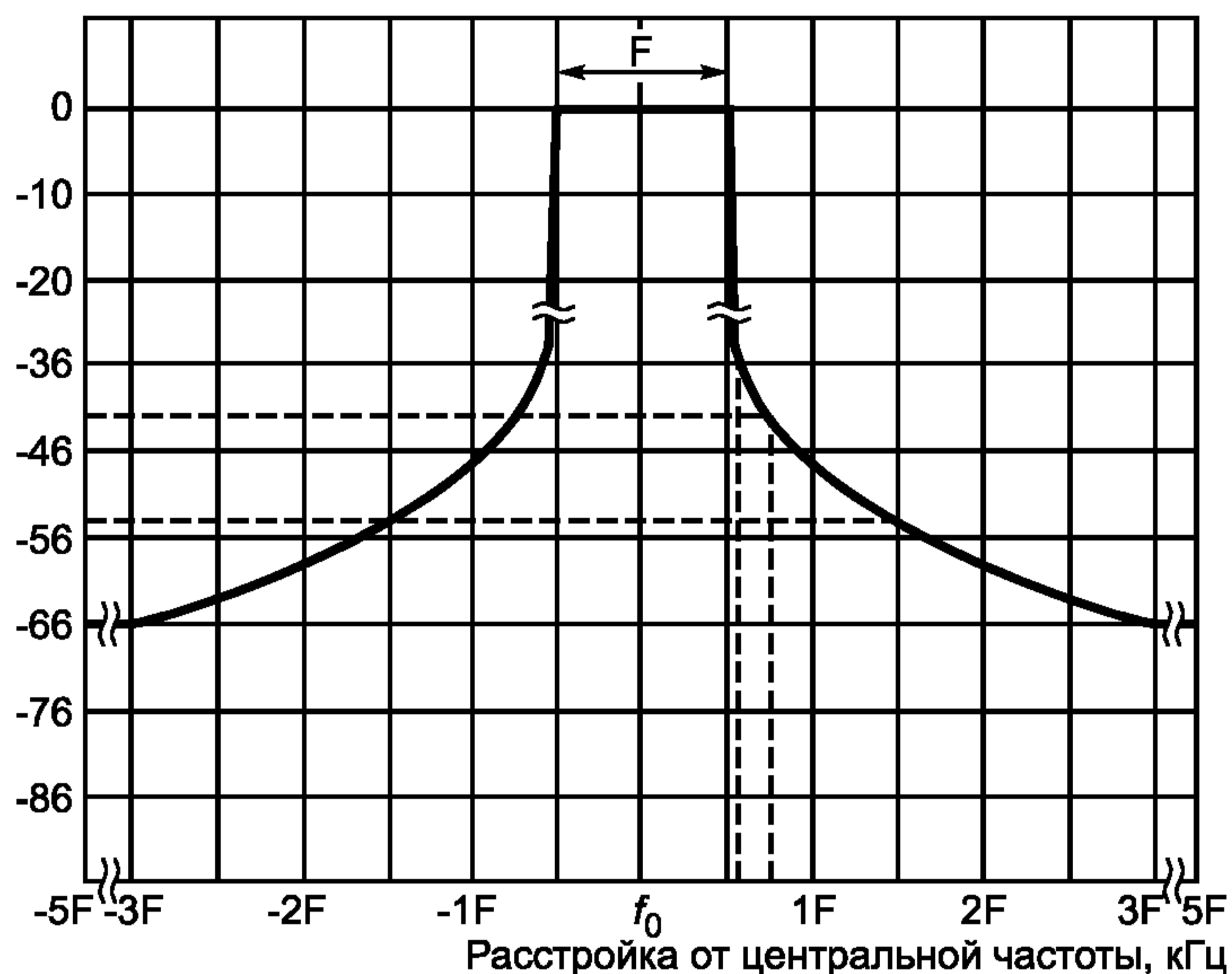
Рисунок 1 — Маска огибающей внеполосных радиоколечаний в линейных координатах
