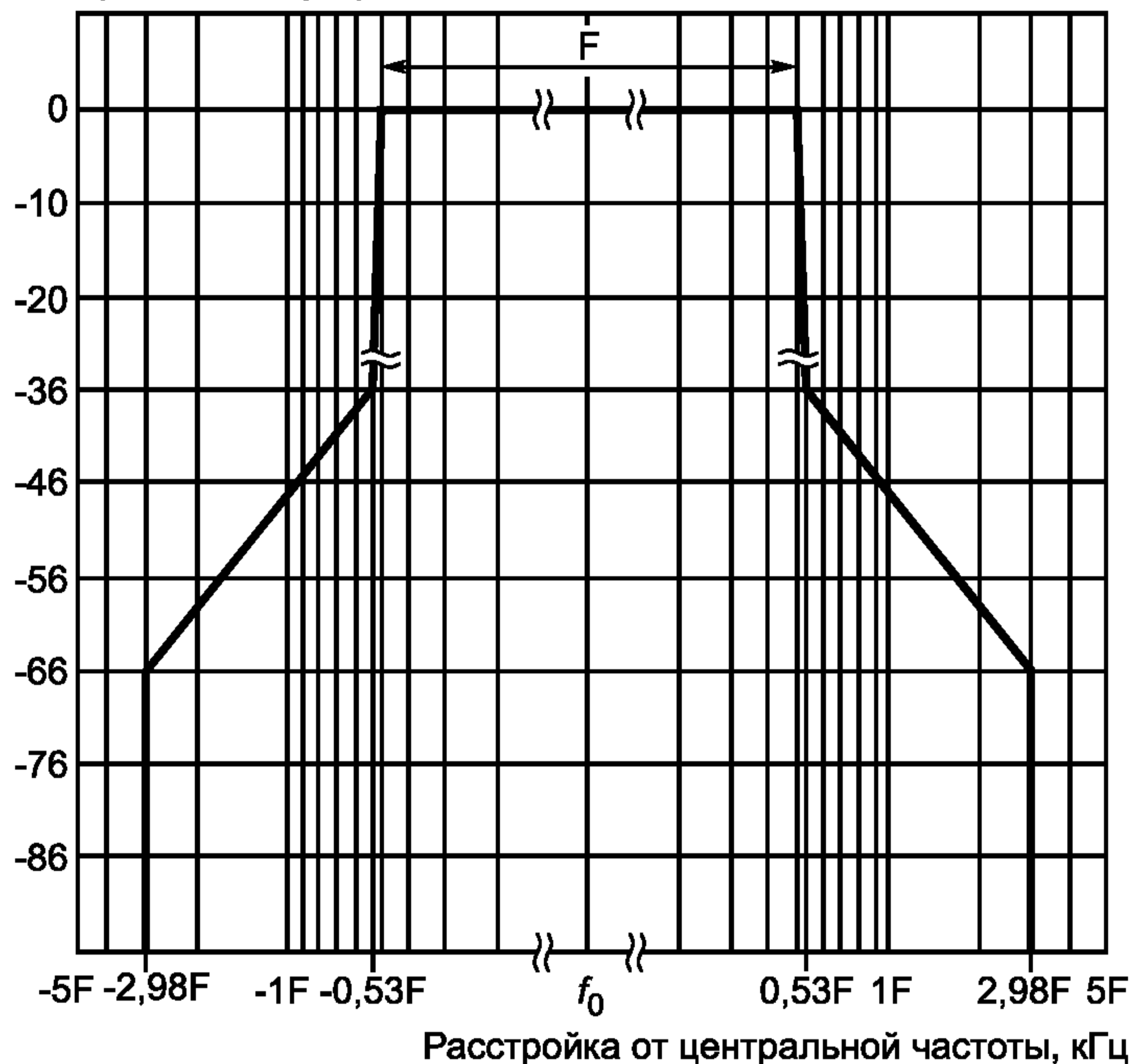
Рисунок 2 — Маска огибающей внеполосных радиоколечаний в логарифмических координатах
