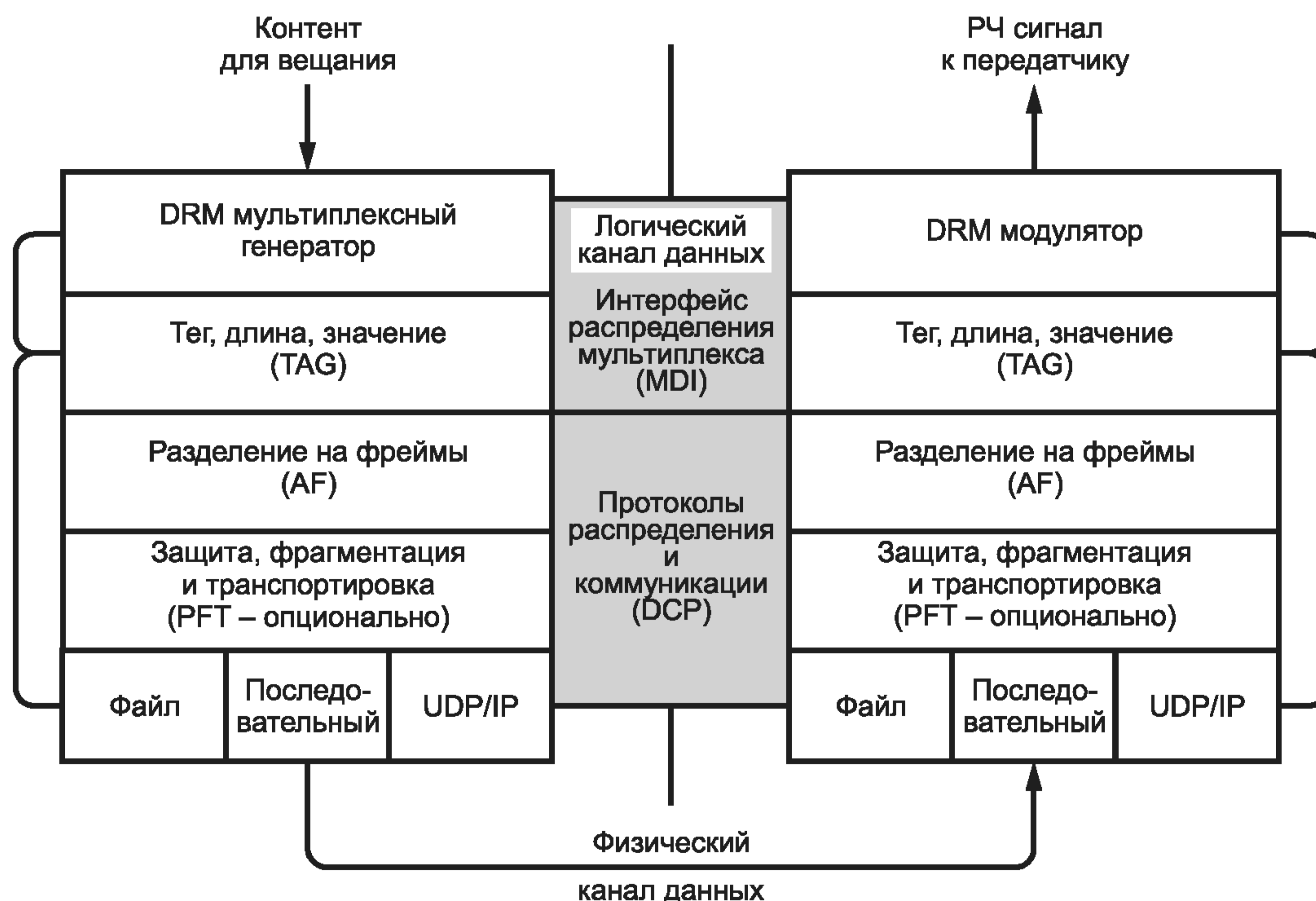
Рисунок 1 — MDI и стек протокола DCP
