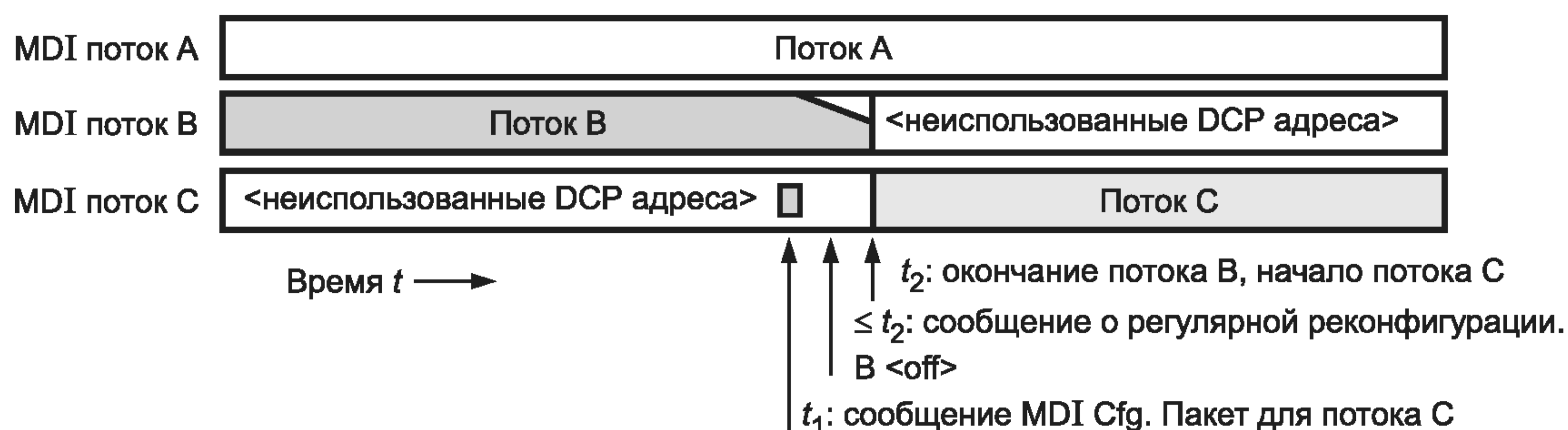
Рисунок Г.2 — Передача двух параллельных MDI потоков
