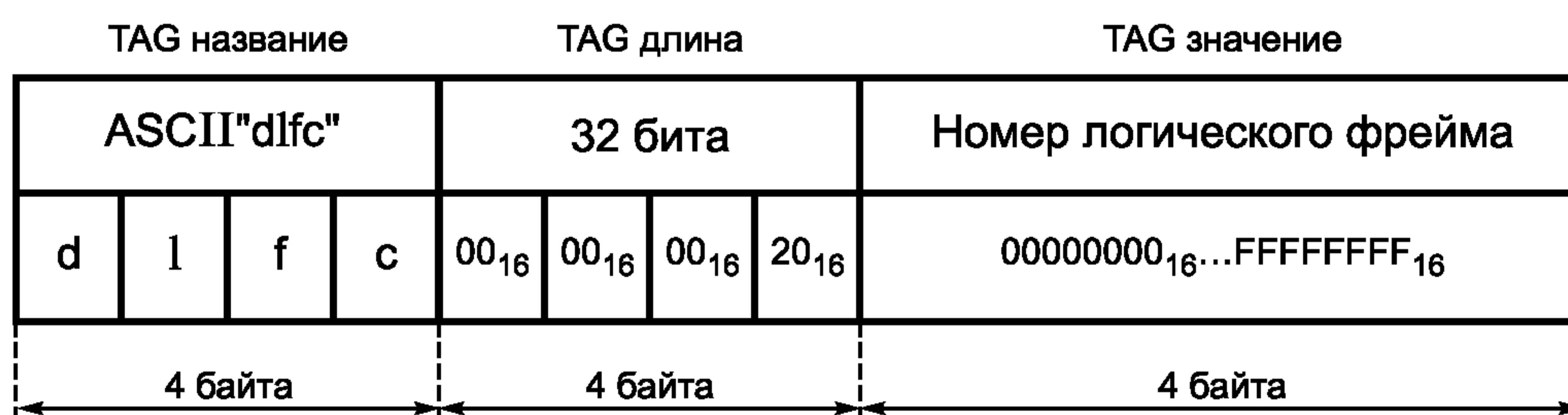
Рисунок 4 — Номер DRM логического фрейма
