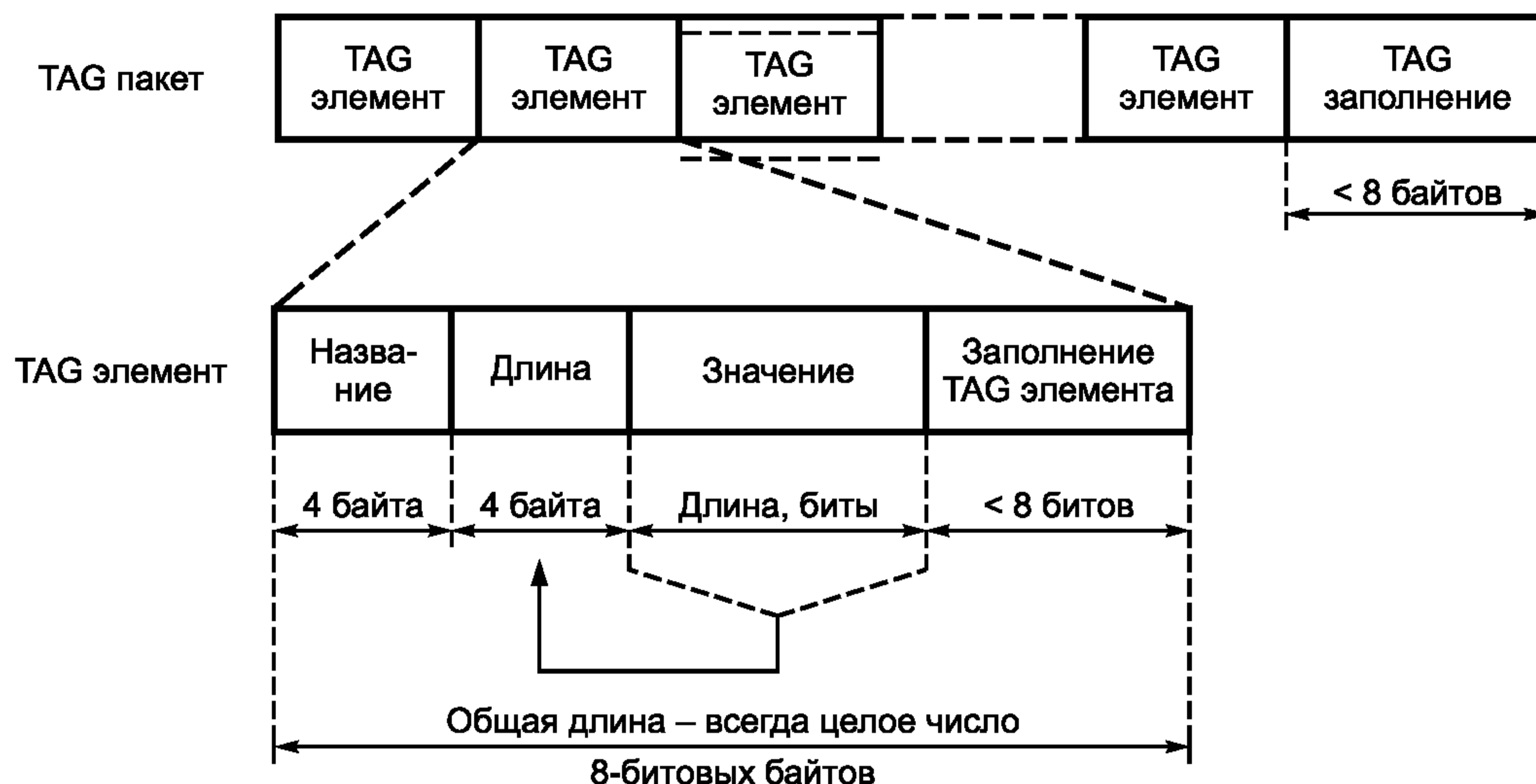
Рисунок 2 — Структура TAG пакета и TAG элемента
