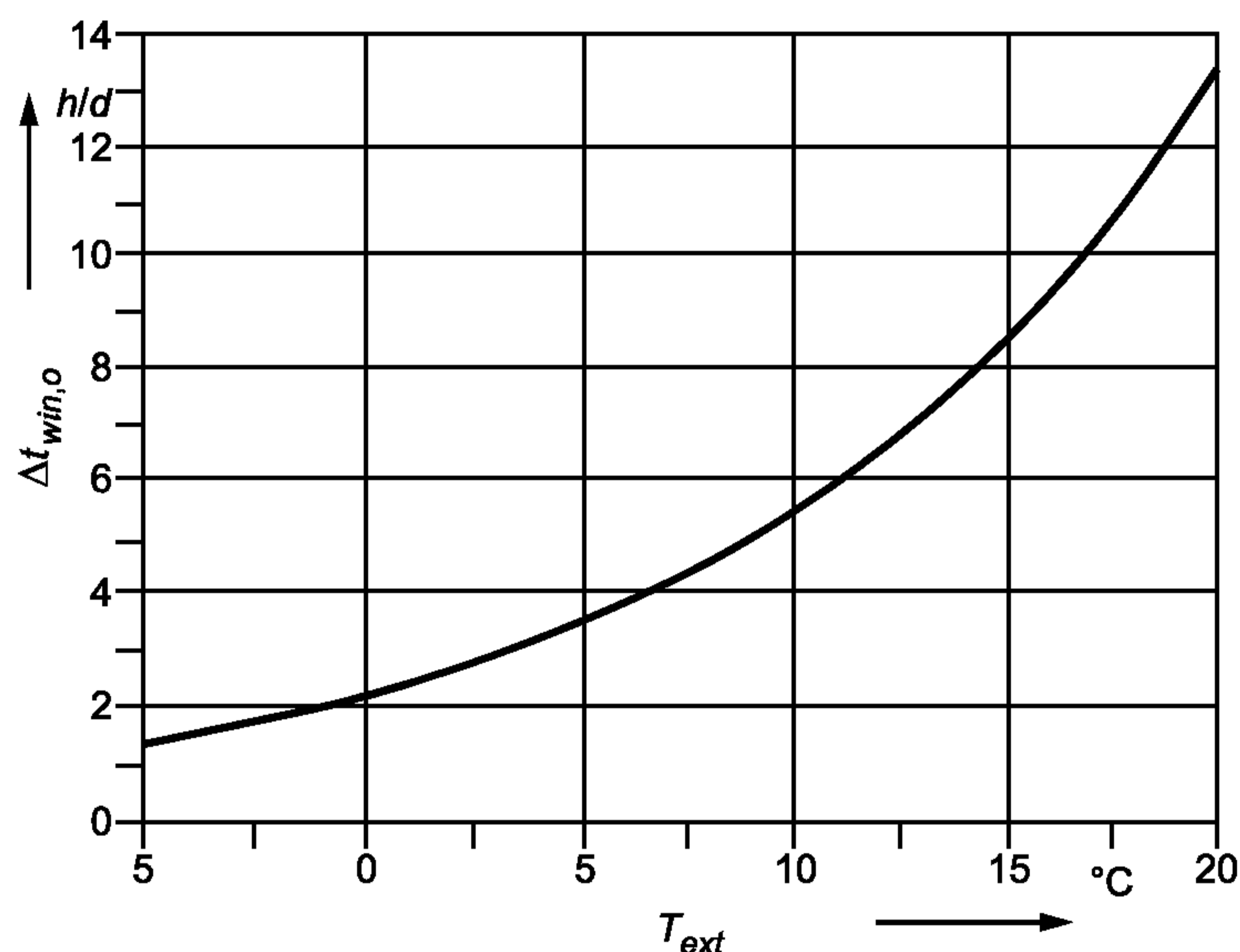
Рисунок А.3 — Продолжительность проветривания
