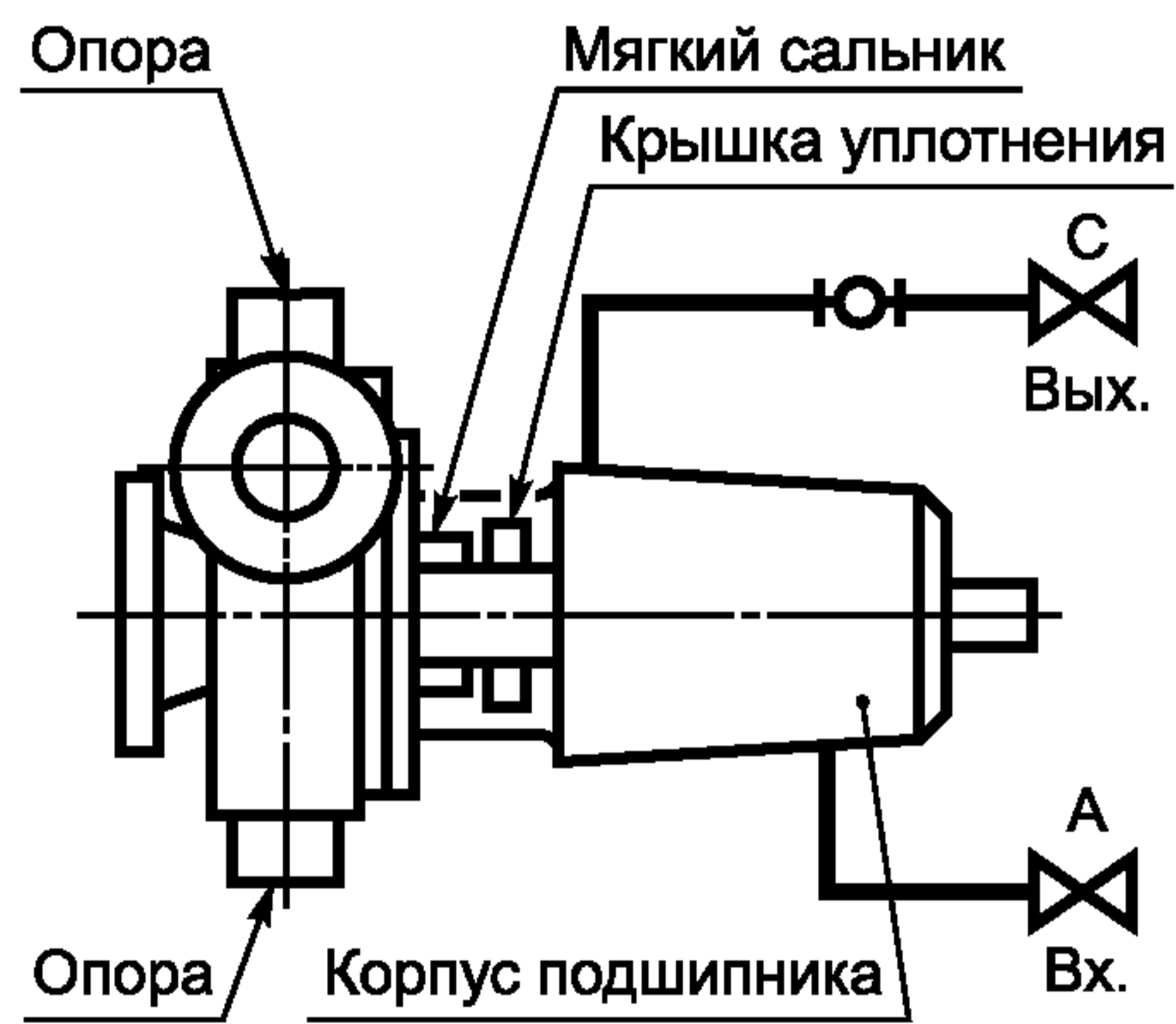
Схема А Охлаждение корпуса подшипника
