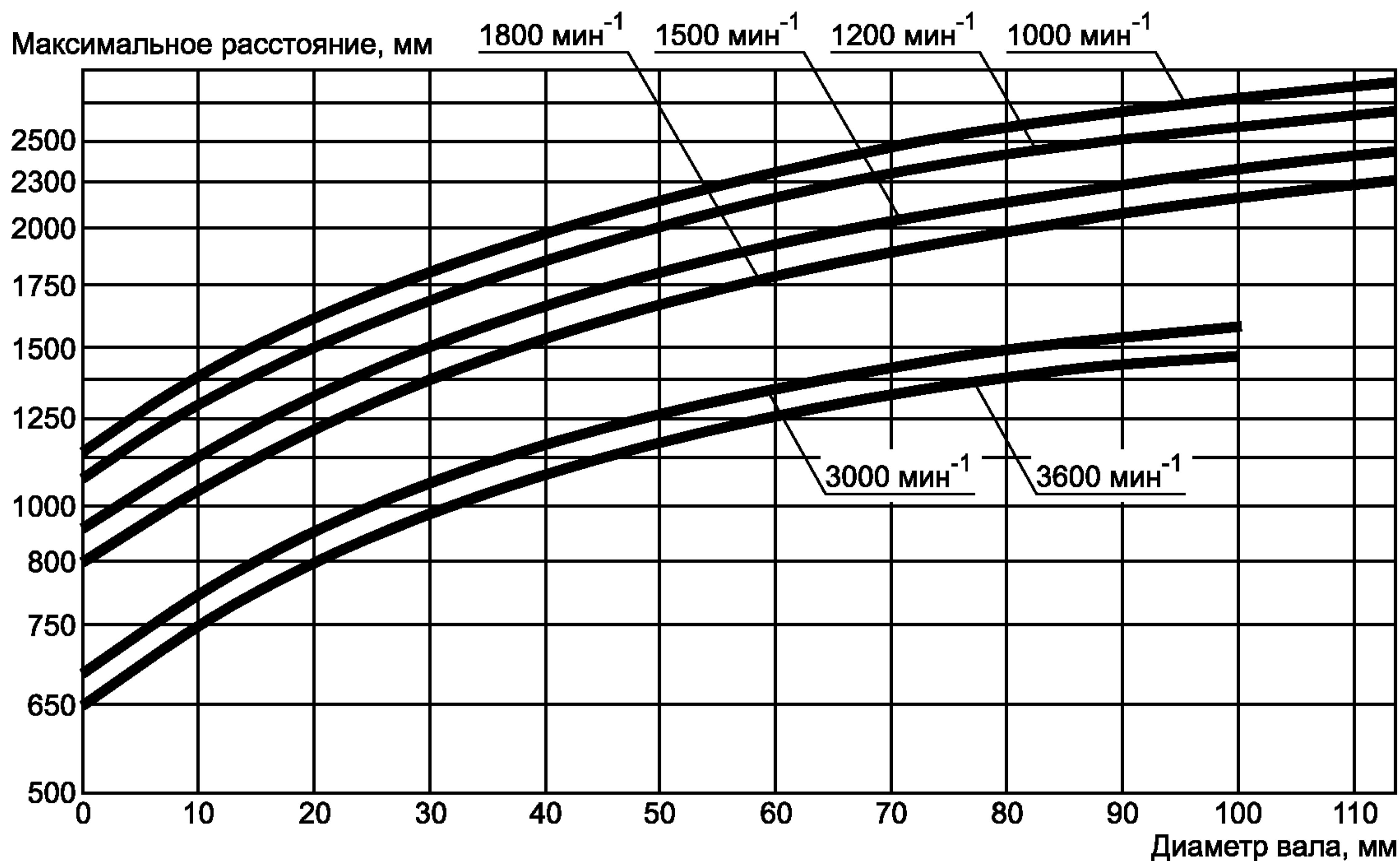
Рисунок 3 — Максимальное расстояние между направляющими втулками вала
