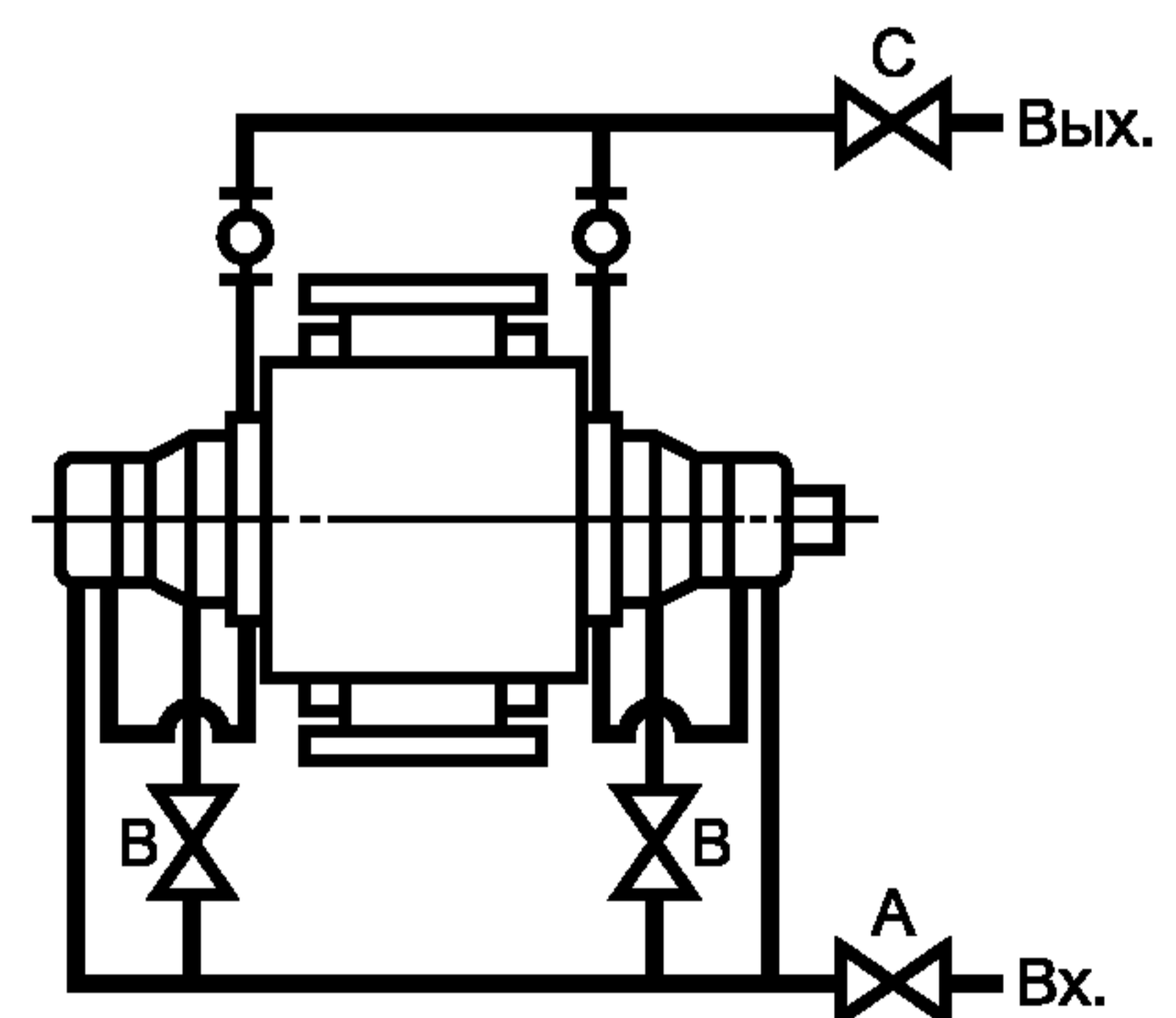
Схема F Последовательное охлаждение камеры мягкого сальника и корпуса подшипника с параллельной подачей в крышку уплотнения
