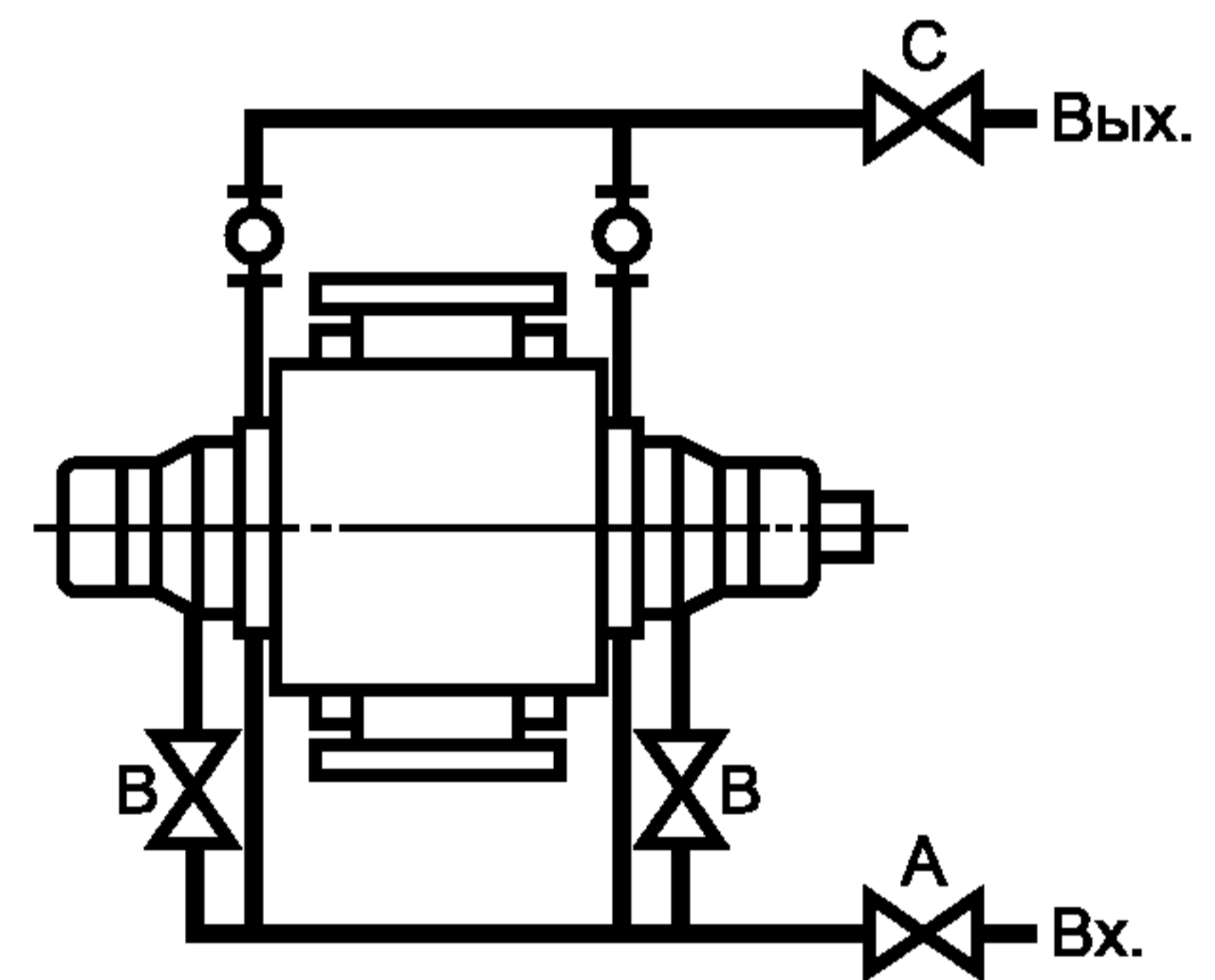
Схема D Охлаждение камеры мягкого сальника с параллельной подачей в крышку уплотнения
