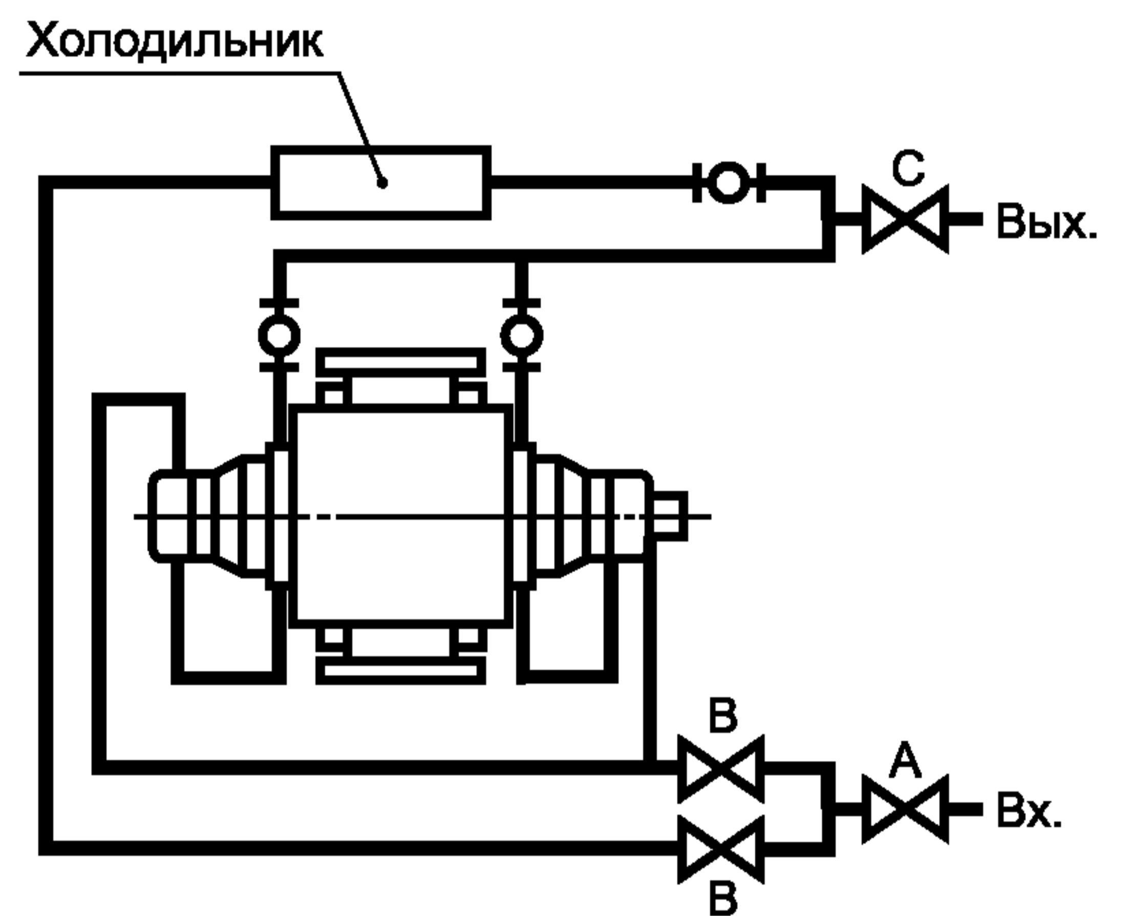
Схема К Последовательное охлаждение камеры мягкого сальника и корпуса подшипника с параллельной подачей в холодильник
