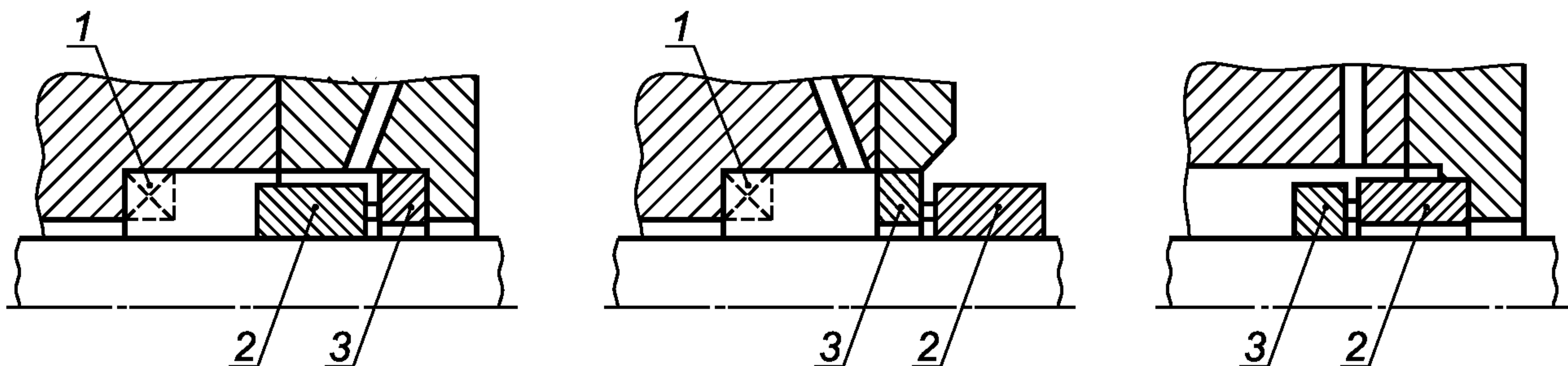
S1 — внутреннее расположение вращающегося подвижного уплотнительного кольца
