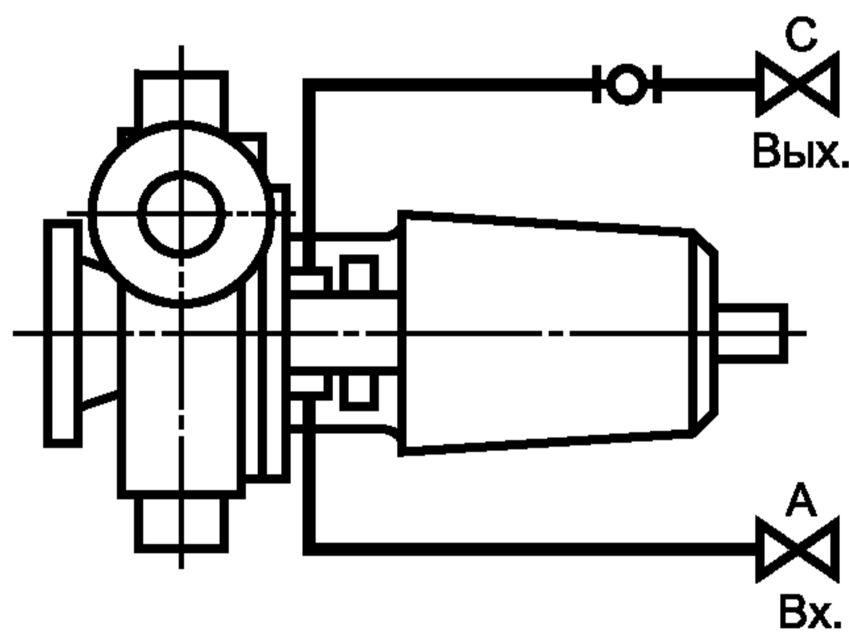
Схема С Охлаждение камеры мягкого сальника
