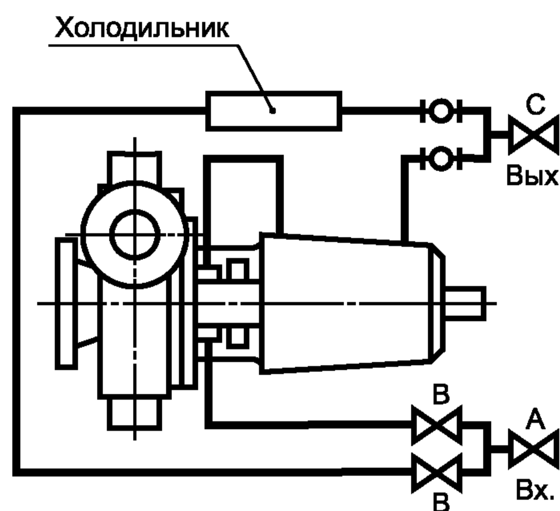
Схема К Последовательное охлаждение камеры мягкого сальника и корпуса подшипника с параллельной подачей в холодильник
