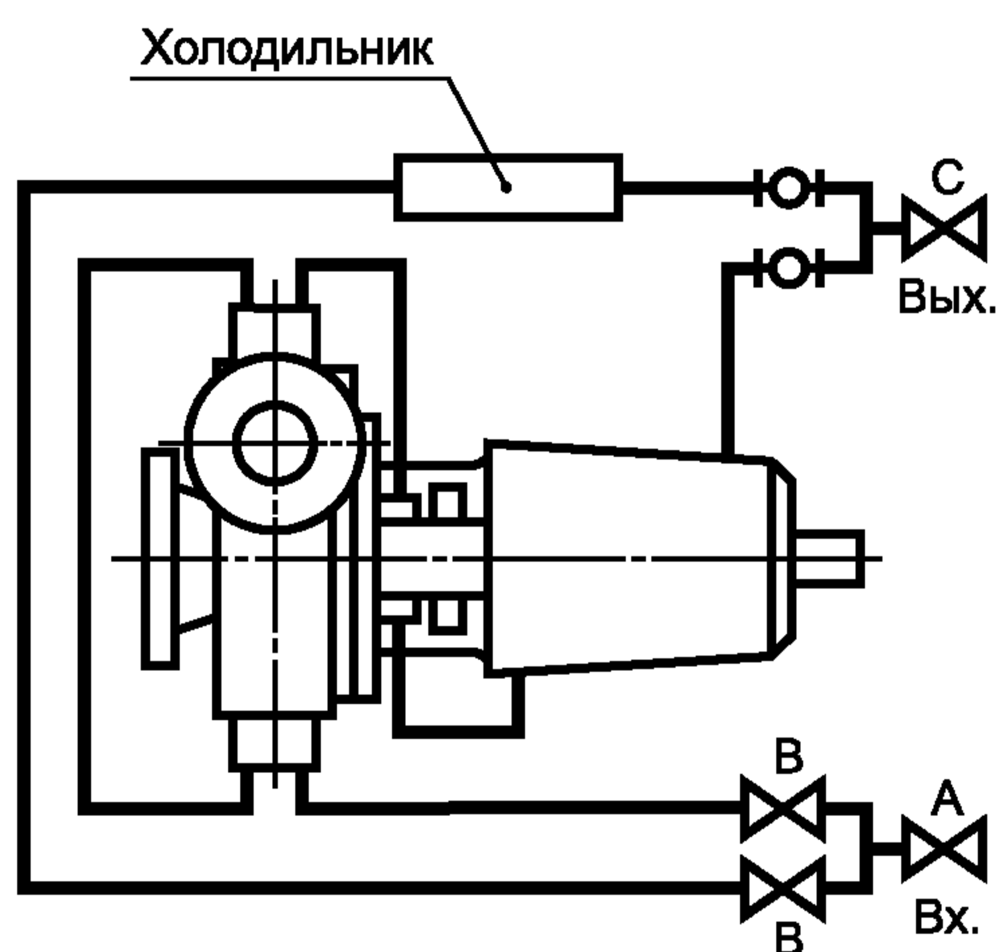
Схема Л Последовательное охлаждение опорных плит, корпуса подшипника и камеры мягкого сальника с параллельной подачей в холодильник
