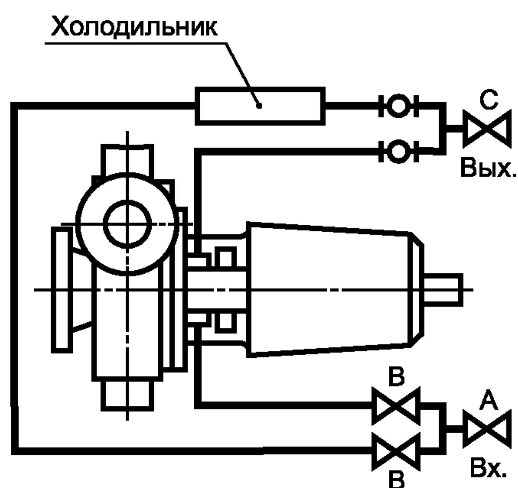
Схема Ж Охлаждение камеры мягкого сальника с параллельной подачей в холодильник
