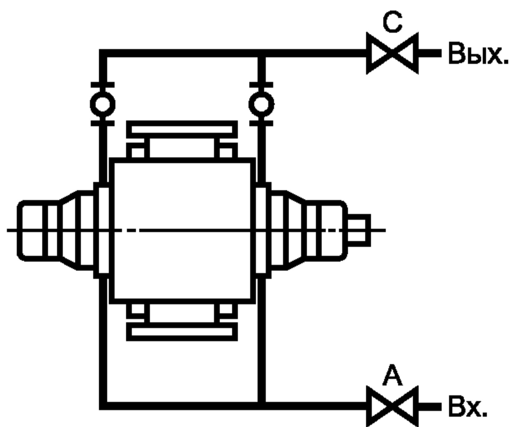
Схема С Охлаждение камеры мягкого сальника
