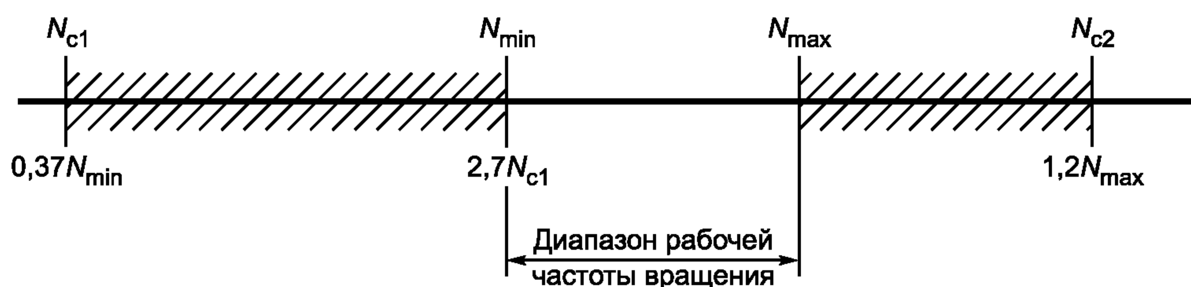
Рисунок 2 — Предельные значения критических частот вращения относительно диапазона рабочих скоростей (см. 4.3.1.3)
