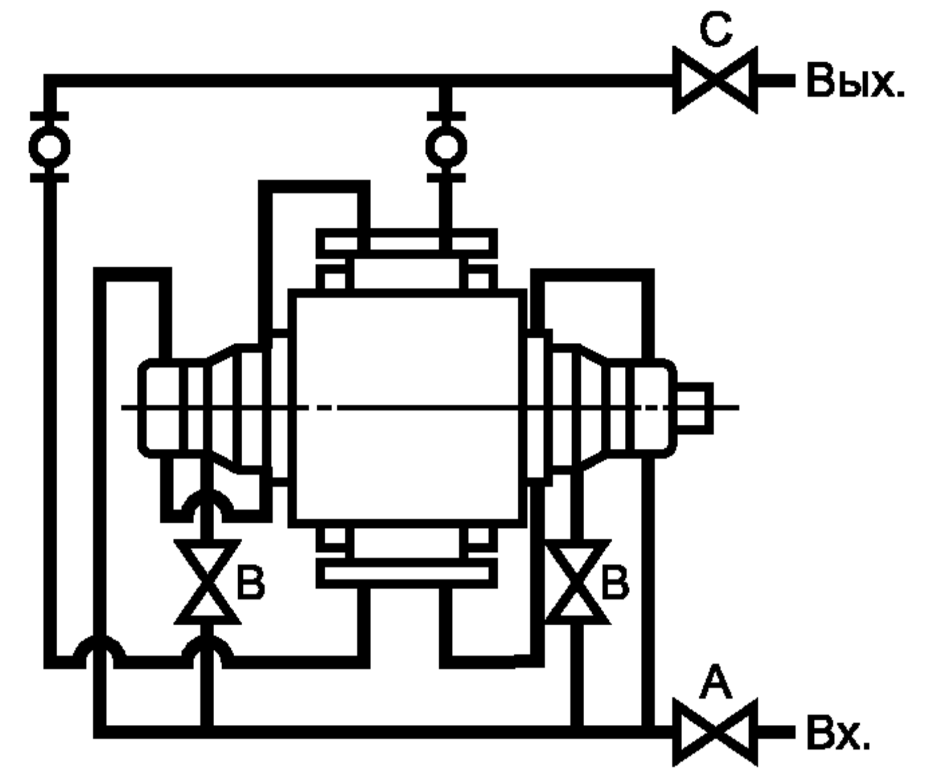
Схема Н Последовательное охлаждение опорных плит, корпуса подшипника и камеры мягкого сальника с параллельной подачей в крышку уплотнения
