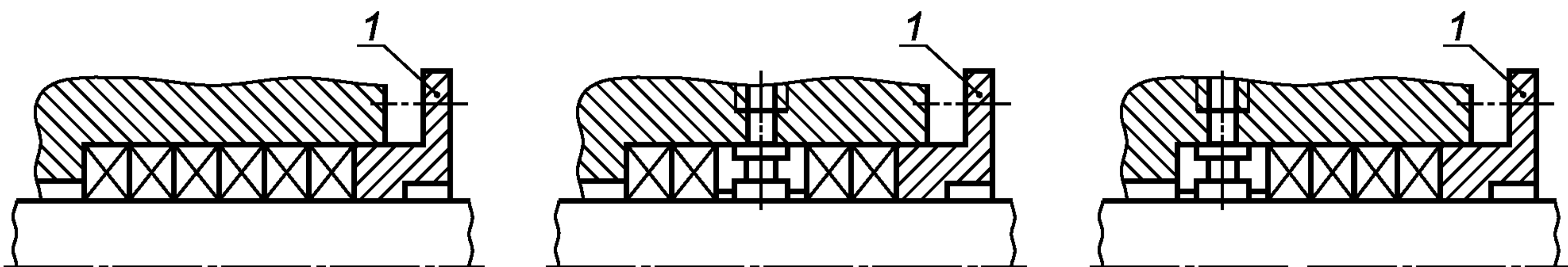
P1 — мягкий сальник (одинарная компоновка)**
