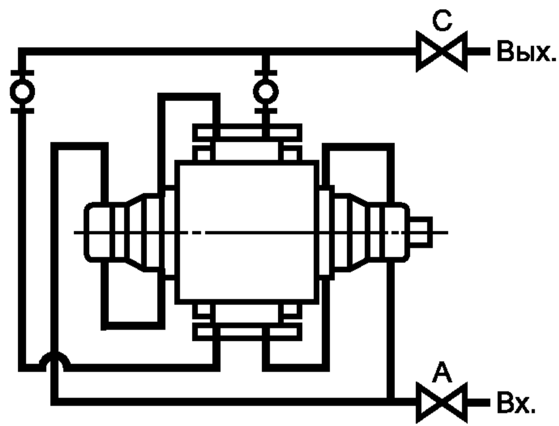
Схема Г Последовательное охлаждение опорных плит, корпуса подшипника и камеры мягкого сальника
