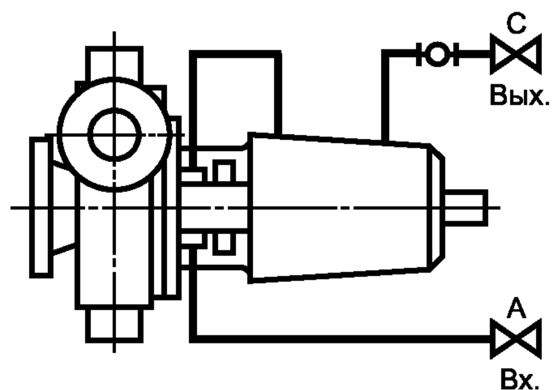
Схема Е Последовательное охлаждение камеры мягкого сальника и корпуса подшипника
