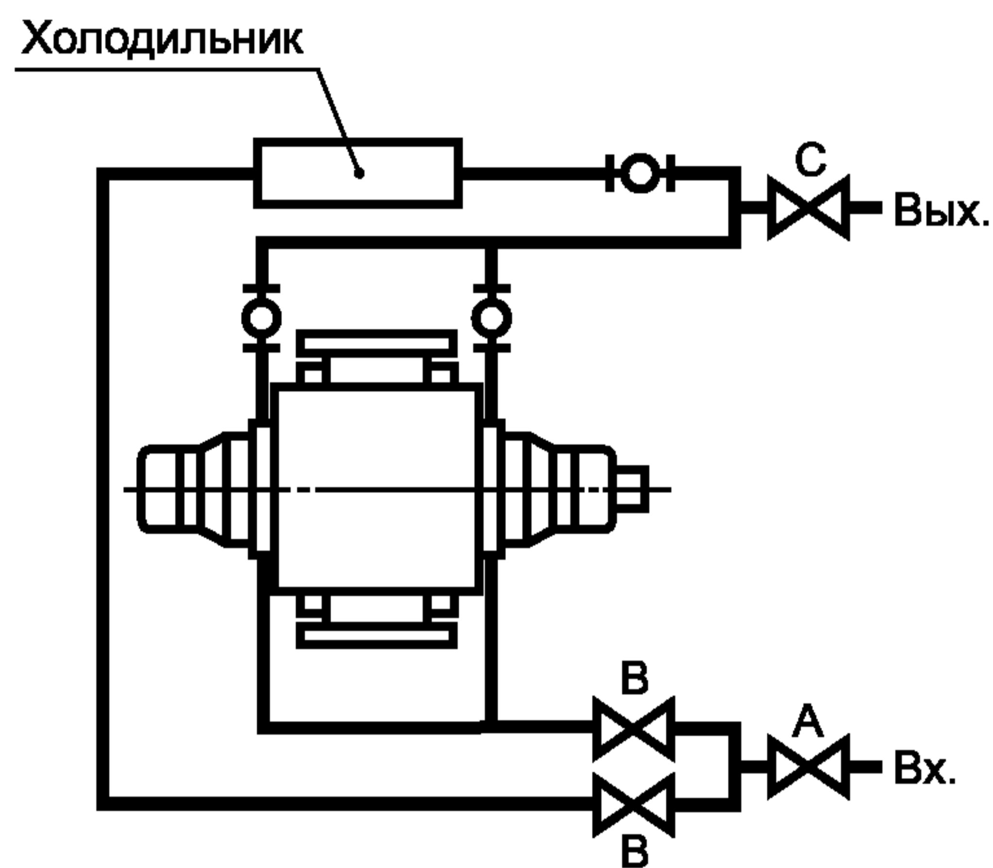
Схема Ж Охлаждение камеры мягкого сальника с параллельной подачей в холодильник
