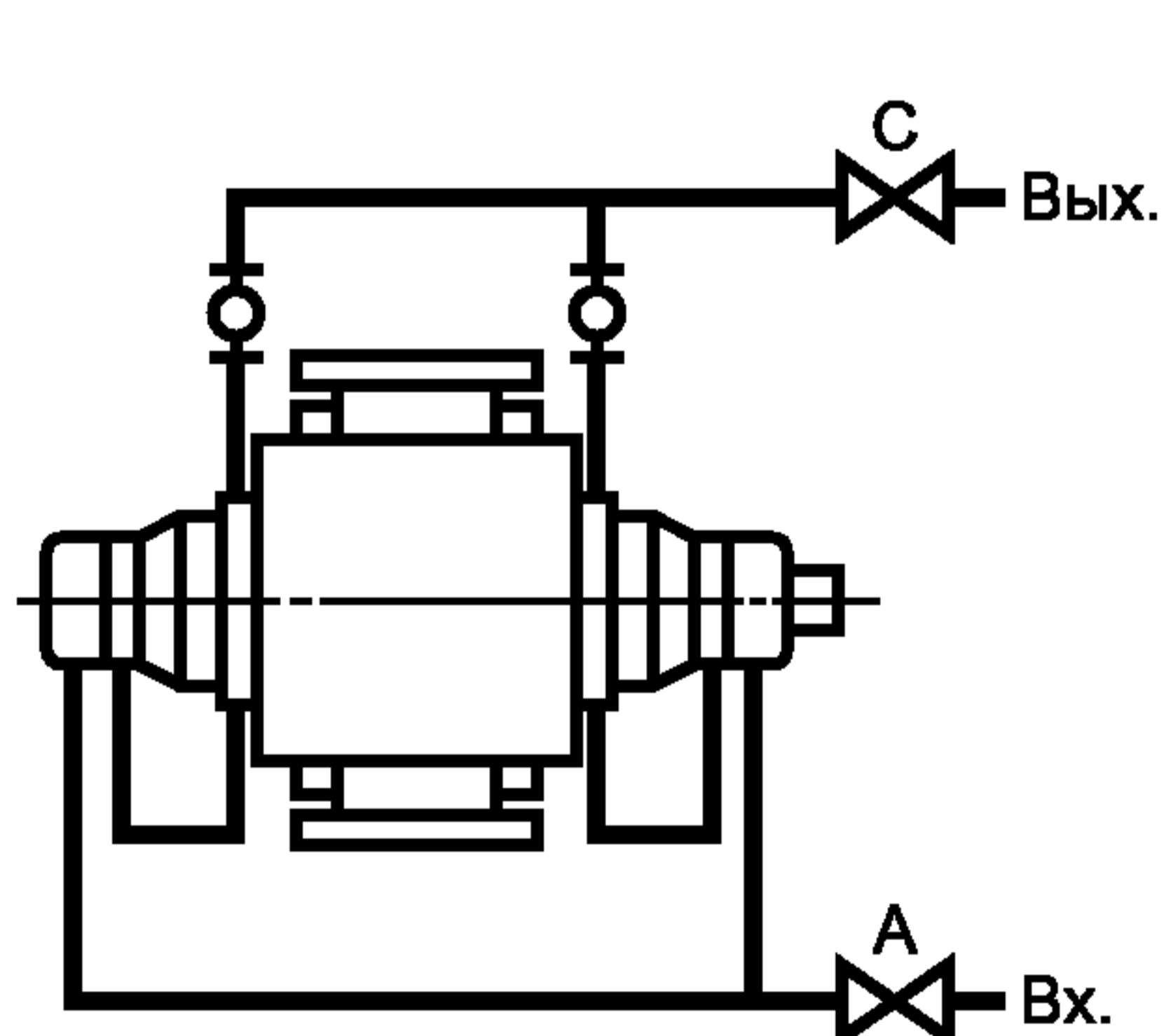
Схема Е Последовательное охлаждение камеры мягкого сальника и корпуса подшипника
