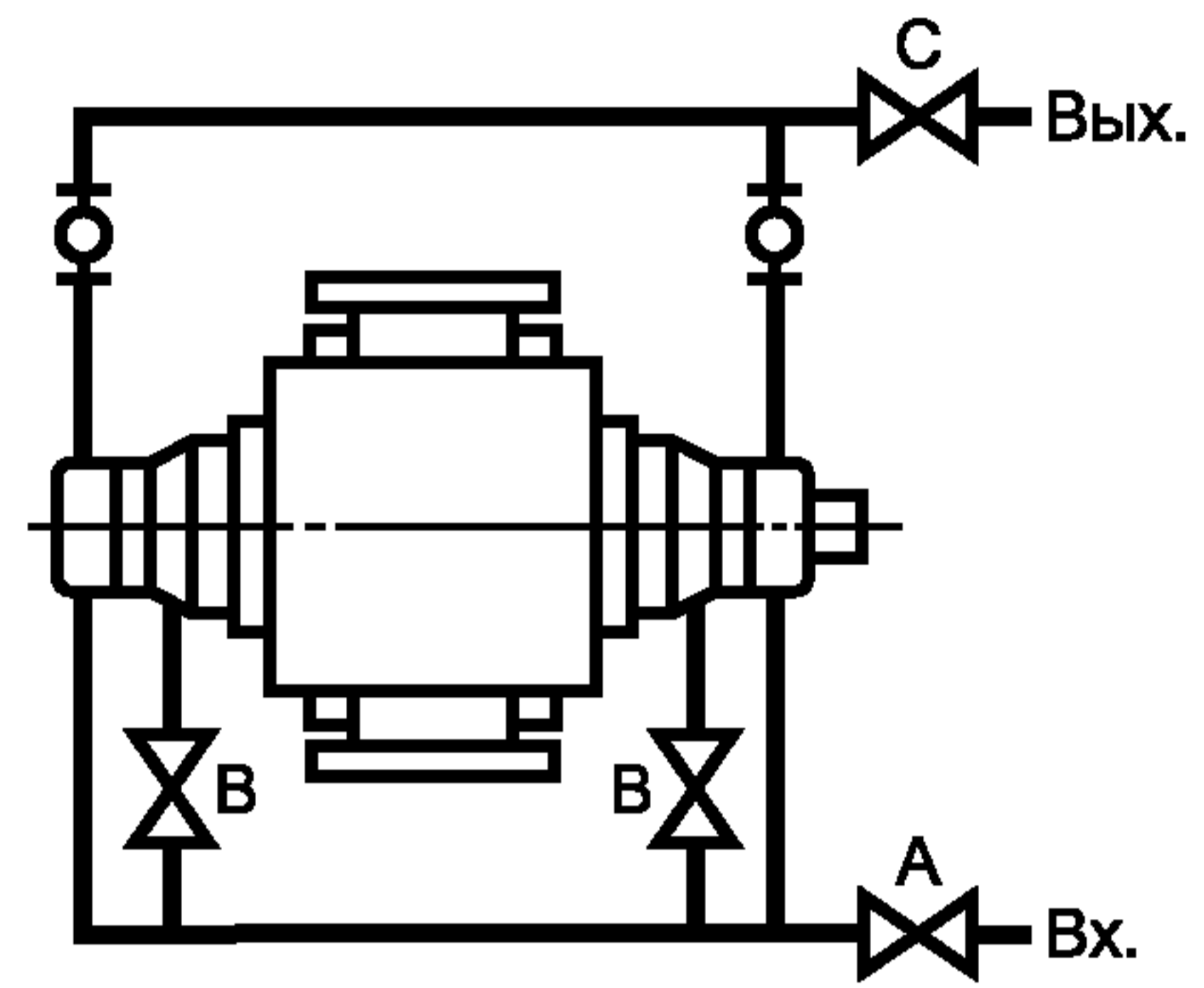
Схема В Охлаждение корпуса подшипника с параллельной подачей в крышку уплотнения
