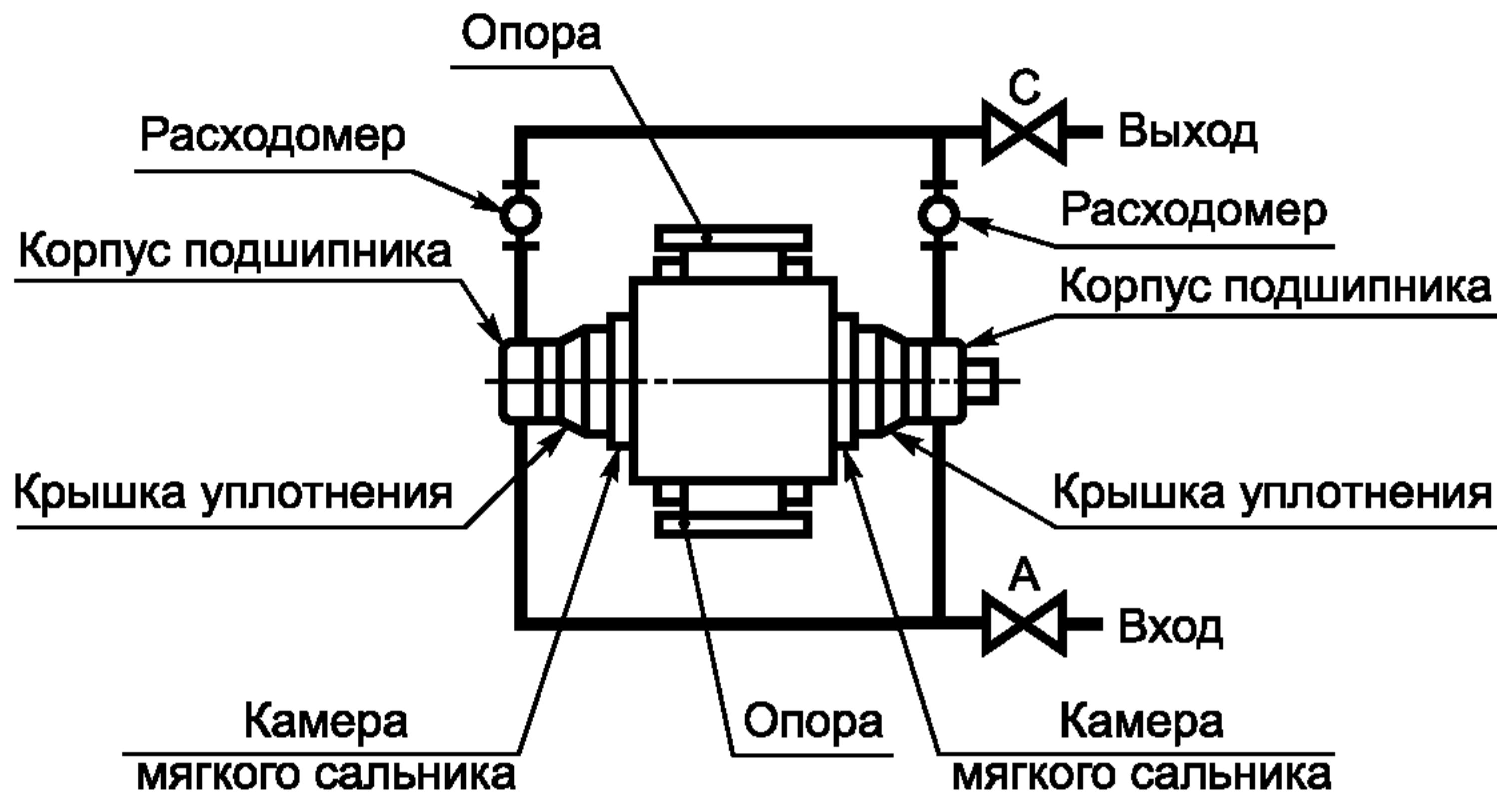
Схема А Охлаждение корпуса подшипника
