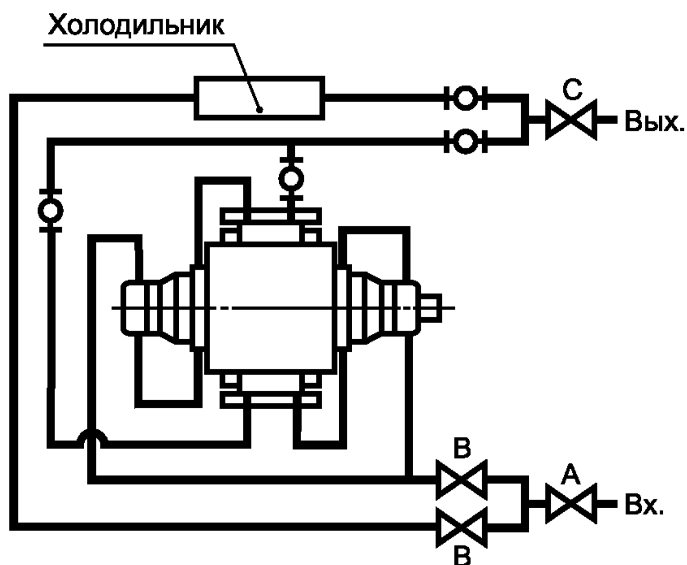
Схема Л Последовательное охлаждение опорных плит, корпуса подшипника и камеры мягкого сальника с параллельной подачей в холодильник
