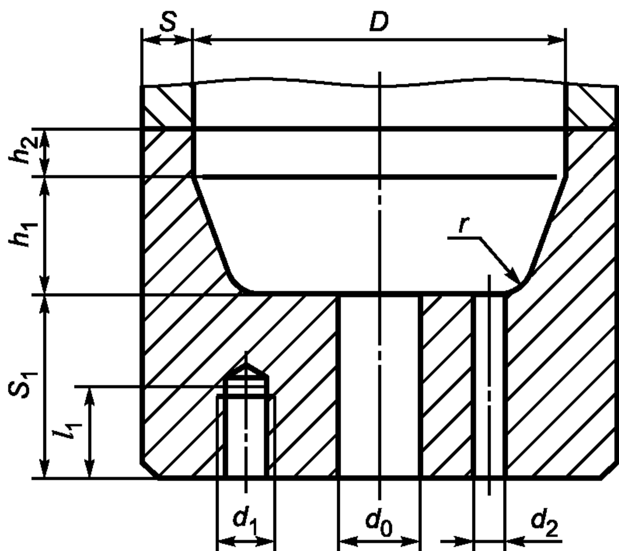
Рисунок 6.1 — Плоское днище с коническим переходом
