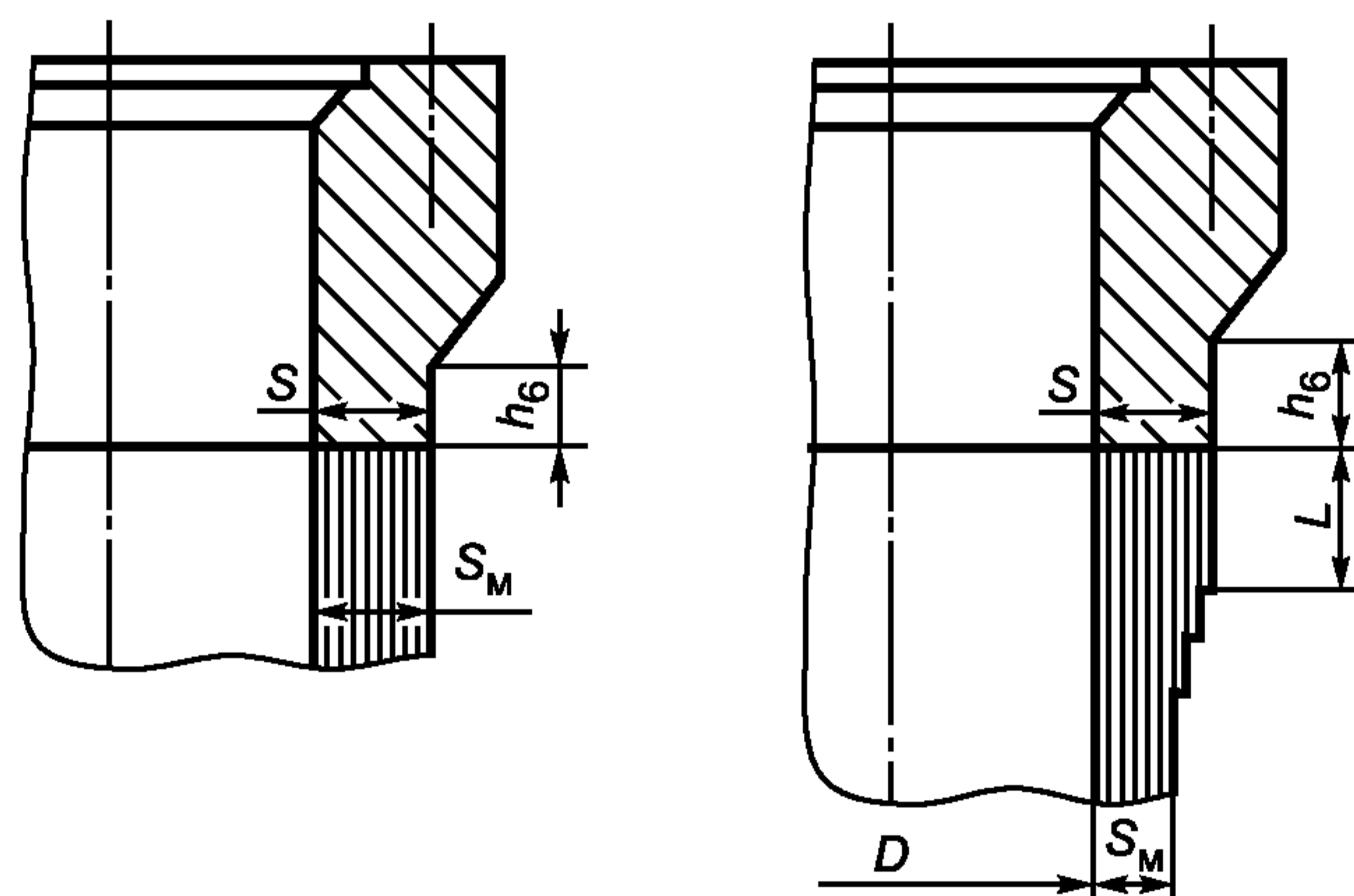
Рисунок 7.2 — Кованый фланец, сопряженный с многослойной обечайкой
