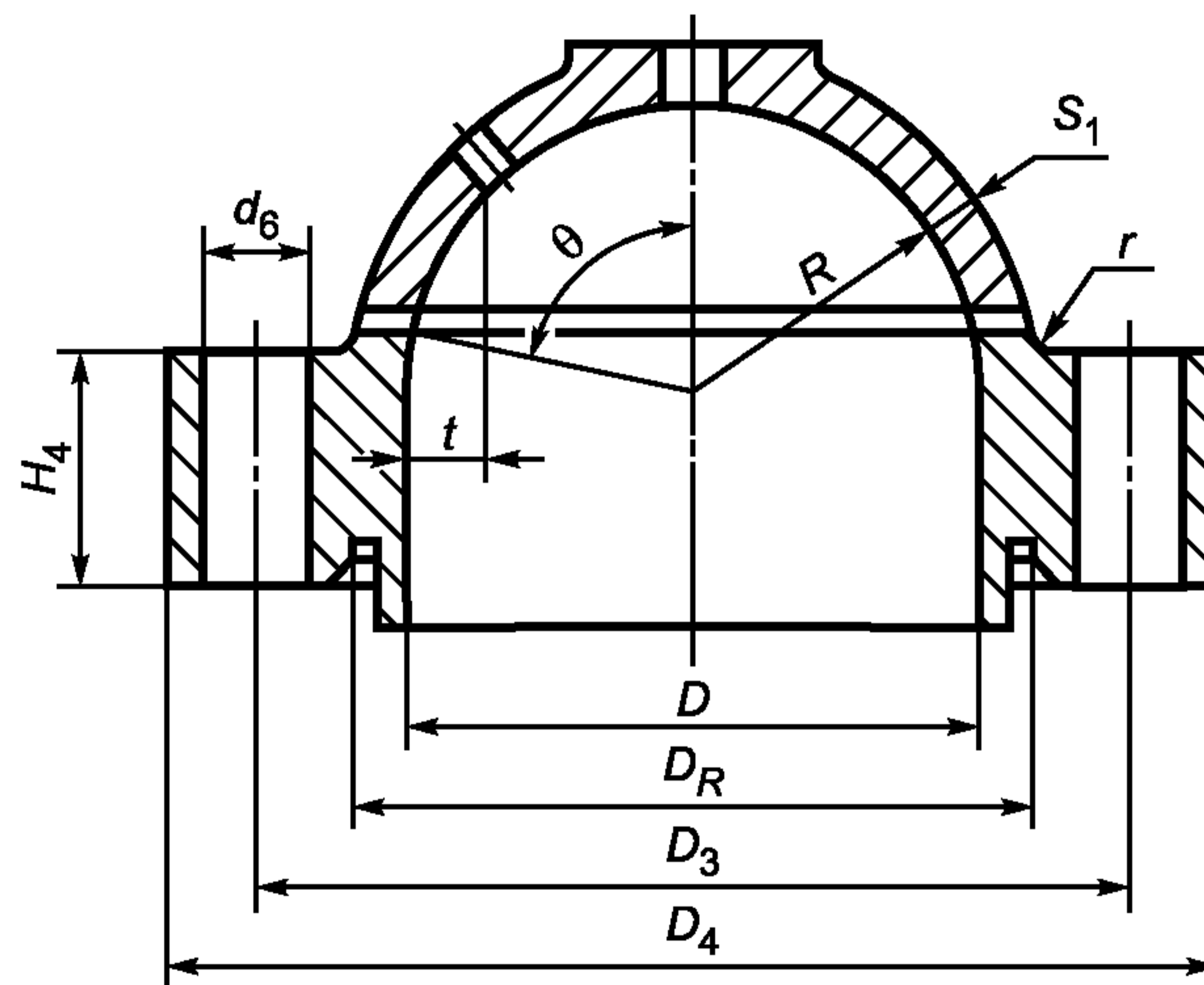
Рисунок 8.2 — Схема конструкции выпуклой крышки
