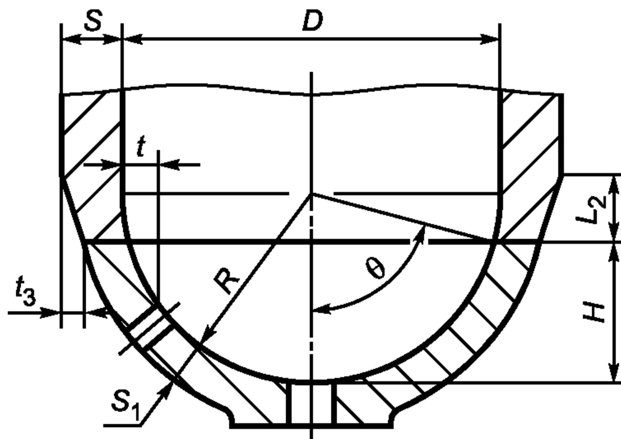
Рисунок 6.5 — Сферическое днище
