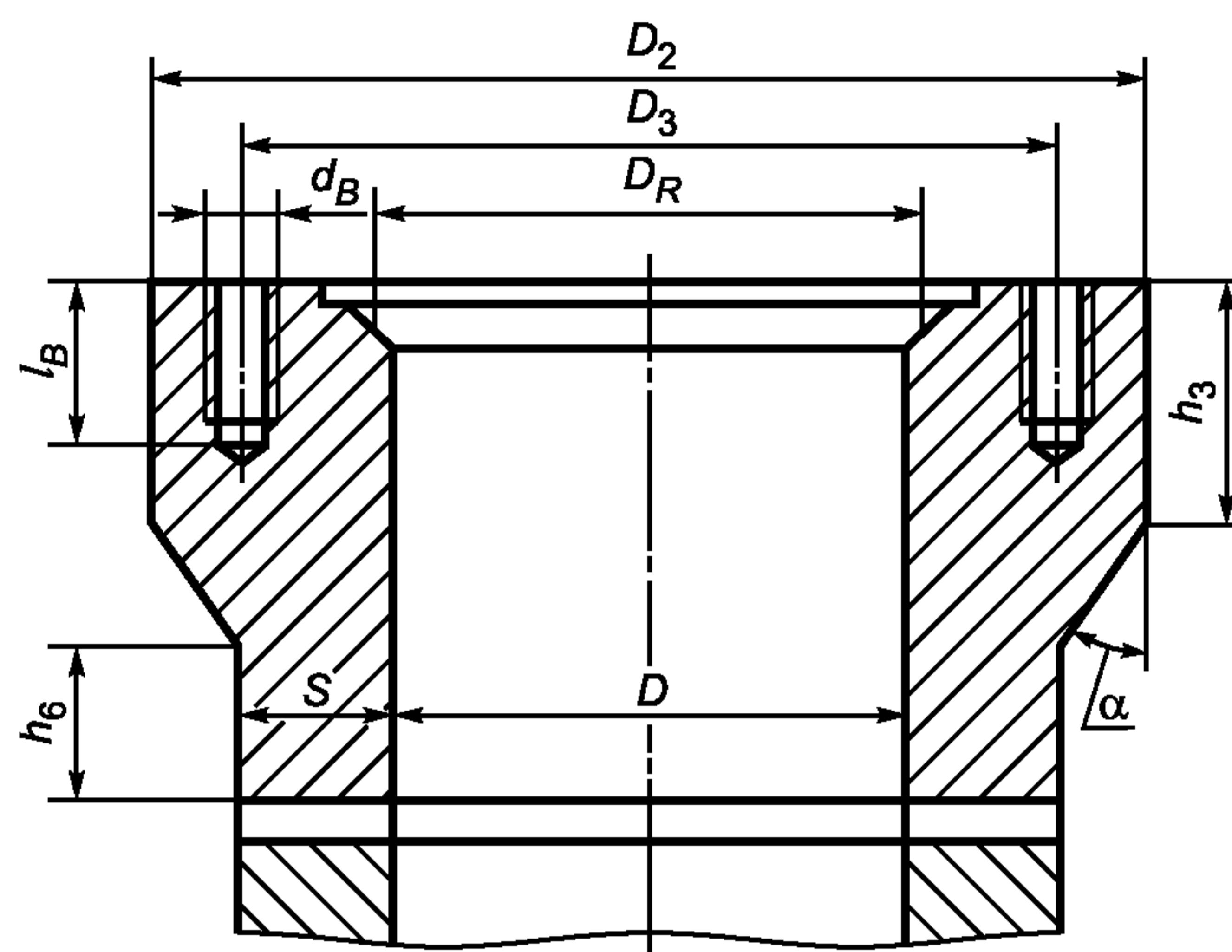
Рисунок 7.1 — Кованый фланец
