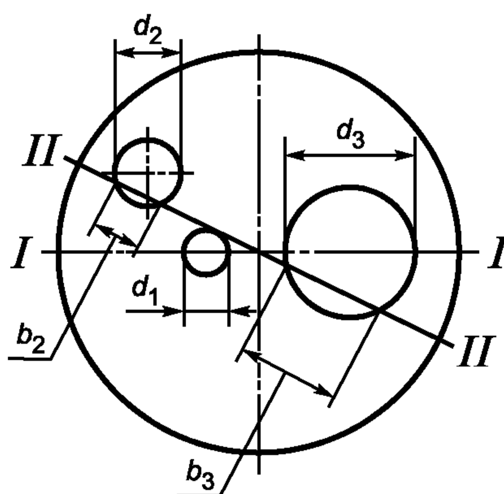
Рисунок 6.4 — Наиболее ослабленные диаметральные сечения днища
