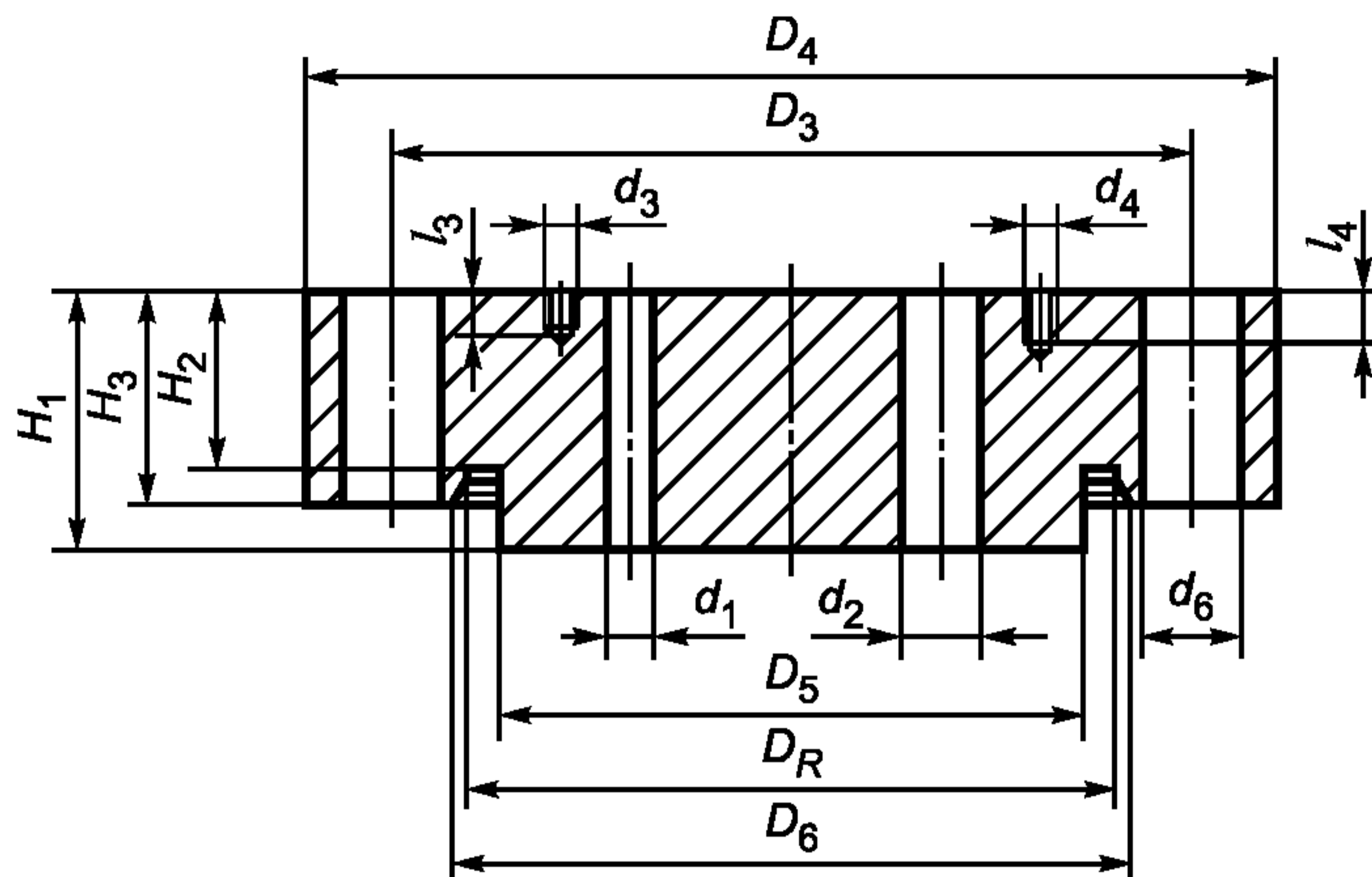
Рисунок 8.1 — Схема плоской крышки
