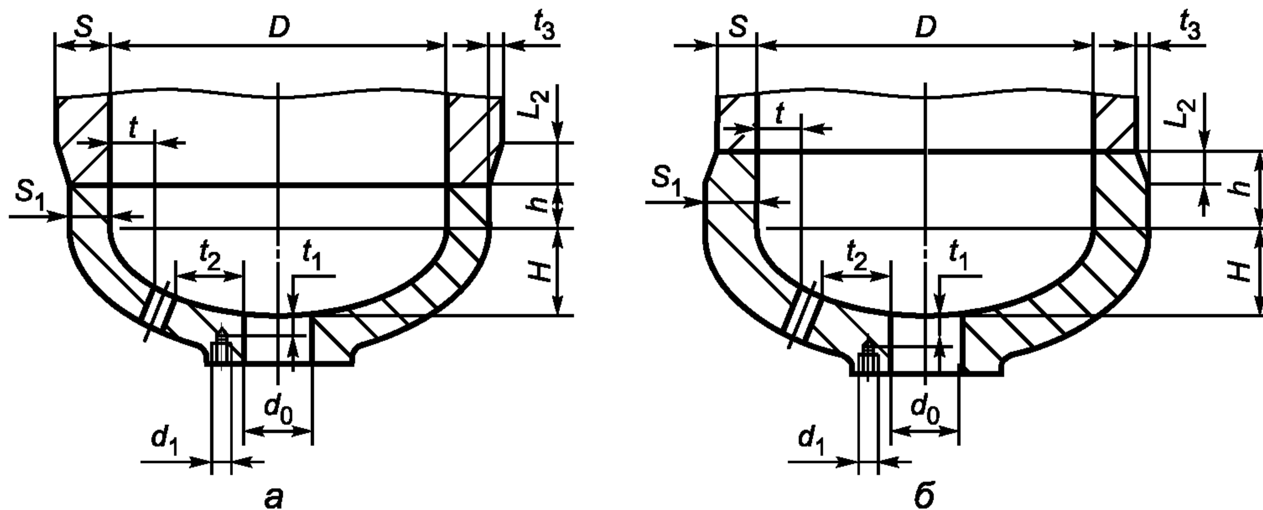
Рисунок 6.6 — Эллиптическое днище
