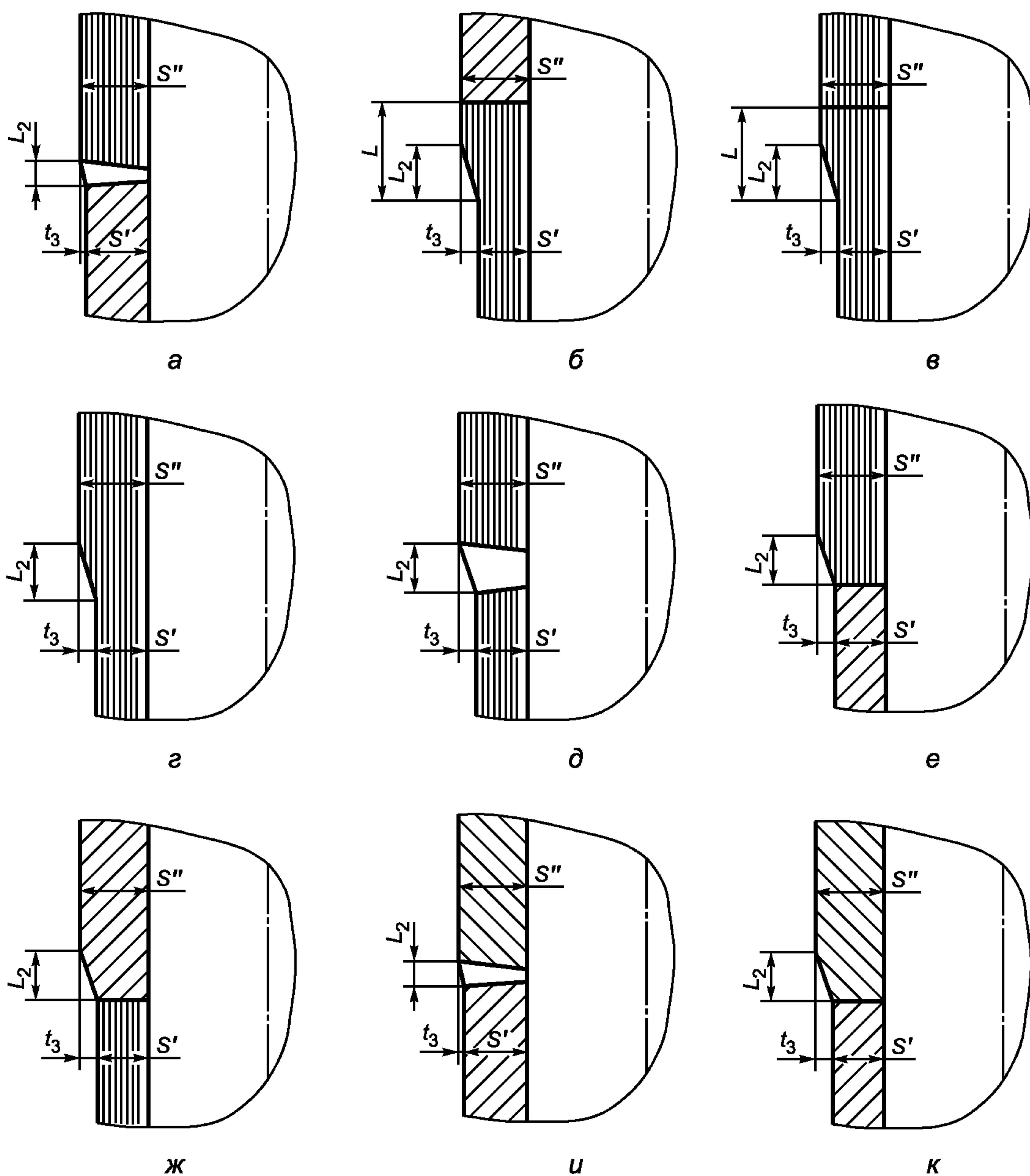
Рисунок 5.1 — Соединение цилиндрических обечаек
