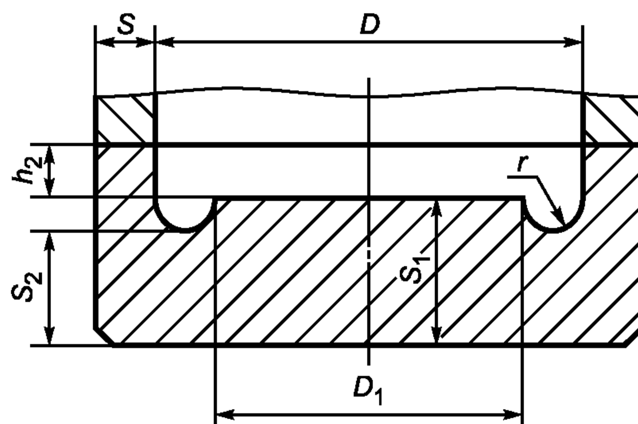
Рисунок 6.3 — Плоское днище с проточкой
