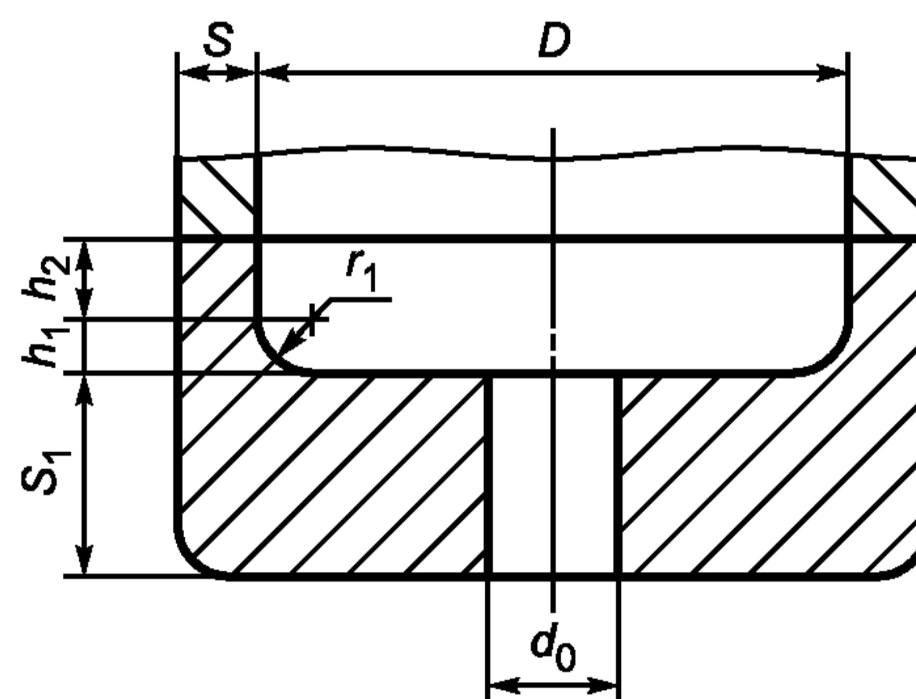
Рисунок 6.2 — Плоское днище с радиусным переходом
