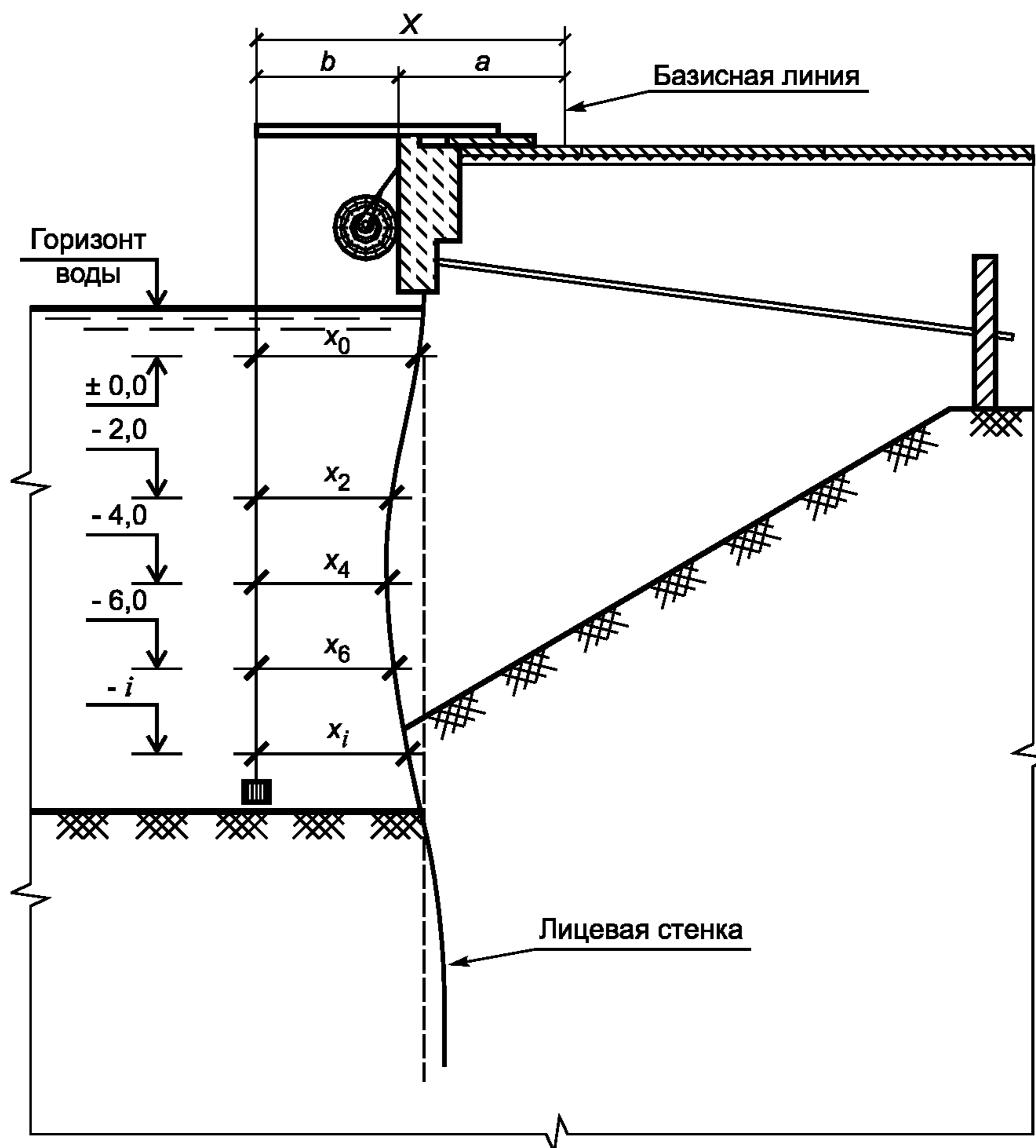
Рисунок 8.1 — Схема измерений наклона (прогиба) лицевой стенки сооружения
