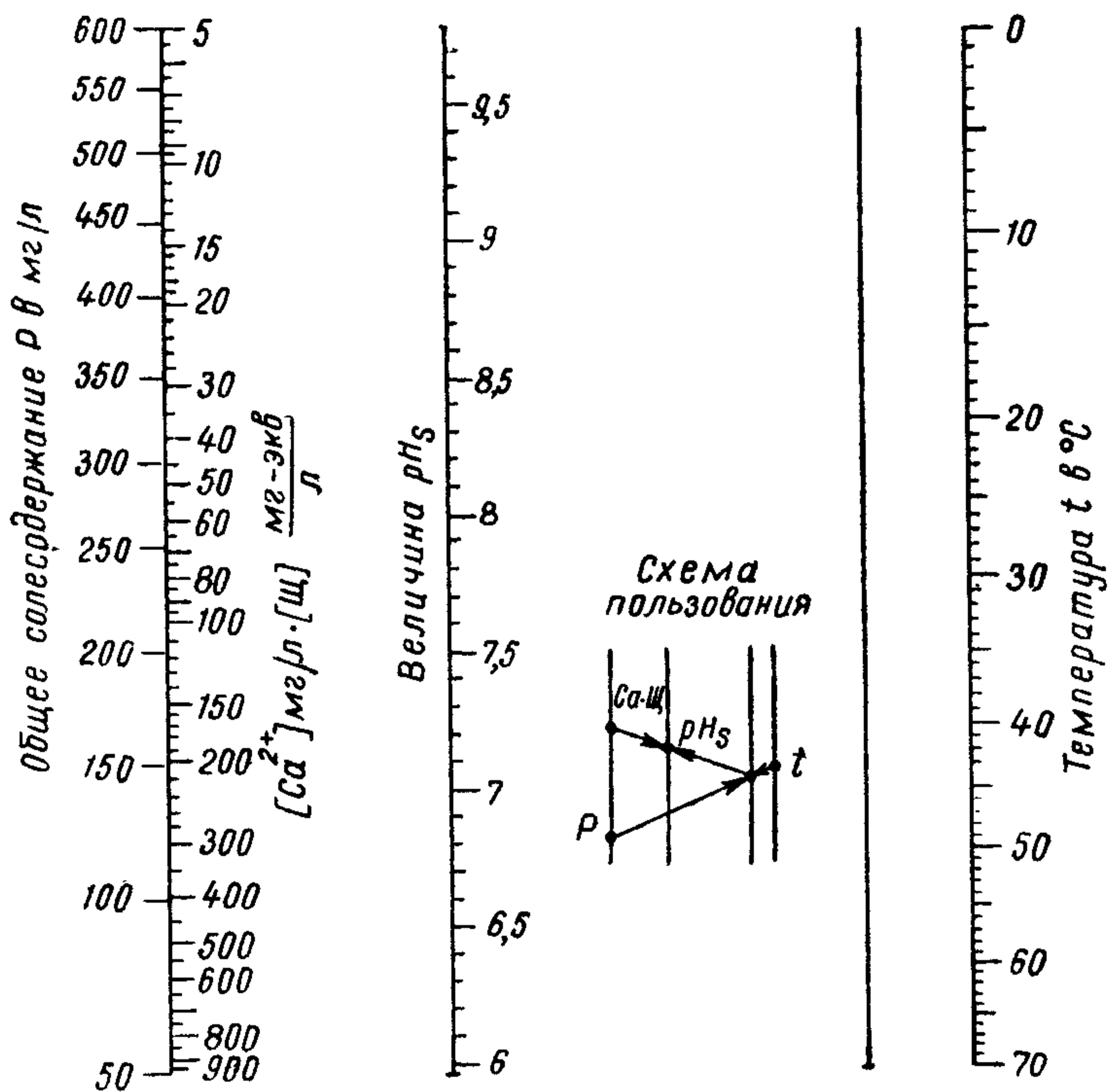
Рис. 1. Номограмма для определения величины pH_s
