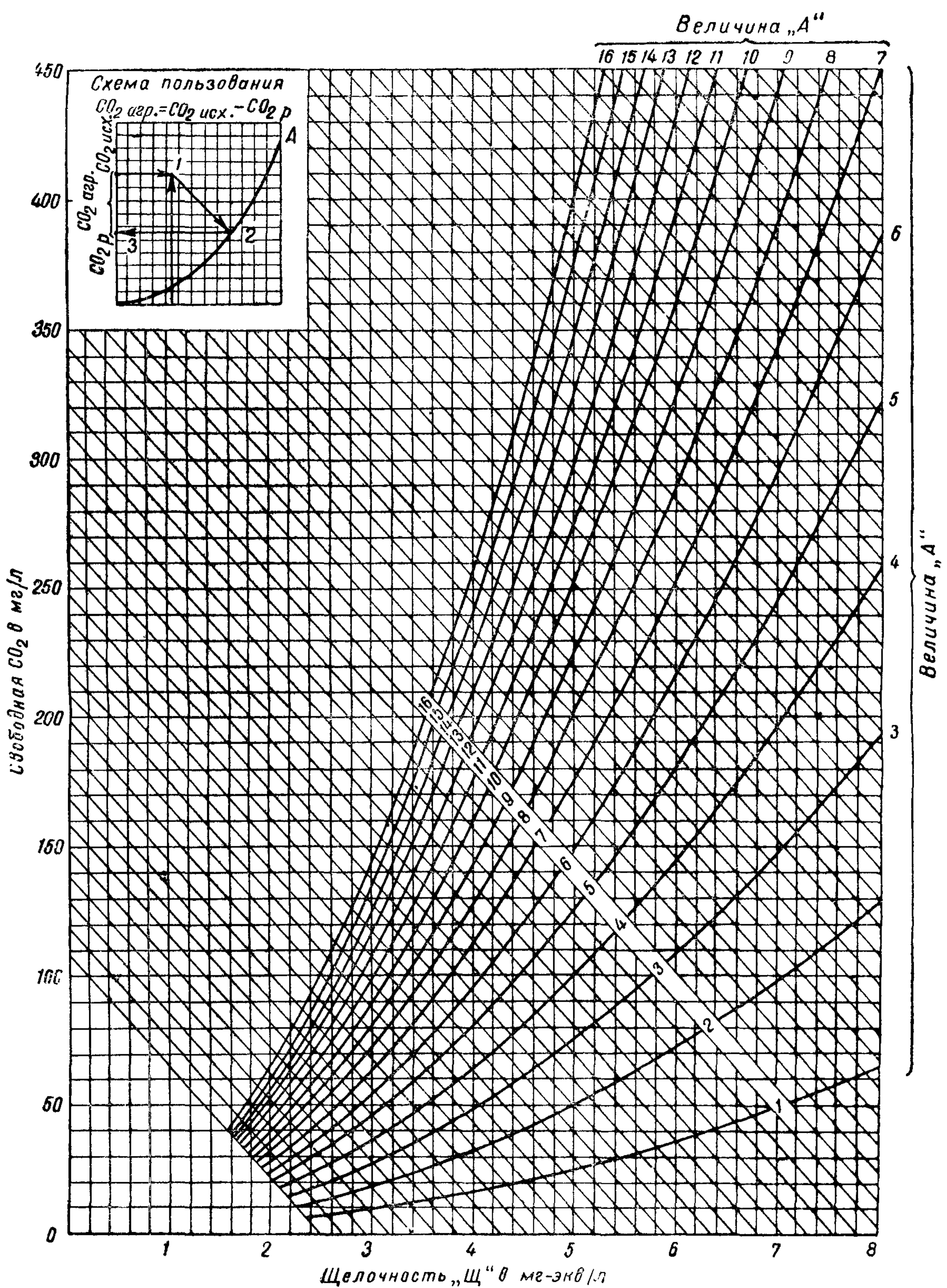
Рис. 7. Помограмма для определения концентрации агрессивной углекислоты в воде (от 0 до 450 мг/л)
