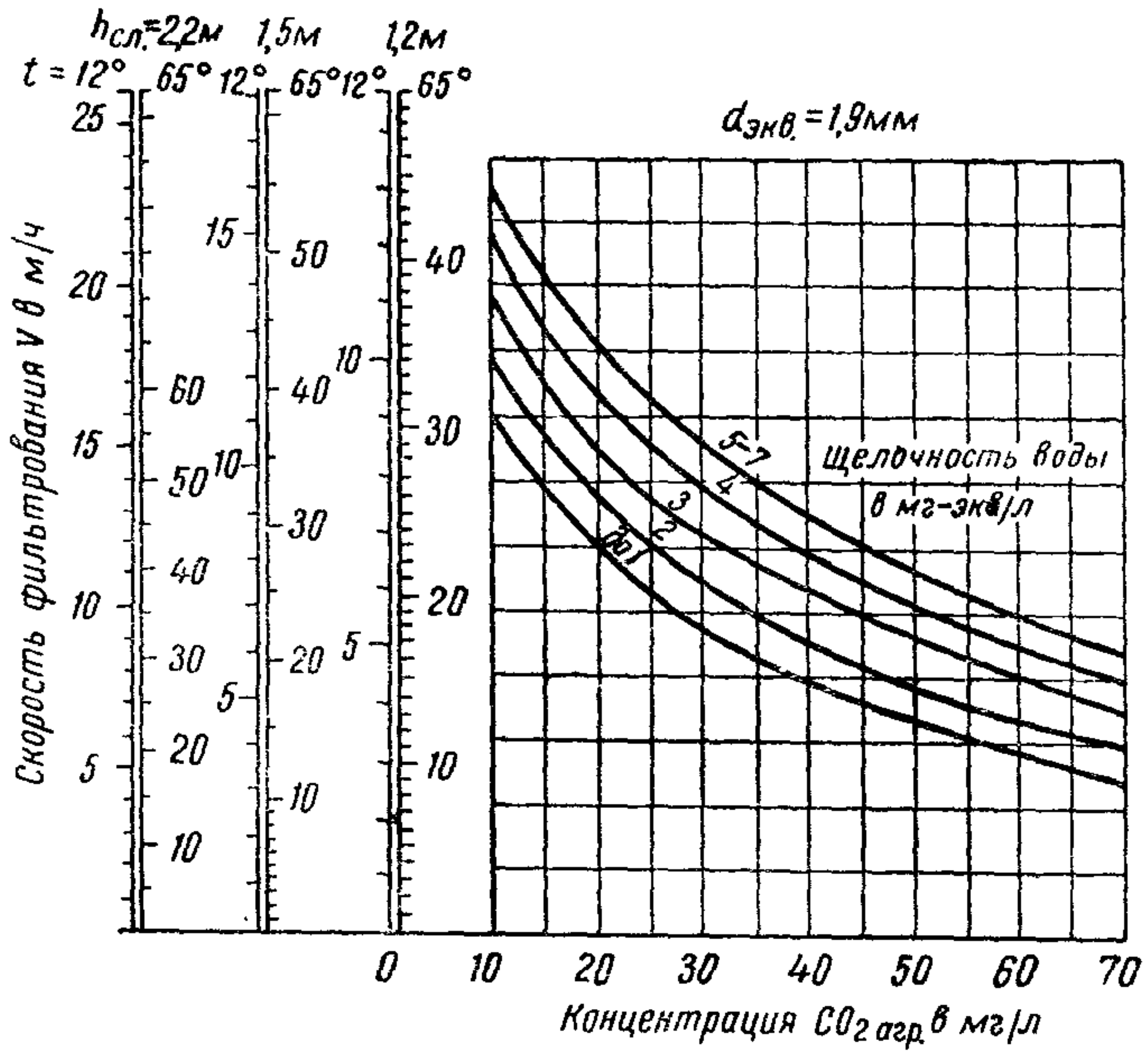
Рис. 4. График для определения скорости фильтрования воды в магномассовых фильтрах
