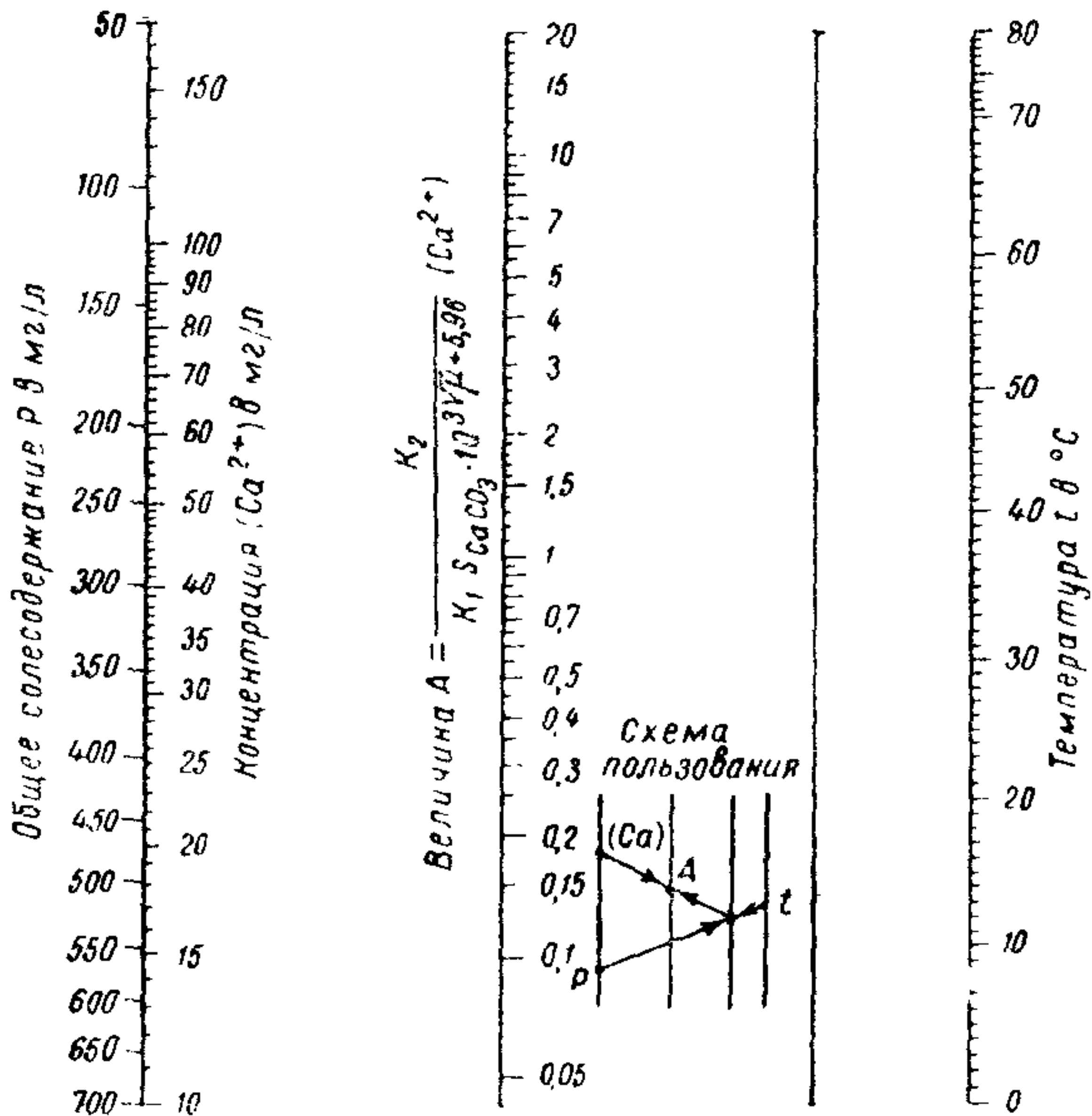
Рис. 5. Номограмма для определения величины «А»
