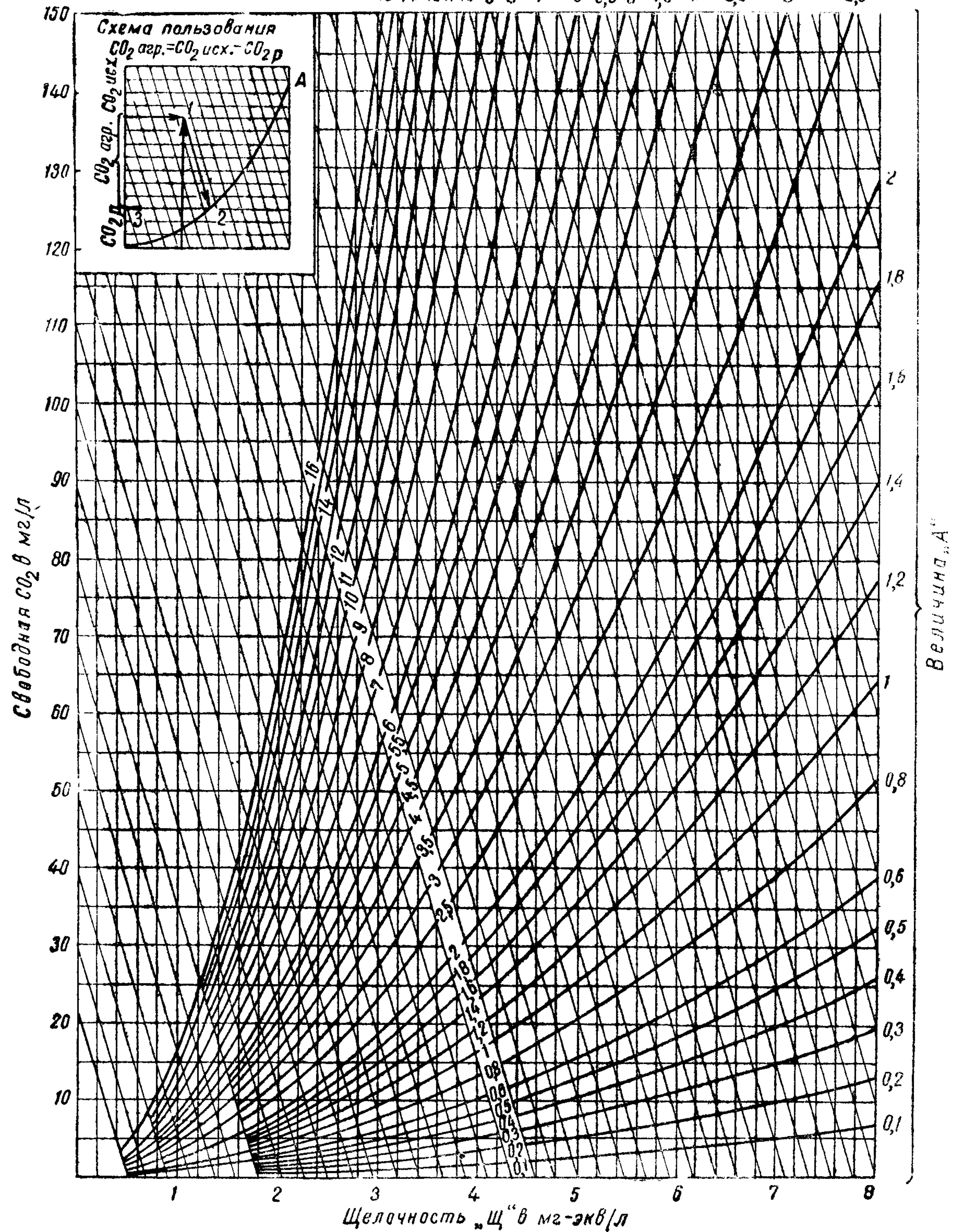
Рис. 6. Номограмма для определения концентрации агрессивной углекислоты в воде (от 0 до 150 мг/л)
