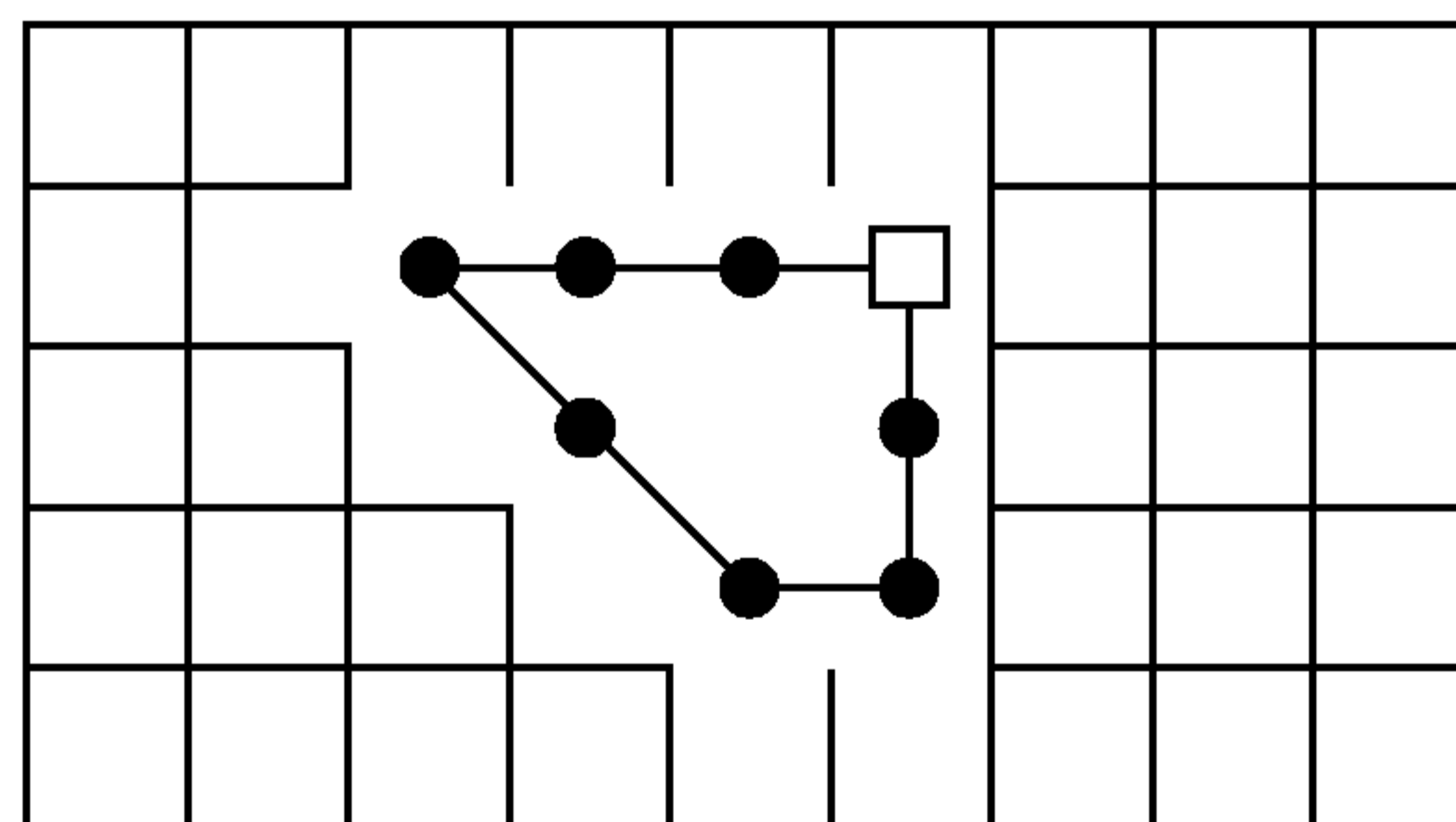
а) 8-связный ЦКФ внутренней границы = «4», «4», «4», «7», «7», «0», «2», «2»
