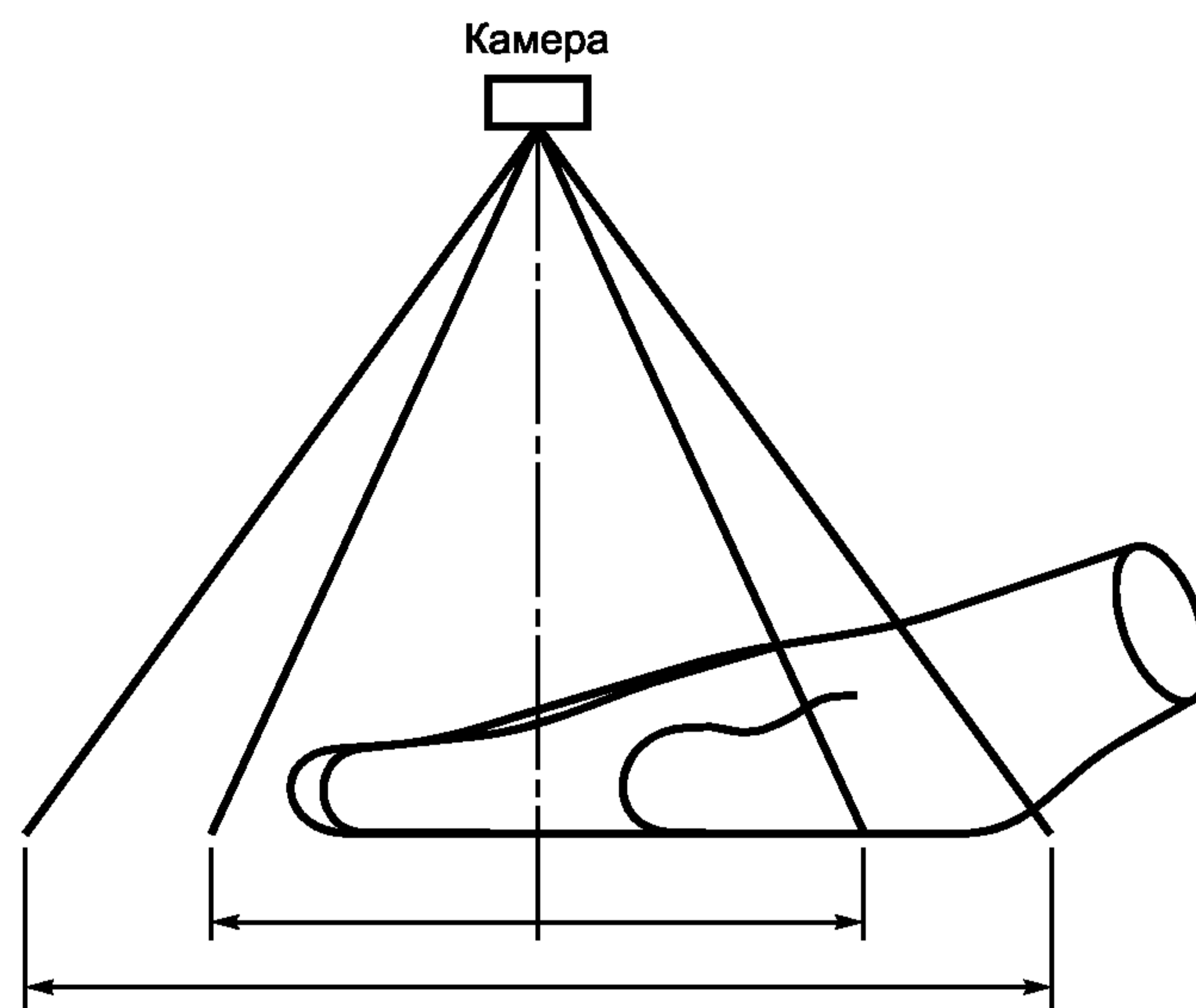
Рисунок 6 — Область интереса для измерения оптического искажения
