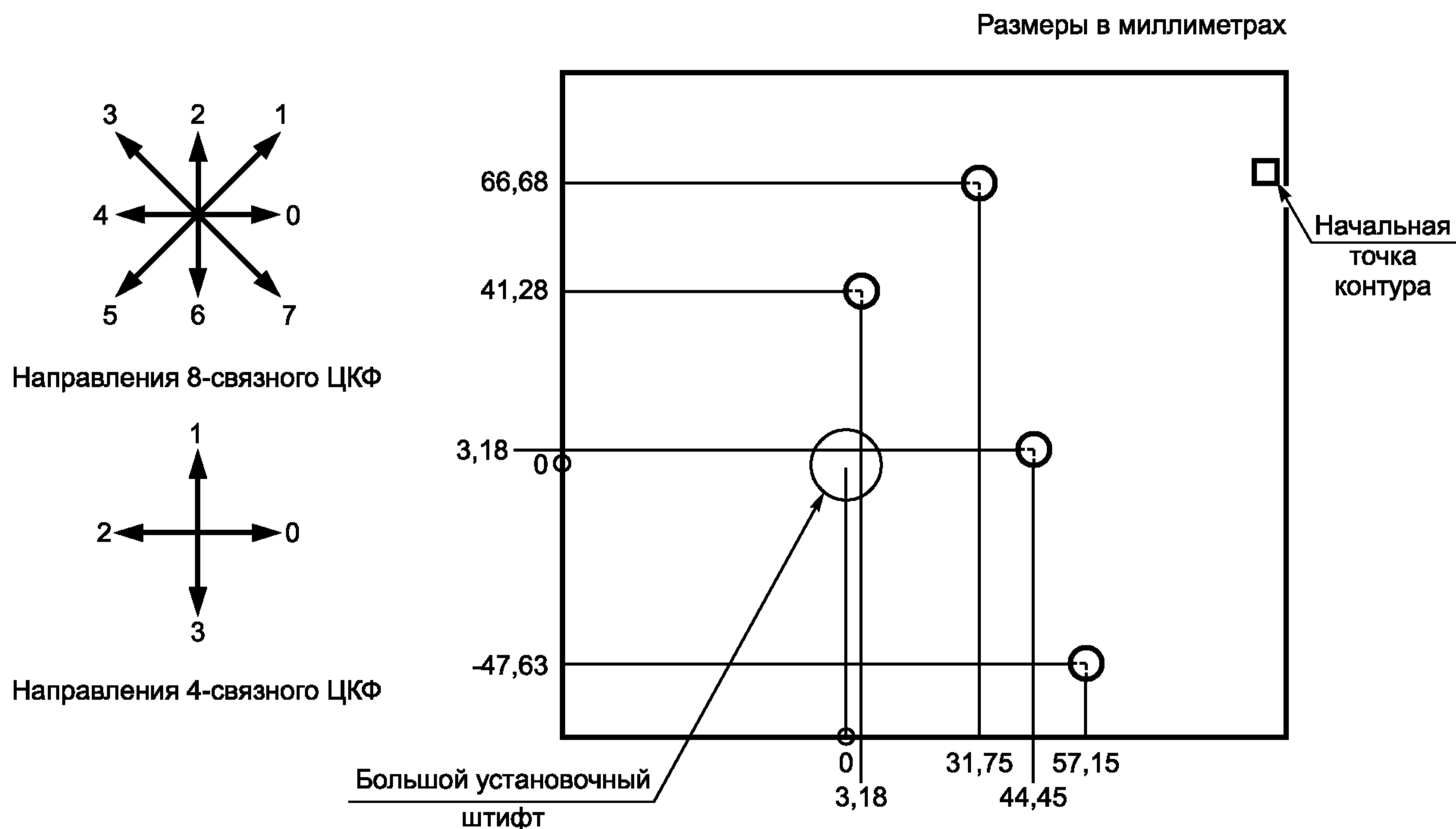
Рисунок В.1 — Примерное расположение установочных штифтов
