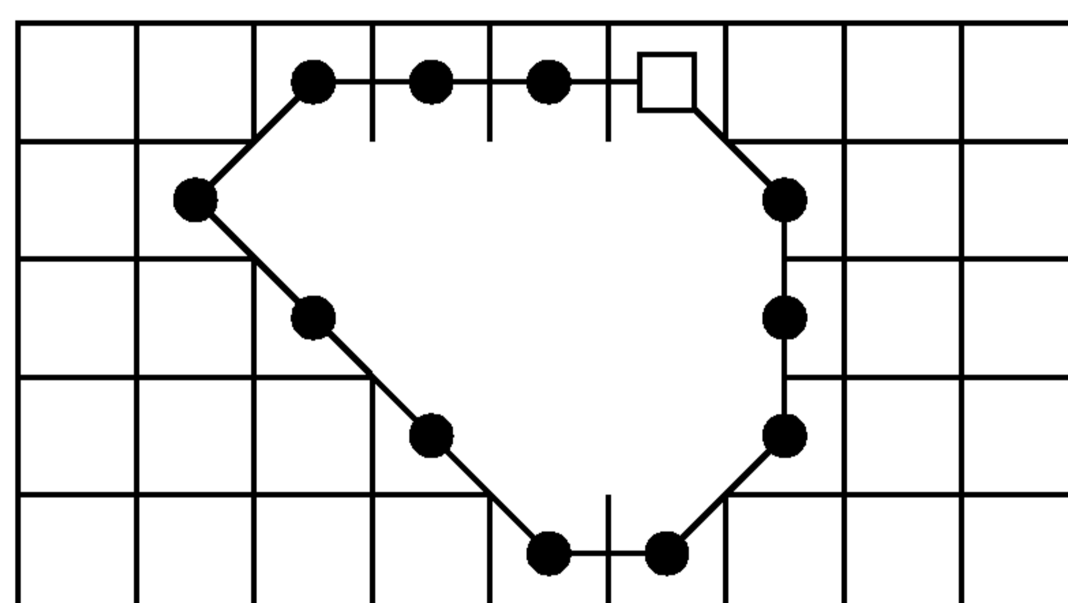
б) 8-связный ЦКФ внешней границы = «4», «4», «4», «5», «7», «7», «7», «0», «1», «2», «2», «3»
