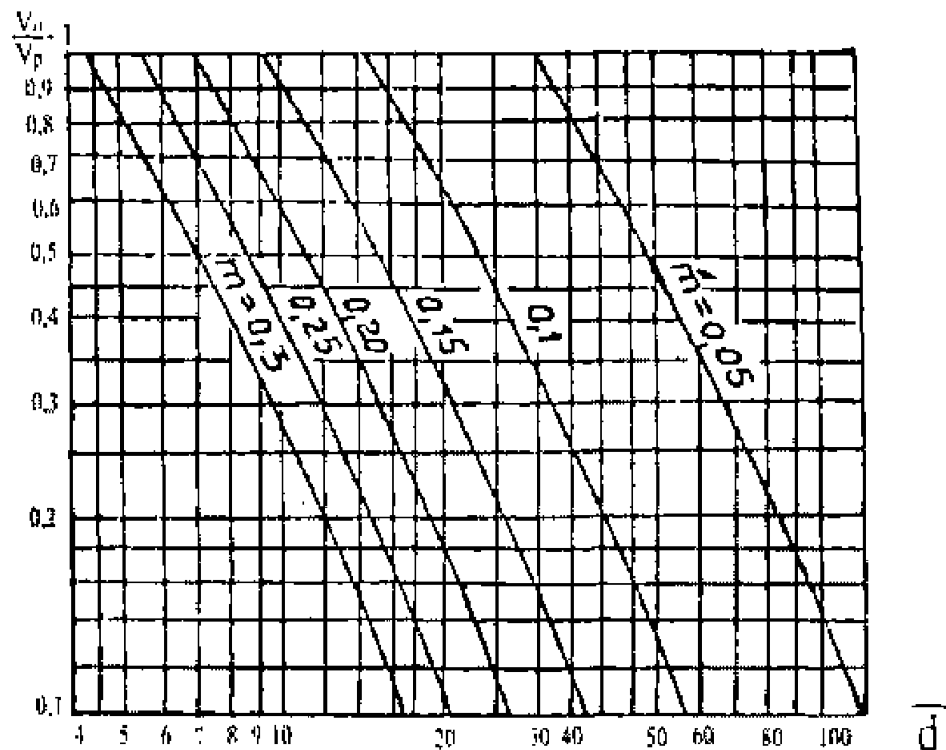
Рисунок 1 – Номограмма для определения диаметра несжатой струи \bar{d} = \frac{d}{d_0}
