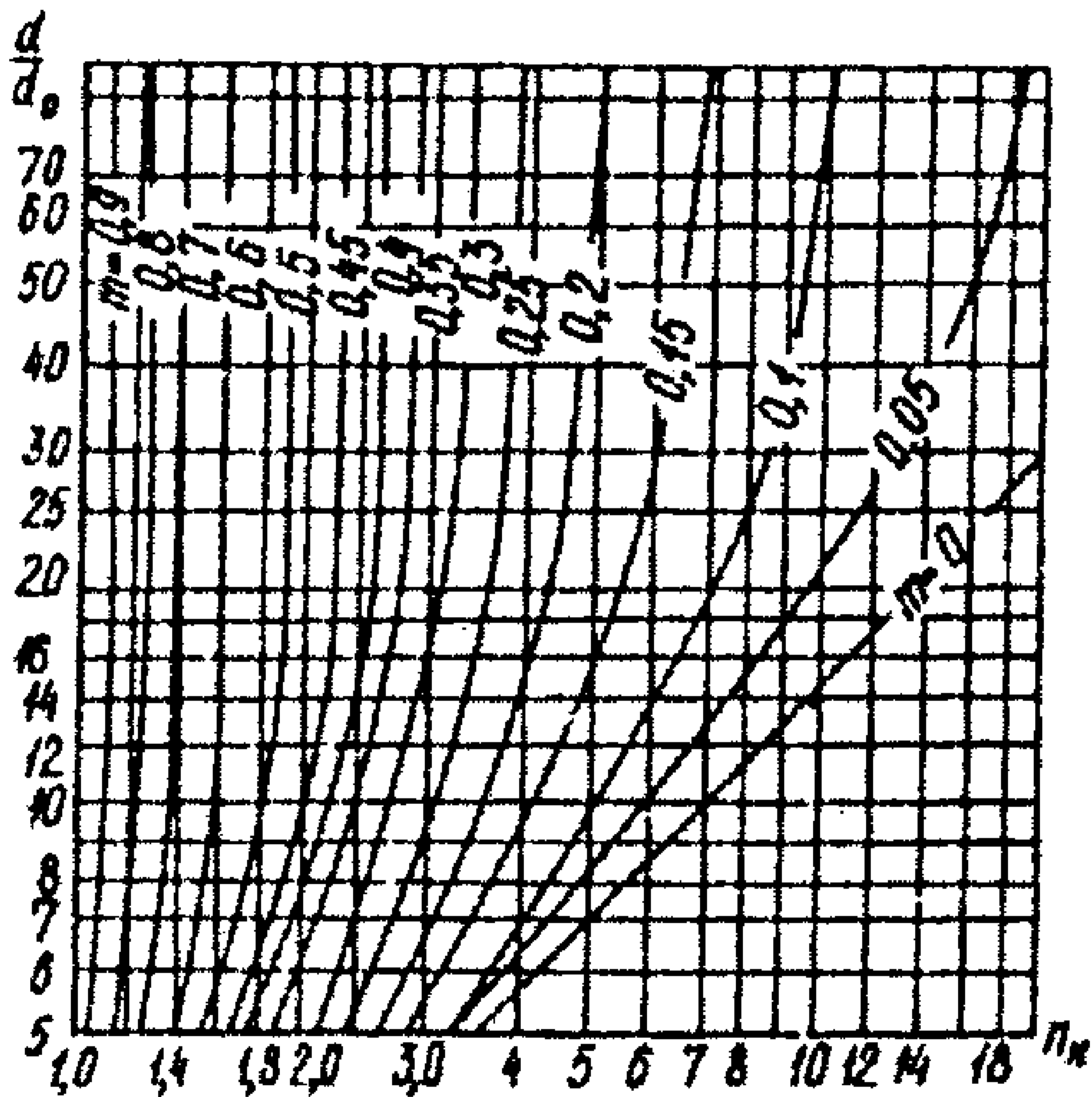
Рисунок 2 – Номограмма для определения начального разбавления в потоке
