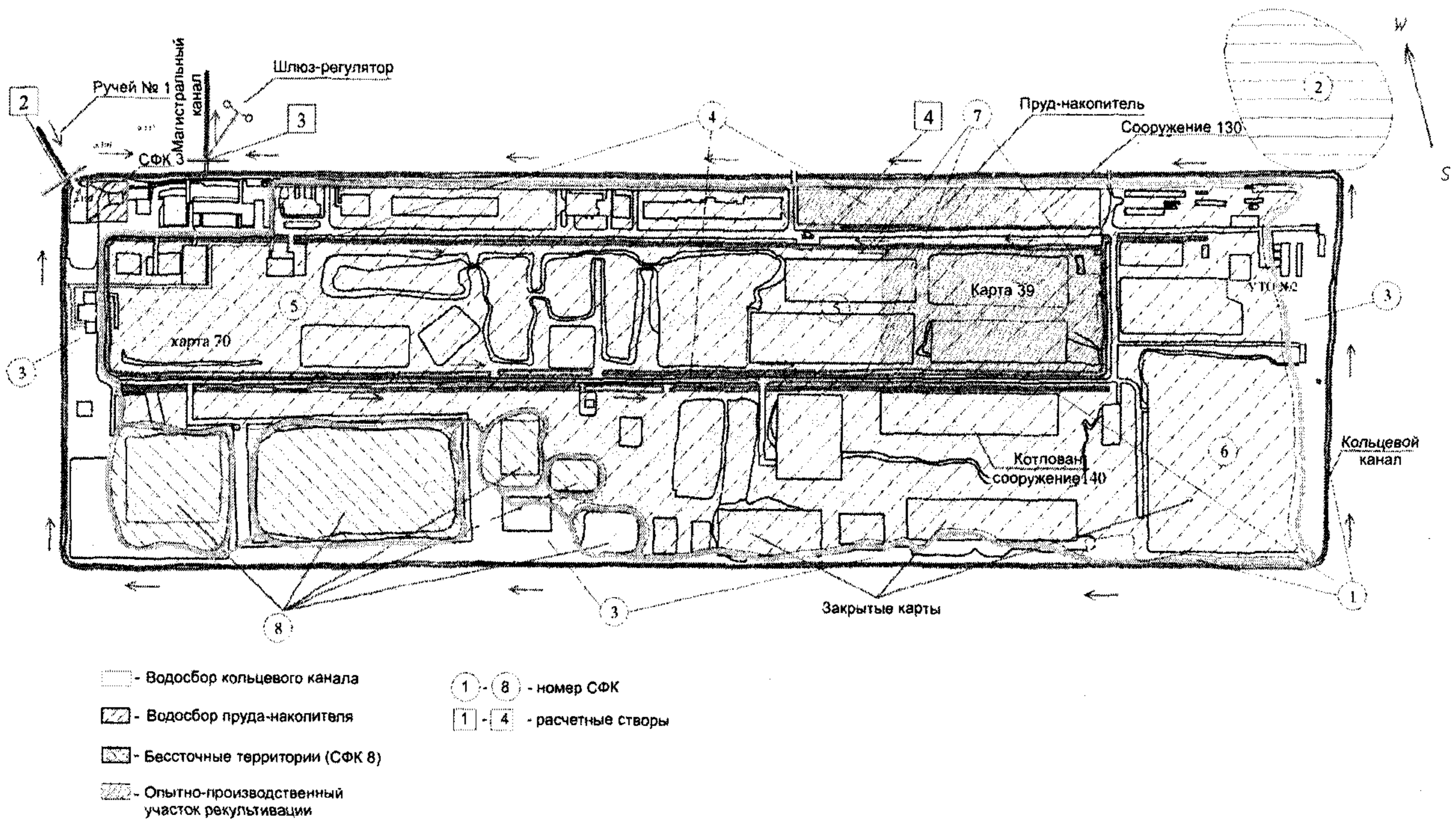
Рис. П.3.1. Схема территории полигона «Красный Бор»
