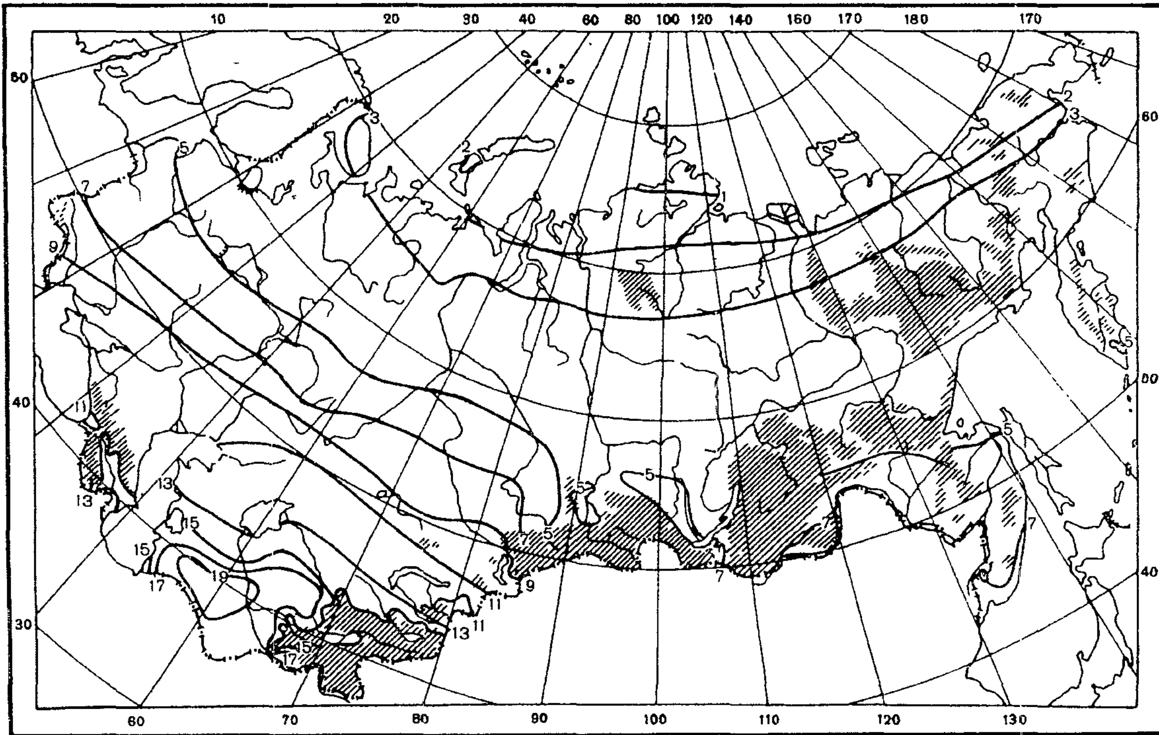
Рис. П2.11. Средняя месячная испаряемость, см. Сентябрь
