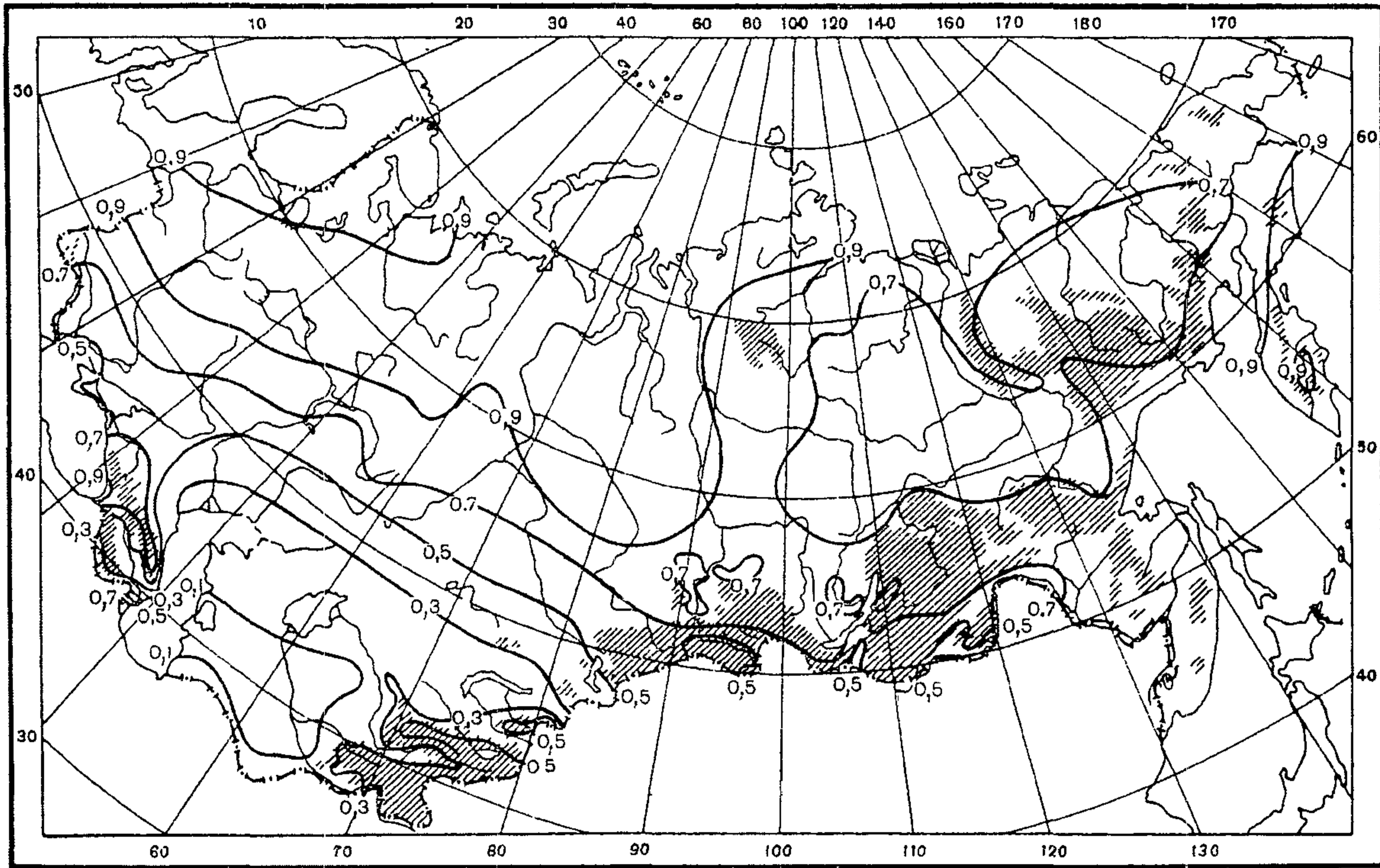
Рис. П2.3. Среднее годовое относительное испарение, E/E_0 ▨ – горные районы
