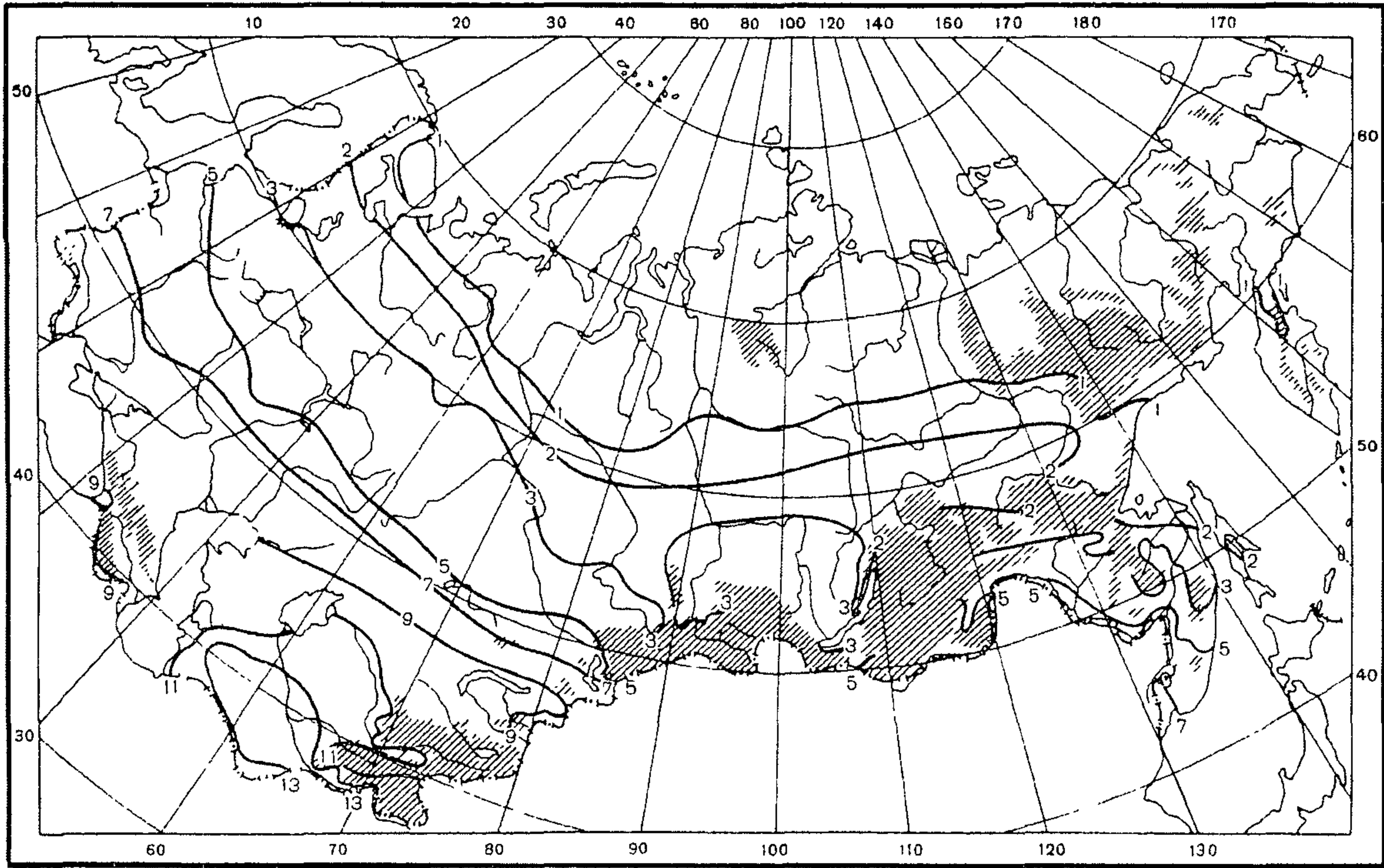
Рис. П2.6. Средняя месячная испаряемость, см. Апрель
