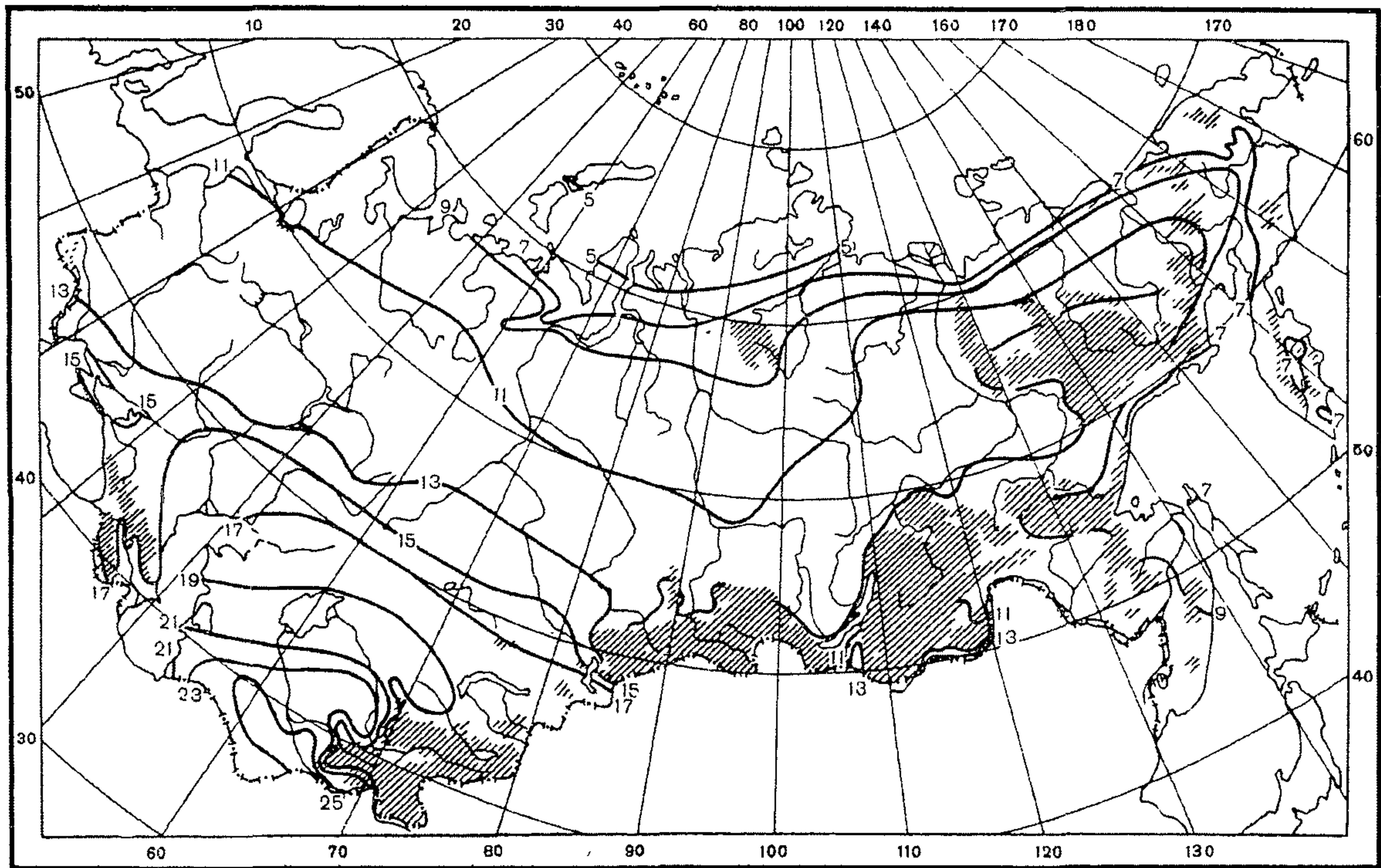
Рис. П2.8. Средняя месячная испаряемость, см. Июнь
