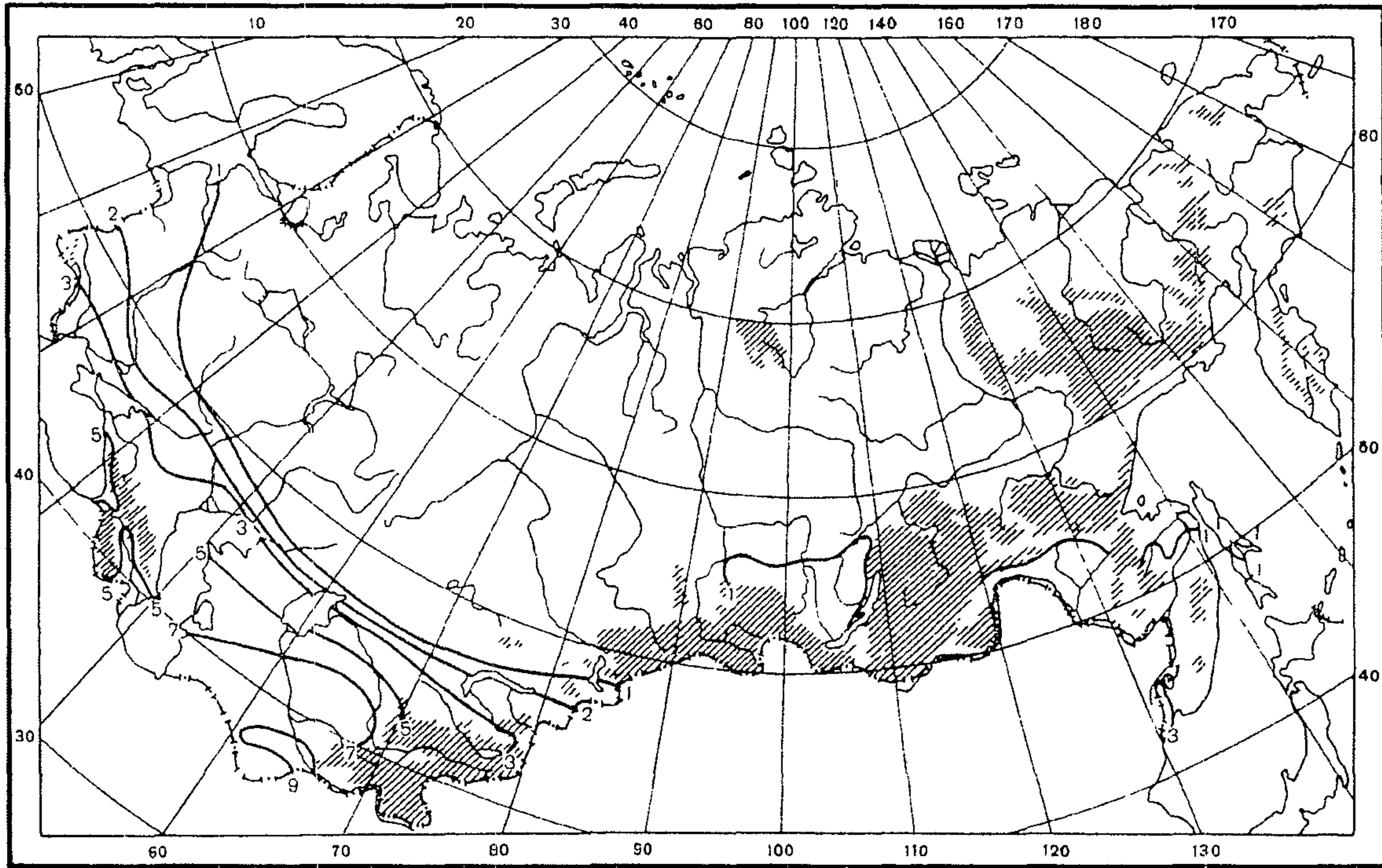
Рис. П2.5. Средняя месячная испаряемость, см. Март
