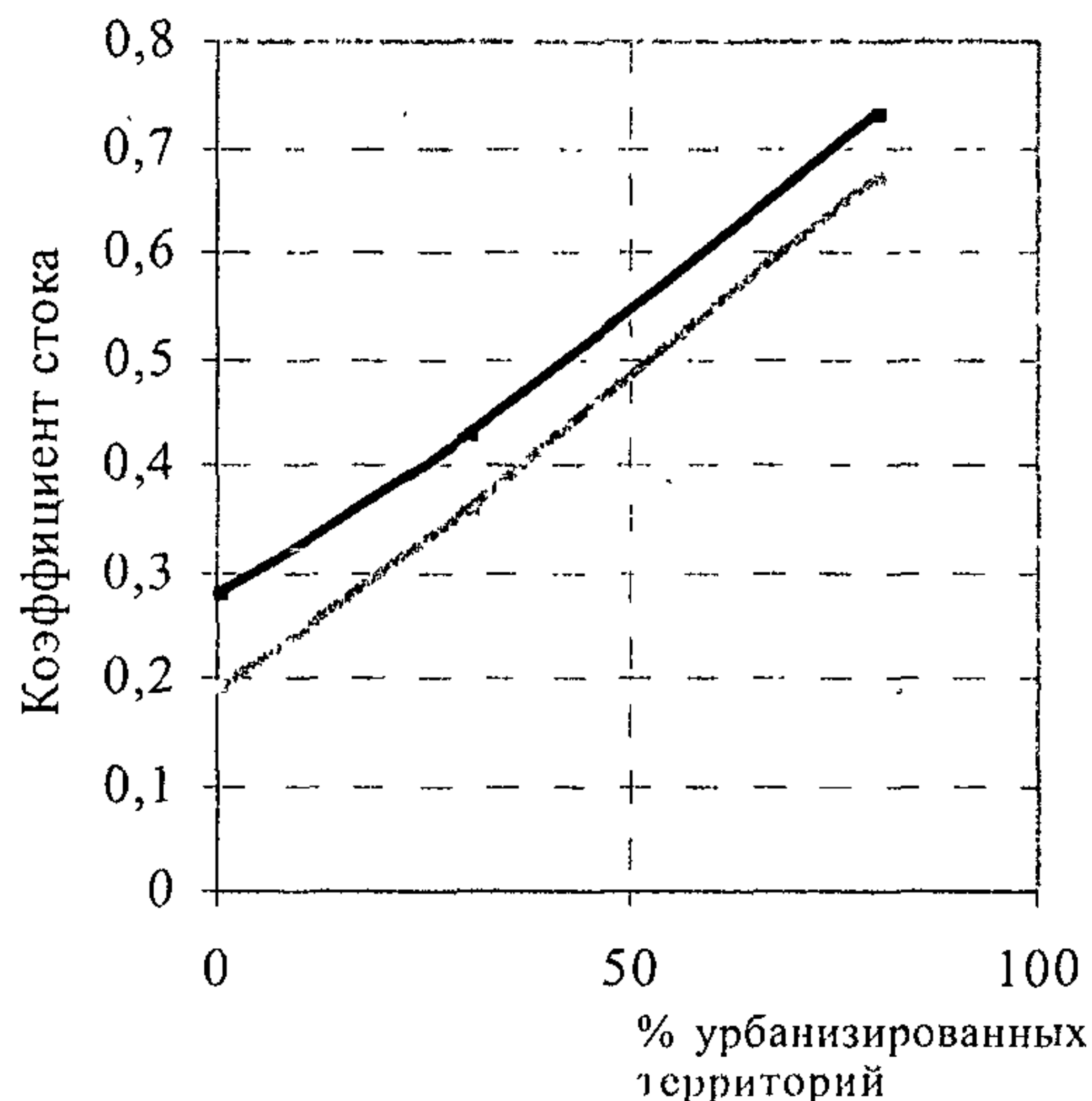
Рис. 2. Зависимость коэффициентов годового полного и поверхностного стока от площади урбанизированных территорий (в процентах от общей площади): — коэффициент полного стока; — коэффициент поверхностного стока
