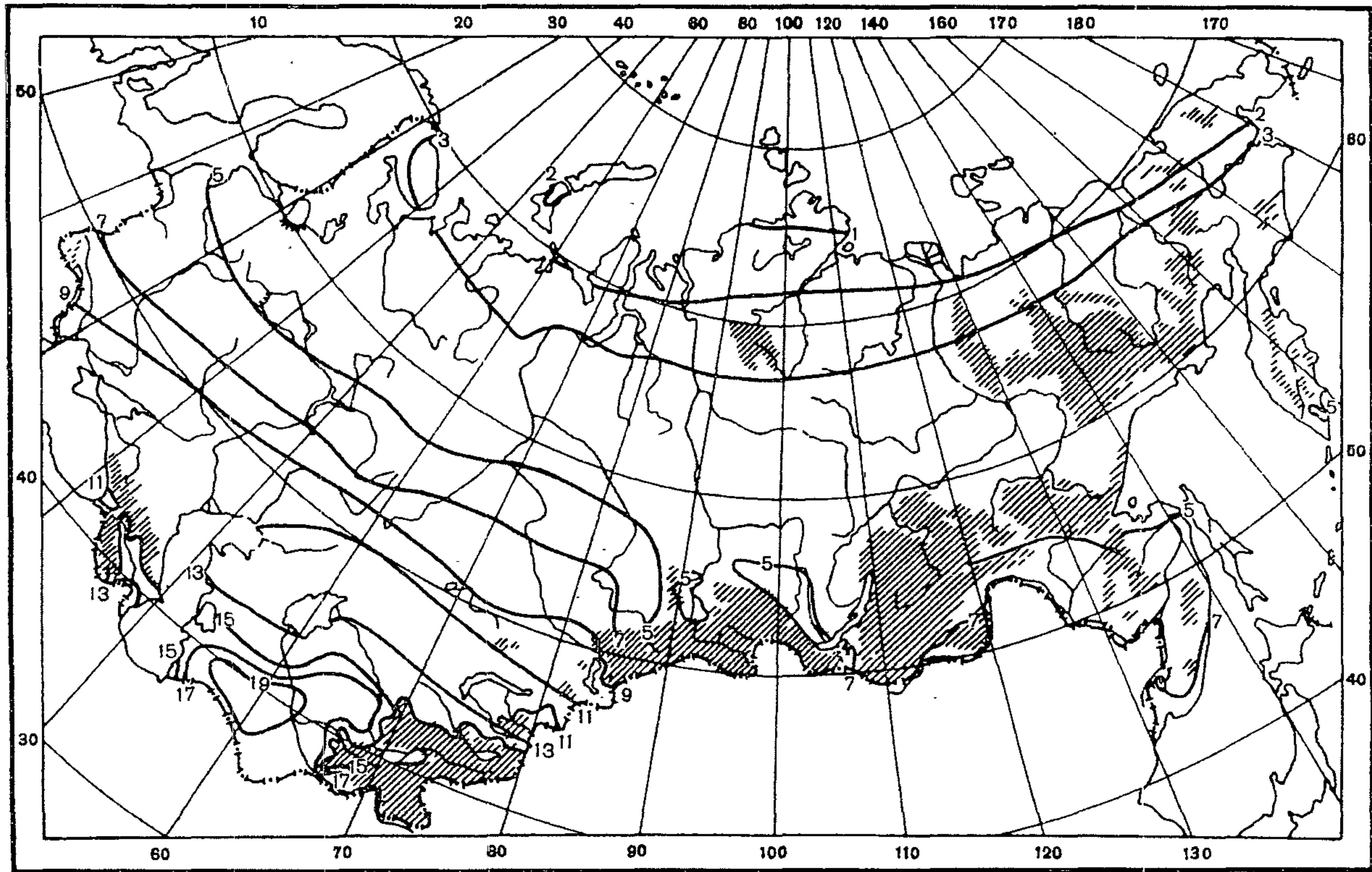
Рис. П2.11. Средняя месячная испаряемость, см. Сентябрь
