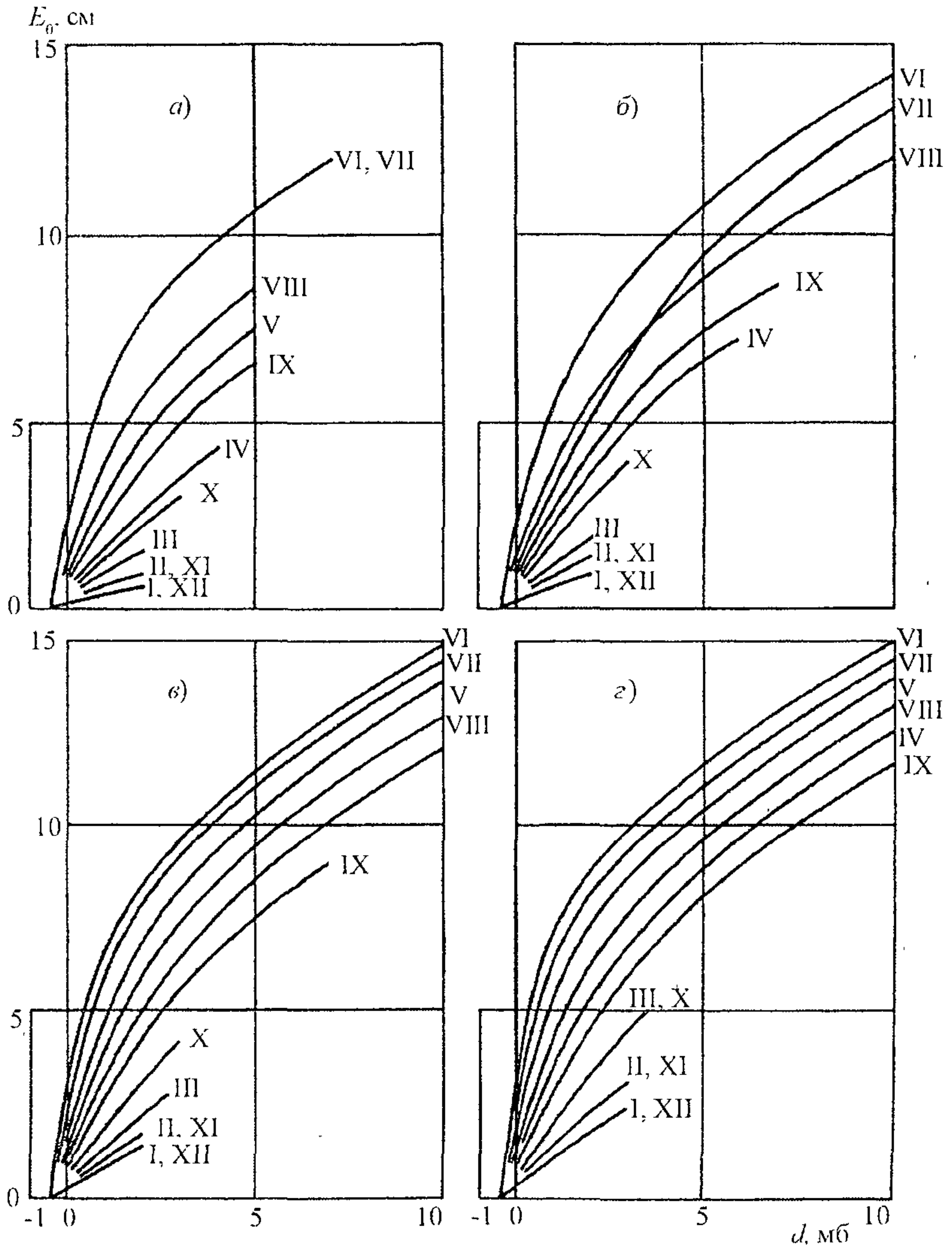
Рис. П2.4 Зависимость испаряемости E_0 от дефицита влажности воздуха d : а – зона тундры и лесотундры, б – зона хвойных лесов, в – зона смешанных лесов, г – зона лиственных лесов
