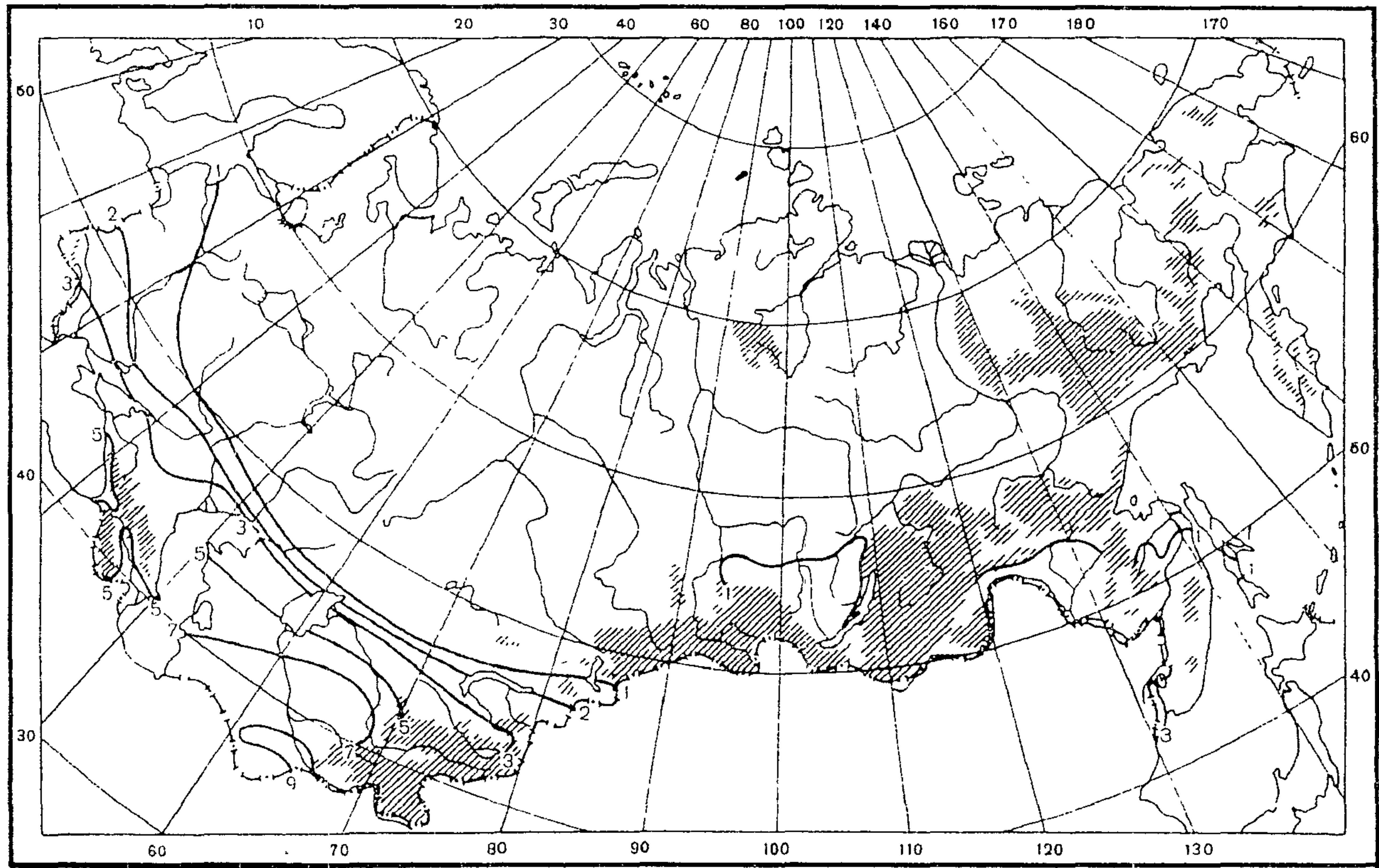
Рис П2.5 Средняя месячная испаряемость, см. Март
