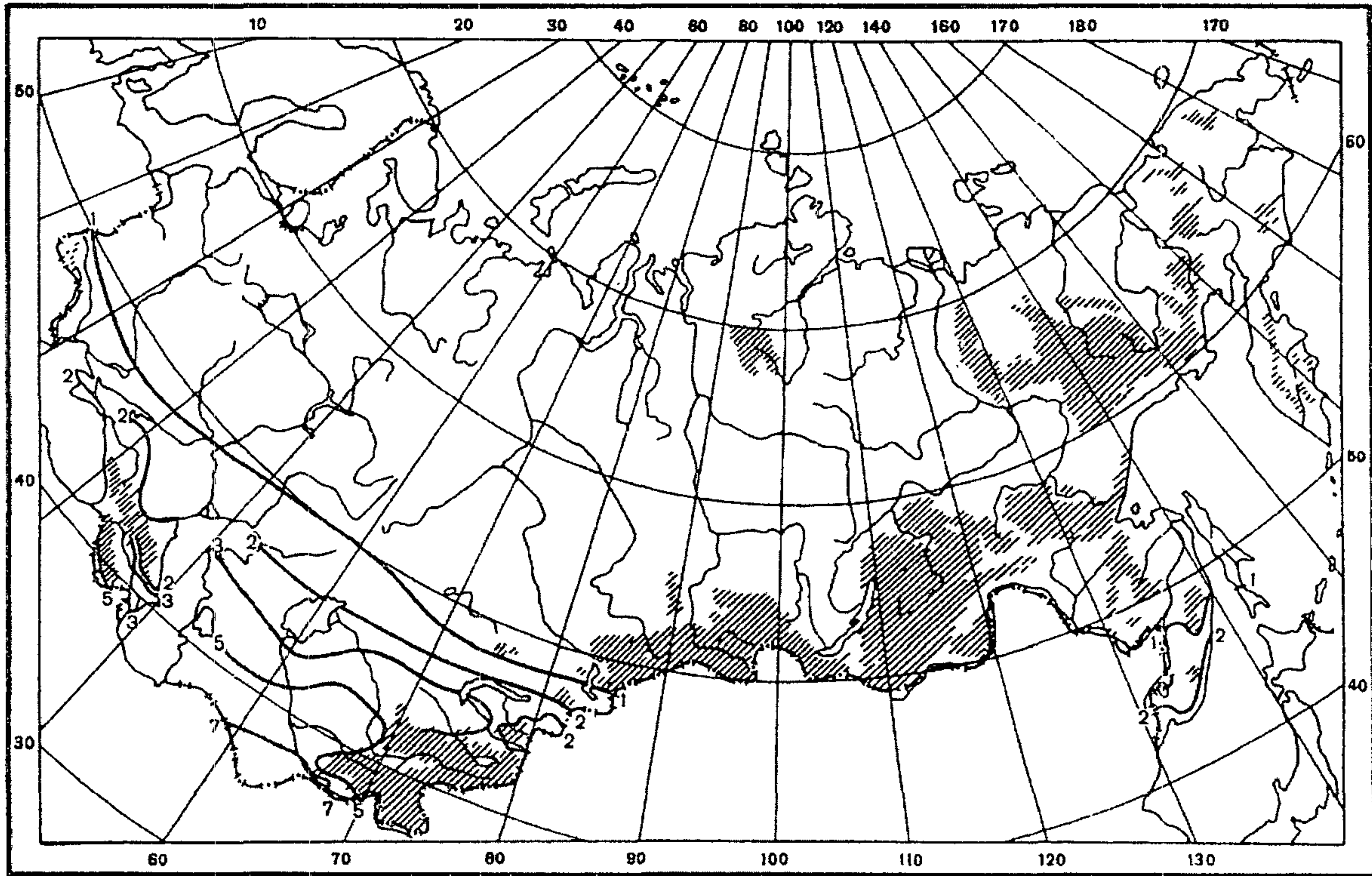
Рис. П2.13. Средняя месячная испаряемость, см. Ноябрь
