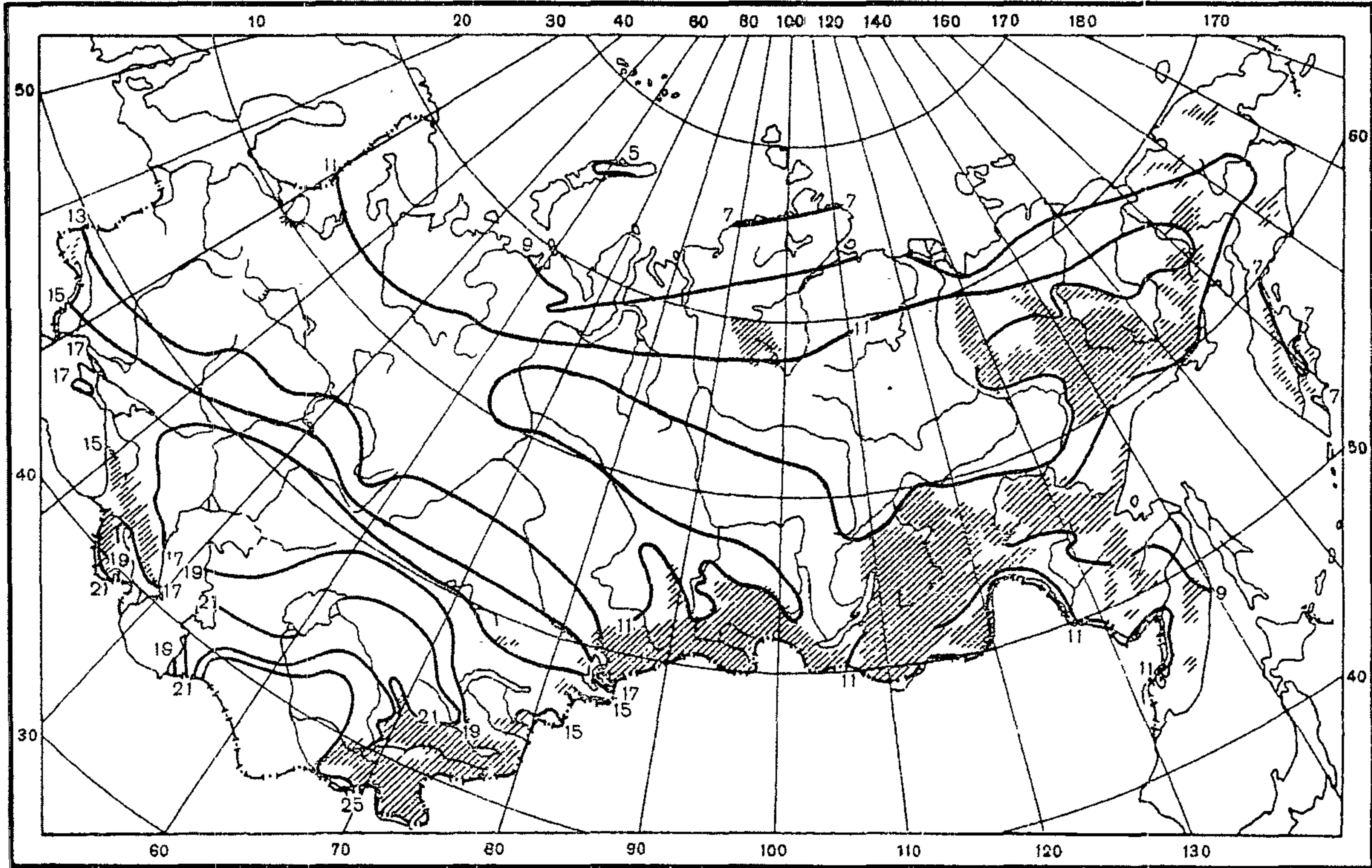
Рис. П2.9. Средняя месячная испаряемость, см. Июль
