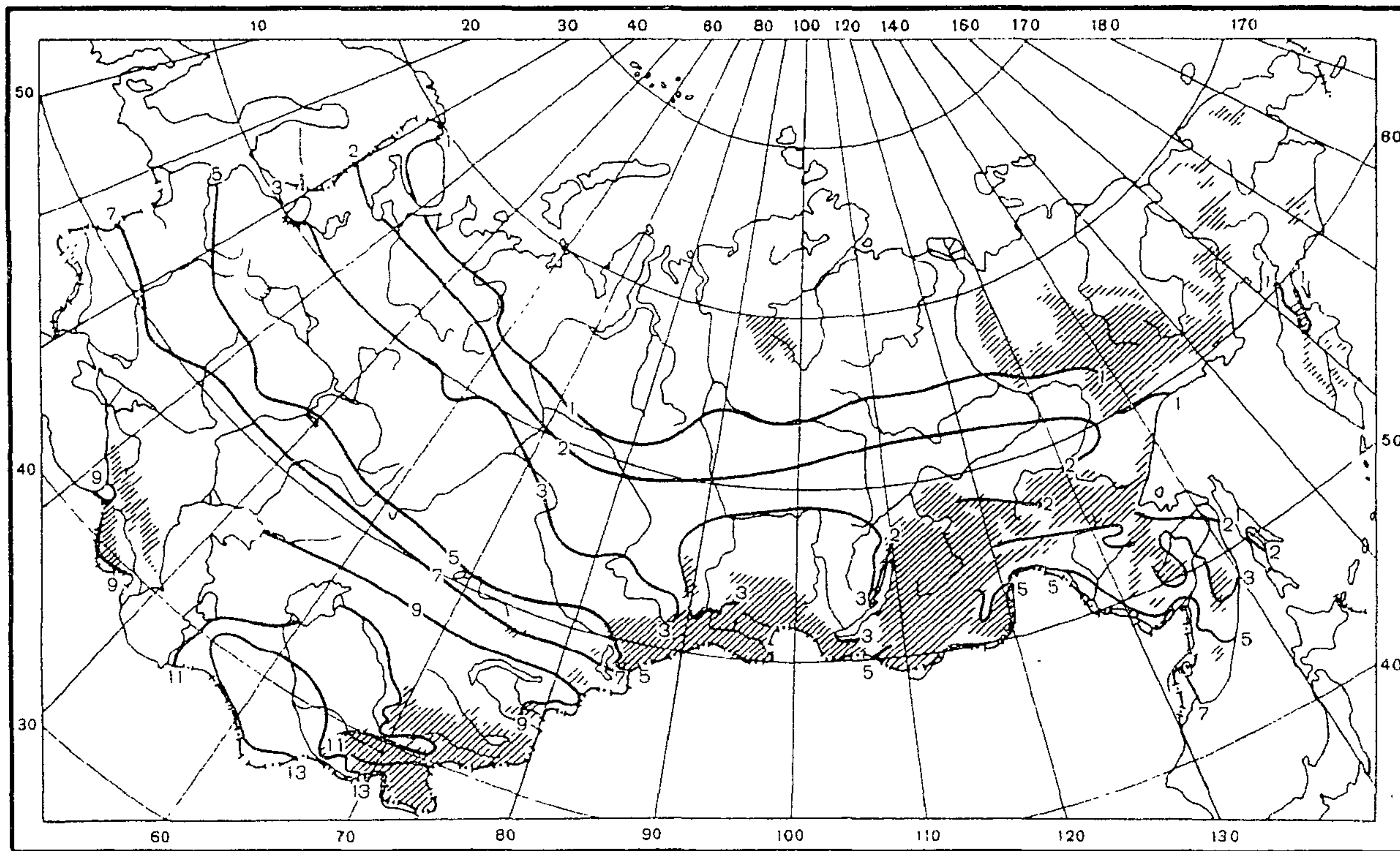
Рис. П2 6 Средняя месячная испаряемость, см. Апрель
