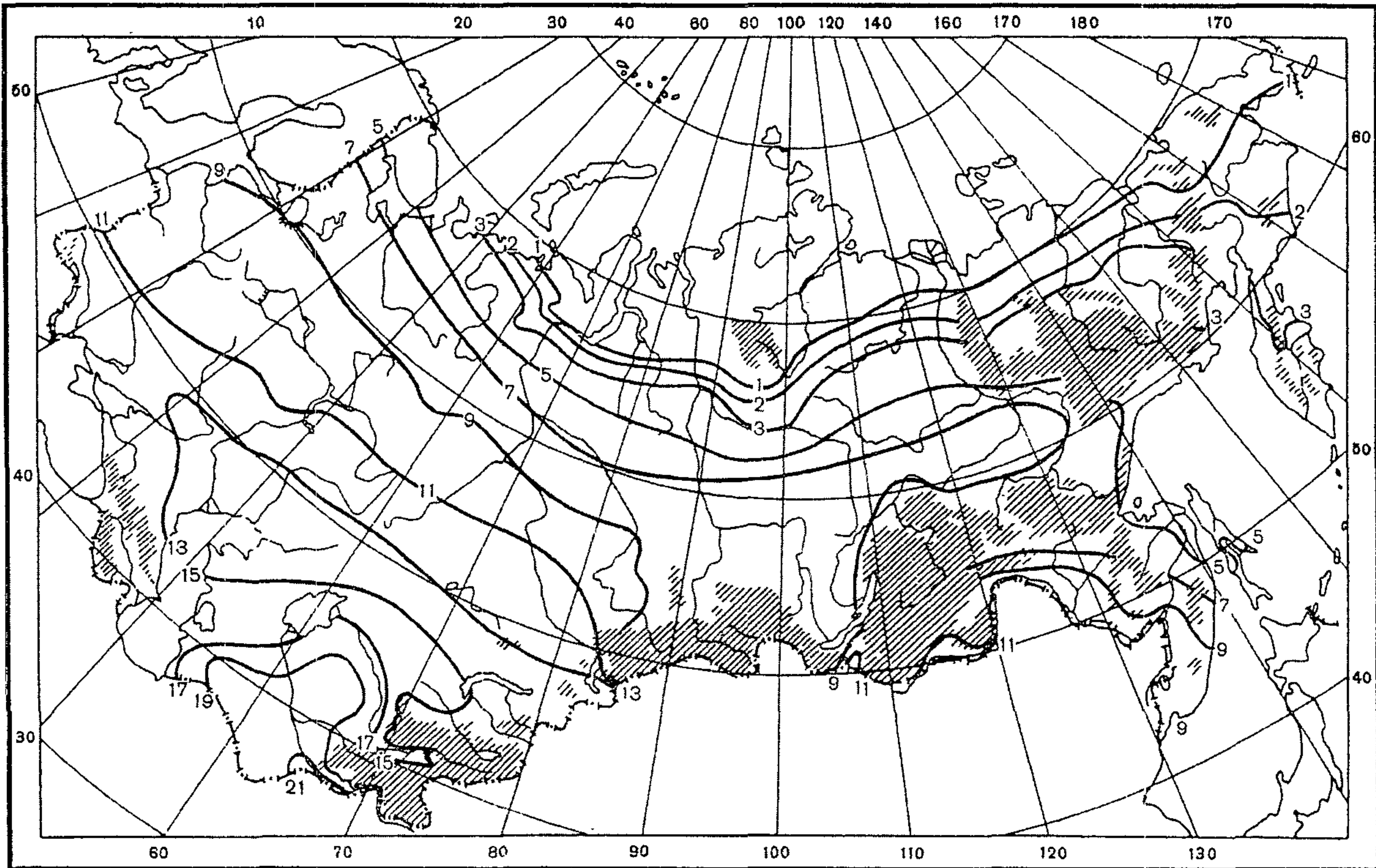
Рис. П2.7. Средняя месячная испаряемость, см. Май
