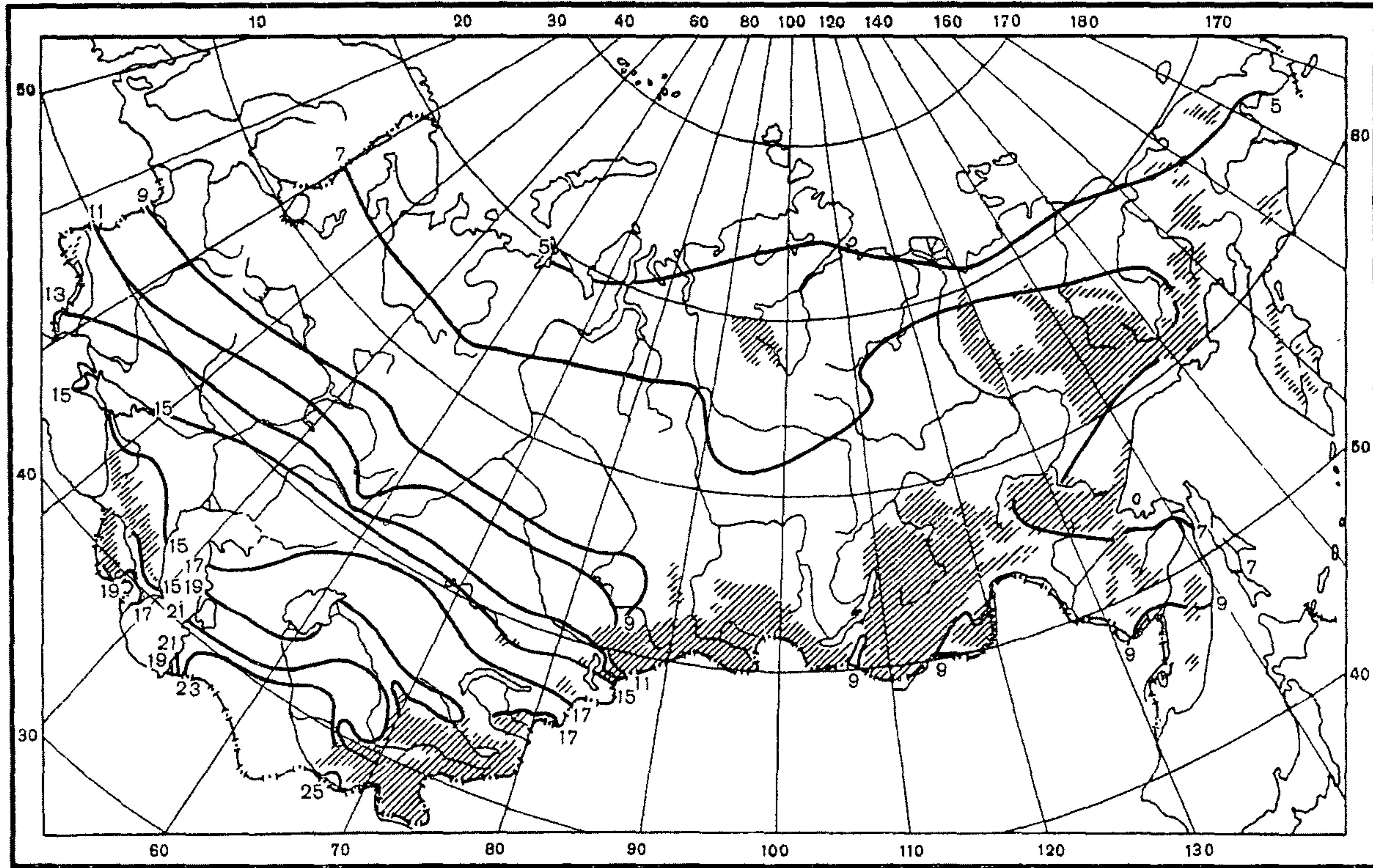
Рис. П2.10. Средняя месячная испаряемость, см. Август
