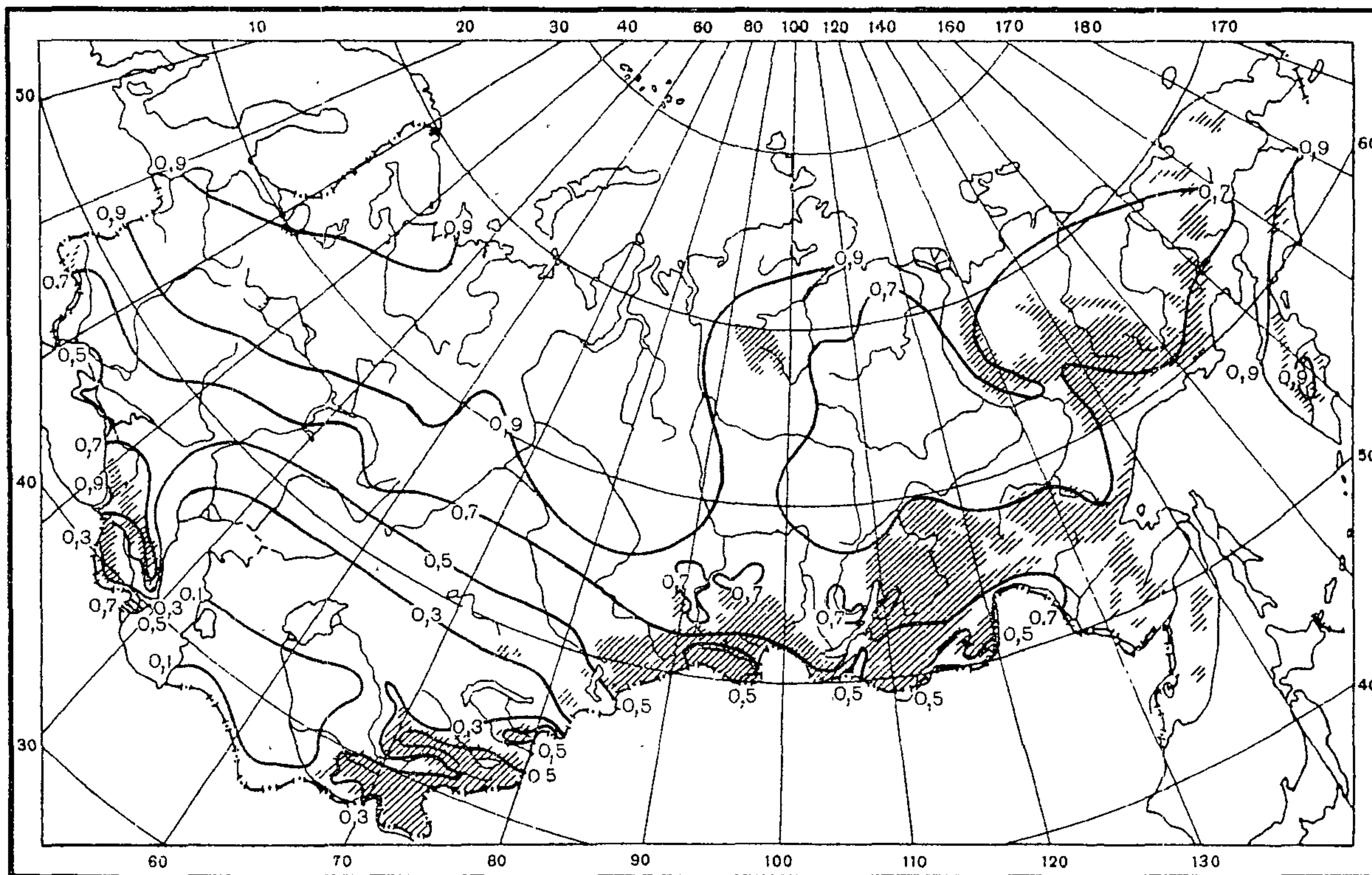
Рис. П2.3. Среднее годовое относительное испарение. E/E_0
