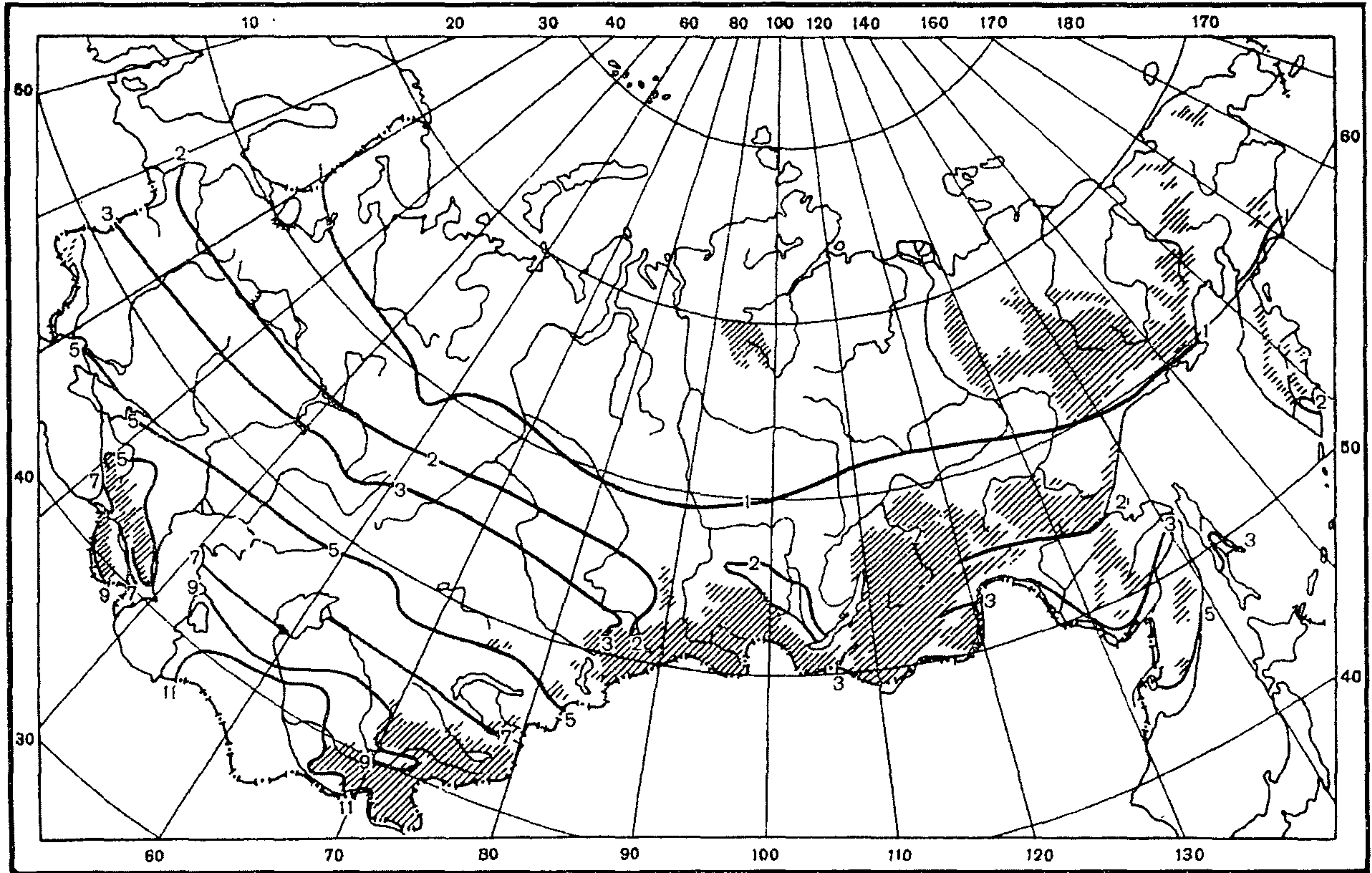
Рис. П2. 12. Средняя месячная испаряемость, см. Октябрь
