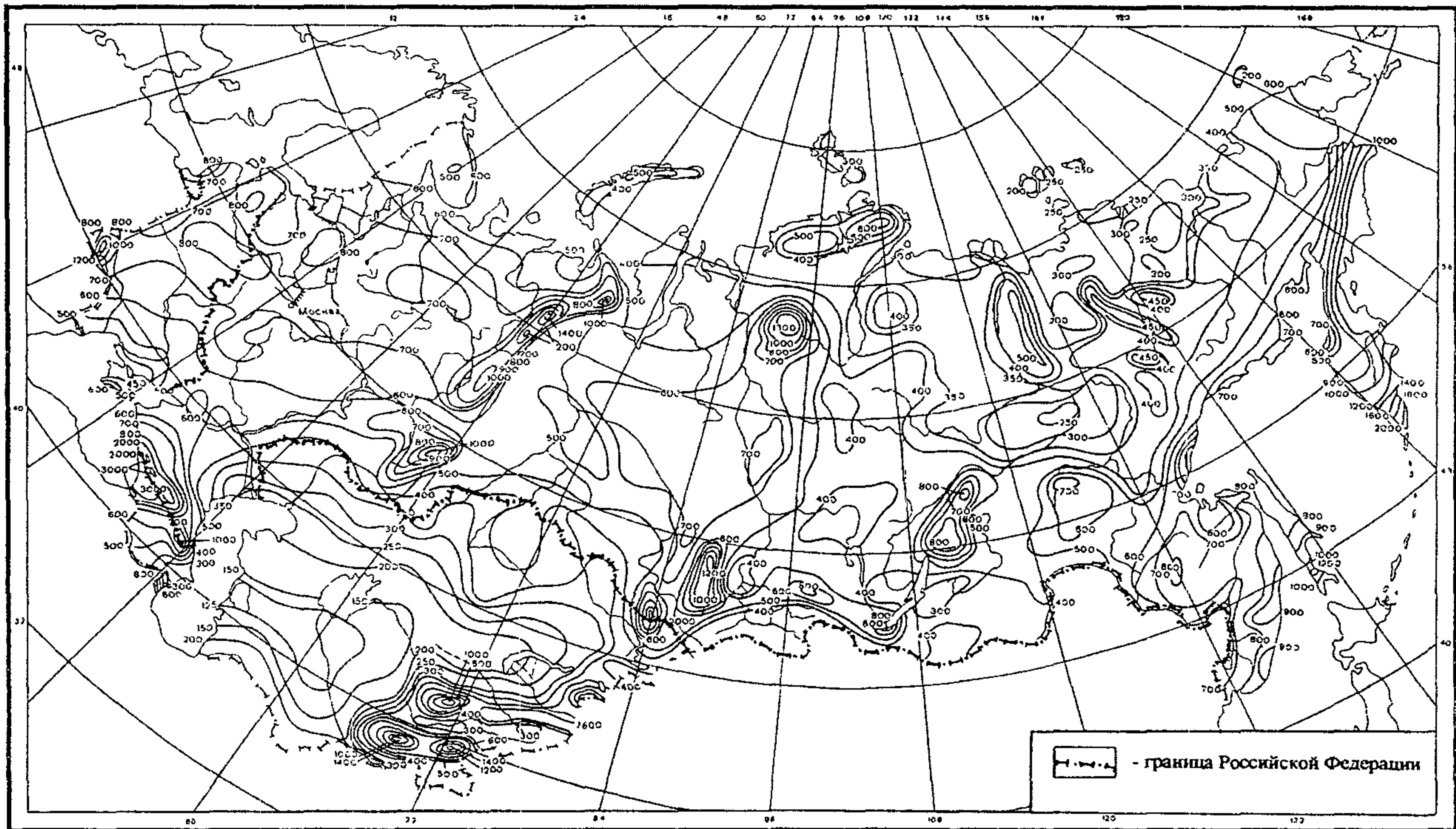
Рис. П2.1. Среднее годовое количество осадков, мм
