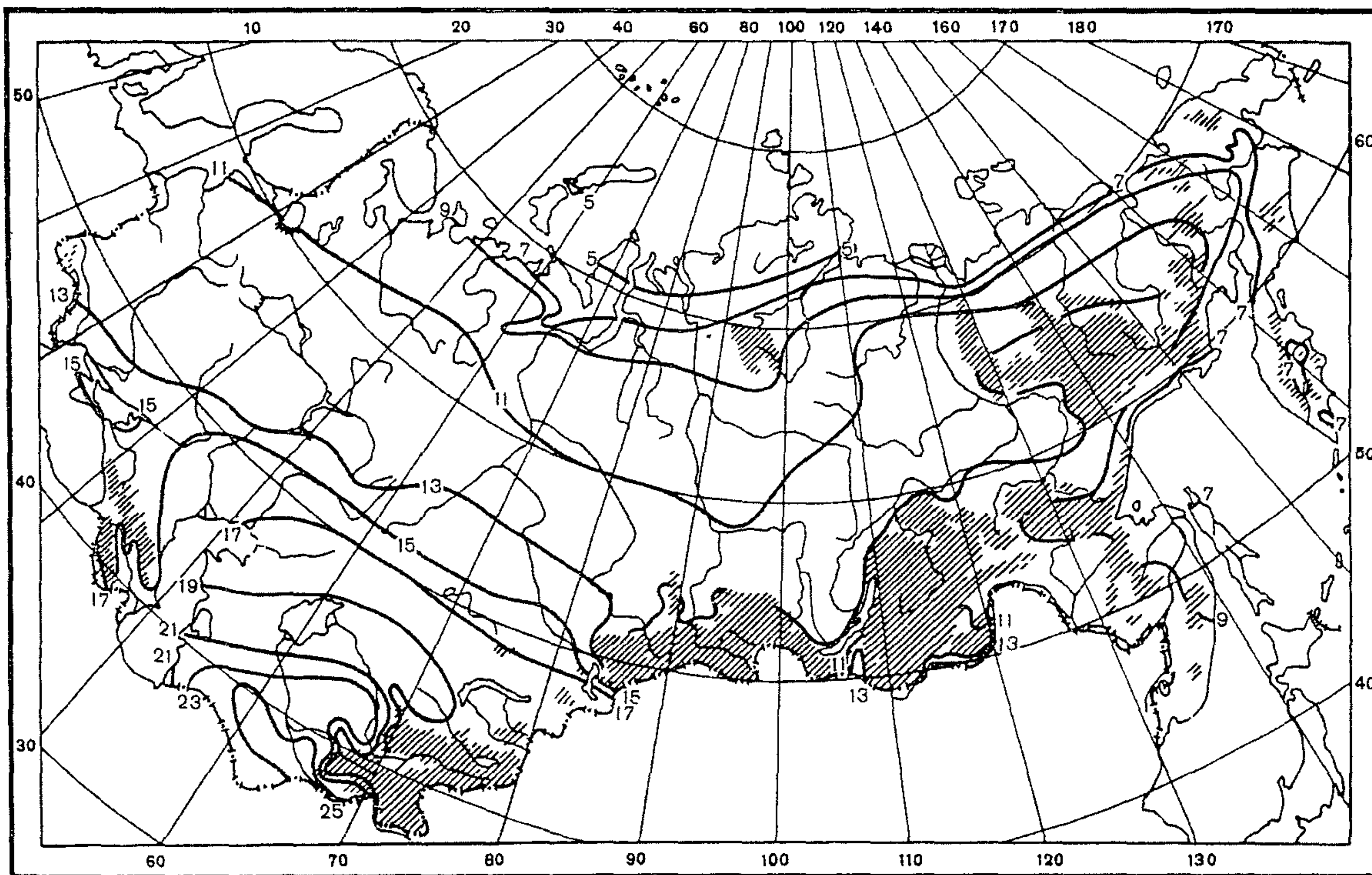
Рис. П2.8. Средняя месячная испаряемость, см. Июнь
