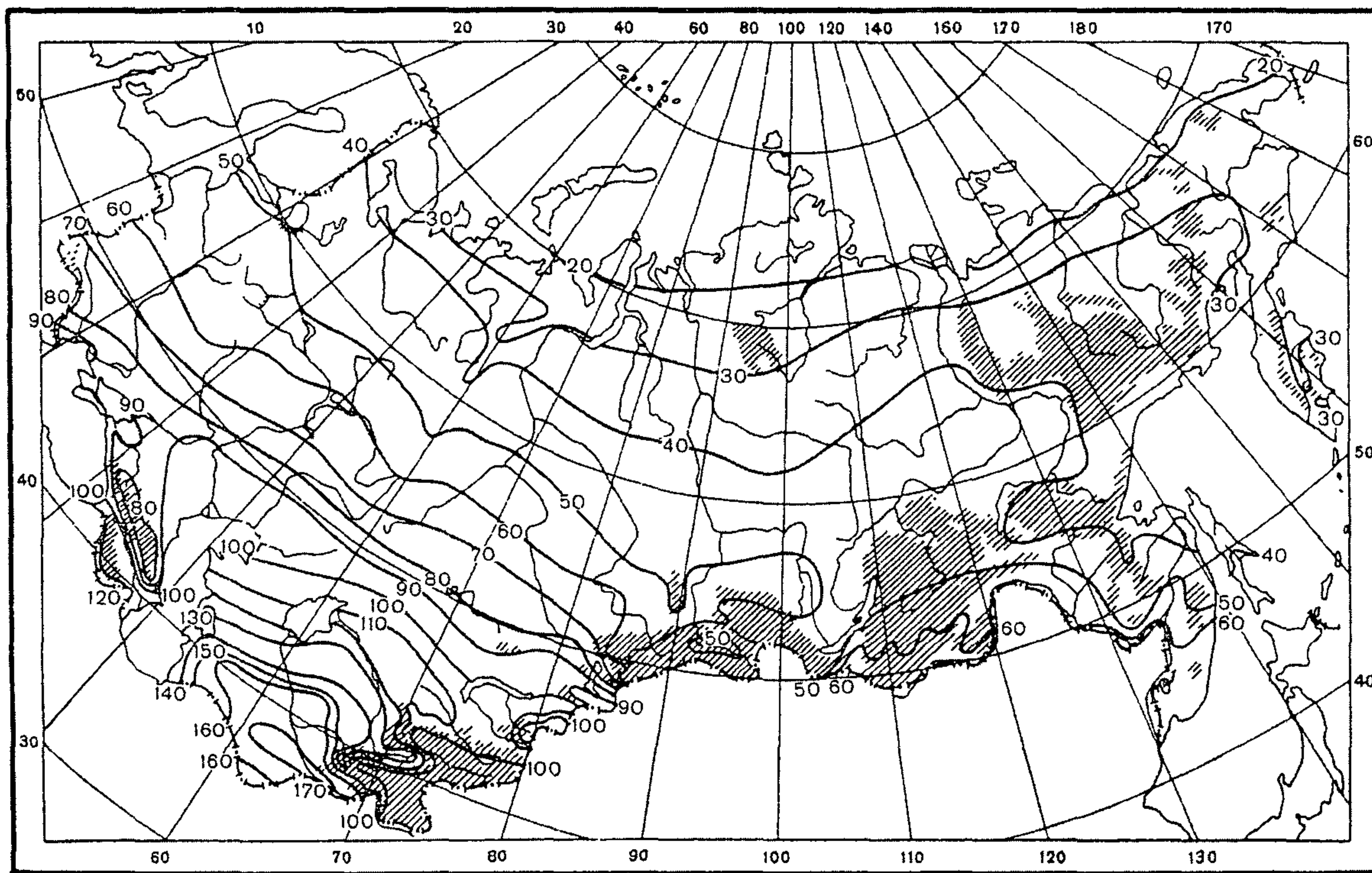
Рис. П2.2. Средняя годовая испаряемость, см
