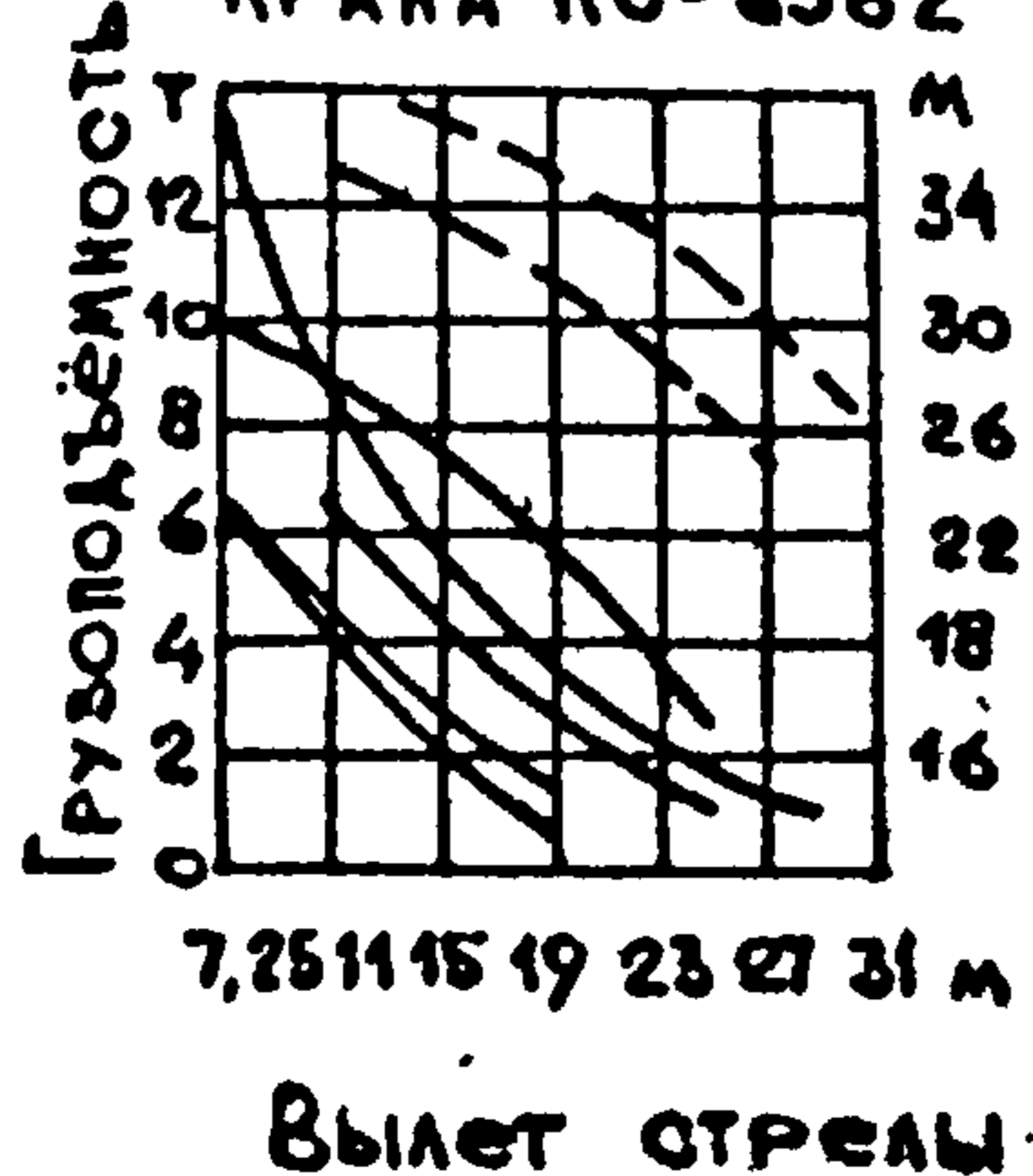
График грузоподъемности крана КС-6362
