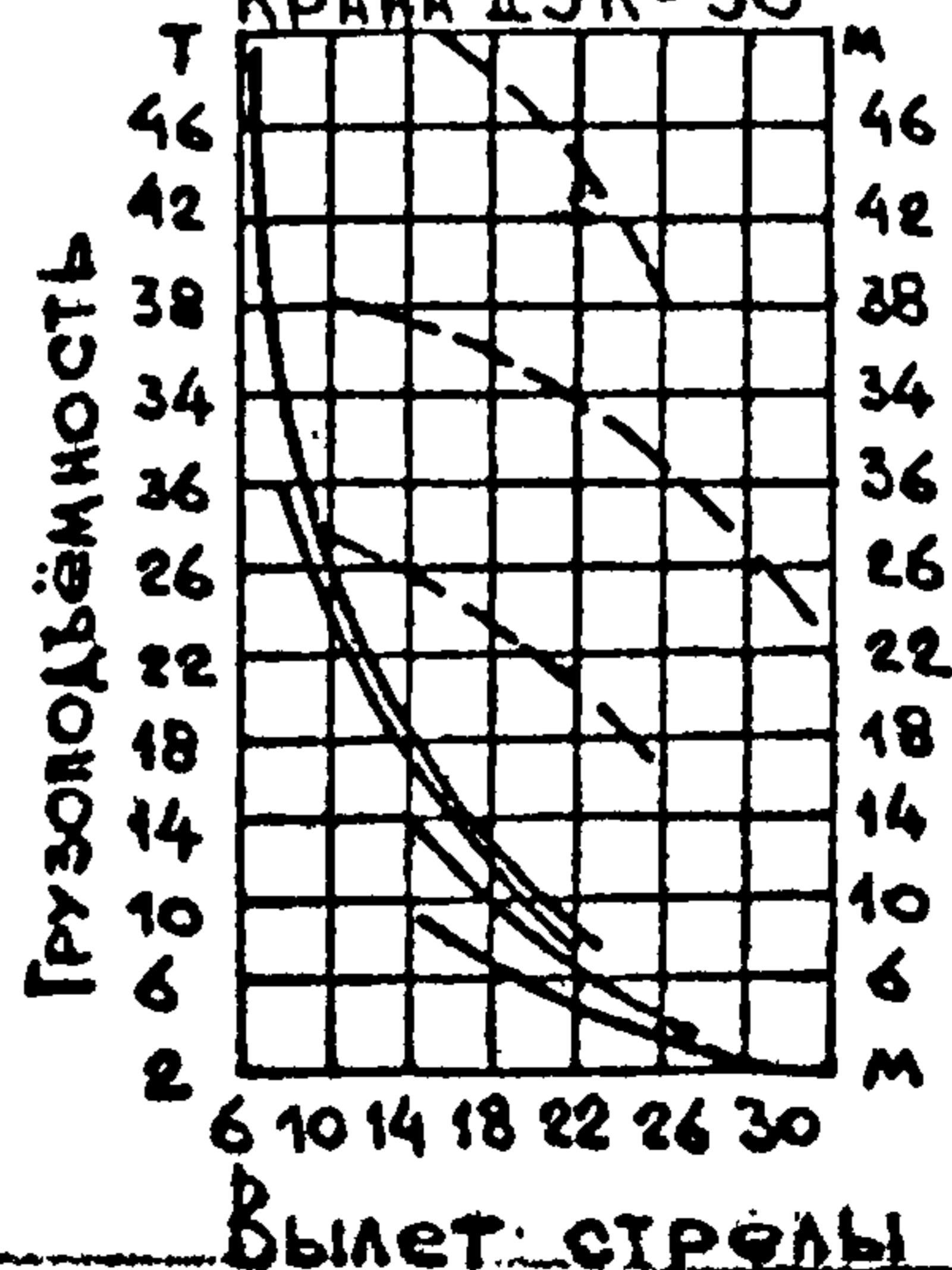
График грузоподъемности крана ДЭК-50
