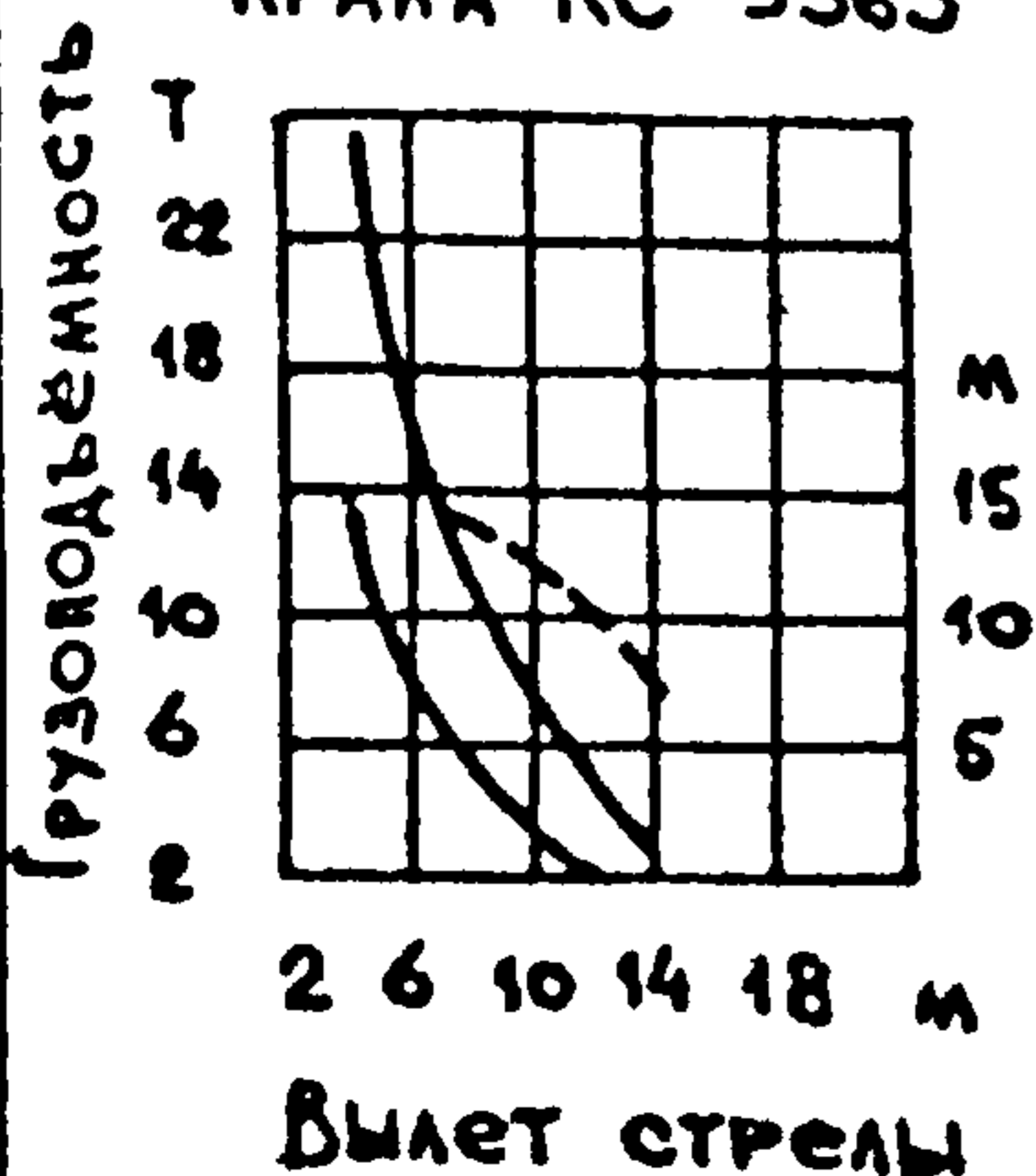
График грузоподъемности крана КС-5363
