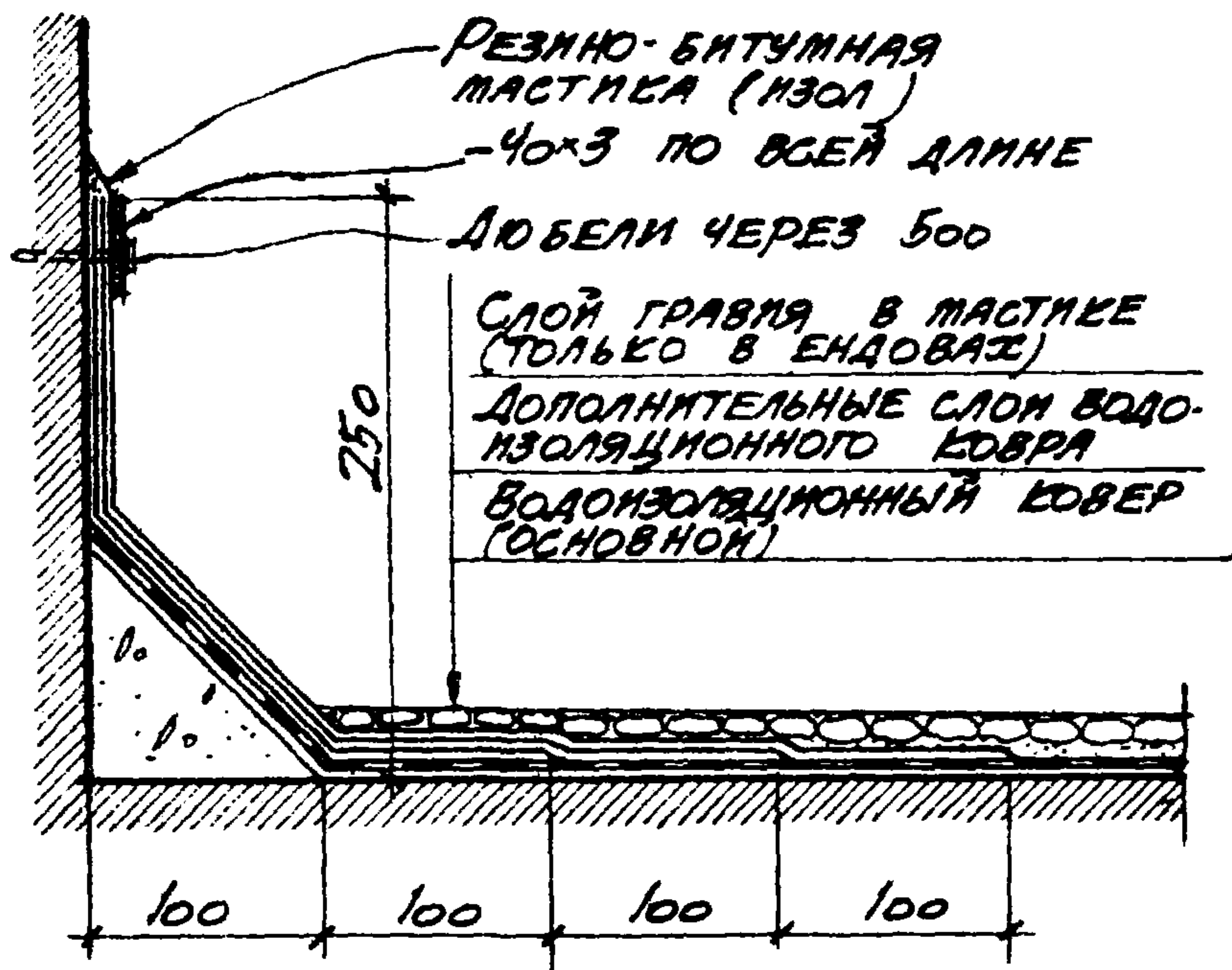
УЗЕЛ А
