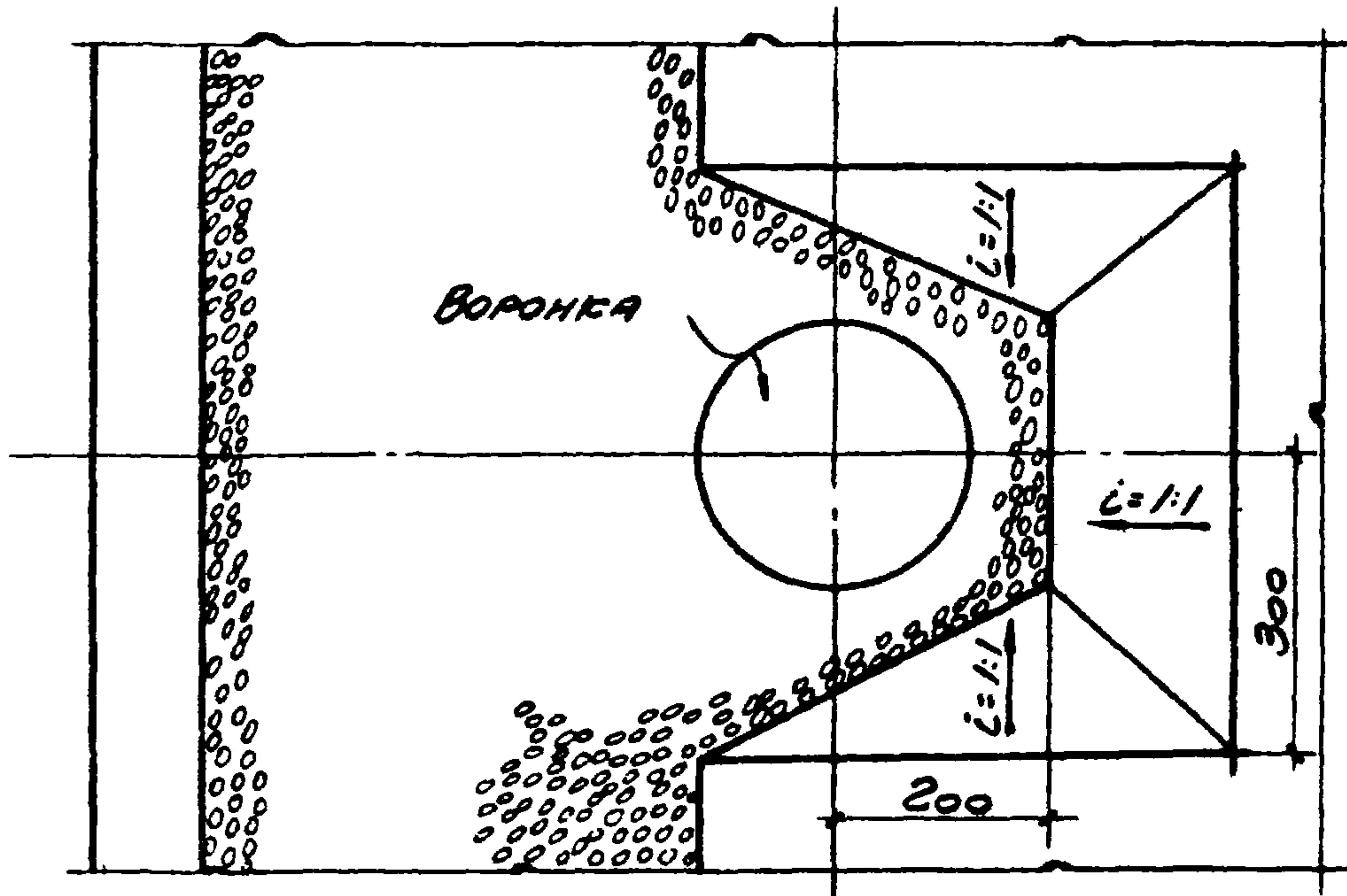
ПЛАН ЕНДОВБИ
