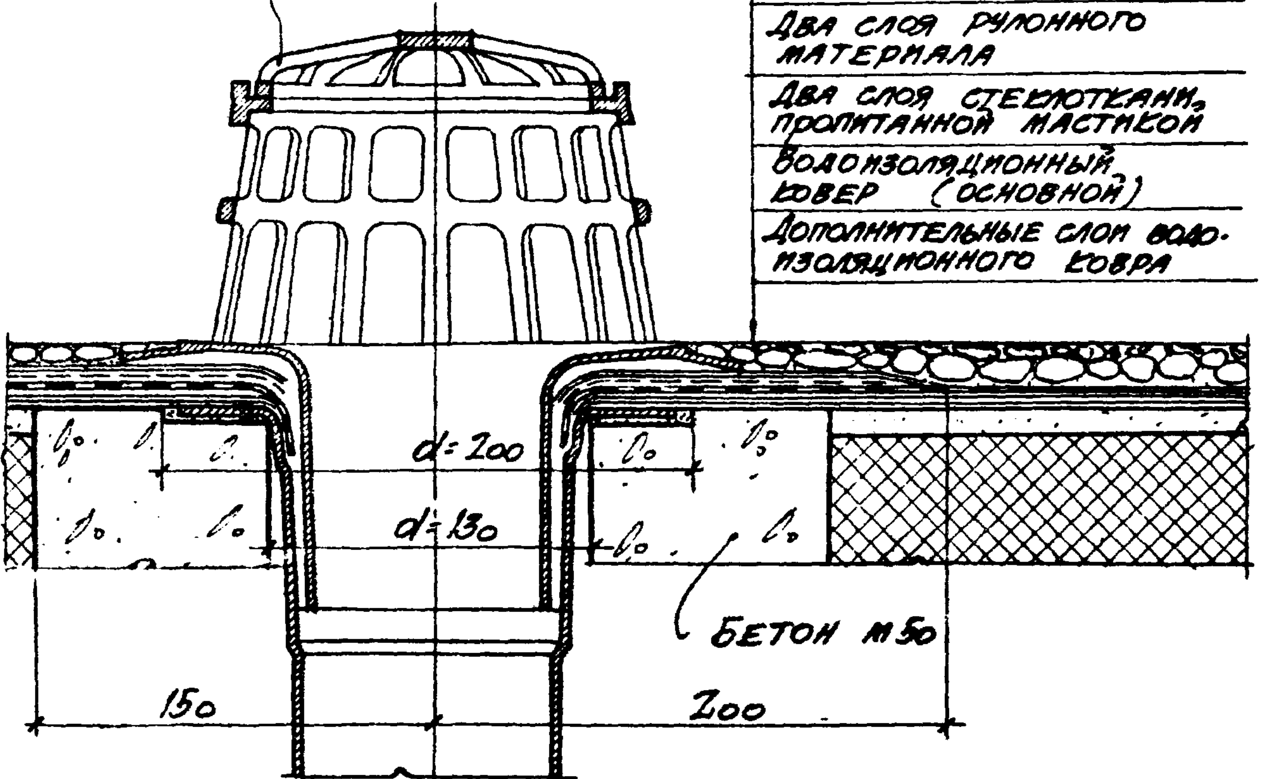
УЗЕЛ Б
