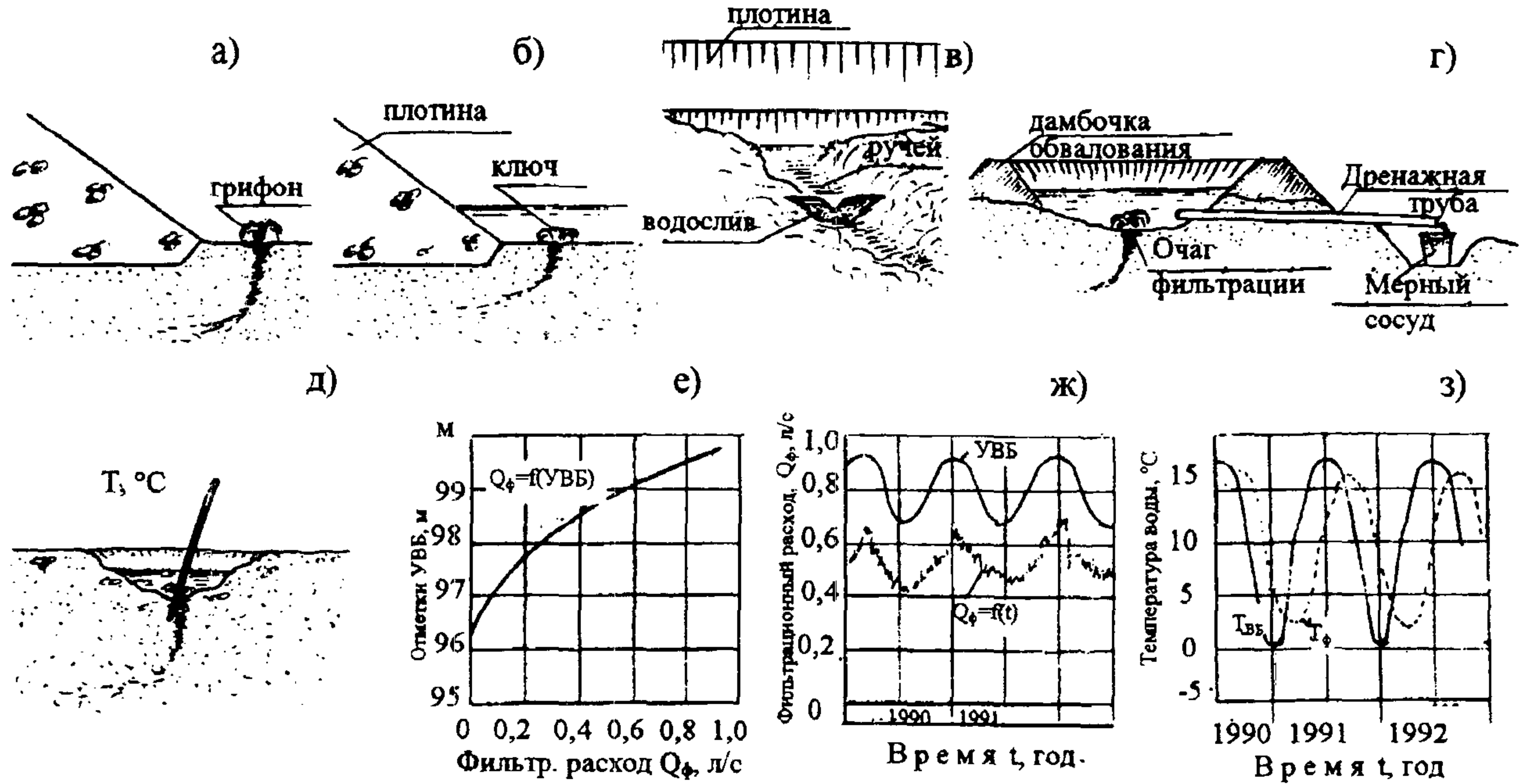
Рис.4.13. Наблюдения за сосредоточенными очагами фильтрации
