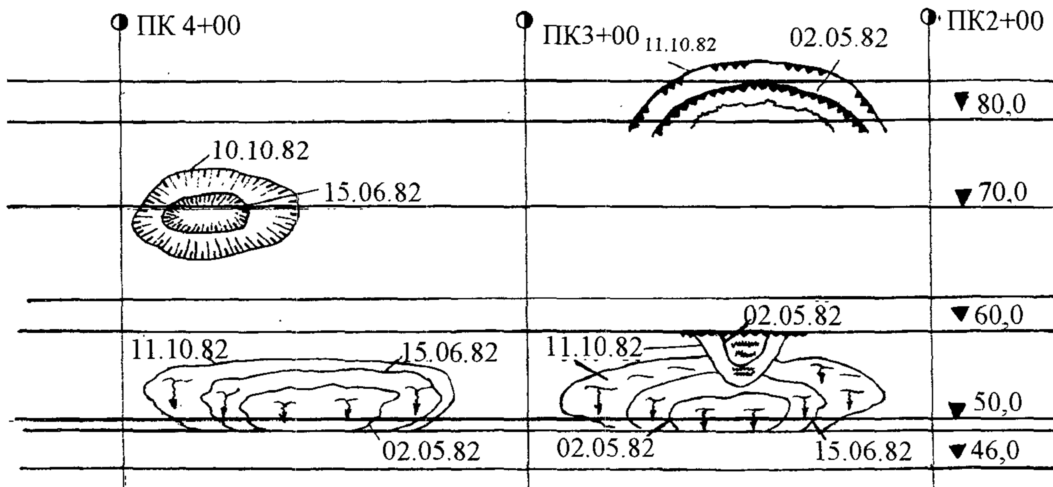
Рис.3.4. Пример карты-развертки фрагмента плотины (низовой откос с бермами)
