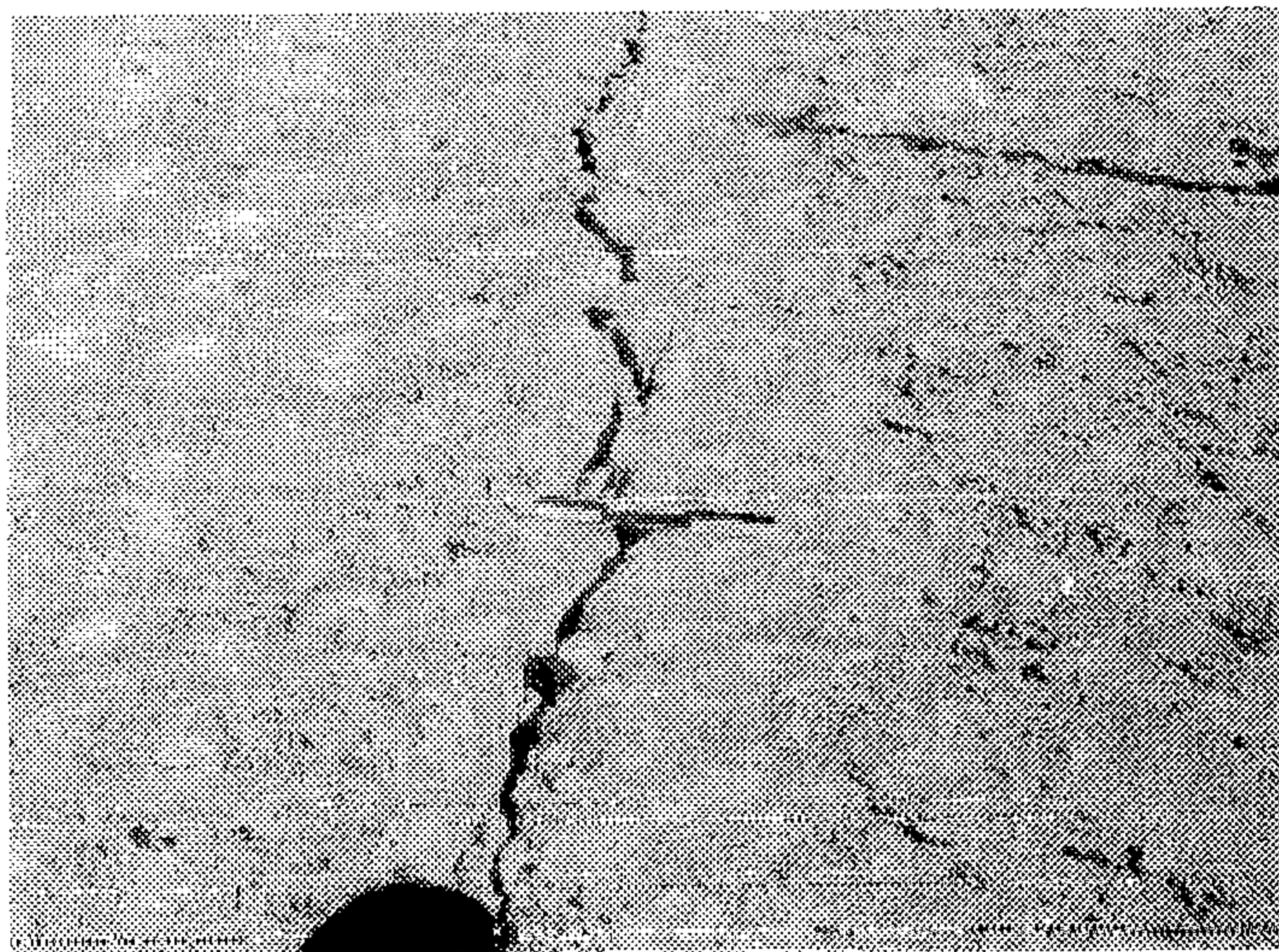
Рис.4.3. Фрагменты трещин a - трещина с уступом; б - трещина без уступа.
