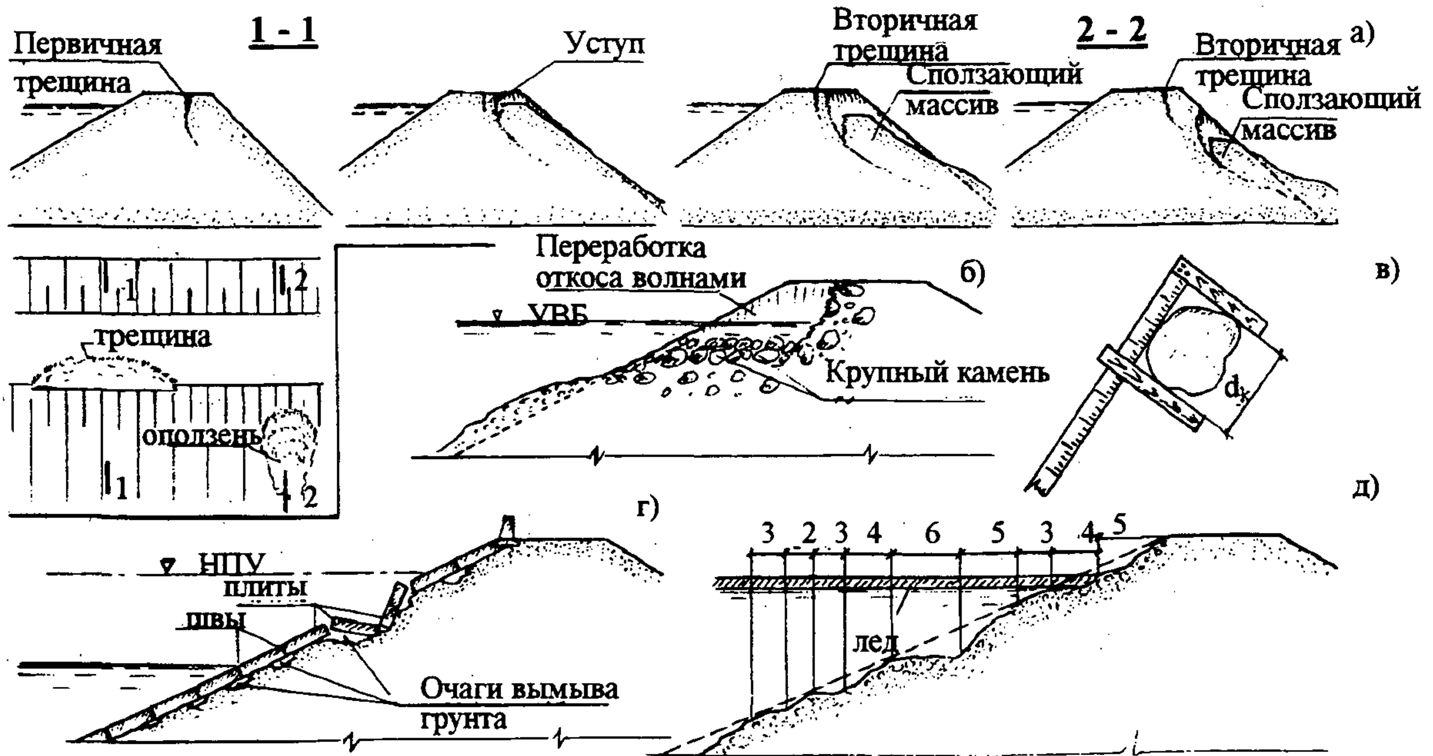
Рис.4.7. Признаки и стадии оползания откоса. Повреждения креплений
