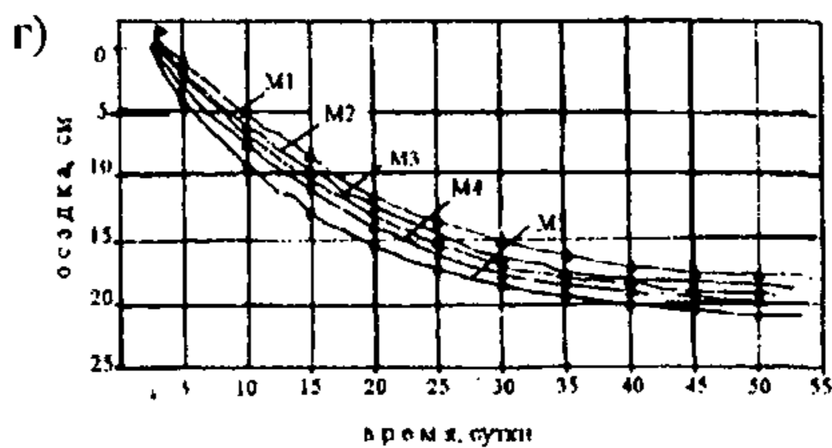
Рис.4.5. Просадки гребня плотины
