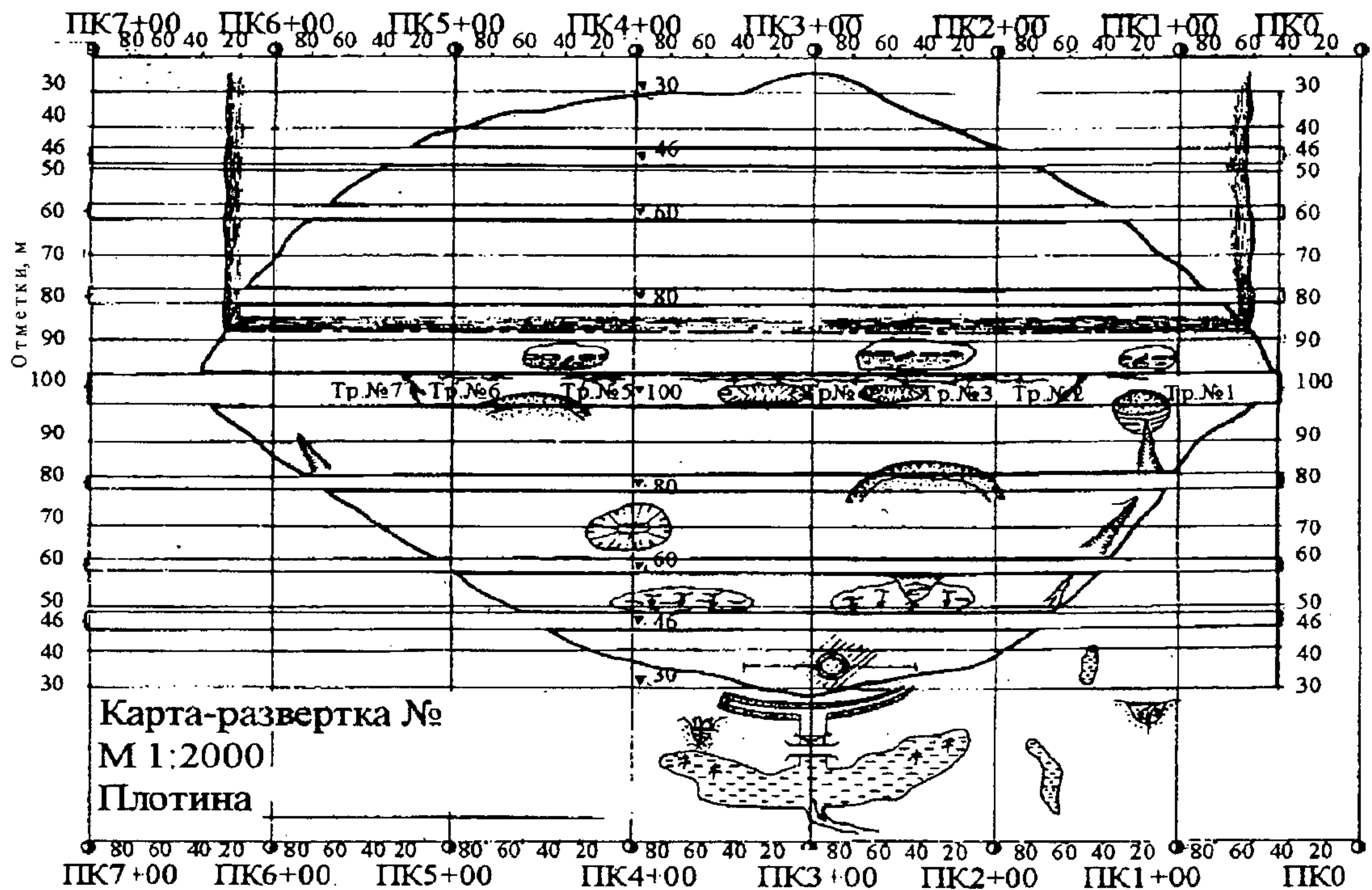
Рис.3.3. Масштабная карта-развертка грунтовой плотины (Условные обозначения см. в табл.3.2).
