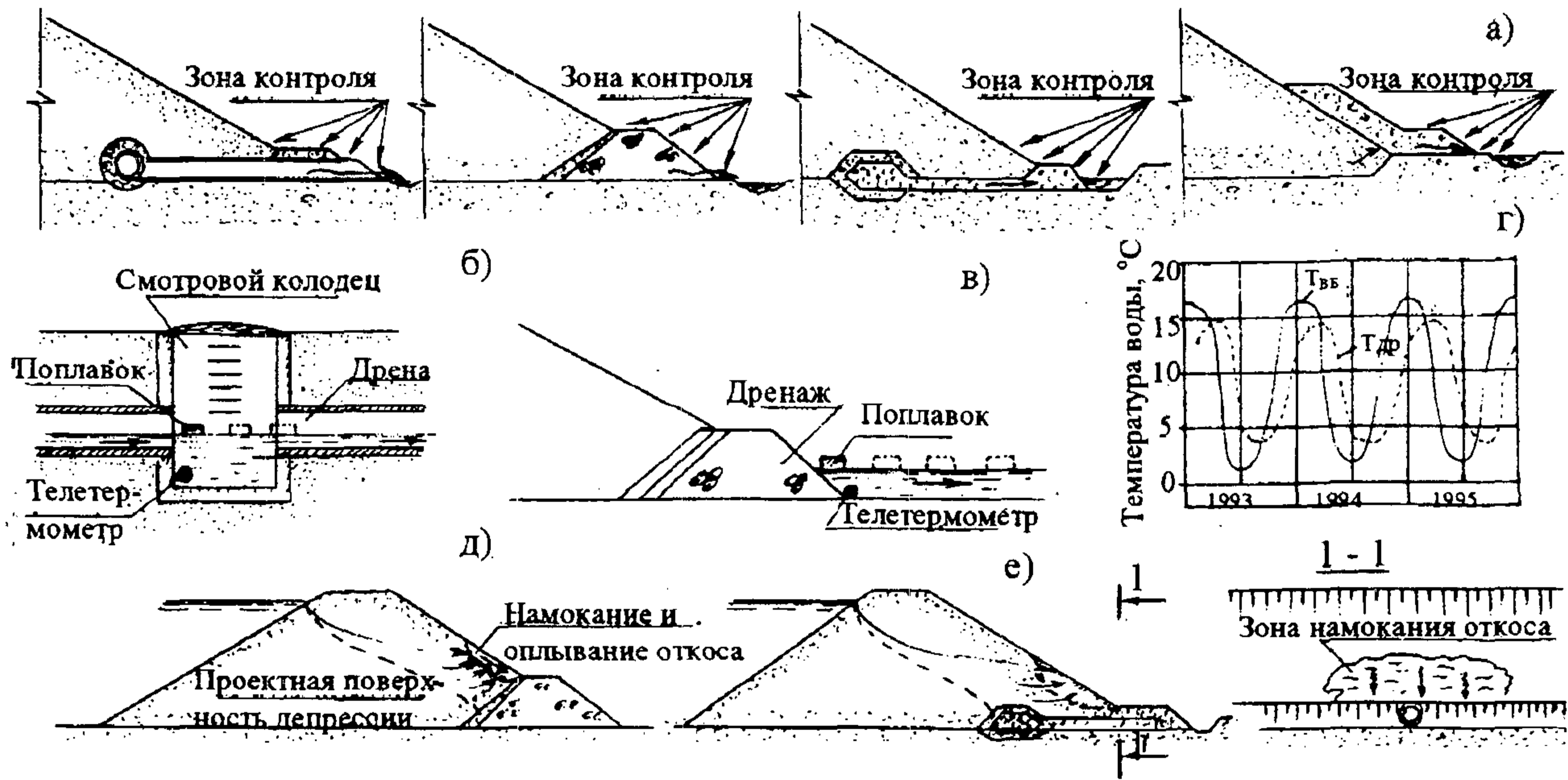
Рис.4.14. Наблюдения за дренажными устройствами плотины
