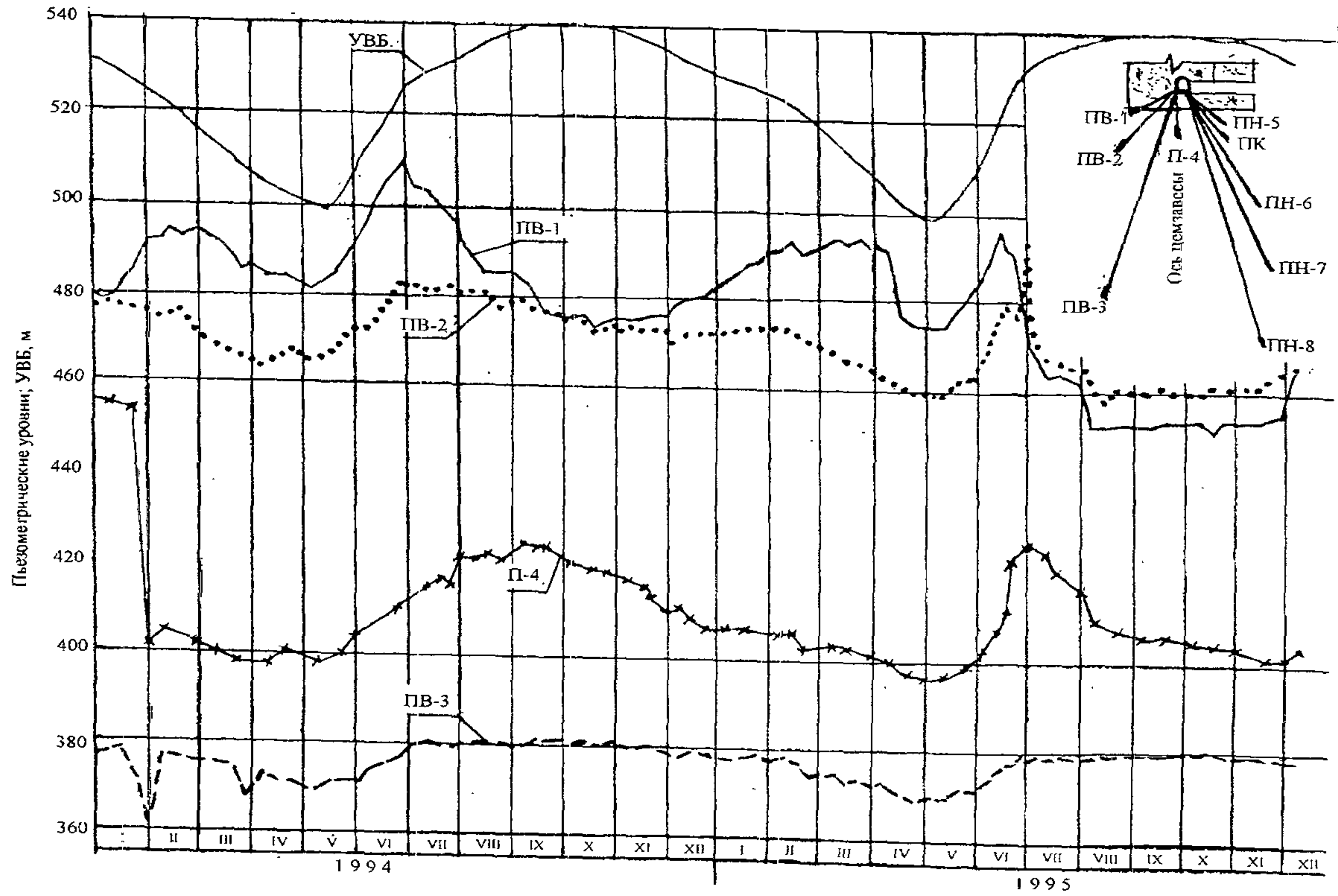
Рис. 1. Пьезометрические уровни в основании станционной секции 18.
