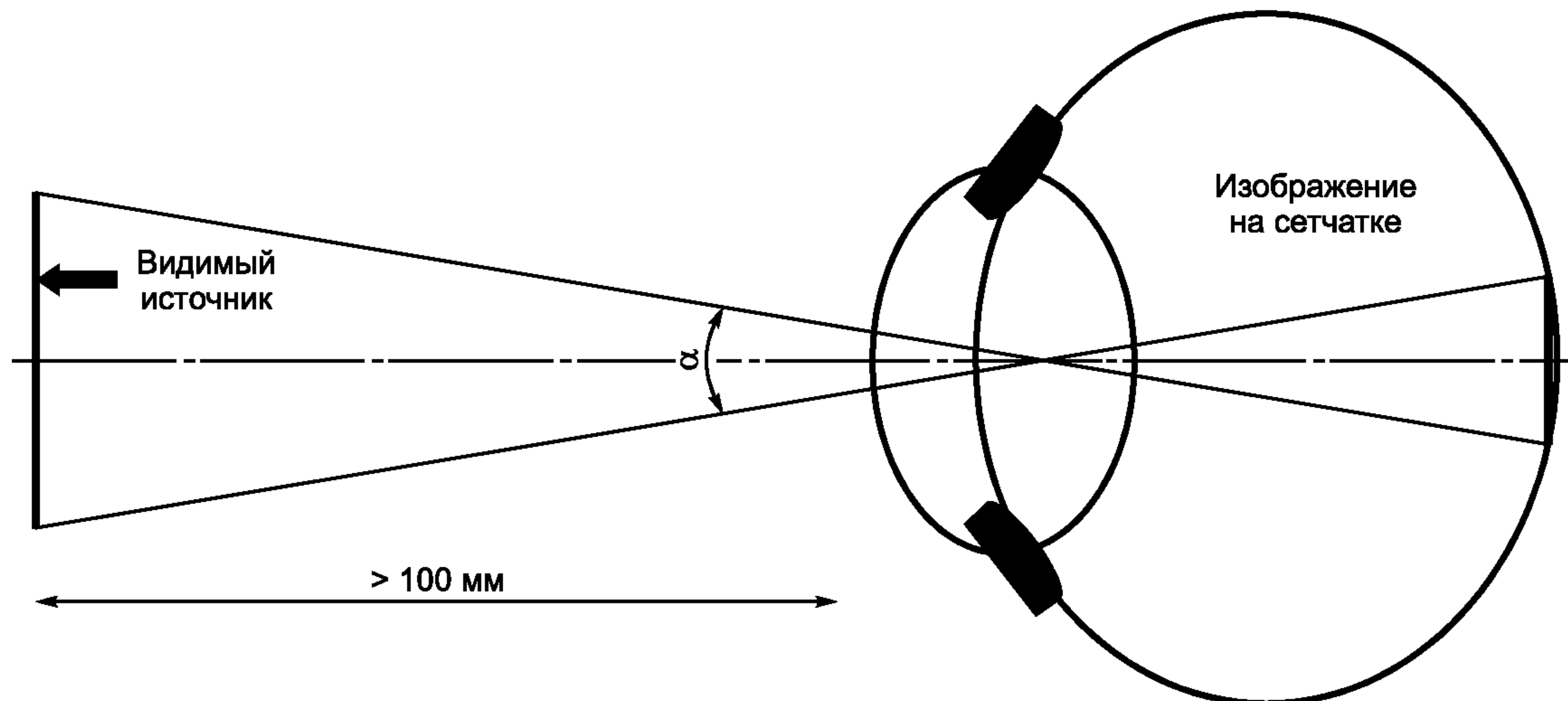
Рисунок 1 — Определение стягиваемого угла \alpha видимого размера источника
