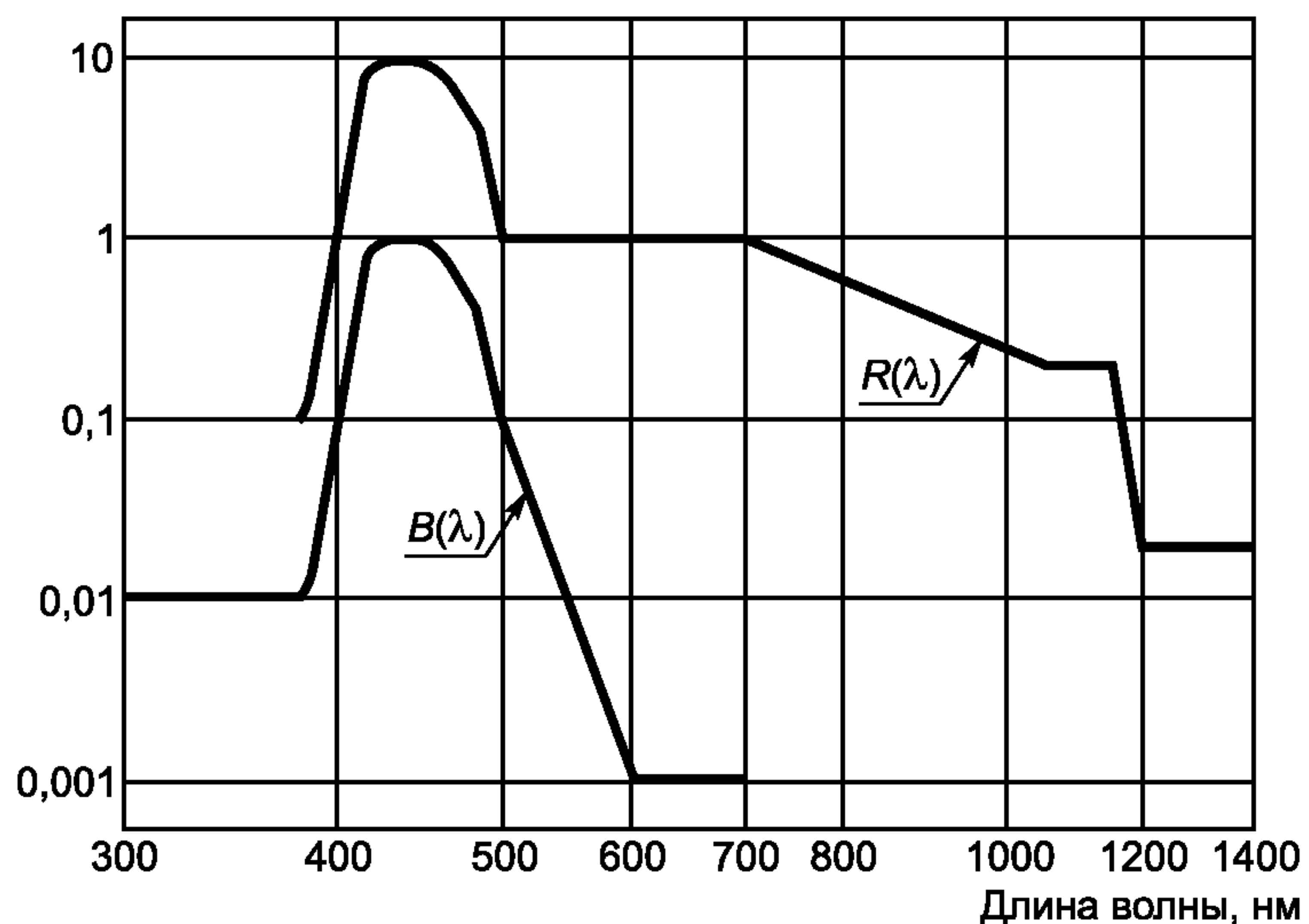
Рисунок 6 — Функция тепловой опасности клетчатки R(\lambda) и функция светло-голубой опасности клетчатки B(\lambda)
