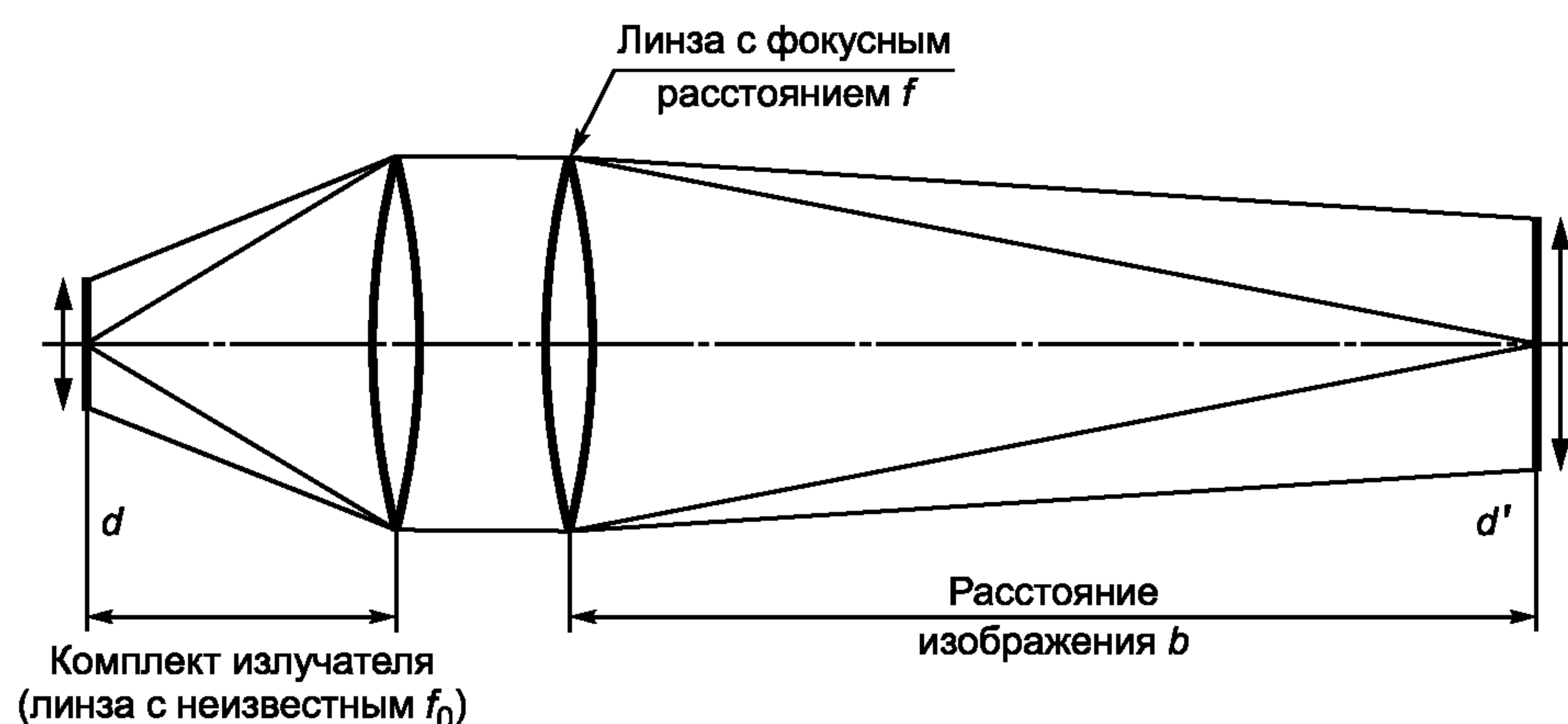
Рисунок 10 — Определение угла стягивания источника
