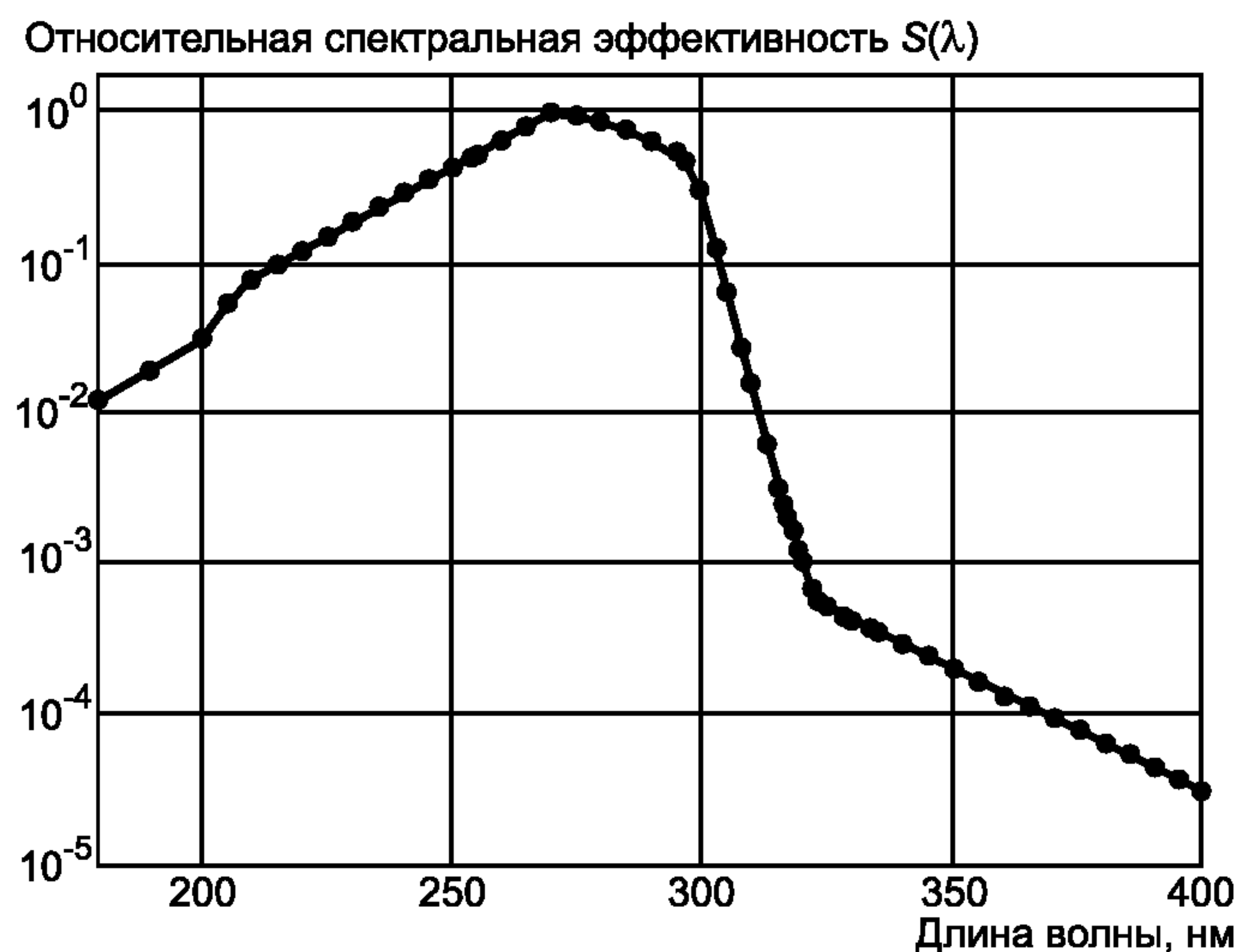
Рисунок 5 — Относительная спектральная эффективность S(\lambda)
