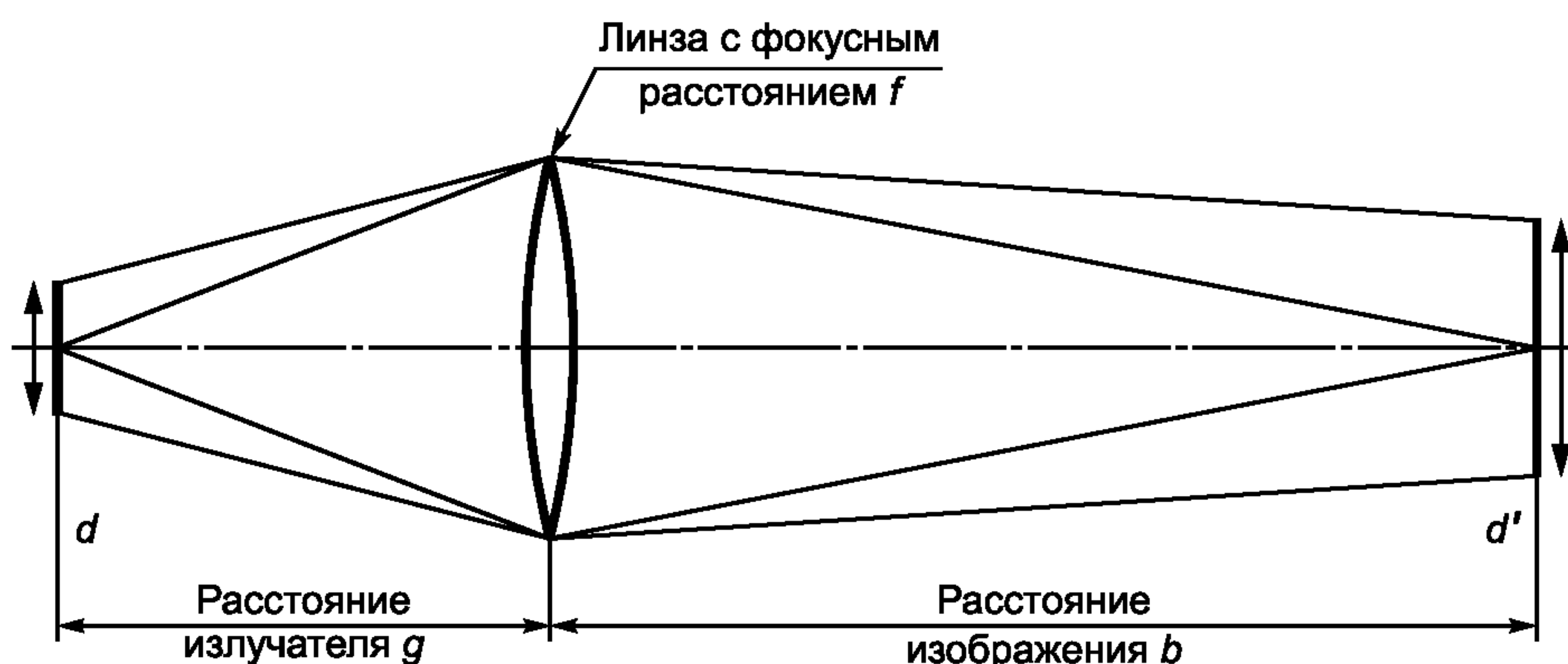
Рисунок 9 — Определение угла стягивания источника
