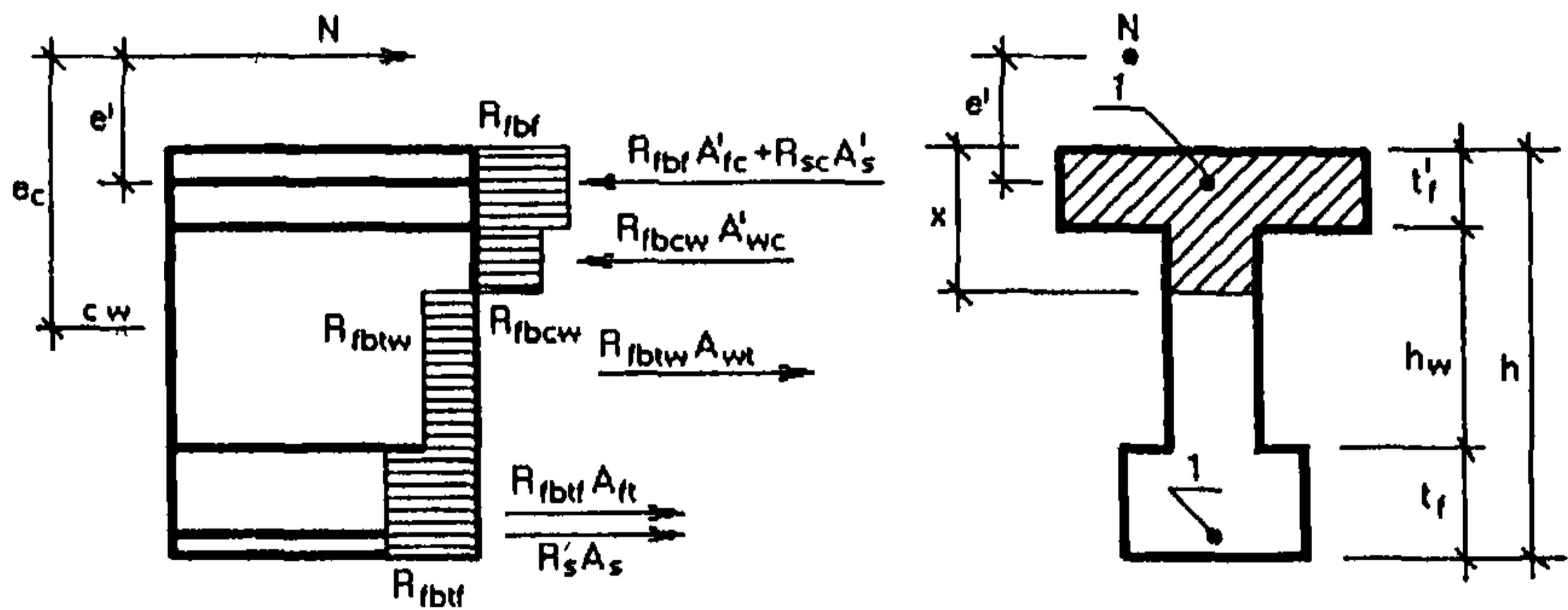
Рис. 6. Схема усилий и эпюра напряжений во внецентренно сжатых элементах двутаврового сечения при комбинированном армировании и x \leq t_f
