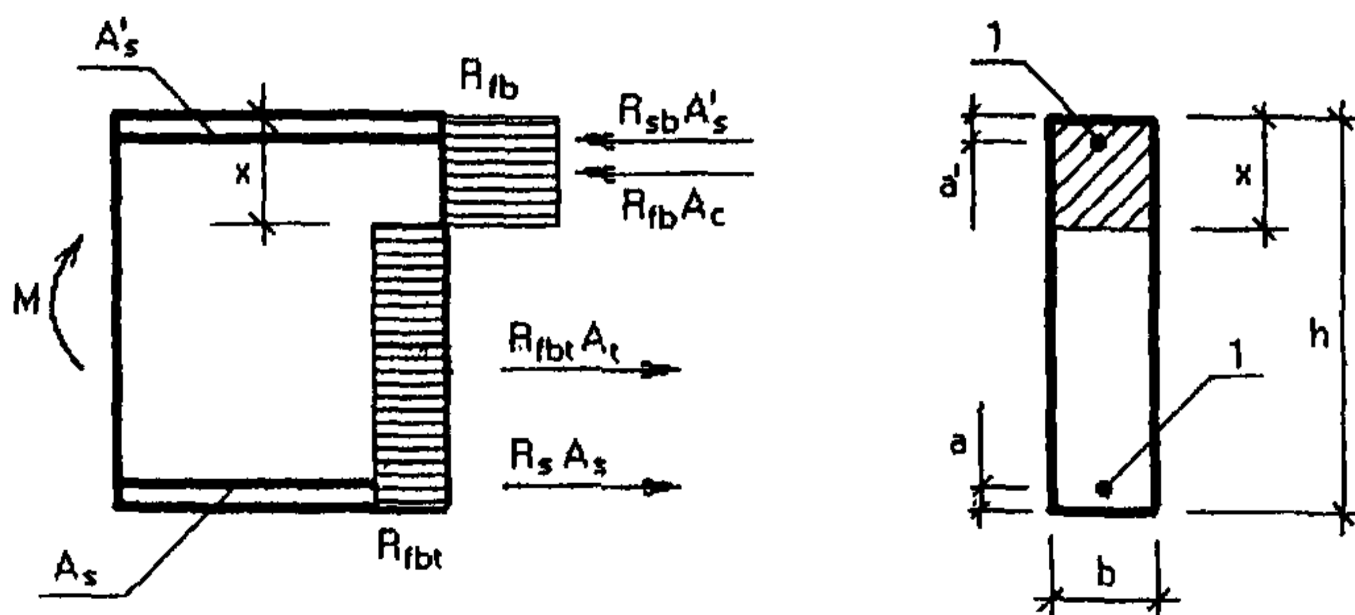
Рис. 3. Схема усилий и эпюра напряжений в сечениях, нормальных к продольной оси изгибаемого железобетонного элемента прямоугольного сечения при комбинированном армировании 1 – стержневая или проволочная арматура
