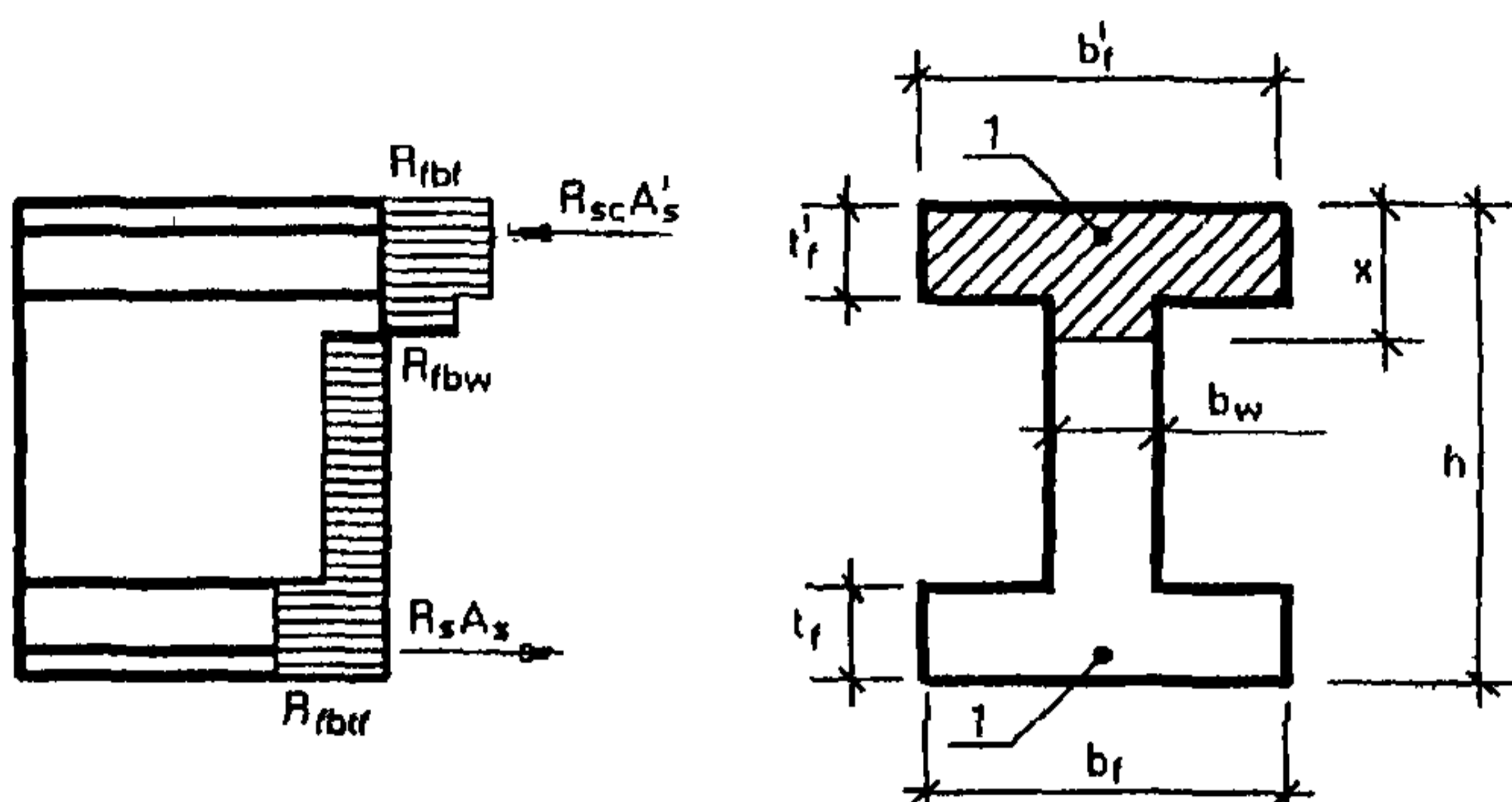
Рис. 1. Схема внутренних усилий и эпюры напряжений в сечении, нормальном к продольной оси элемента (общий случай) 1 – сосредоточенная стержневая или проволочная арматура
