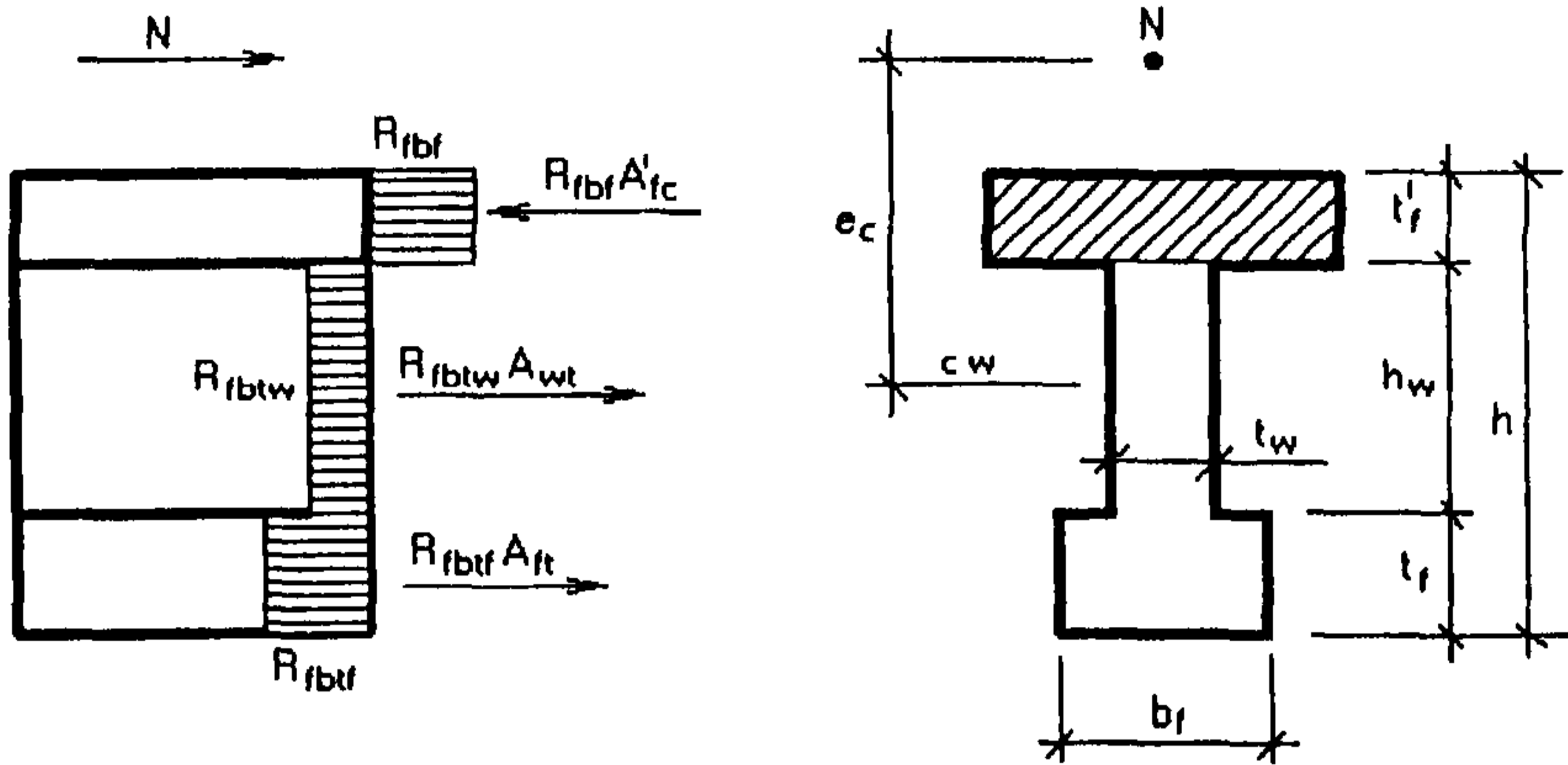
Рис. 5. Схема усилий и эпюра напряжений во внецентренно сжатых элементах двутаврового сечения при фибровом армировании
