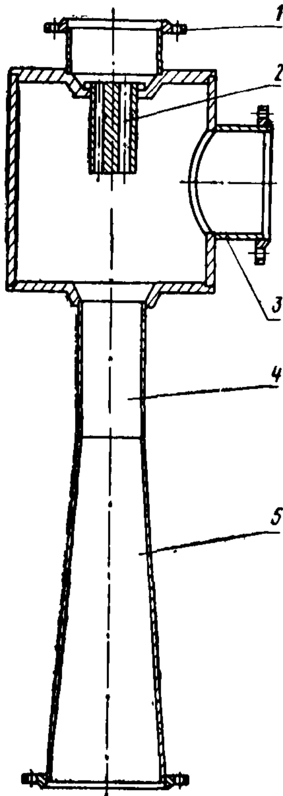
Водоструйный эжектор системы ЦКТИ
