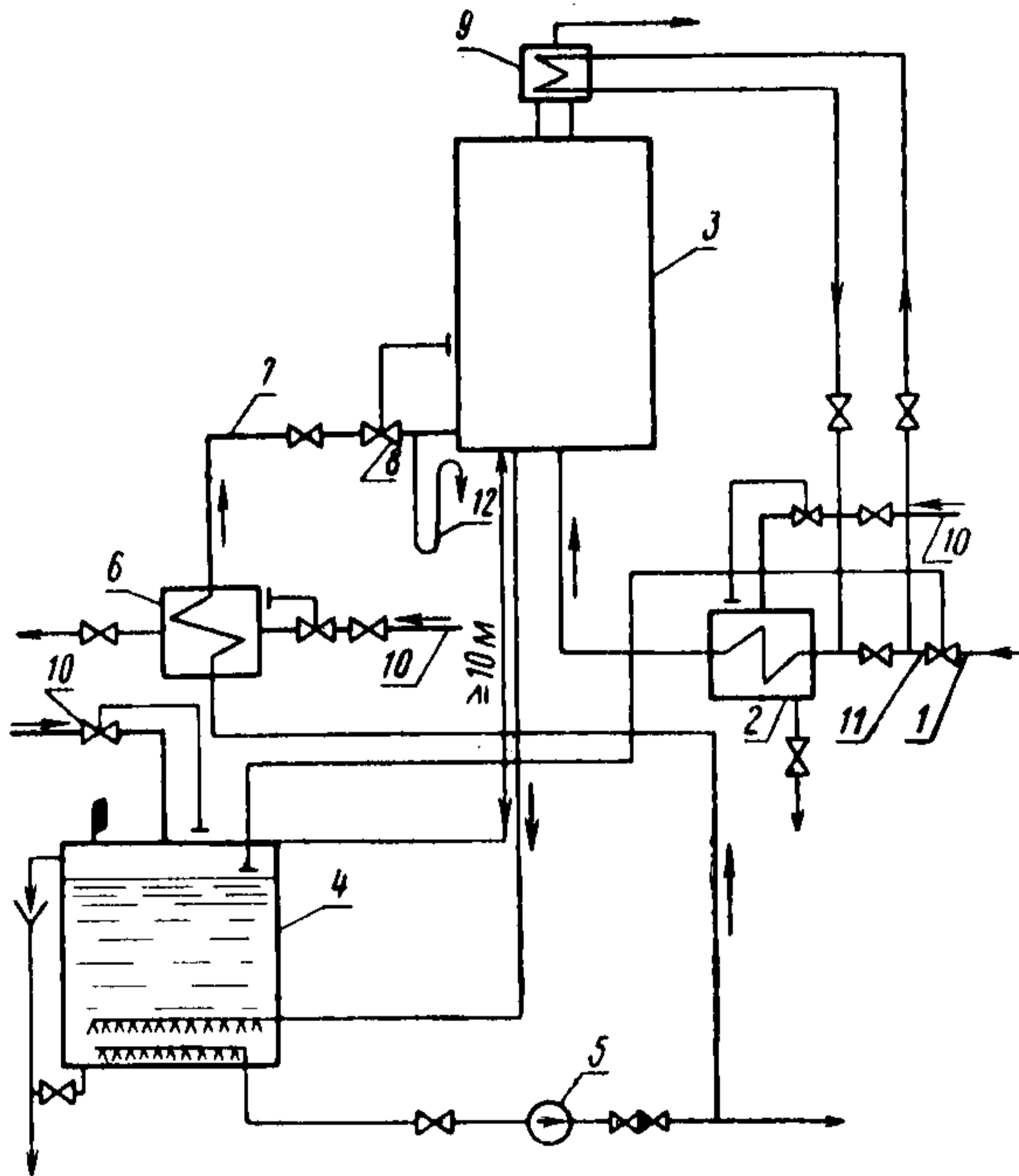
Схема включения вакуумных деаэраторов без потери конденсата
