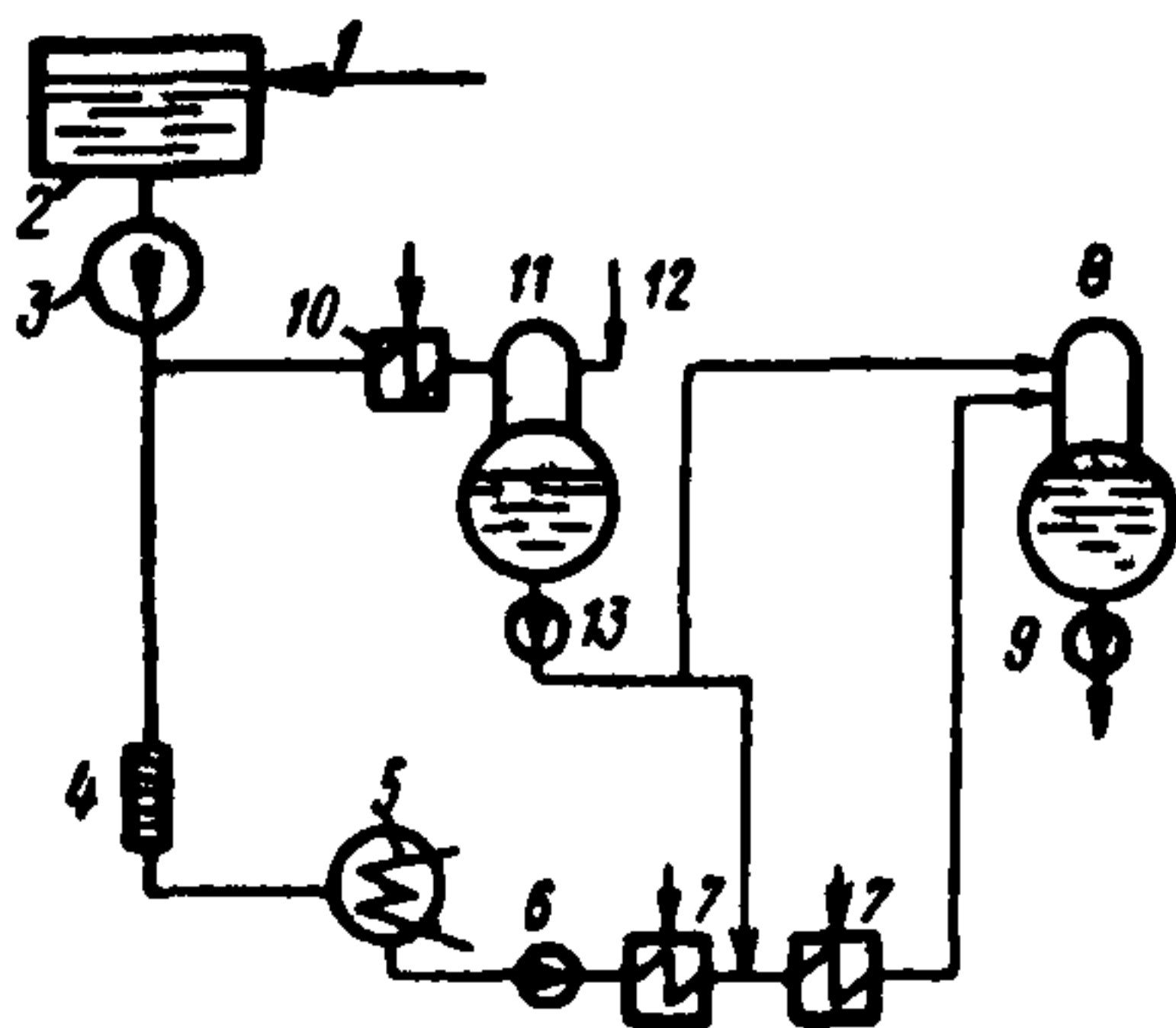
Двухступенчатая схема деаэрации воды
