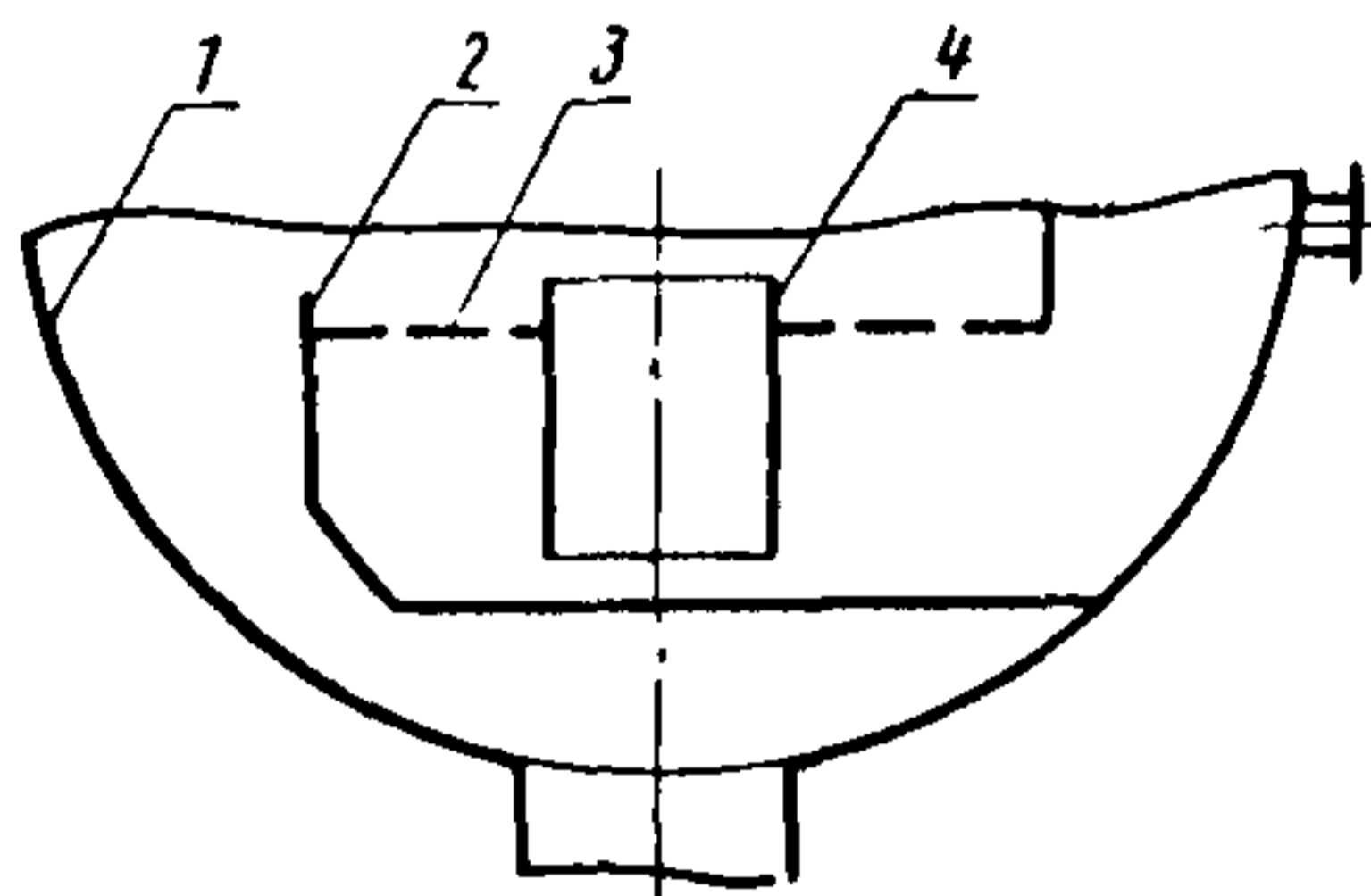
Барботажное устройство горизонтальных колонок ЦКТИ — БКЗ — СЗЭМ
