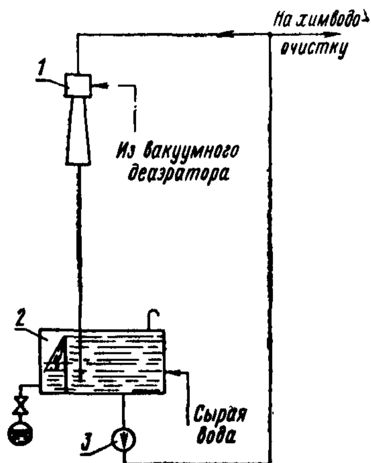
Разомкнутая схема включения водоструйного эжектора
