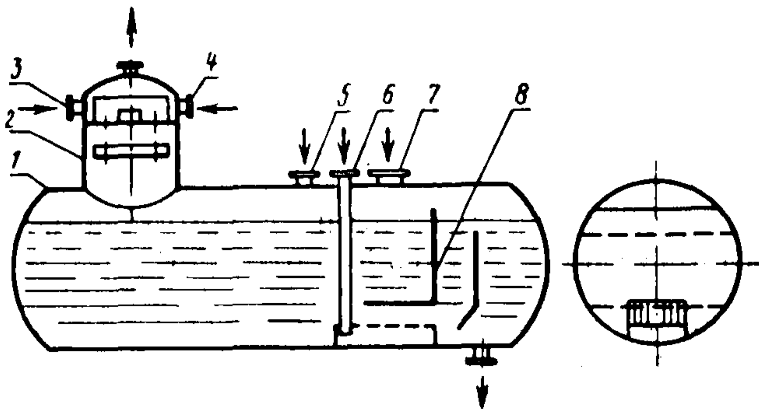
Двухступенчатый термический деаэратор системы ЦКТИ
