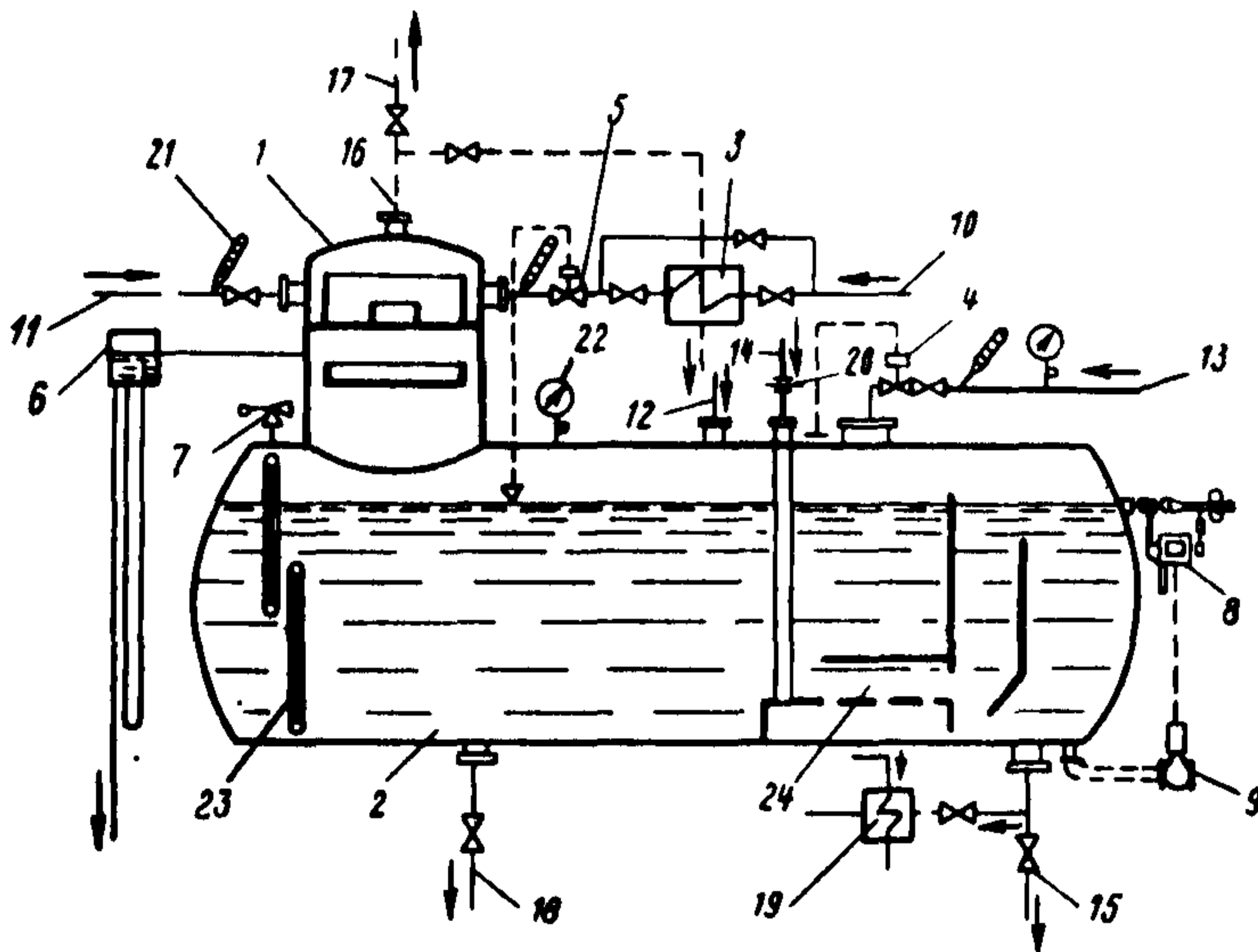
Принципиальная схема двухступенчатой деаэрационной установки системы ЦКТИ
