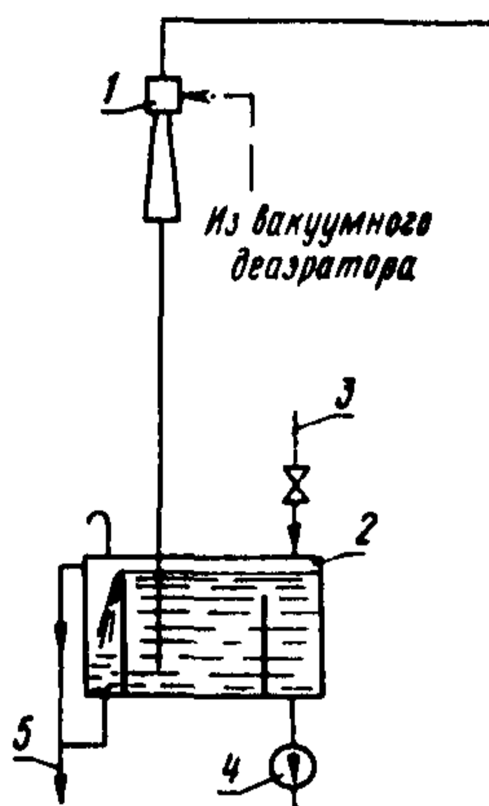
Замкнутая схема включения водоструйного эжектора
