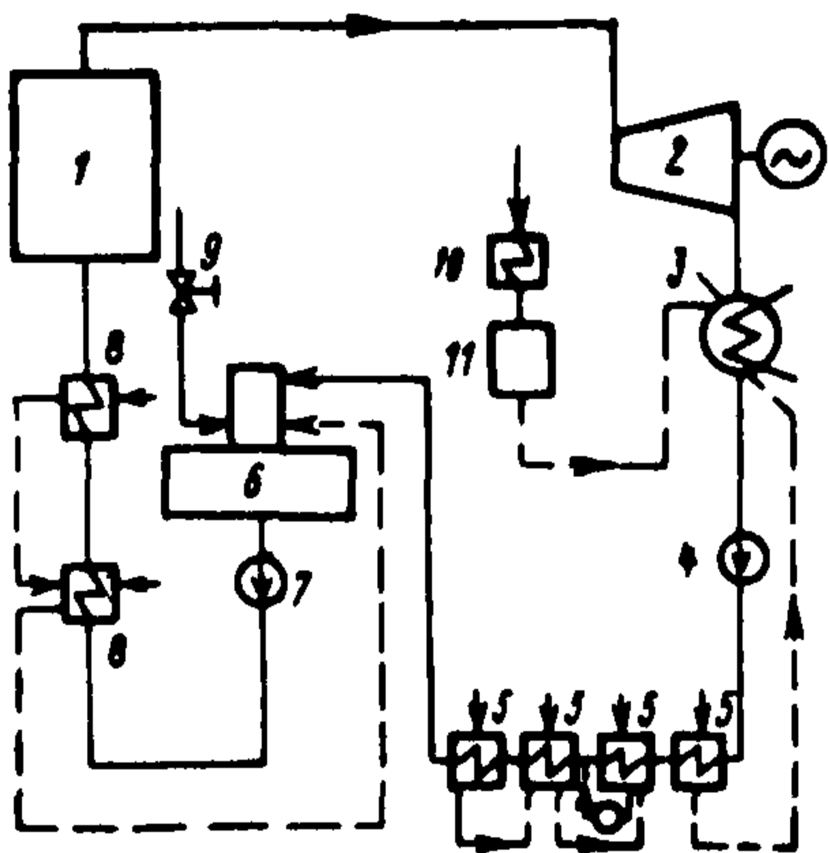
Одноступенчатая схема деаэрации воды
