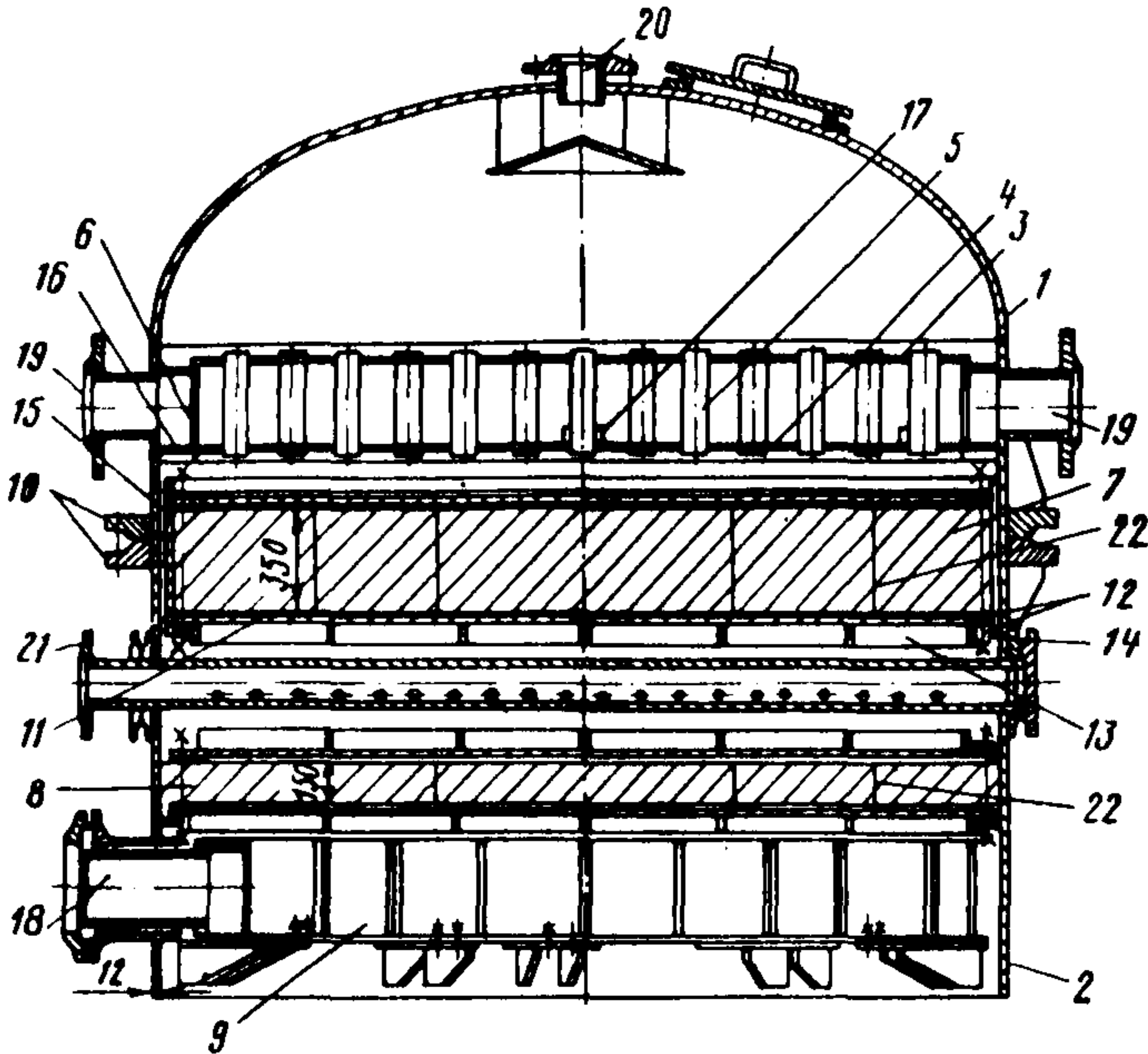
Схема колонки с неупорядоченной насадкой
