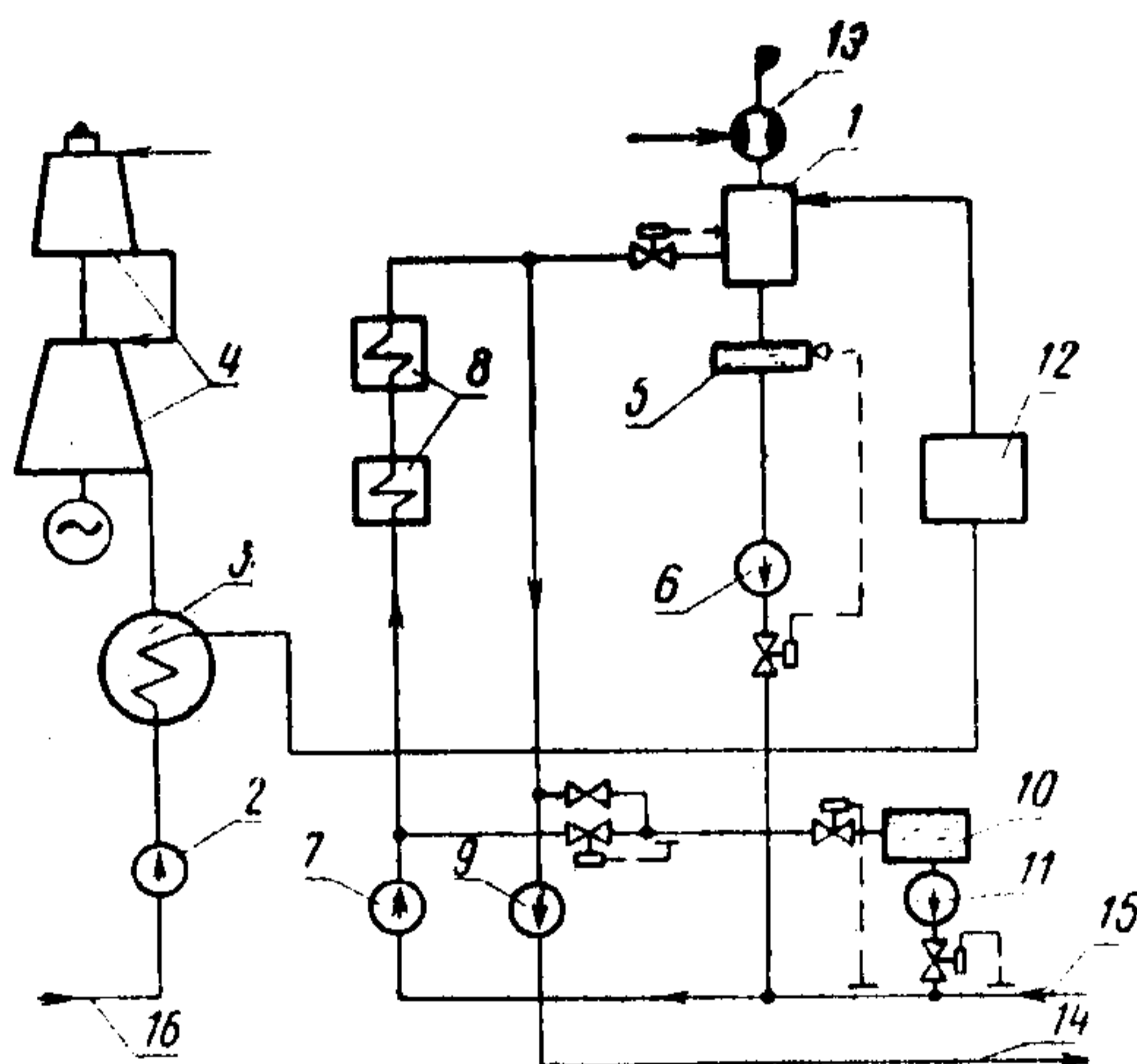
Включение вакуумных деаэраторов подпиточной воды в схему отопительно-производственной ТЭЦ
