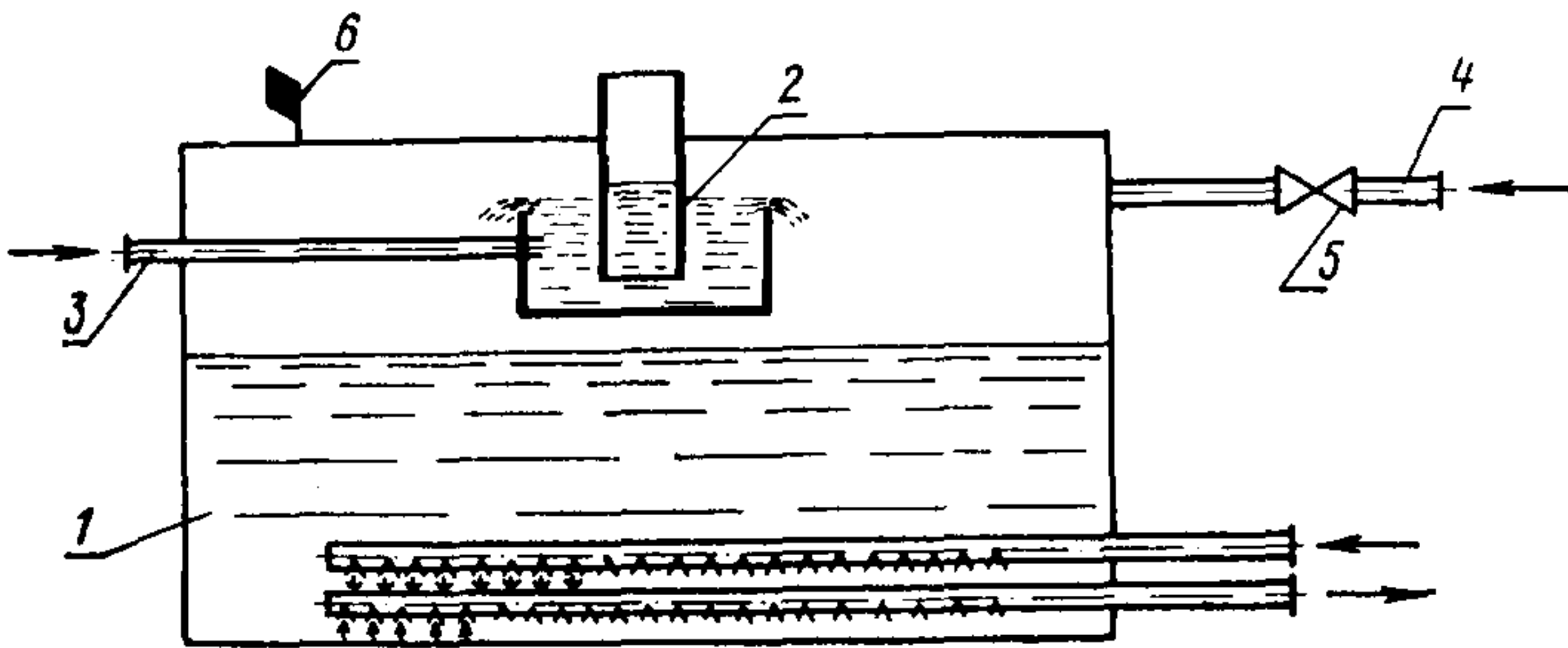
Гидравлический затвор для защиты баков-аккумуляторов
