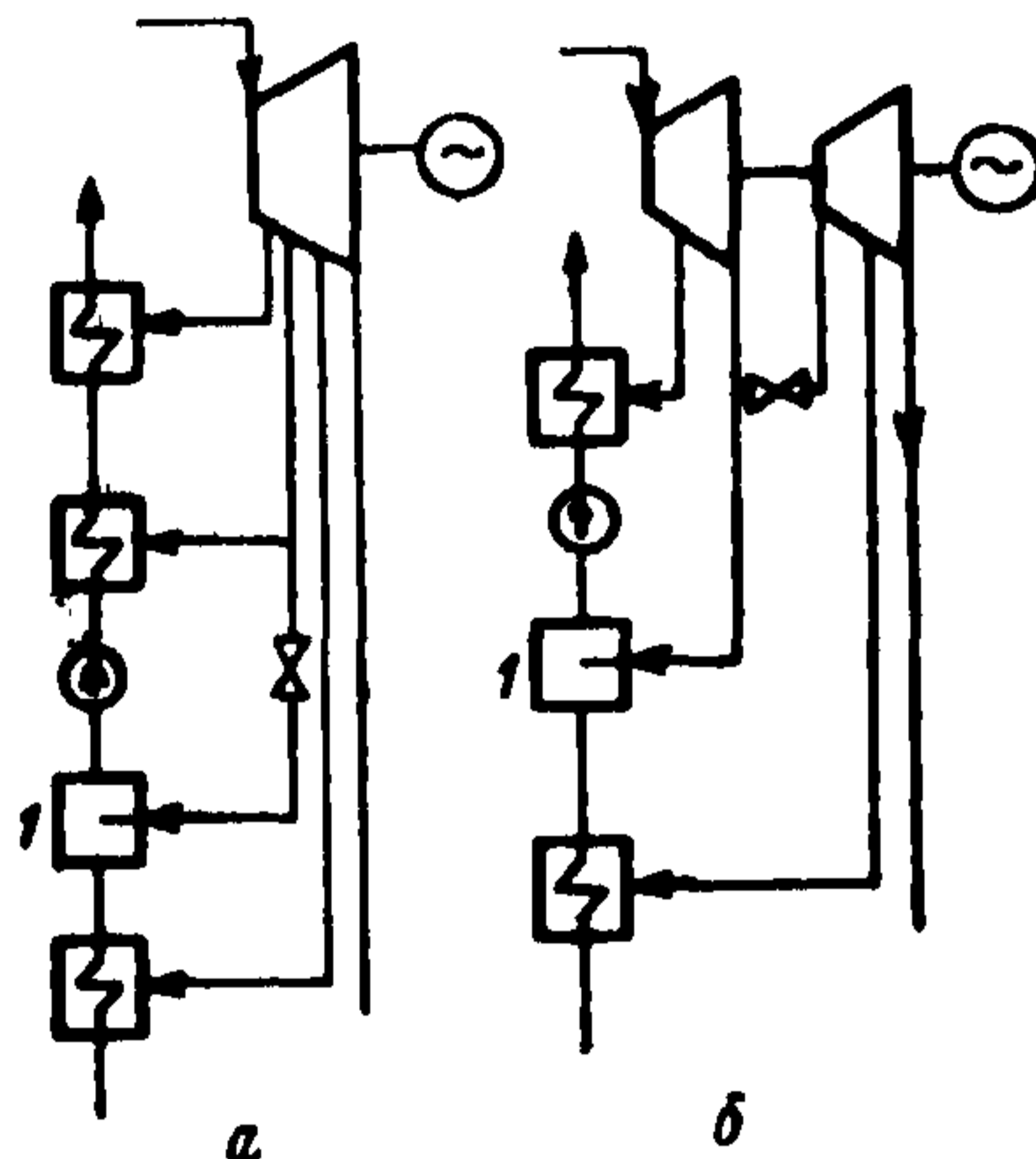
Включение деаэратора в тепловую схему турбоагрегата
