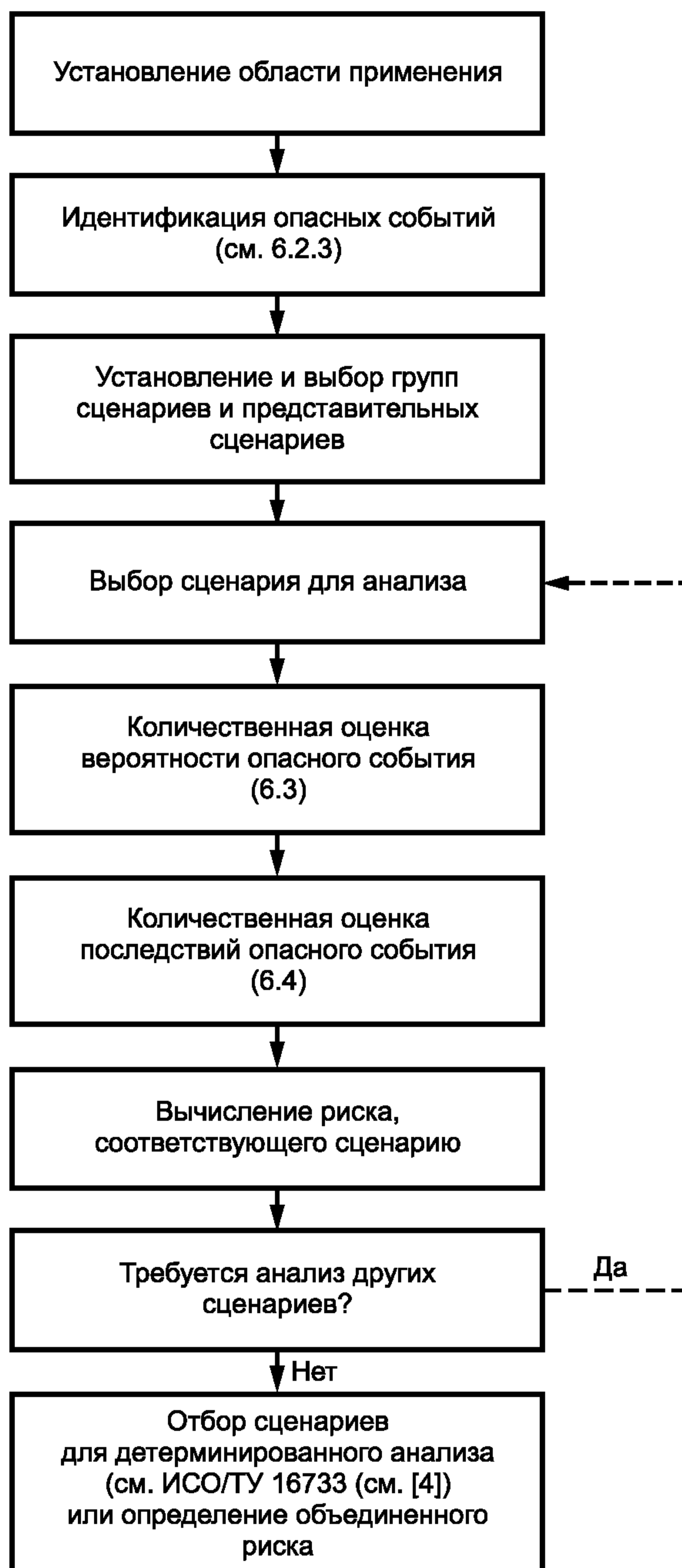
Рисунок 2 — Схема оценки пожарного риска
