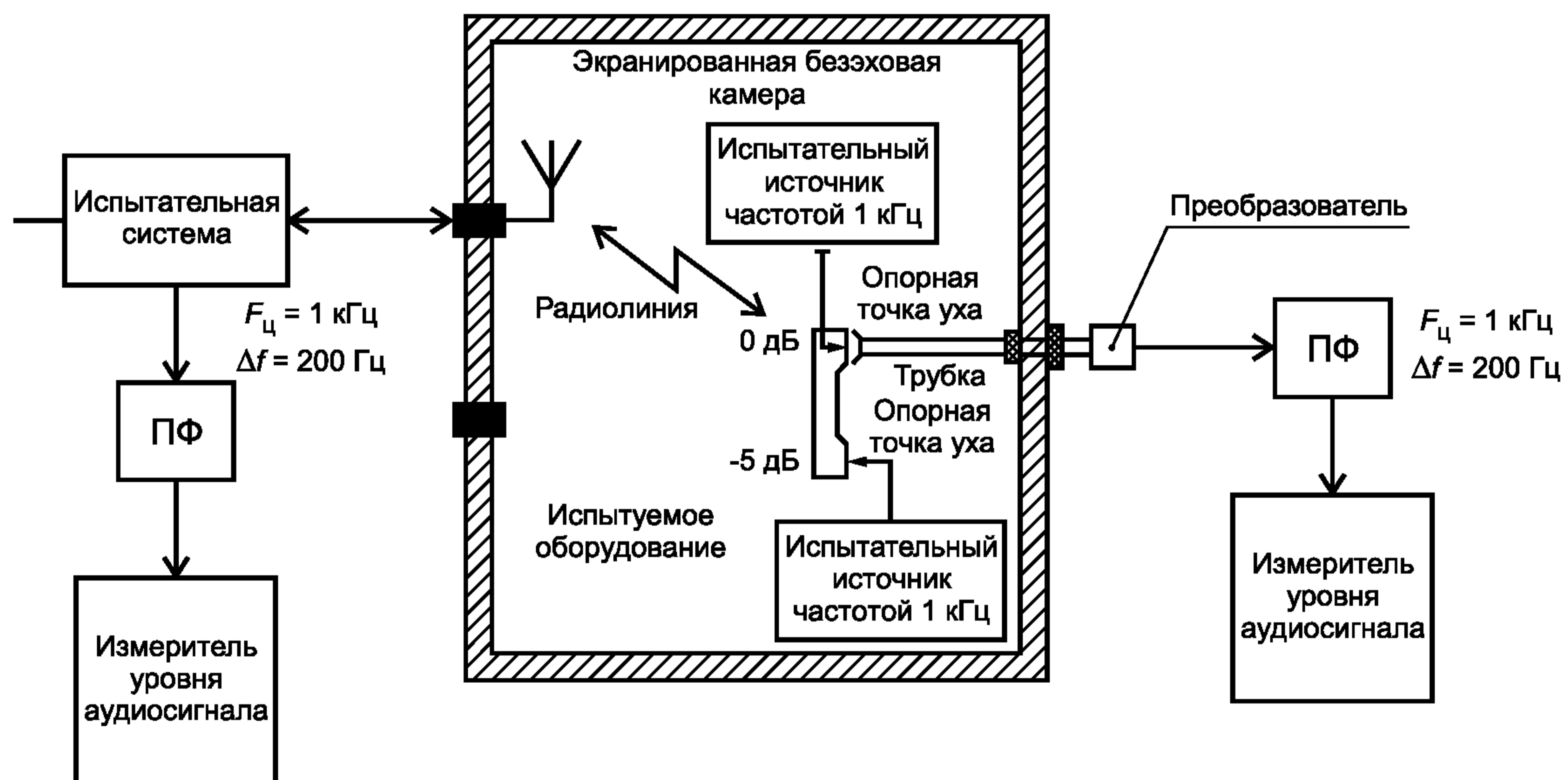
Рисунок 1 — Схема прохождения сигнала при испытаниях
