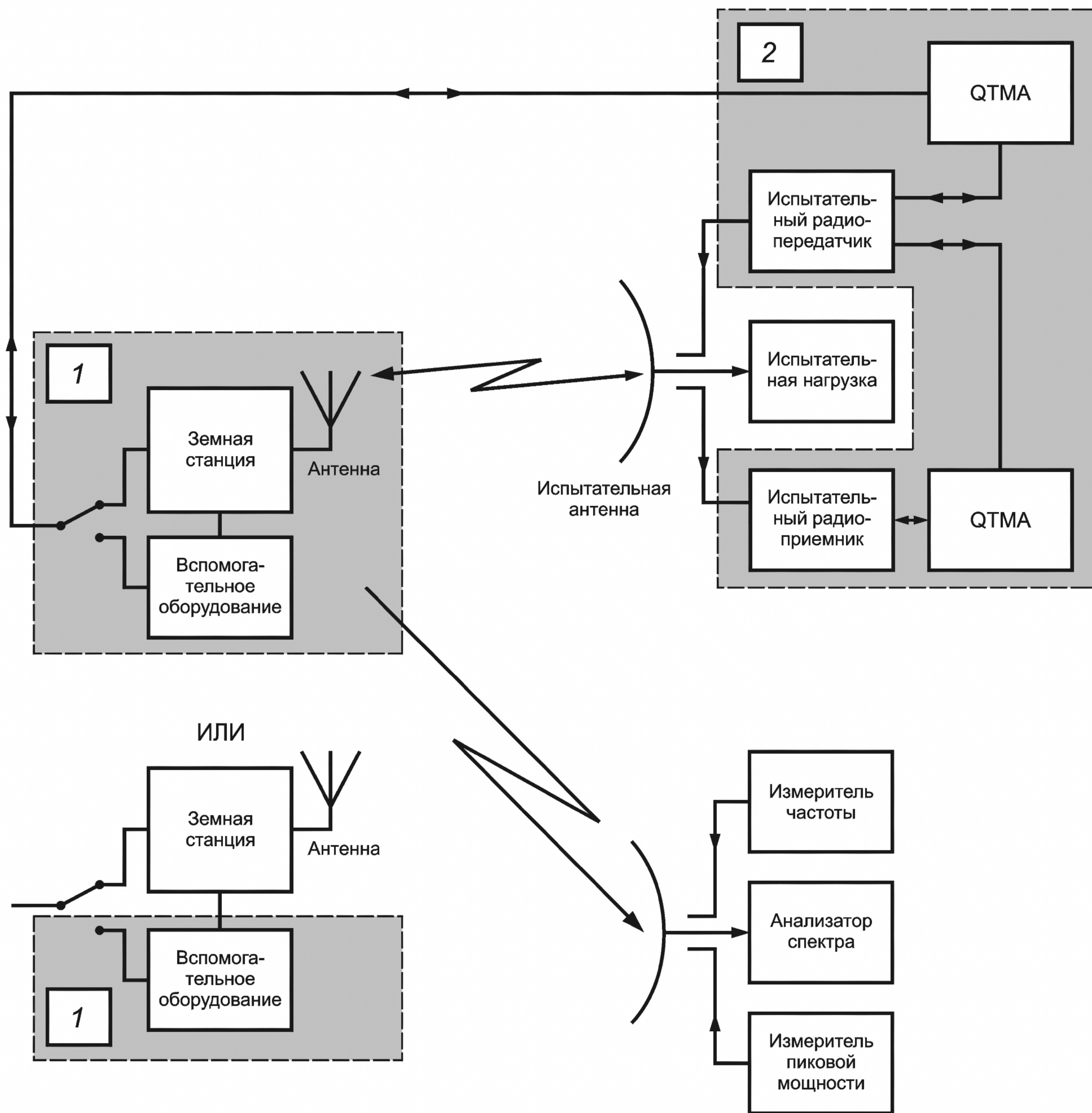
1 — испытуемое оборудование; 2 — испытательная система; QTMA — приборы для измерения параметров качества передачи
