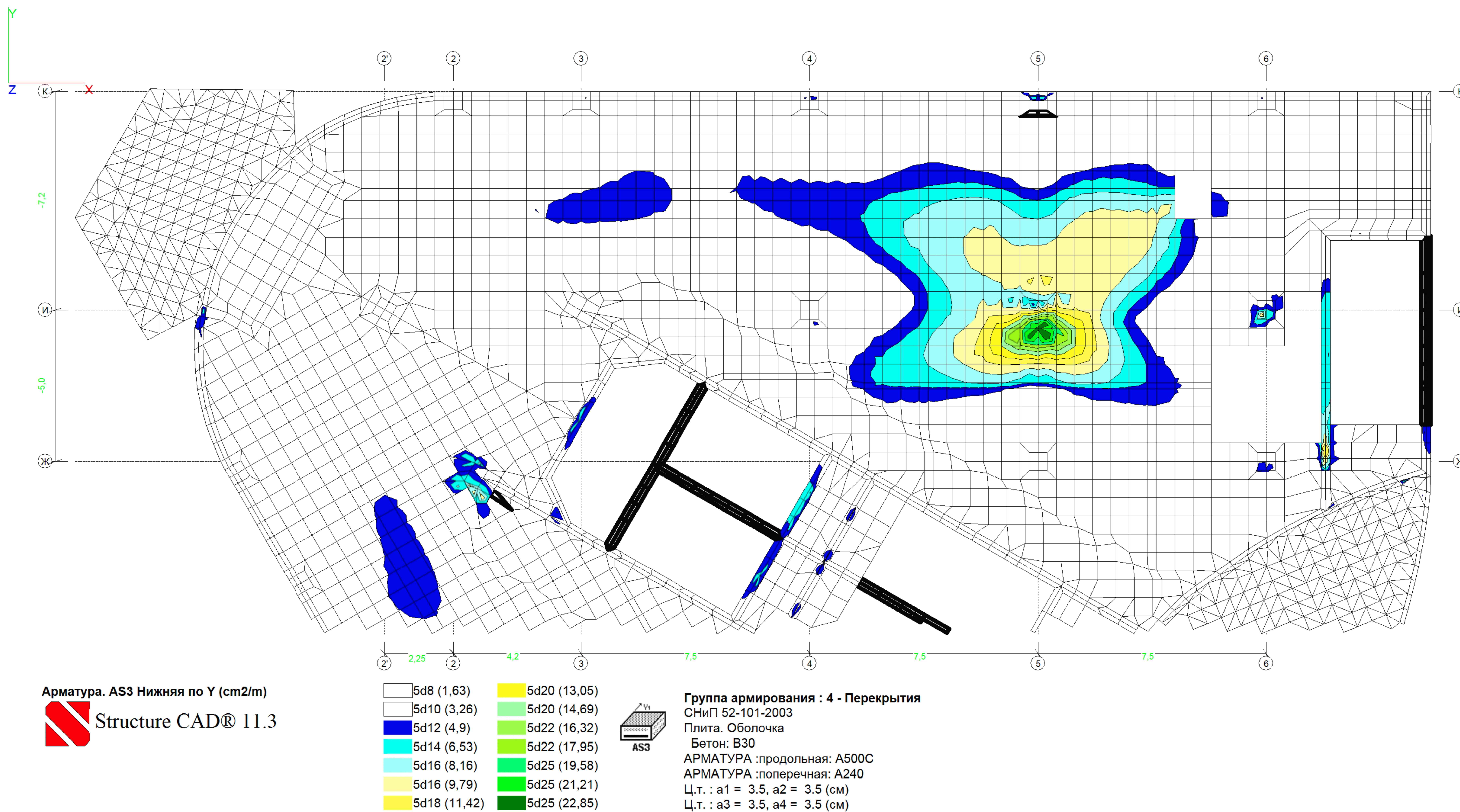
Рис. 8. Армирование перекрытия на отм. 4.500 при удалении на отм. 0.000 колонны №14 на нагрузку 0,71 тс/м 2 . Нижняя арматура вдоль цифровых осей.
