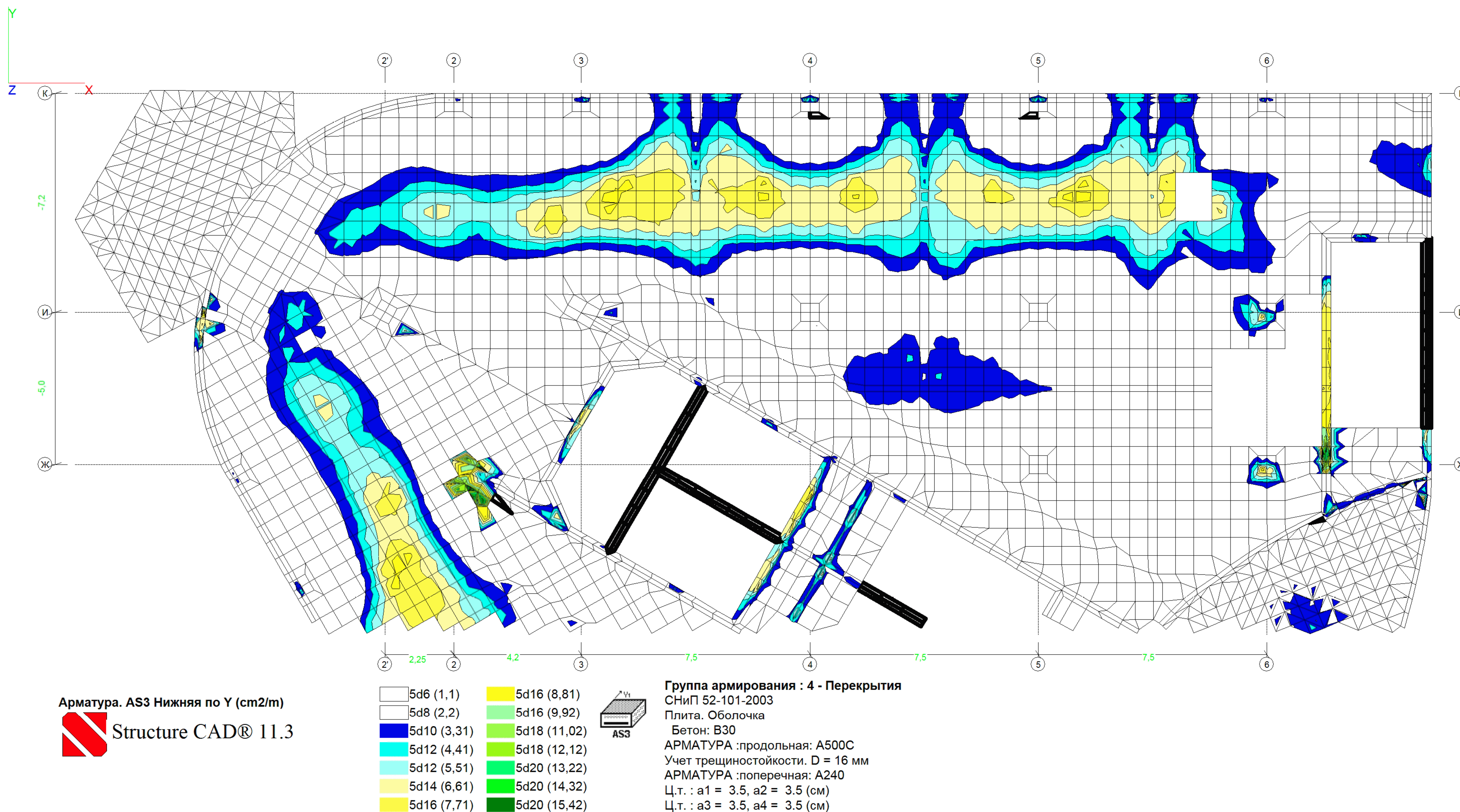
Рис. 6. Армирование перекрытия на отм. 4.500 при первичной конструктивной системе на эксплуатационную расчетную нагрузку 1,07 тс/м 2 . Нижняя арматура вдоль цифровых осей.
