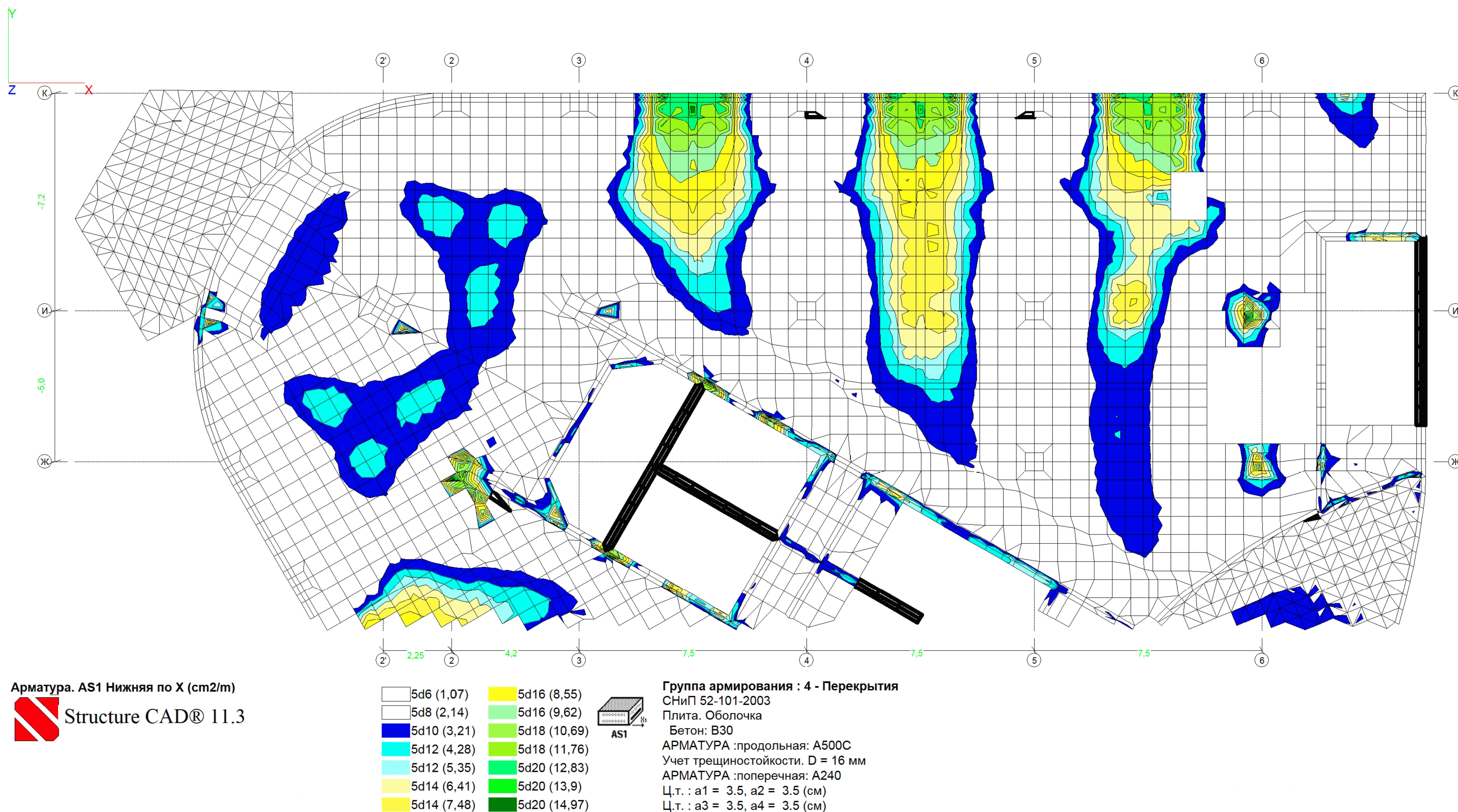
Рис. 5. Армирование перекрытия на отм. 4.500 при первичной конструктивной системе на эксплуатационную расчетную нагрузку 1,07 тс/м 2 . Нижняя арматура вдоль буквенных осей.
