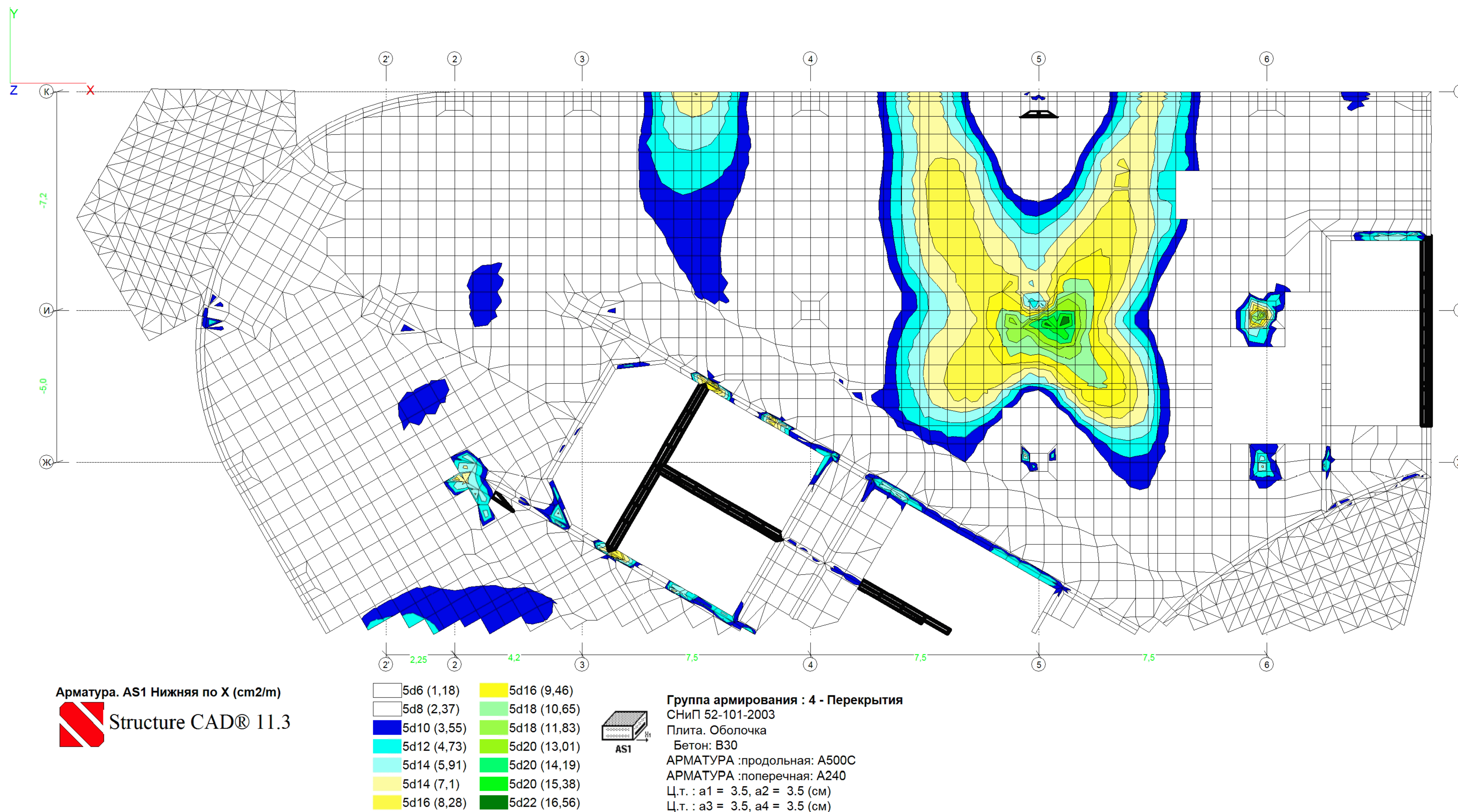
Рис. 7. Армирование перекрытия на отм. 4.500 при удалении на отм. 0.000 колонны №14 на нагрузку 0,71 тс/м 2 . Нижняя арматура вдоль буквенных осей.
