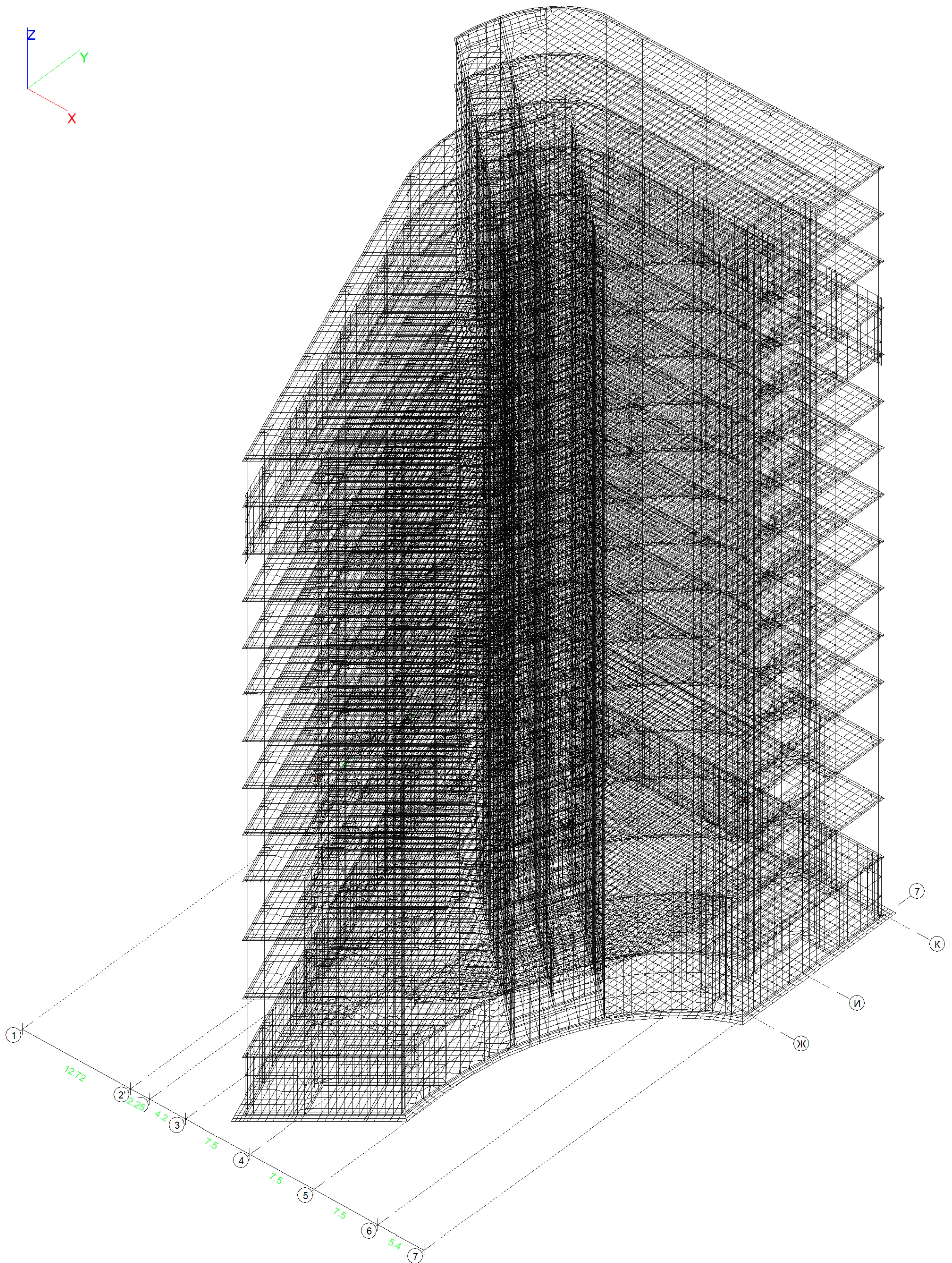
Рис.3. Расчетная схема каркаса здания.
