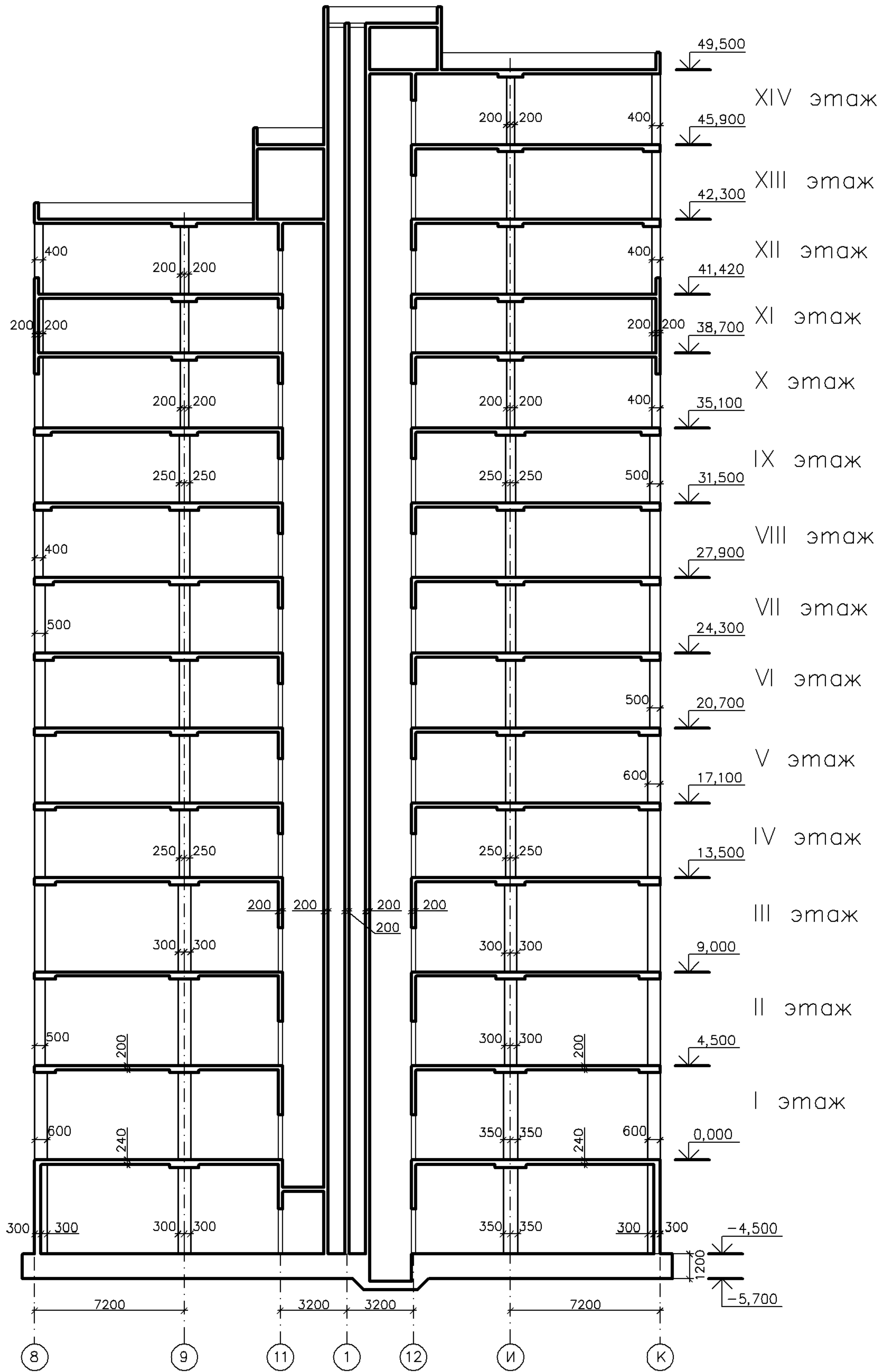
Рис.2. Разрез 1-1.
