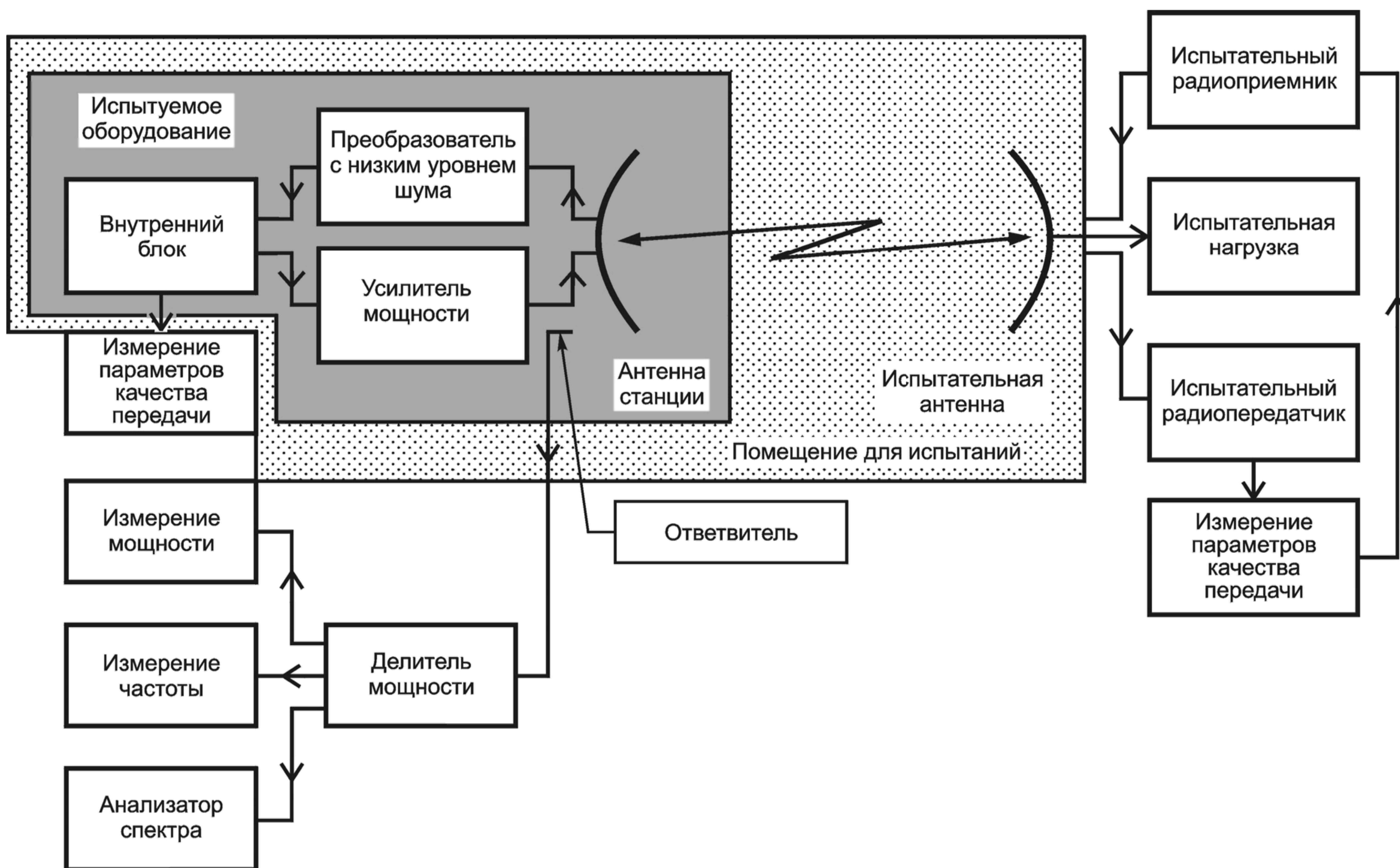
Рисунок 1 — Конфигурация оборудования при испытаниях
