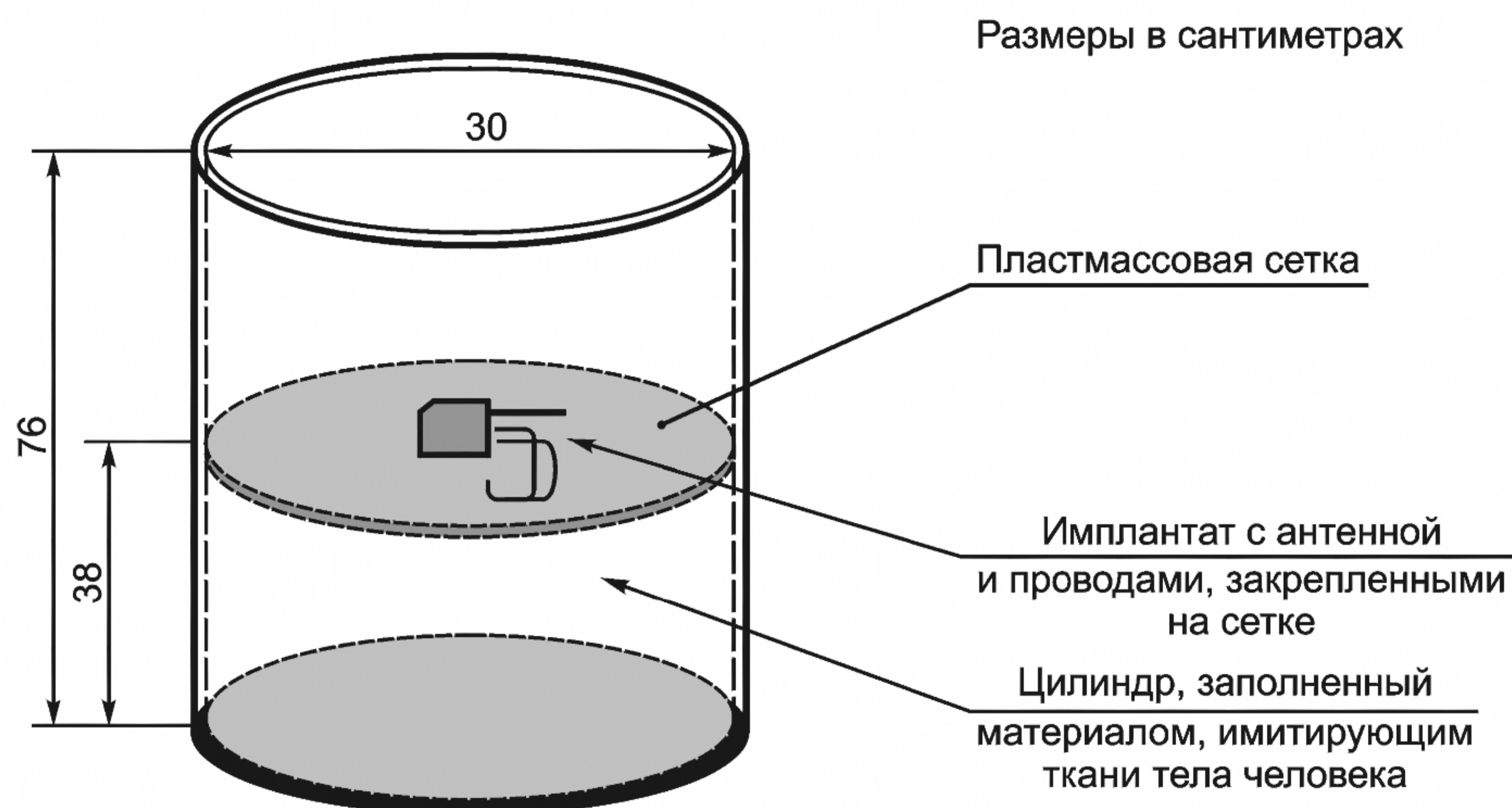
Рисунок В.1 — Эквивалент тела человека
