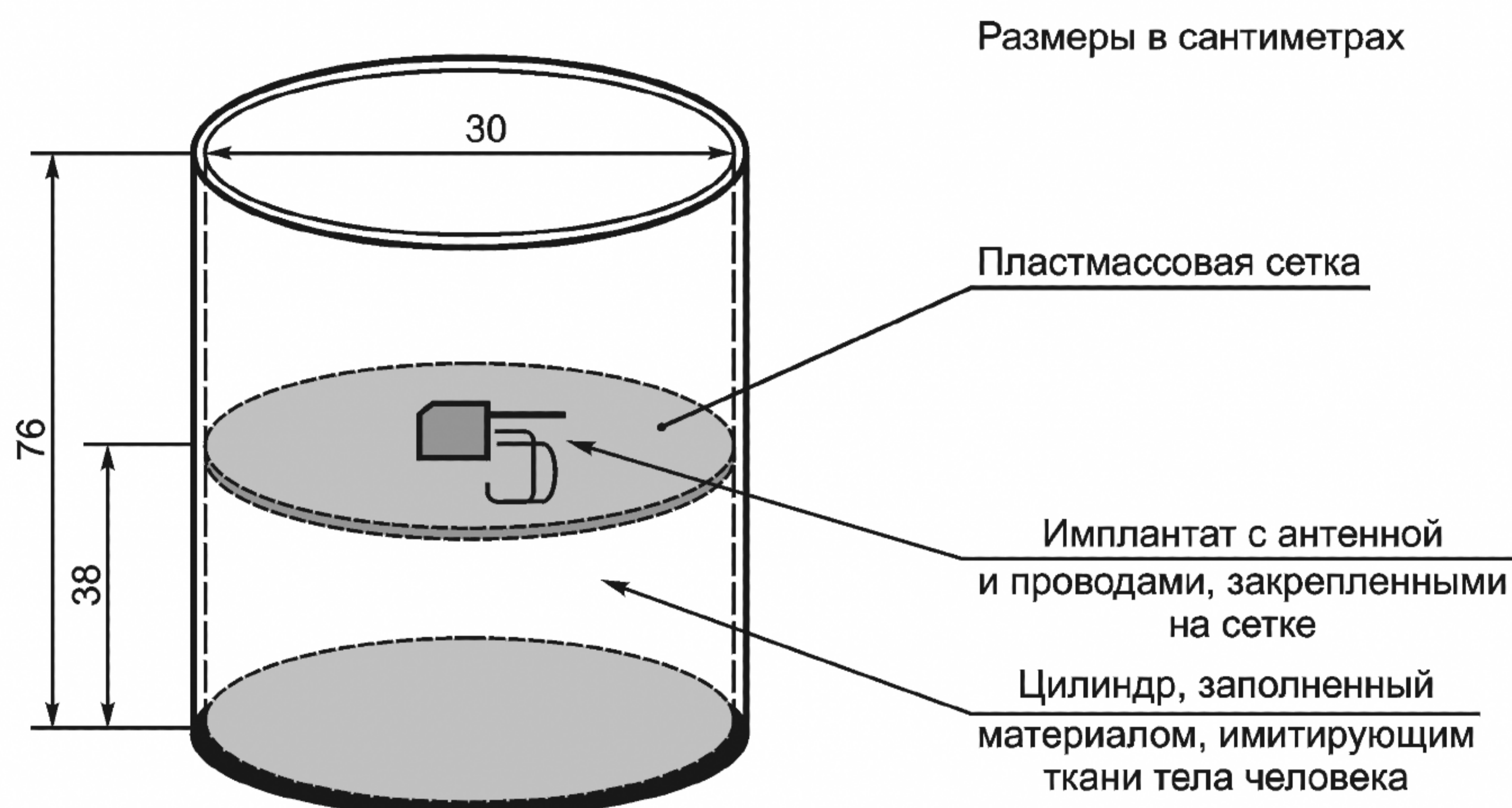
Рисунок В.1 — Эквивалент тела человека
