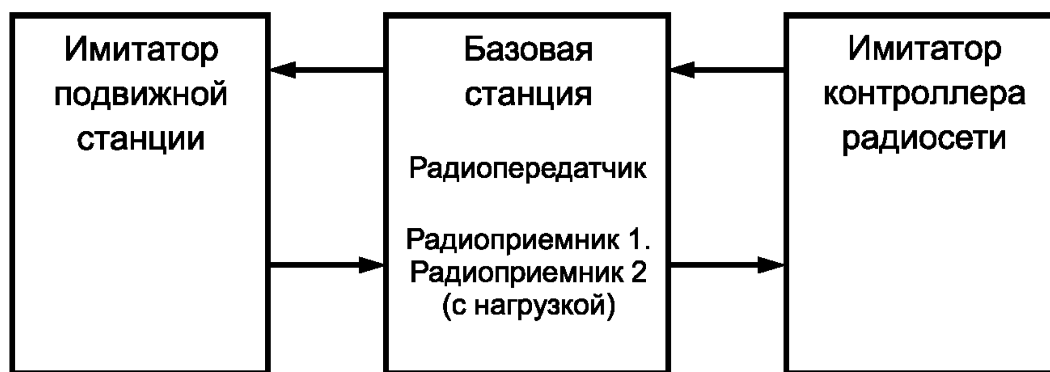
Рисунок 1 — Схема испытаний на помехоустойчивость базовой станции
