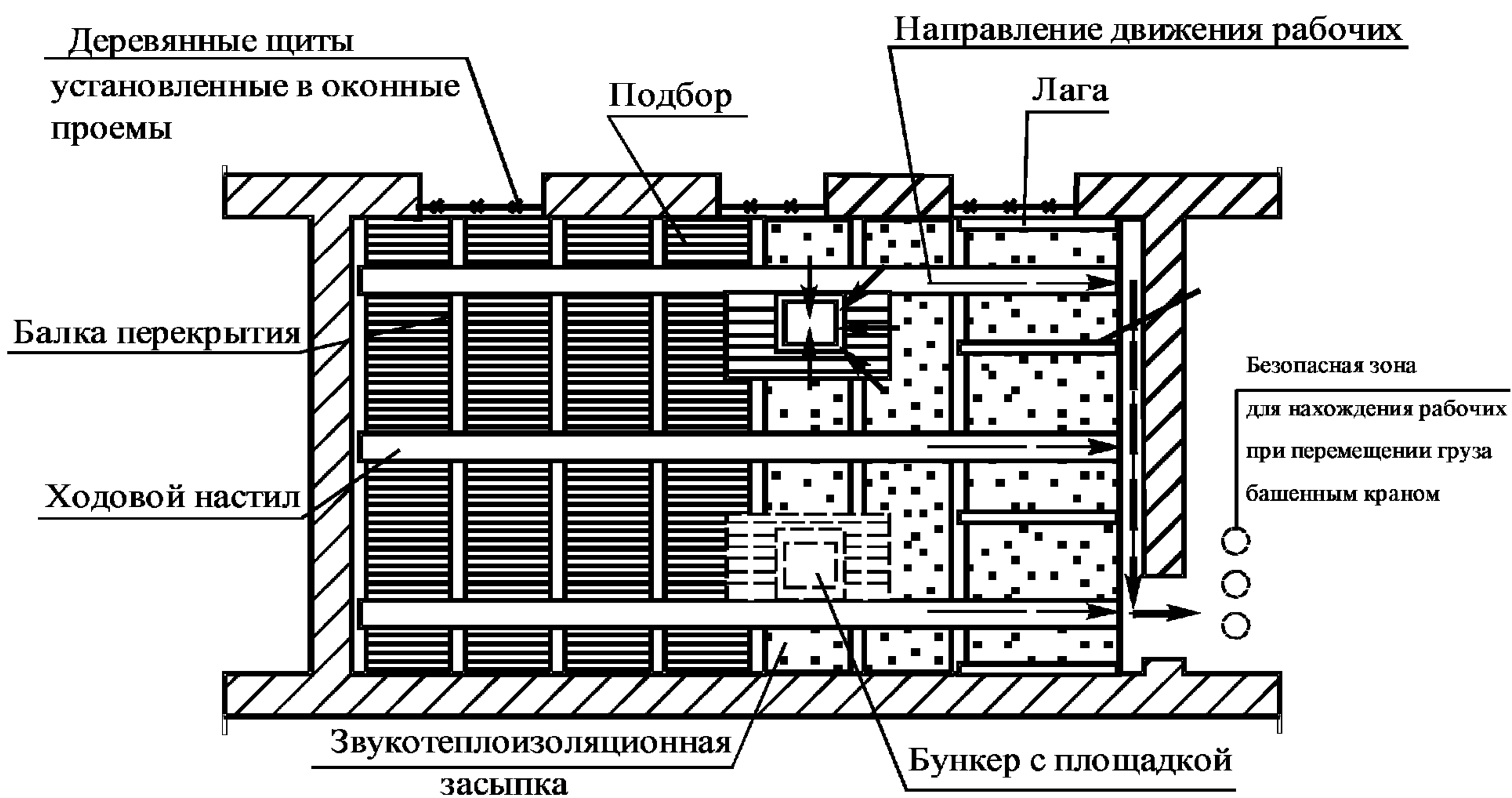
Рисунок 3 – Схема удаления звукотеплоизоляции (засыпки) перекрытия при использовании бункеров
