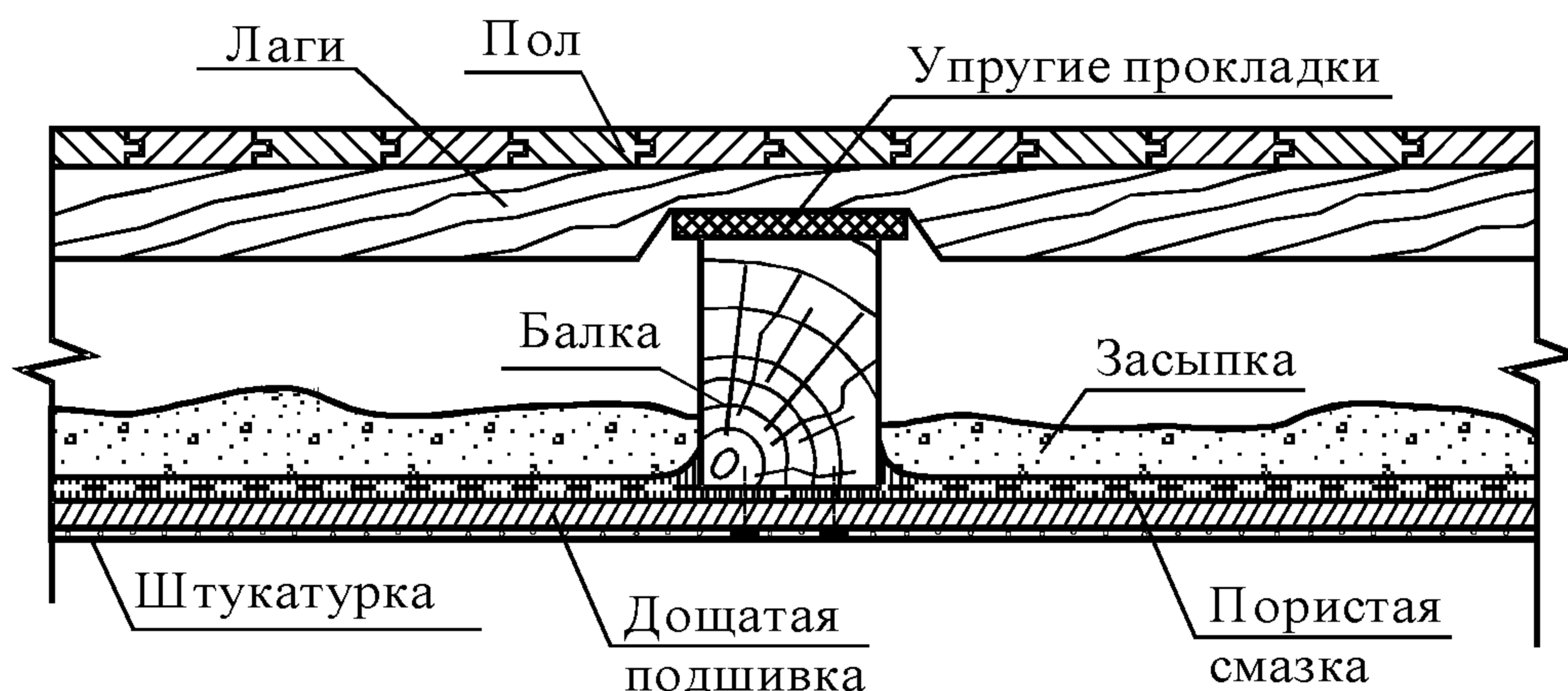
Рисунок 1 – Перекрытие по деревянным балкам с щитовым накатом
