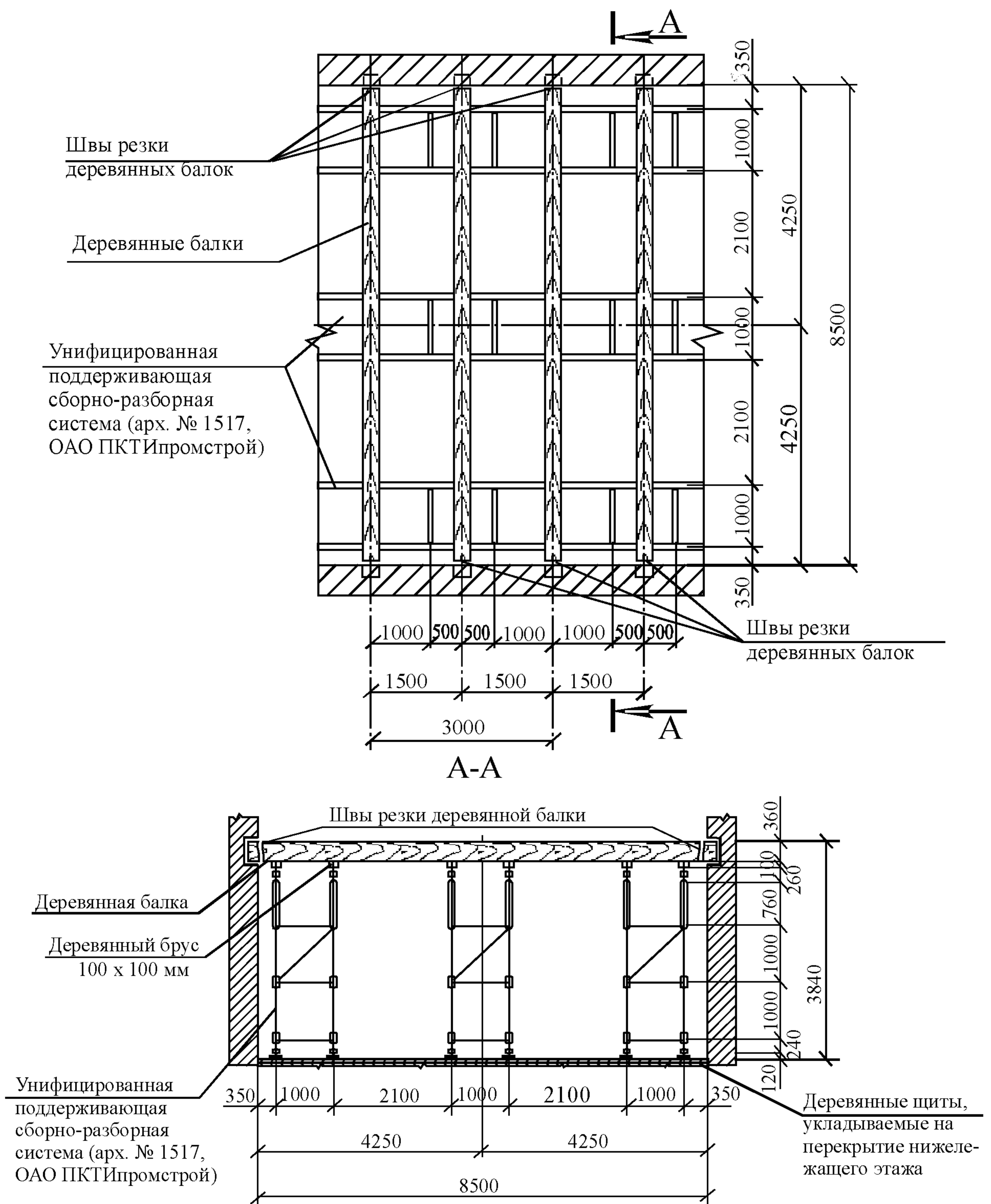
Рисунок 8 – Схема разборки междуэтажного перекрытия по деревянным балкам
