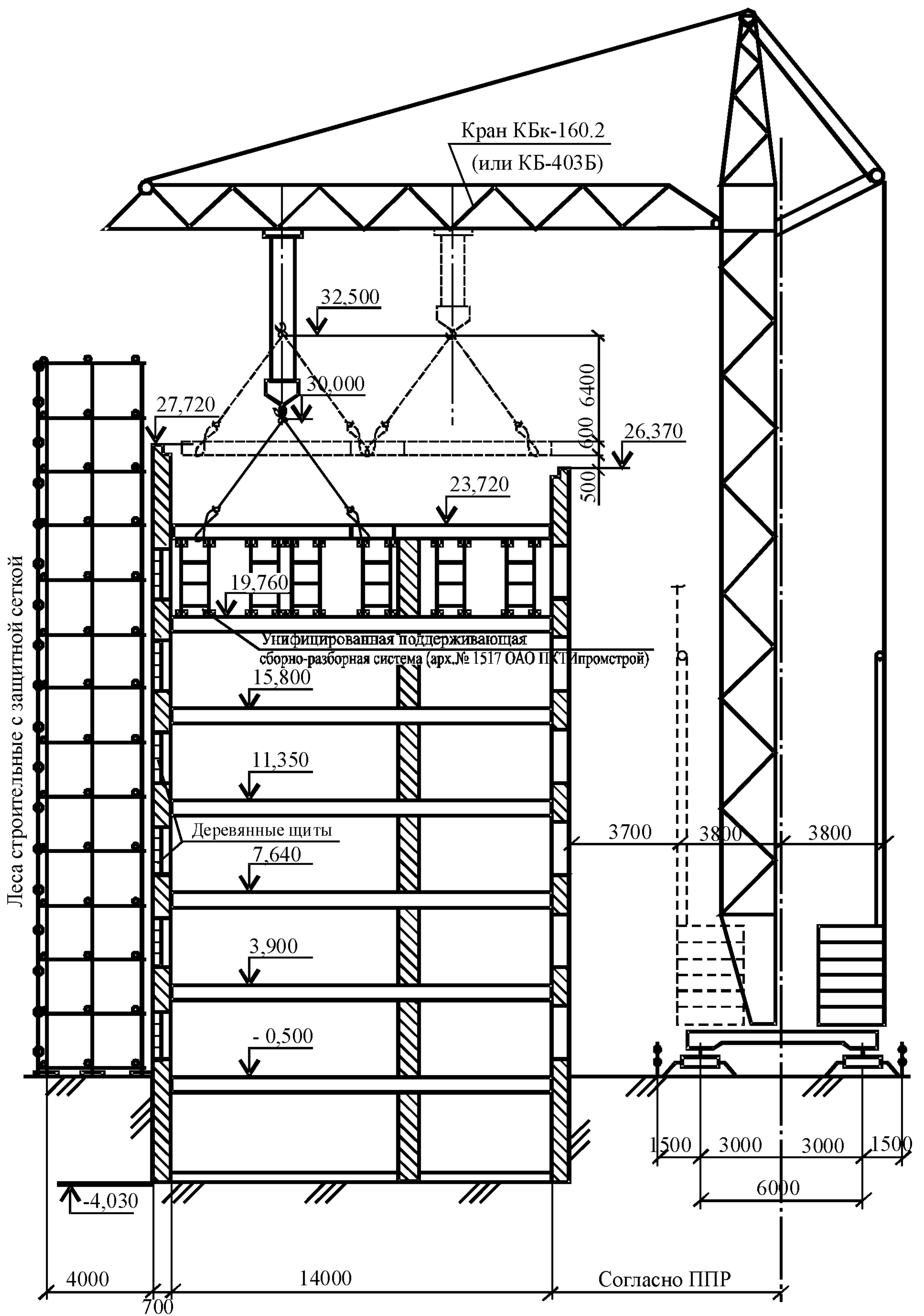
Рисунок 6 – Схема привязки крана на период разборки перекрытий
