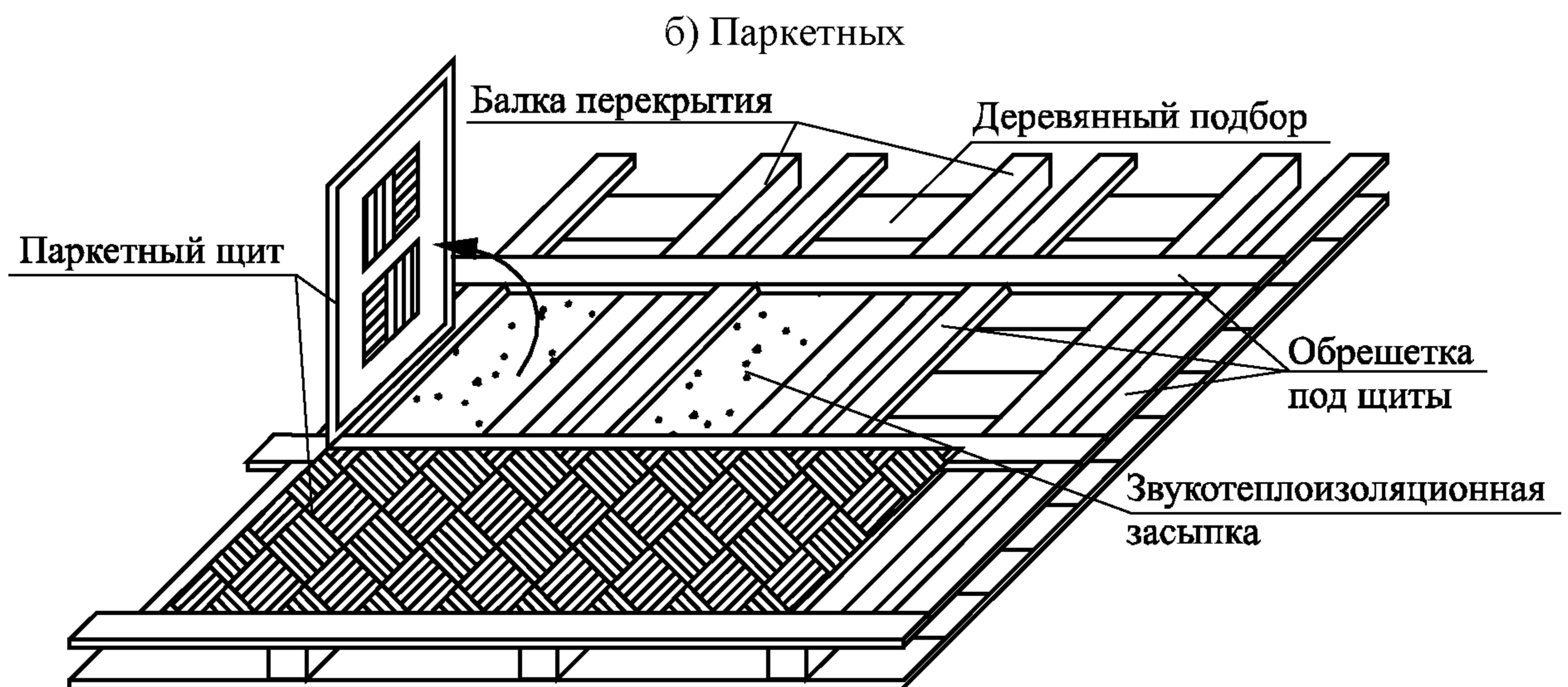
Рисунок 2 – Схема разборки чистых полов и лаг
