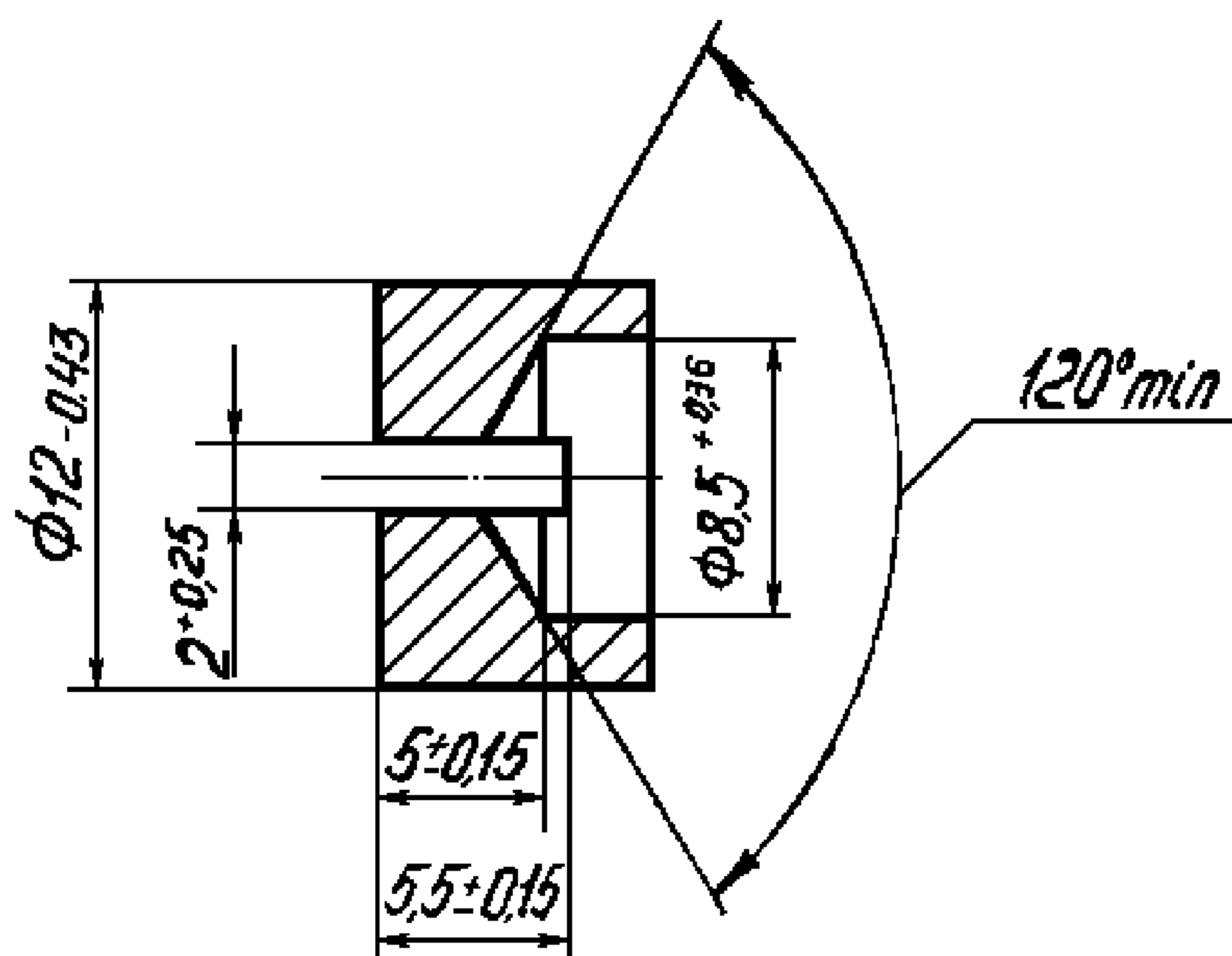
Рисунок А.1 — Насадок-распылитель
