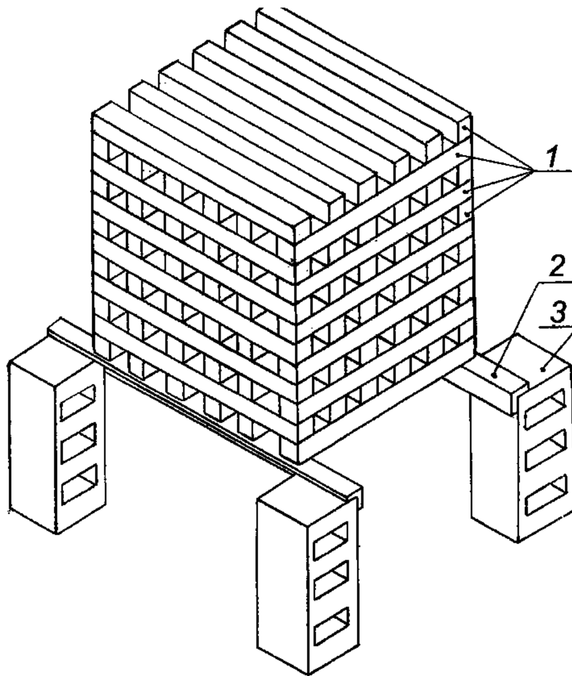
1 — деревянные бруски; 2 — стальной уголок; 3 — бетонный (металлический) блок
