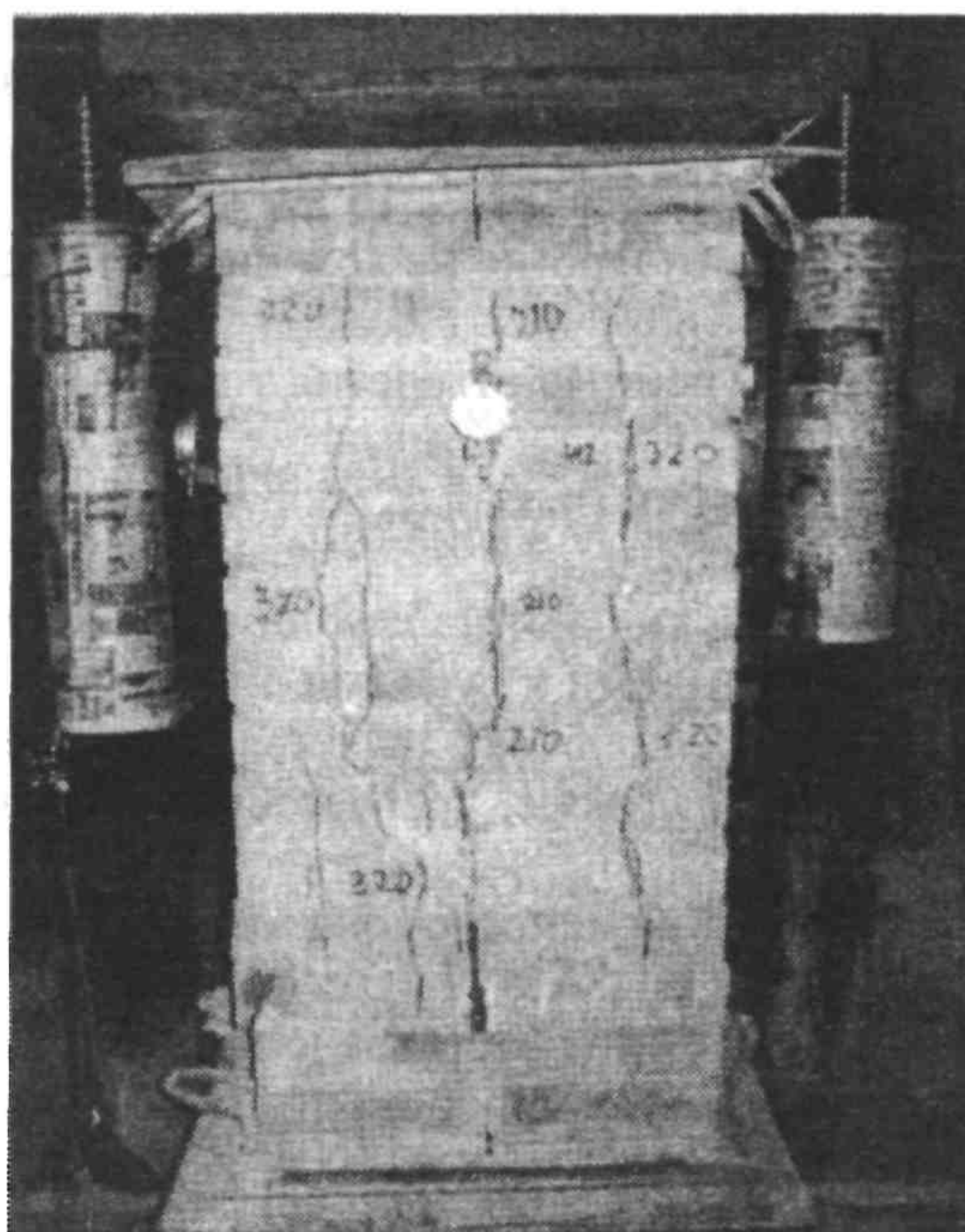
Рисунок 1 — Кирпичная кладка с множественными силовыми трещинами
