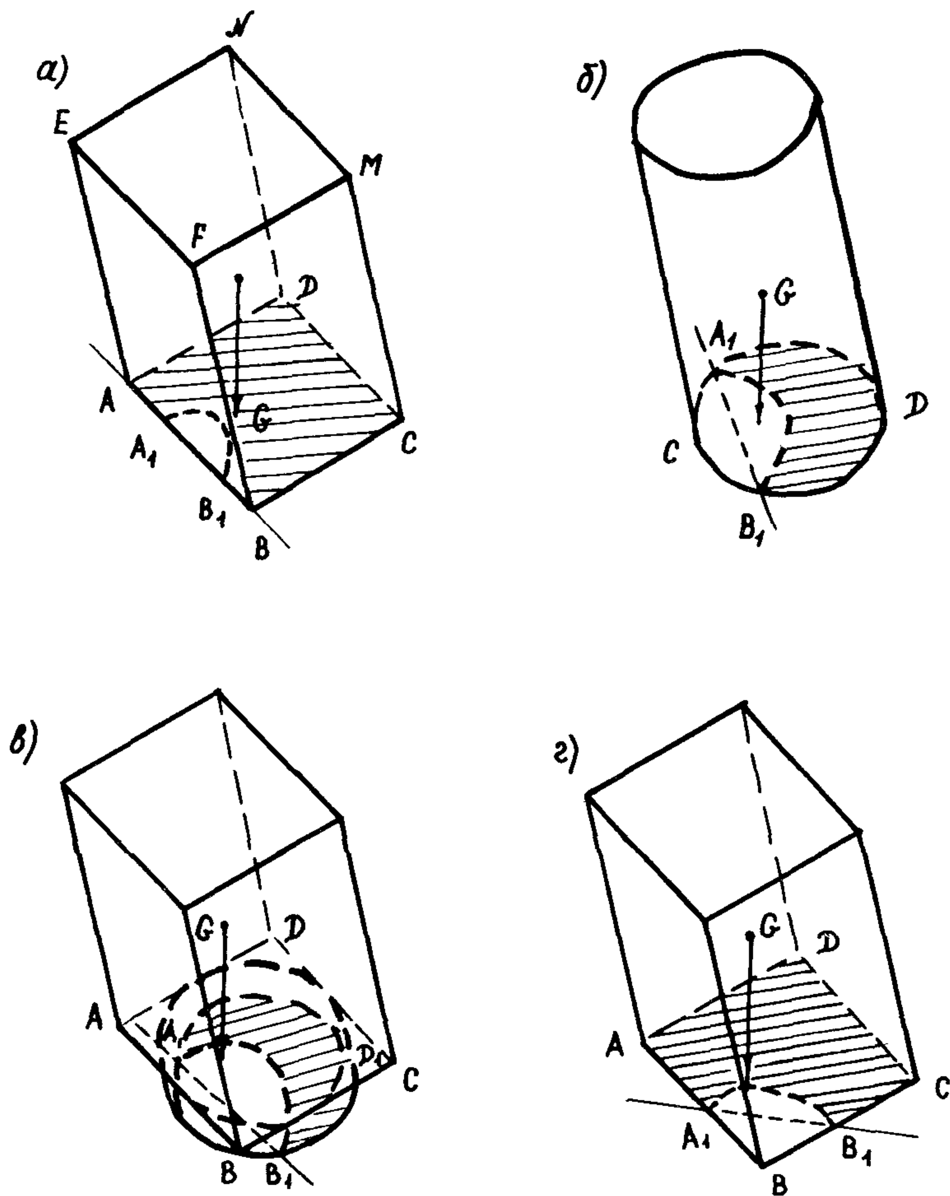
Рис.16. Устойчивость сооружений при образовании карстовых воронок: а – воронка под серединой стороны прямоугольного сооружения; б – воронка под круглым в плане сооружением; в – воронка под прямоугольным сооружением с круглой в плане цокольной частью; г – воронка под углом прямоугольного здания
