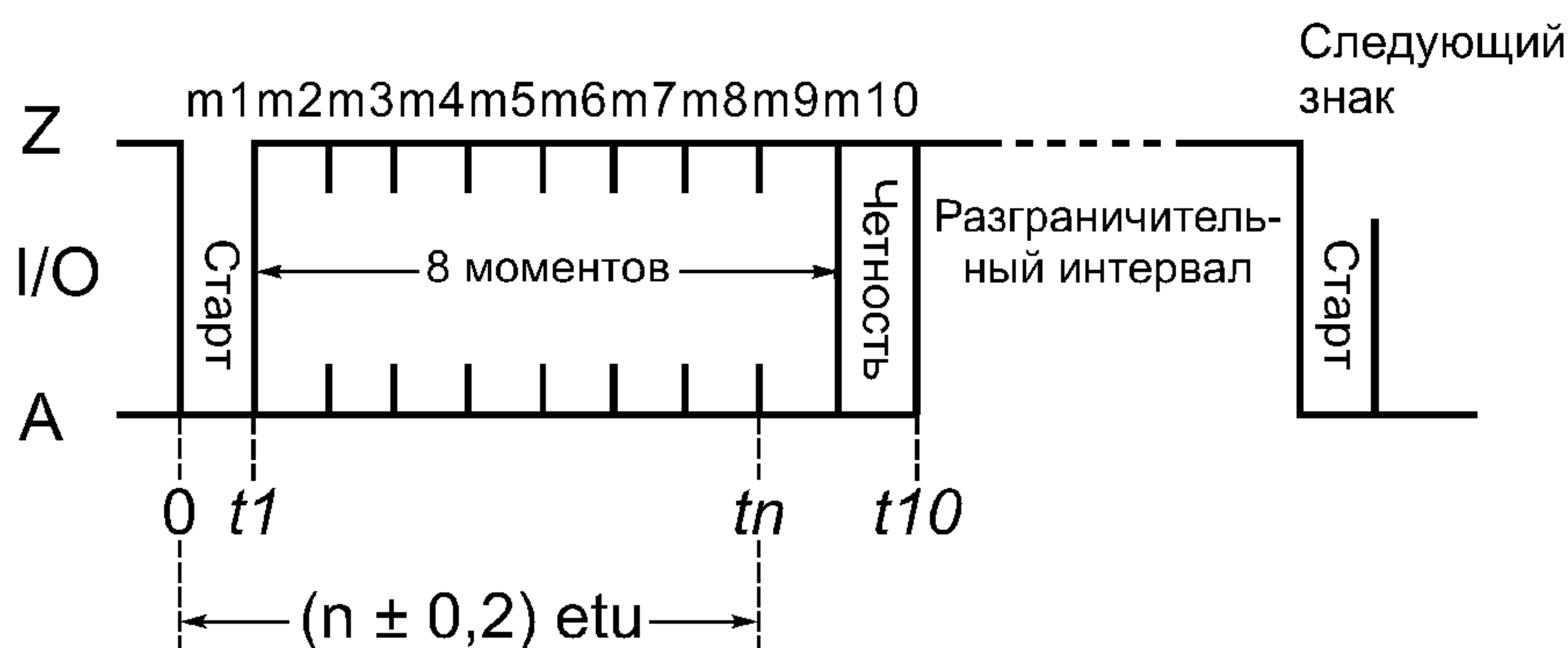
Рисунок 7 — Структура знака
