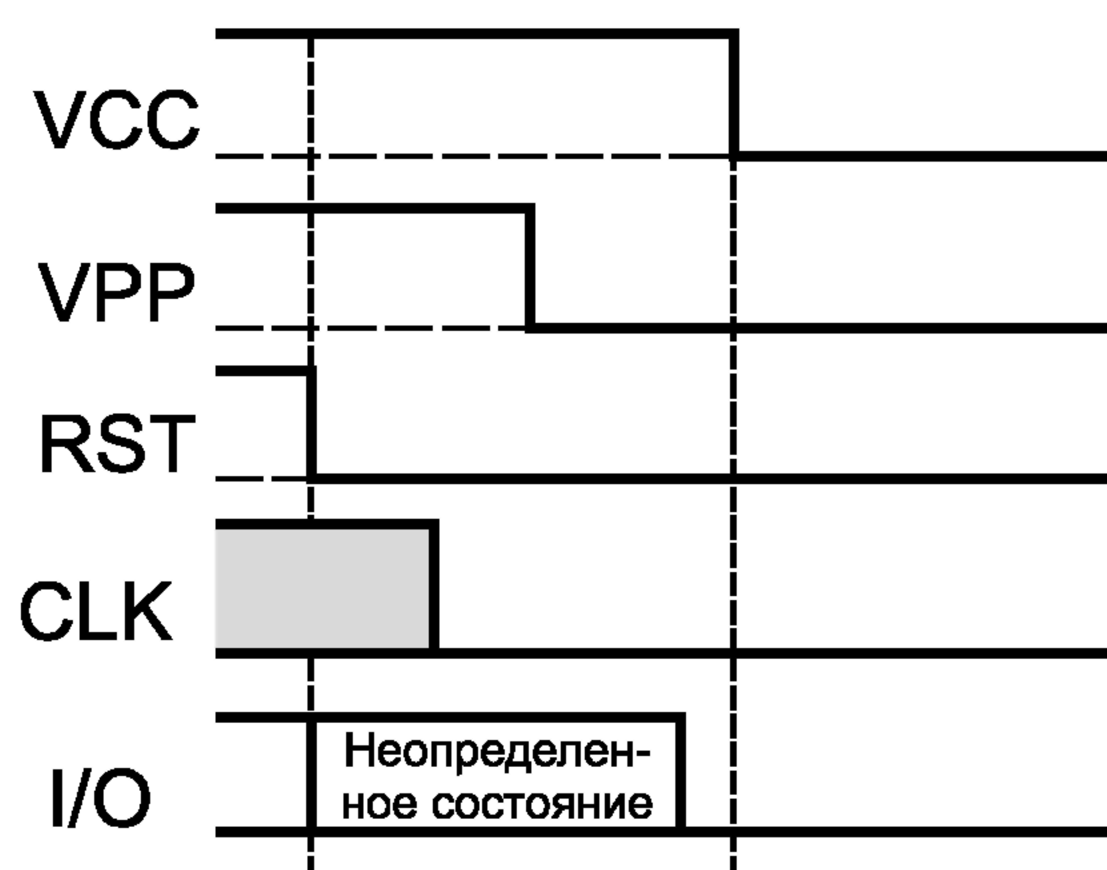
Рисунок 5 — Деактивизация
