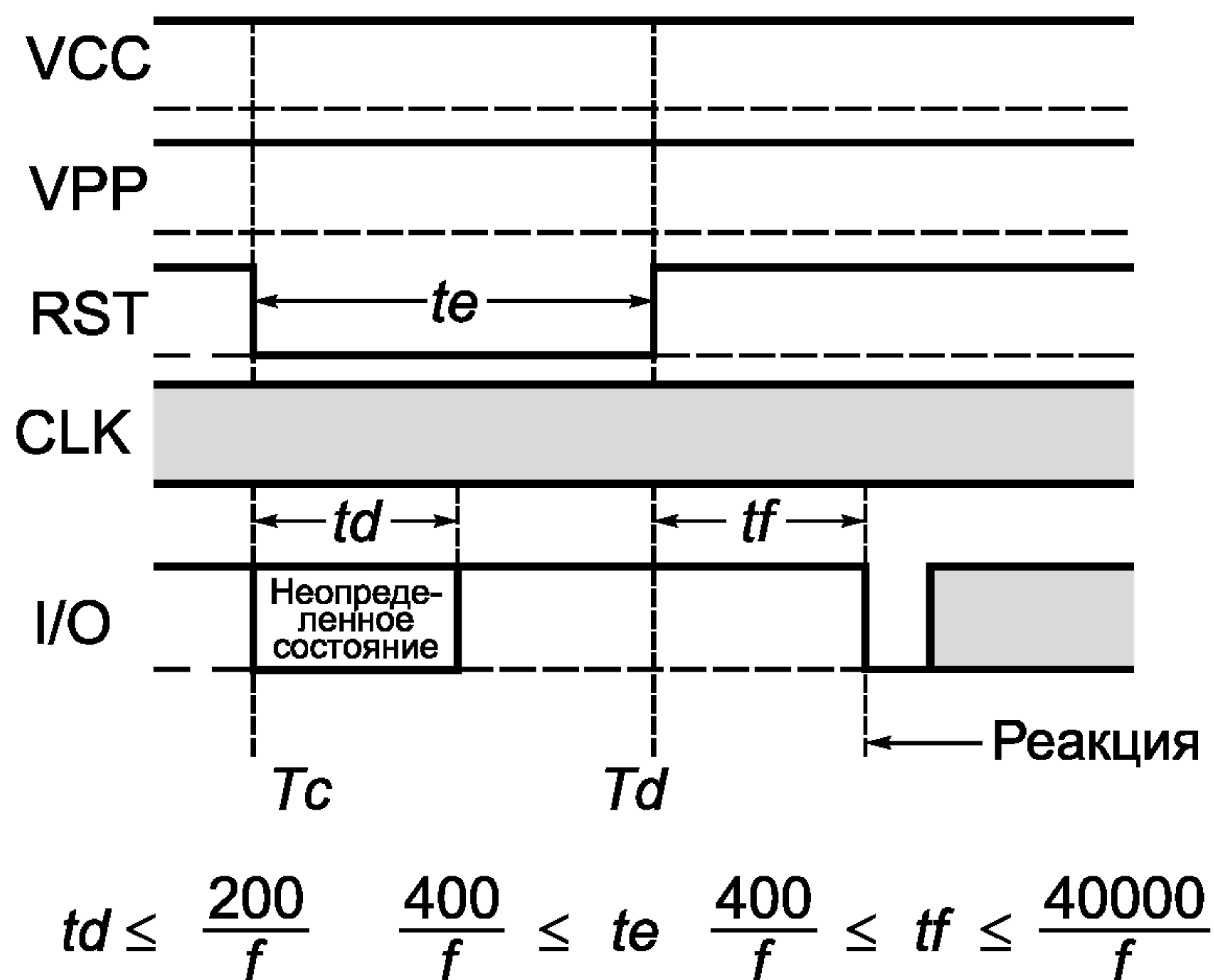
Рисунок 3 — «Горячее» восстановление
