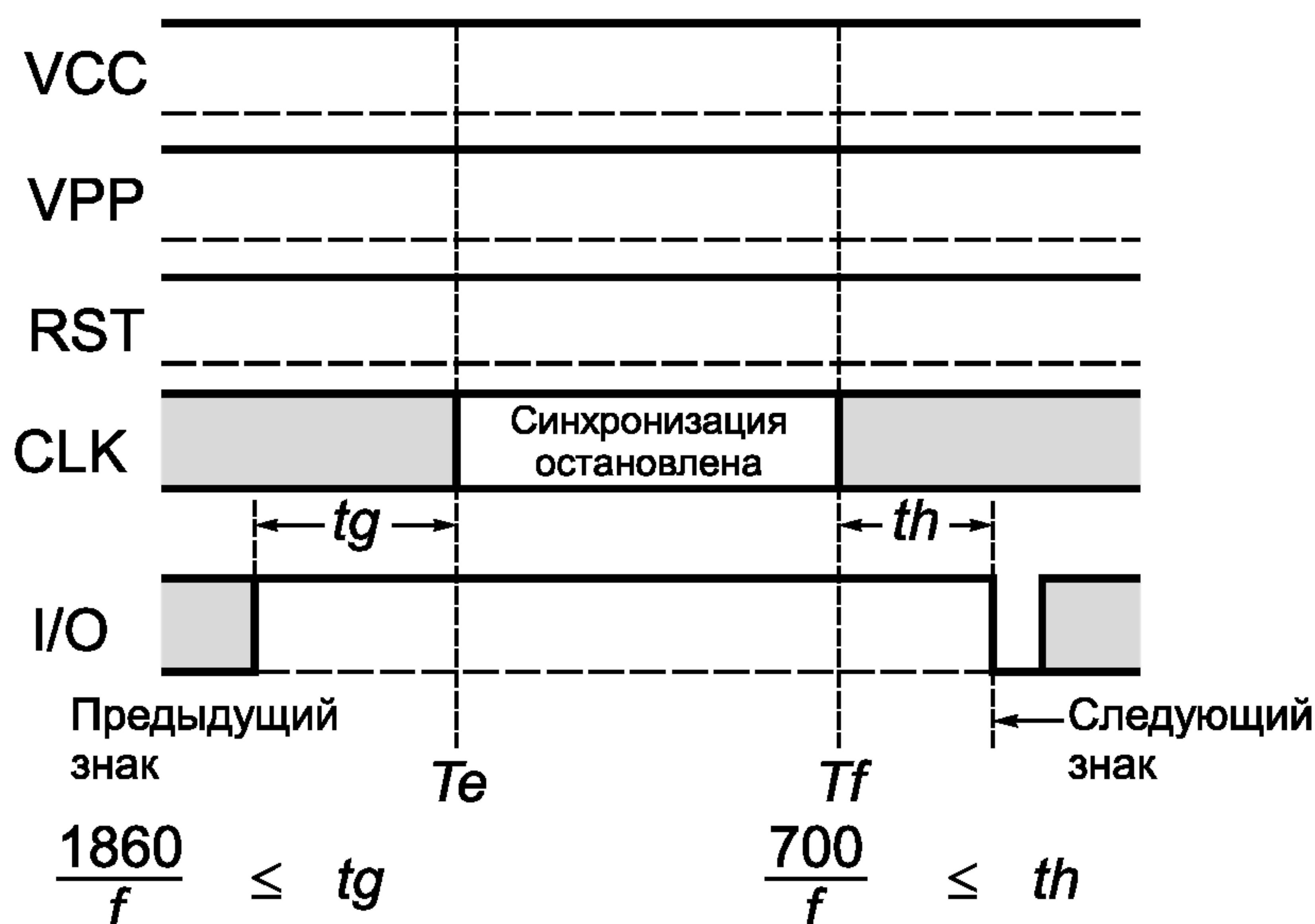
Рисунок 4 — Остановка синхронизации
