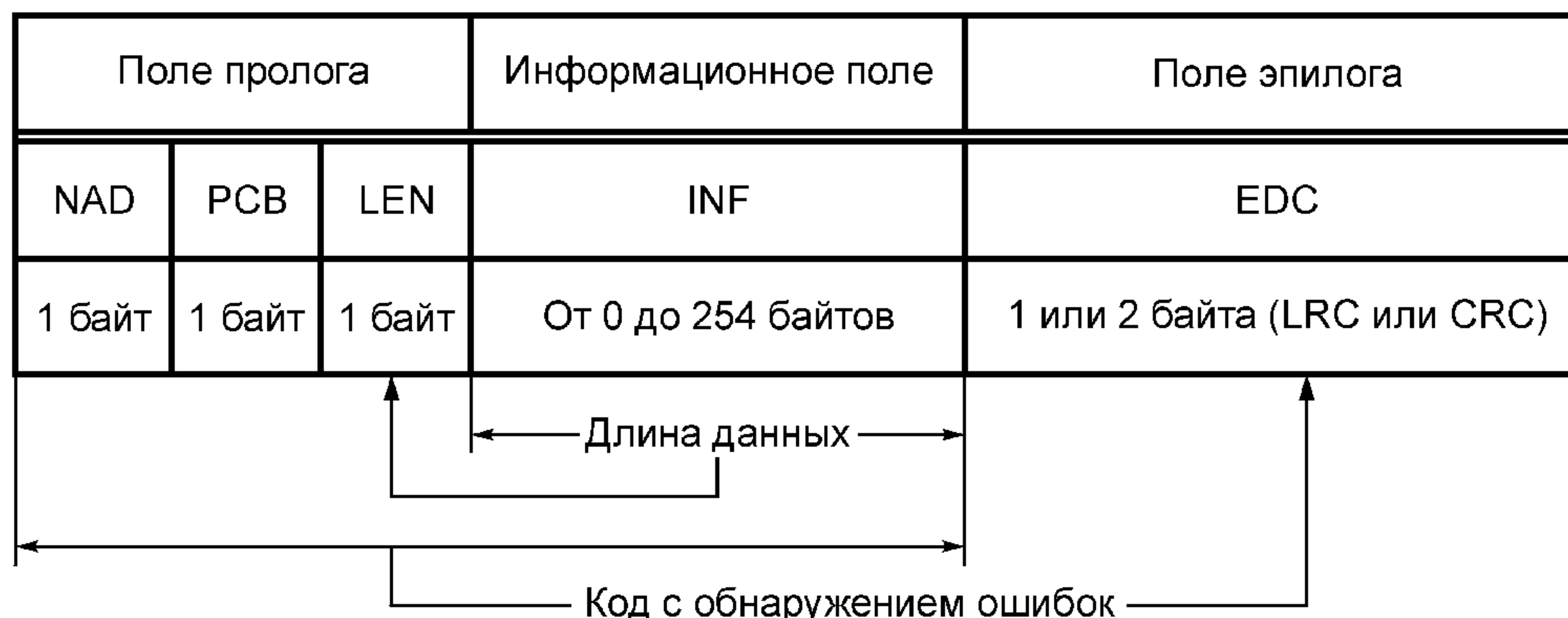
Рисунок 16 — Структура блока
