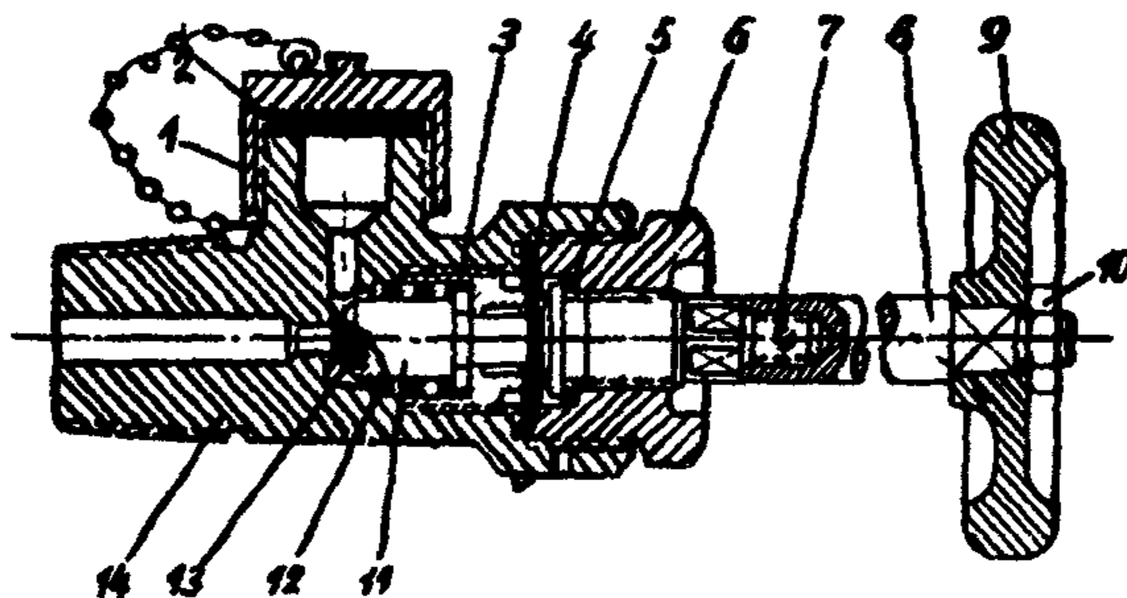
Рис. 4.3 Наполнительный вентиль
