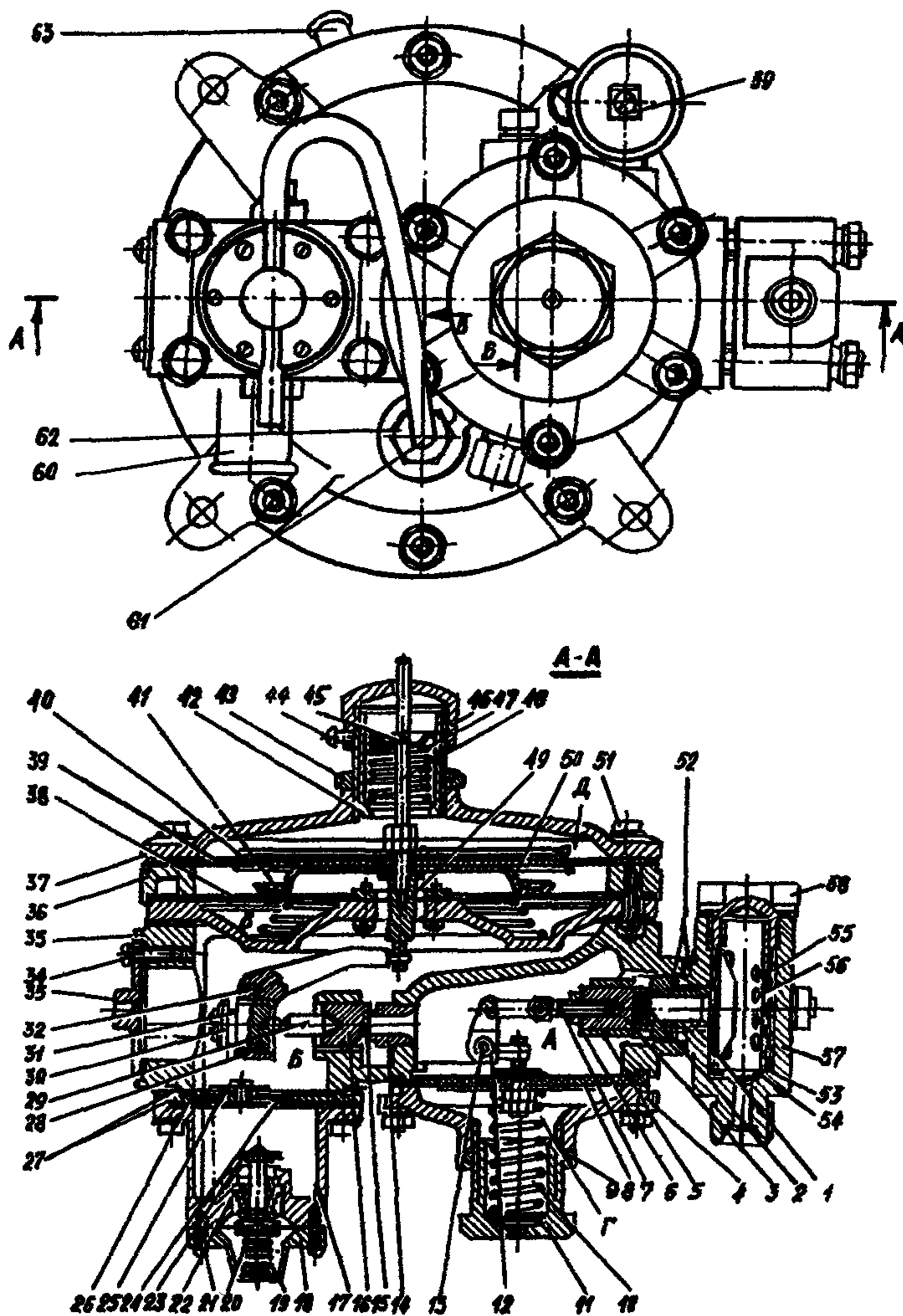
Рис. 4.8 Газовый редуктор низкого давления
