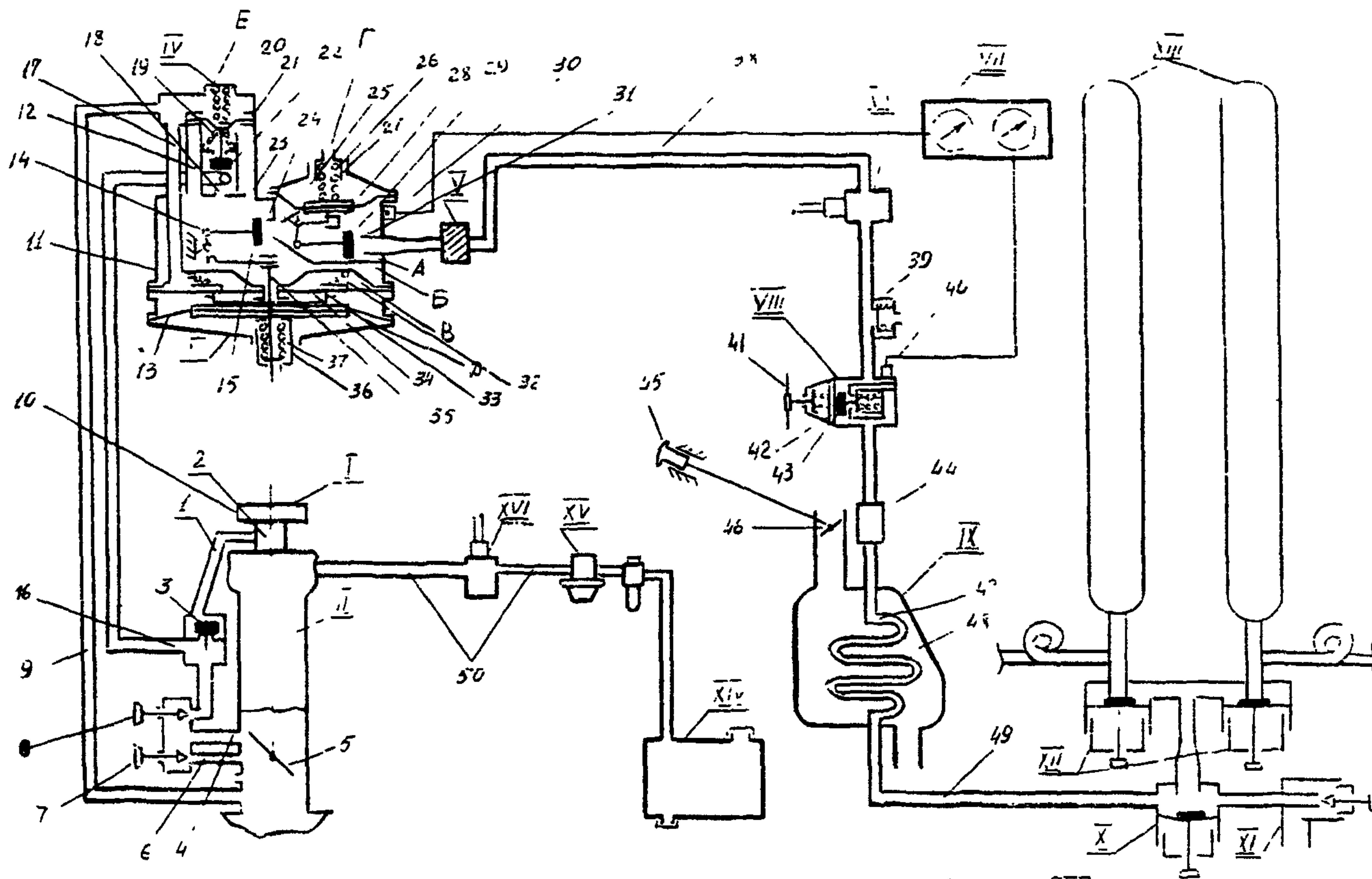
Рис. 5.1 Принципиальная схема работы системы питания автомобиля на СДГ
