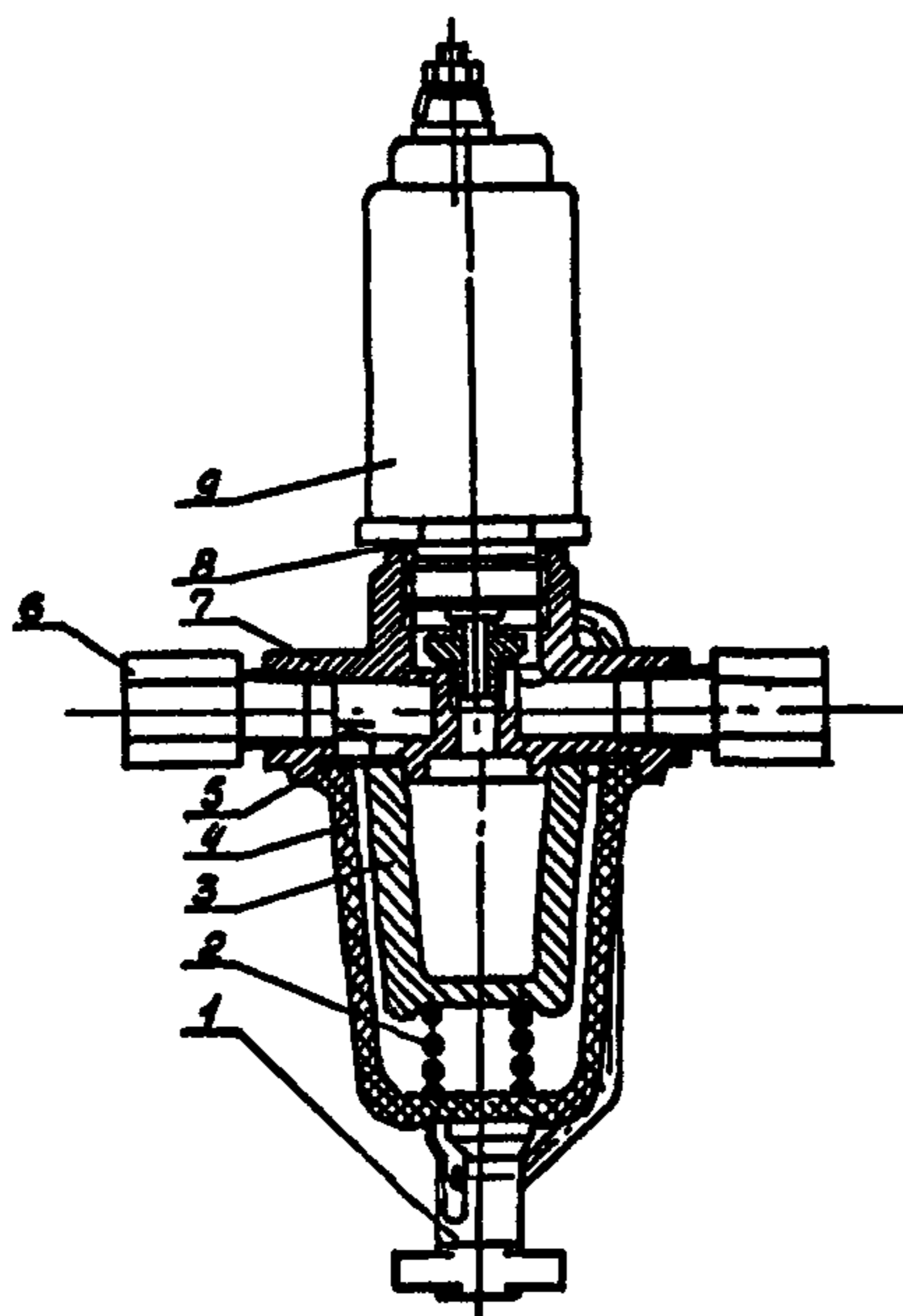
Рис. 4.13 Фильтр с электромагнитным клапаном
