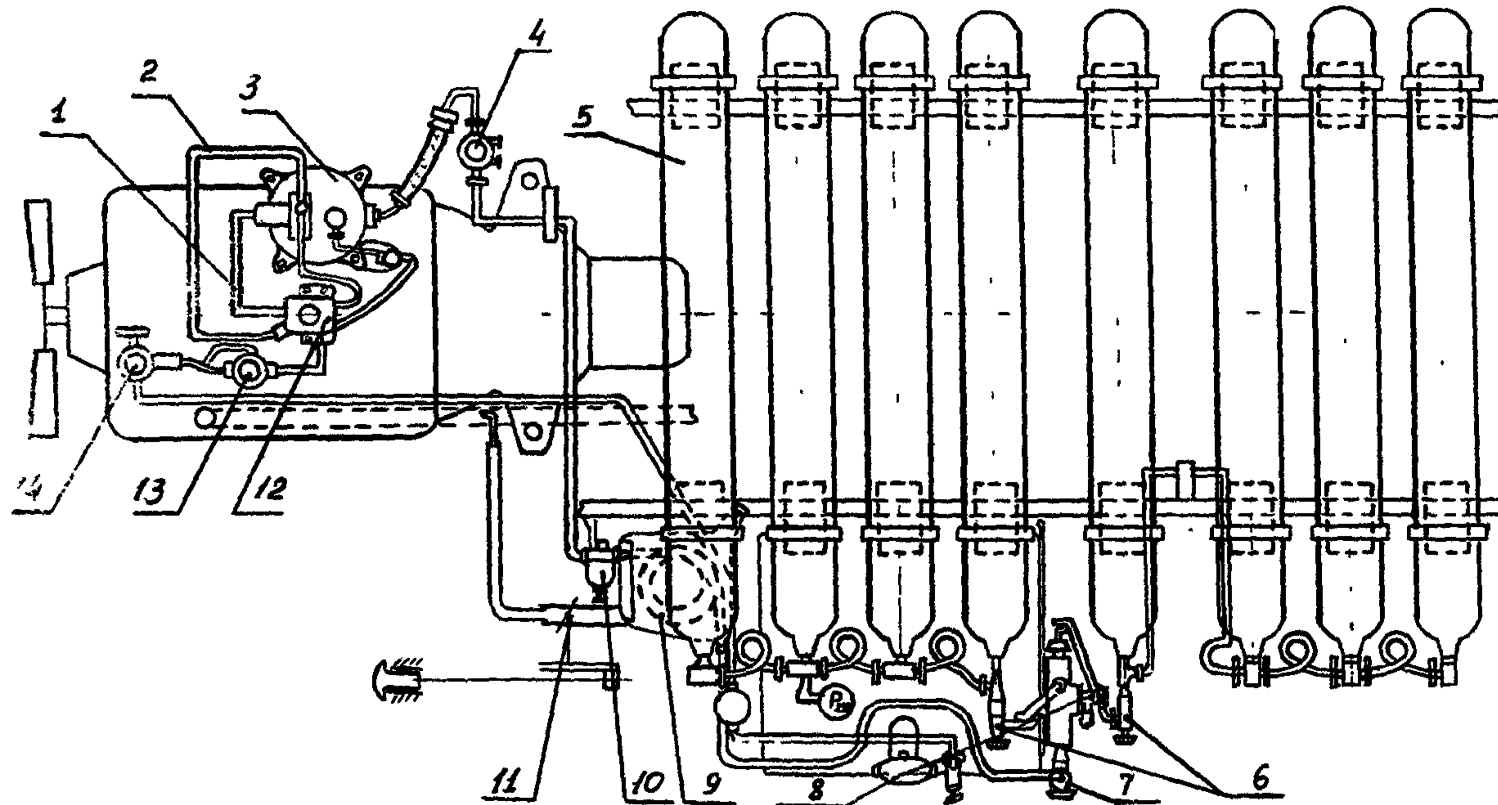
Рис.4.1 Схема газового оборудования автомобиля ЗИЛ-138А
