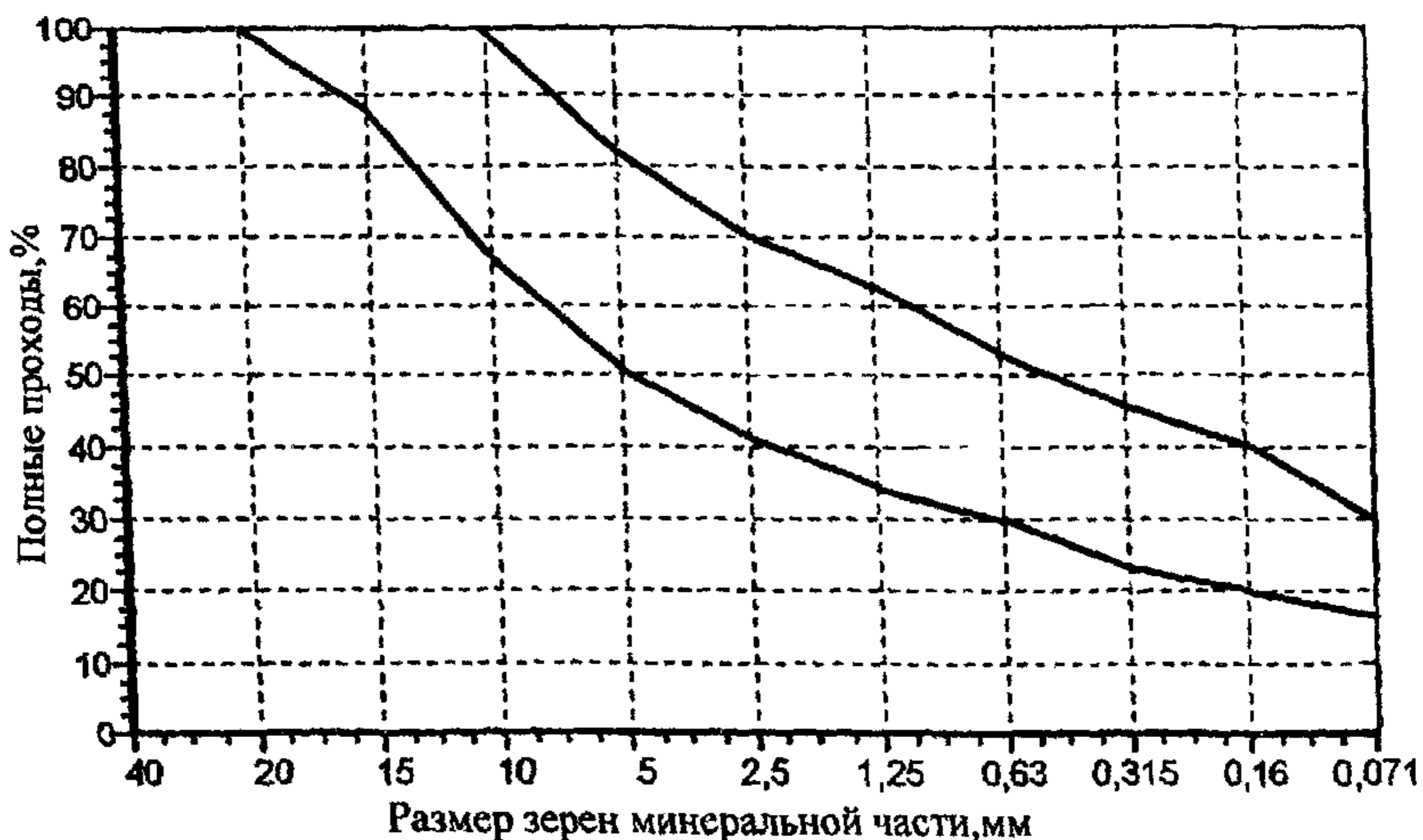
Рисунок 3. Зерновой состав минеральной части асфальтобетона литого типа на битумнорезиновом композиционном вяжущем для механизированной технологии укладки.
