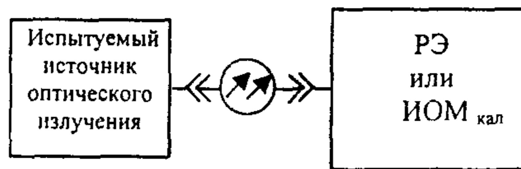
Рисунок 3 - Схема измерения мощности оптического излучения
