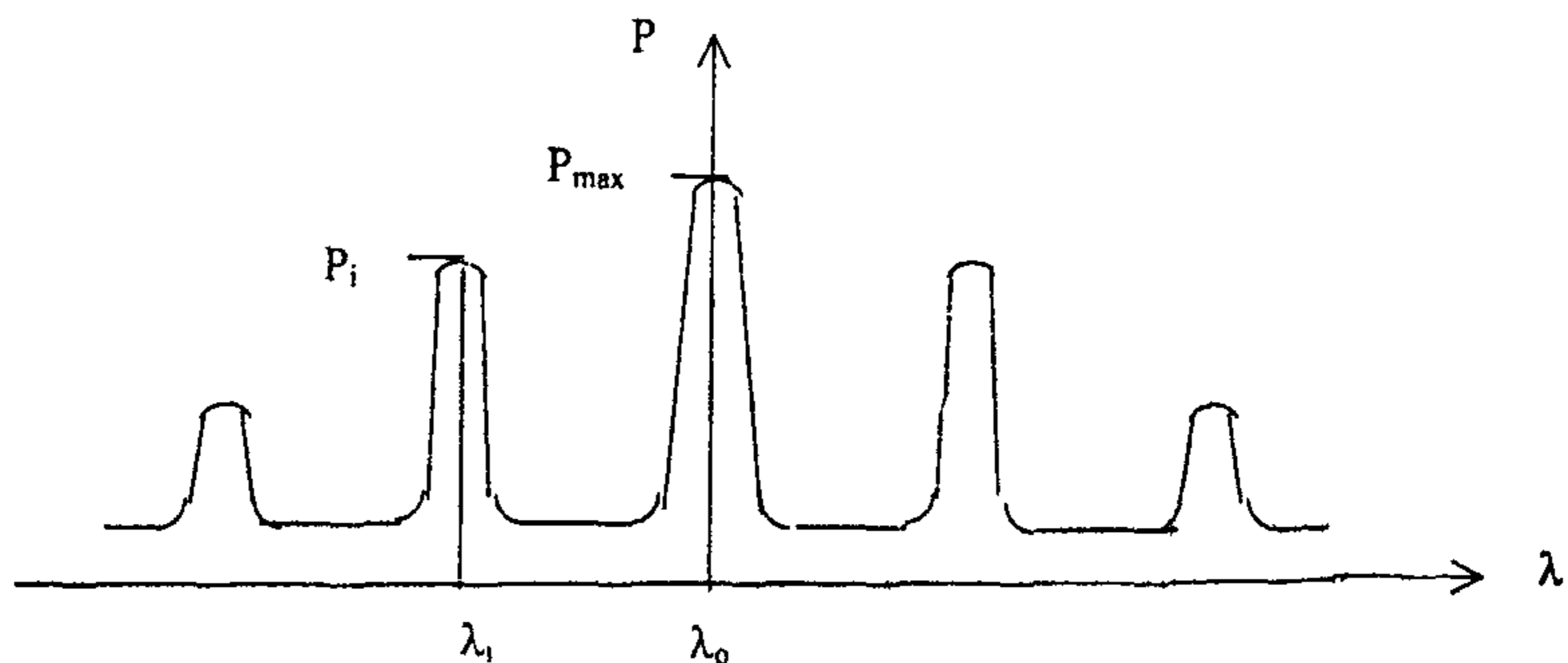
Рисунок 2 - Спектральное распределение мощности и принцип определения ширины спектра лазерного диода с многими продольными модам
